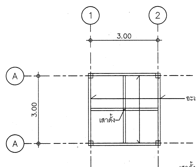
แปลนโครงสร้างชั้นหลังคา-1 มาตราส่วน 1:100
