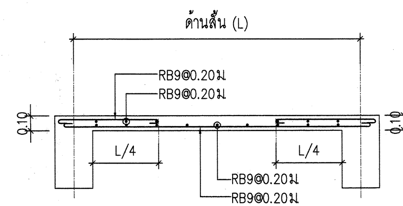
แบบขยายพื้น (SA) มาตราส่วน 1:100
