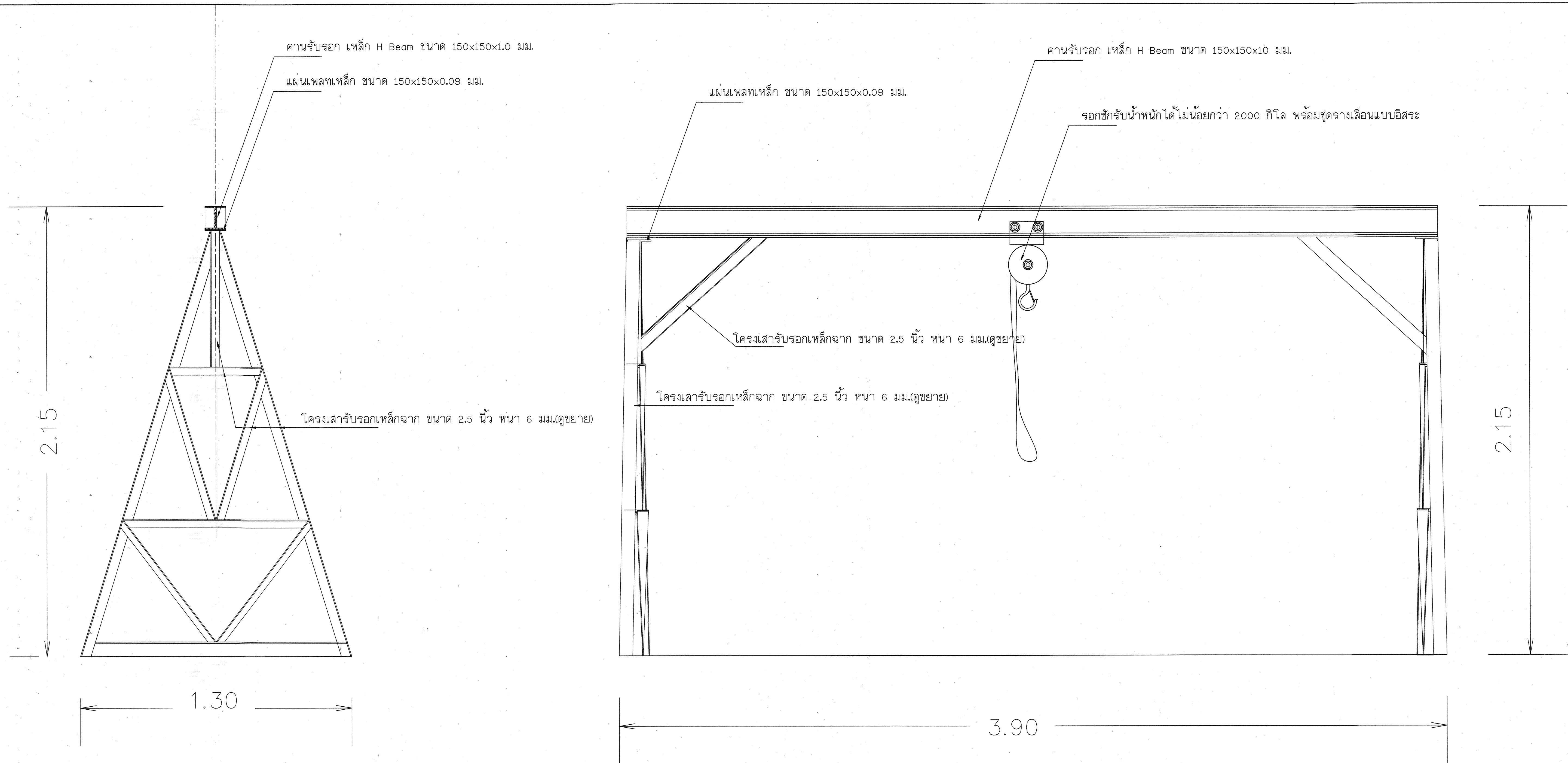
รูปตัดขยายชุดคานารอก มาตราส่วน 1 : 100
