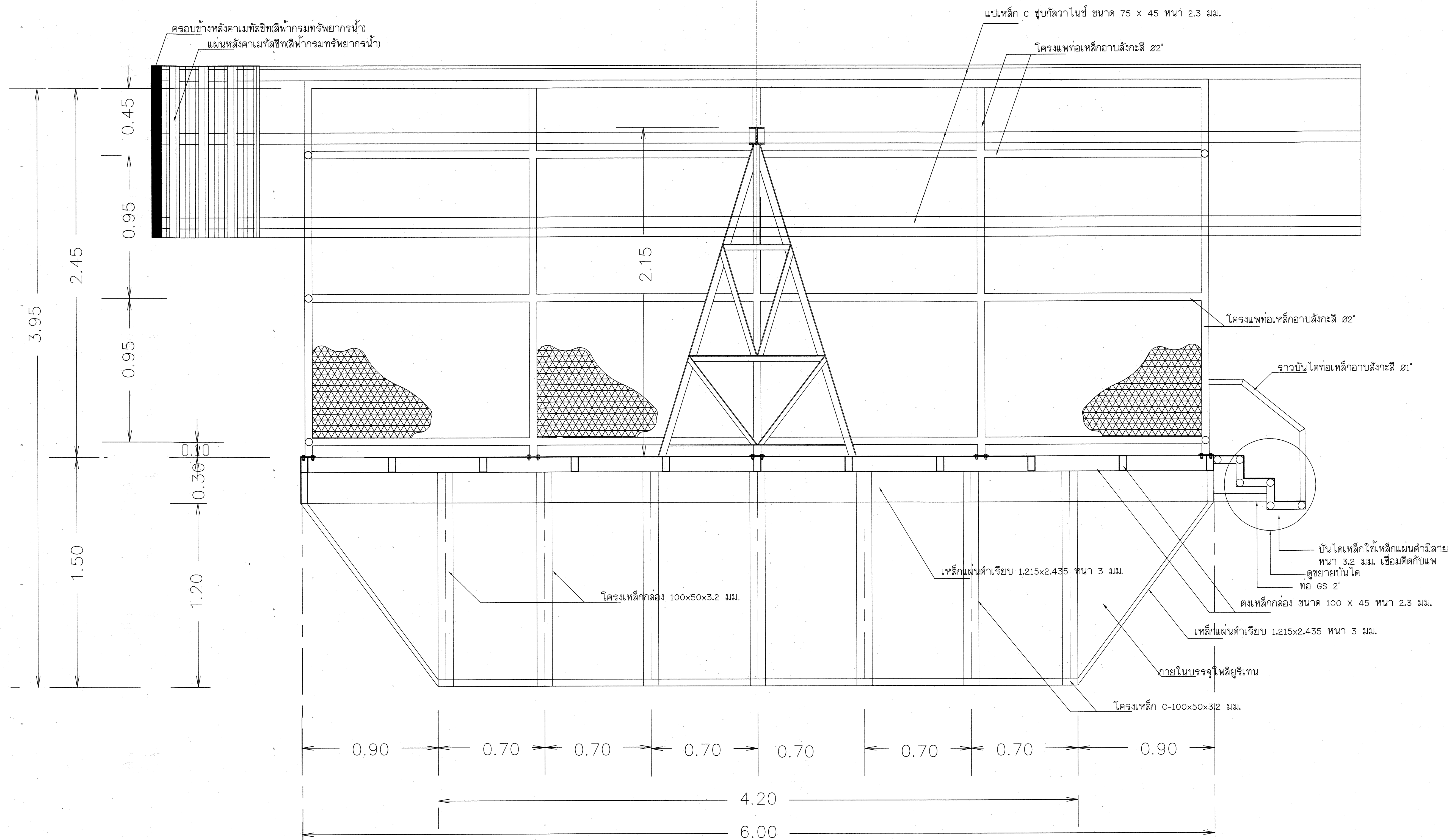
รูปตัดขยาย A - A มาตราส่วน 1:100
