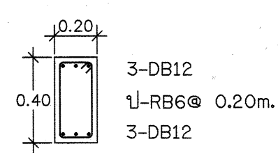
แบบขยายโครงสร้างคาน BA SCALE 1:100
