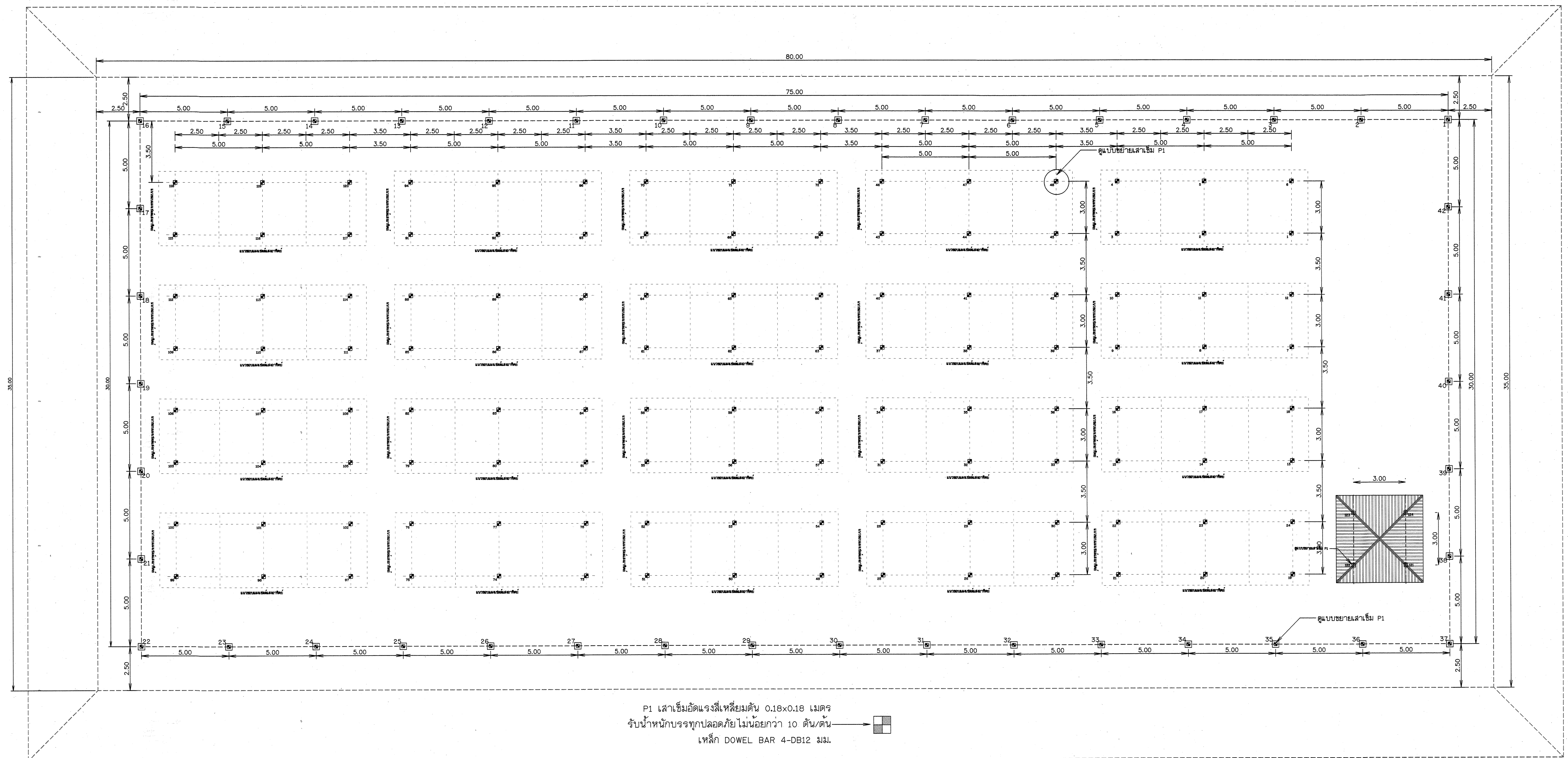
แบบแปลนเสาค้ำเข็ม
