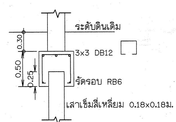
แบบขยายฐานรากอาคารควบคุม มาตราส่วน 1:100
