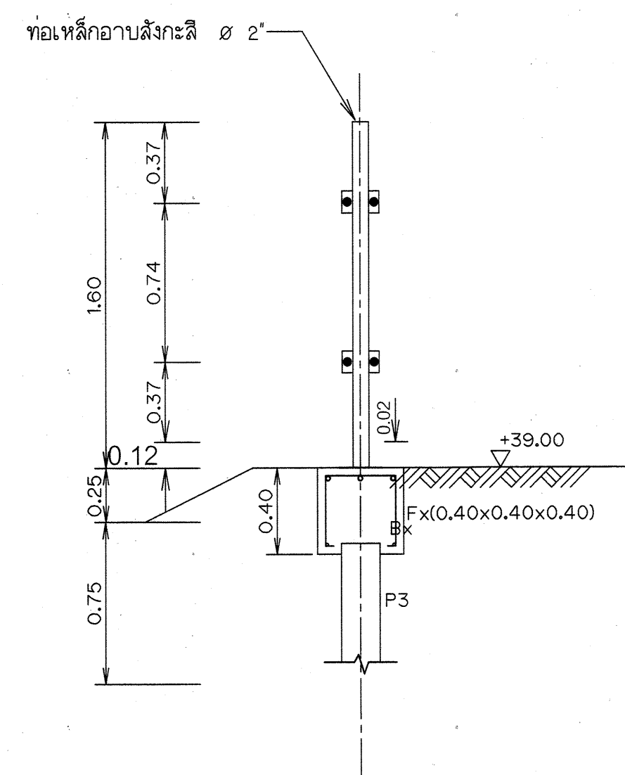
แบบขยายจั่ว (รูปด้านข้าง) มาตราส่วน 1:25
