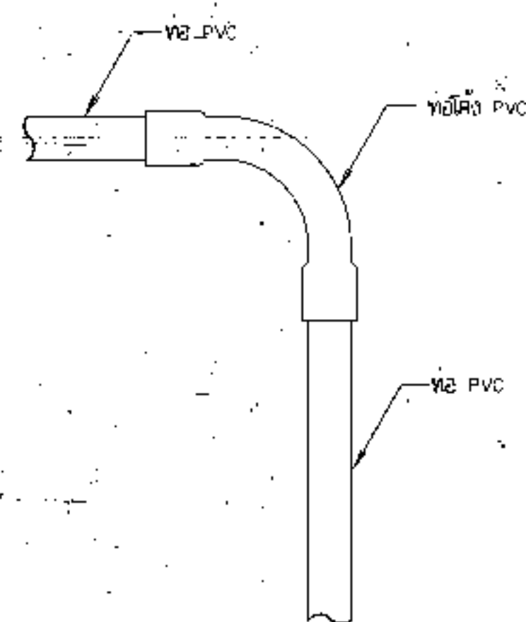
6. แบบการต่อข้อโค้ง 90° PVC ในแนวดิ่งตามขวาง
