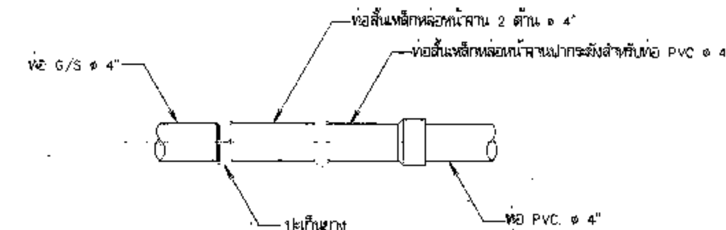
8. การบรรจบท่อเหล็กท่อน้ำกับท่อ PVC ในแนวดิ่งตามขวาง
