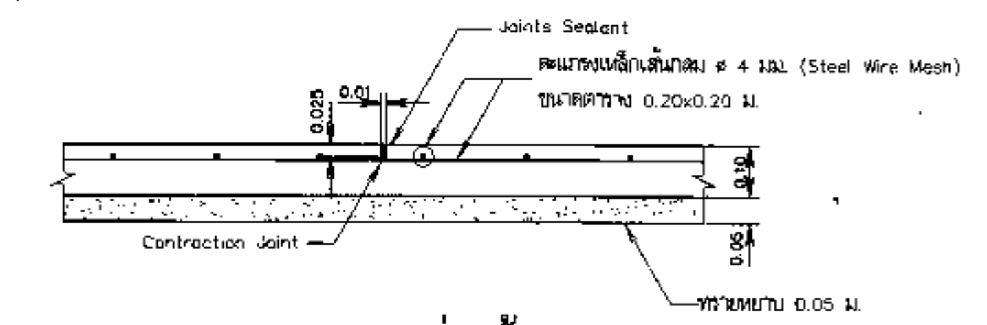
แบบขยายรอยต่อพื้น (Contraction Joint) โมเดลขนาดจริง
