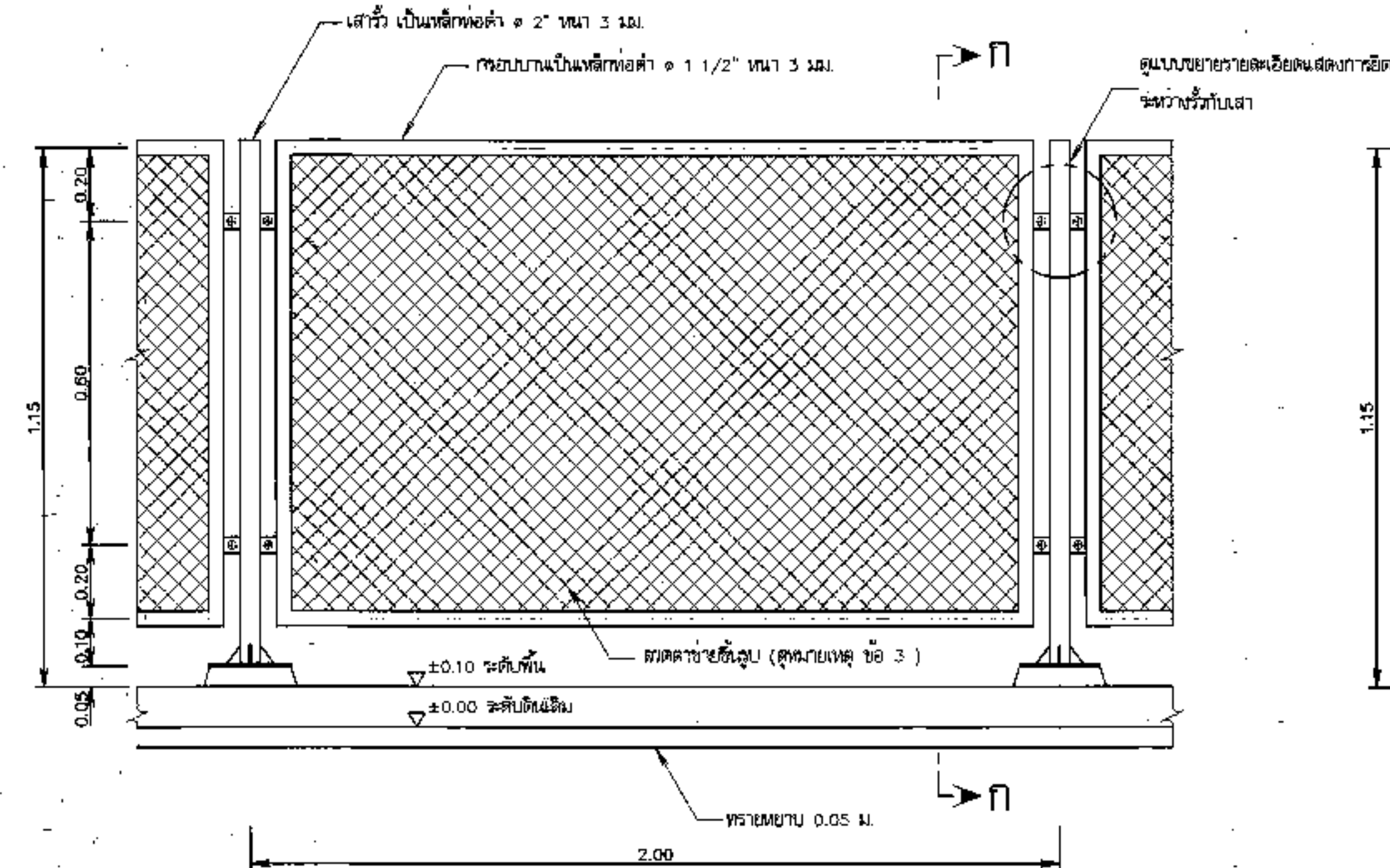
แบบขยายร้อยละตามชาย
