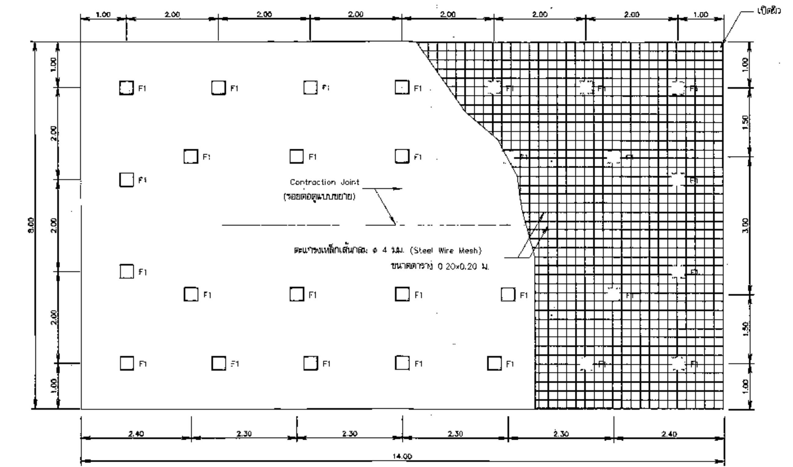
รูปขยายพื้นคอนกรีต
