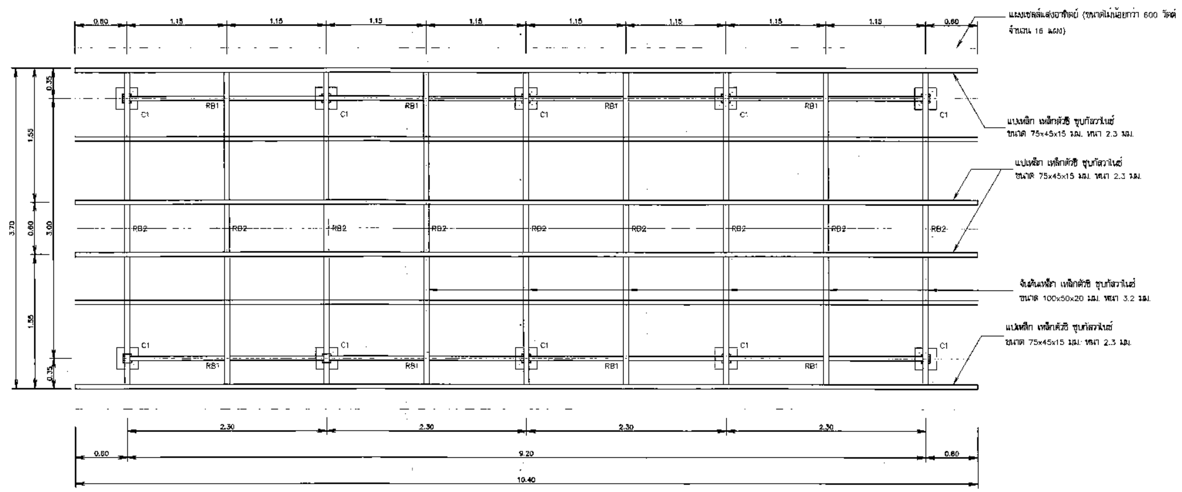
แปลนฐานรากและโครงสร้างหลังคา โมเดลขนาดจริง
