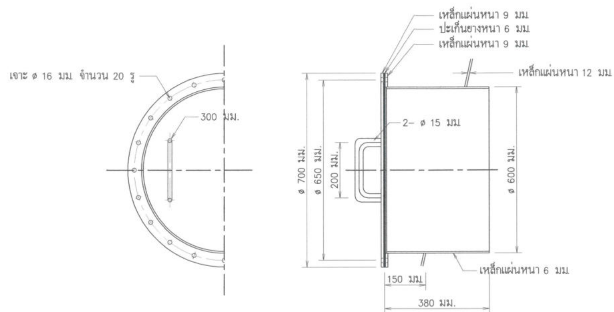
ภาพขยายทางคนเข้า-ออก "2"
