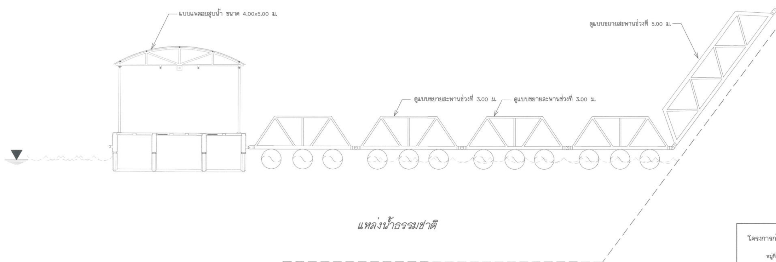
รูปด้านทางเชื่อมพลอยสูบน้ำ ไม่แสดงขนาดราวล้วน
