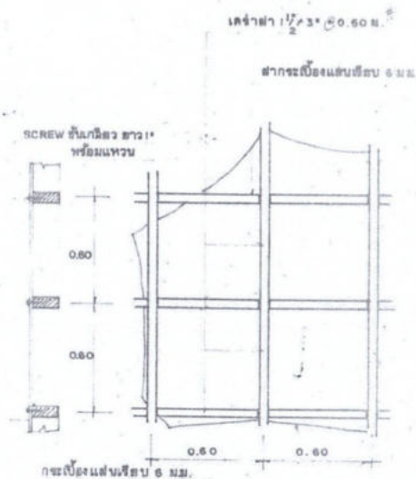
รูปขยายเจาะ, ฝา 1820
