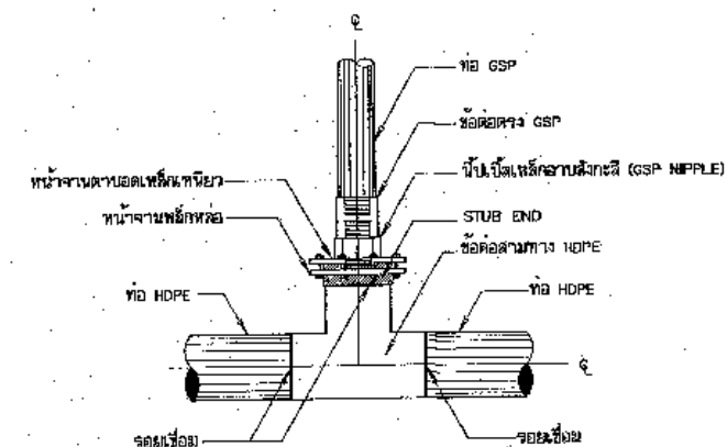
การบรรจุท่อสามทาง HDPE กับท่อ GSP แบบข้อต่อ (สำหรับอาคารจุดปล่อยน้ำ อาคารประสูตระบายกลิ่น อาคารระบายอากาศ กรณีท่อส่งน้ำขนาดเล็กมีขนาดเส้นผ่าศูนย์กลางมากกว่า 315 มม.)
