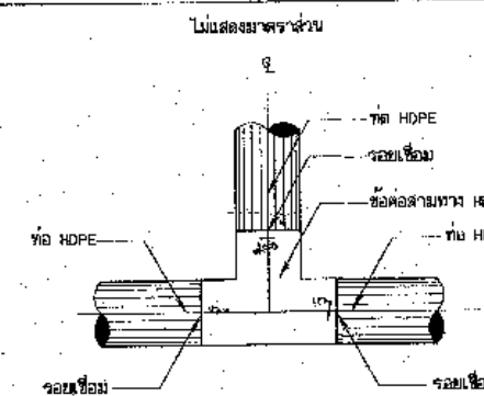
การบรรจุท่อสามทาง HDPE กับท่อ HDPE ไม่แสดงขนาดส่วน
