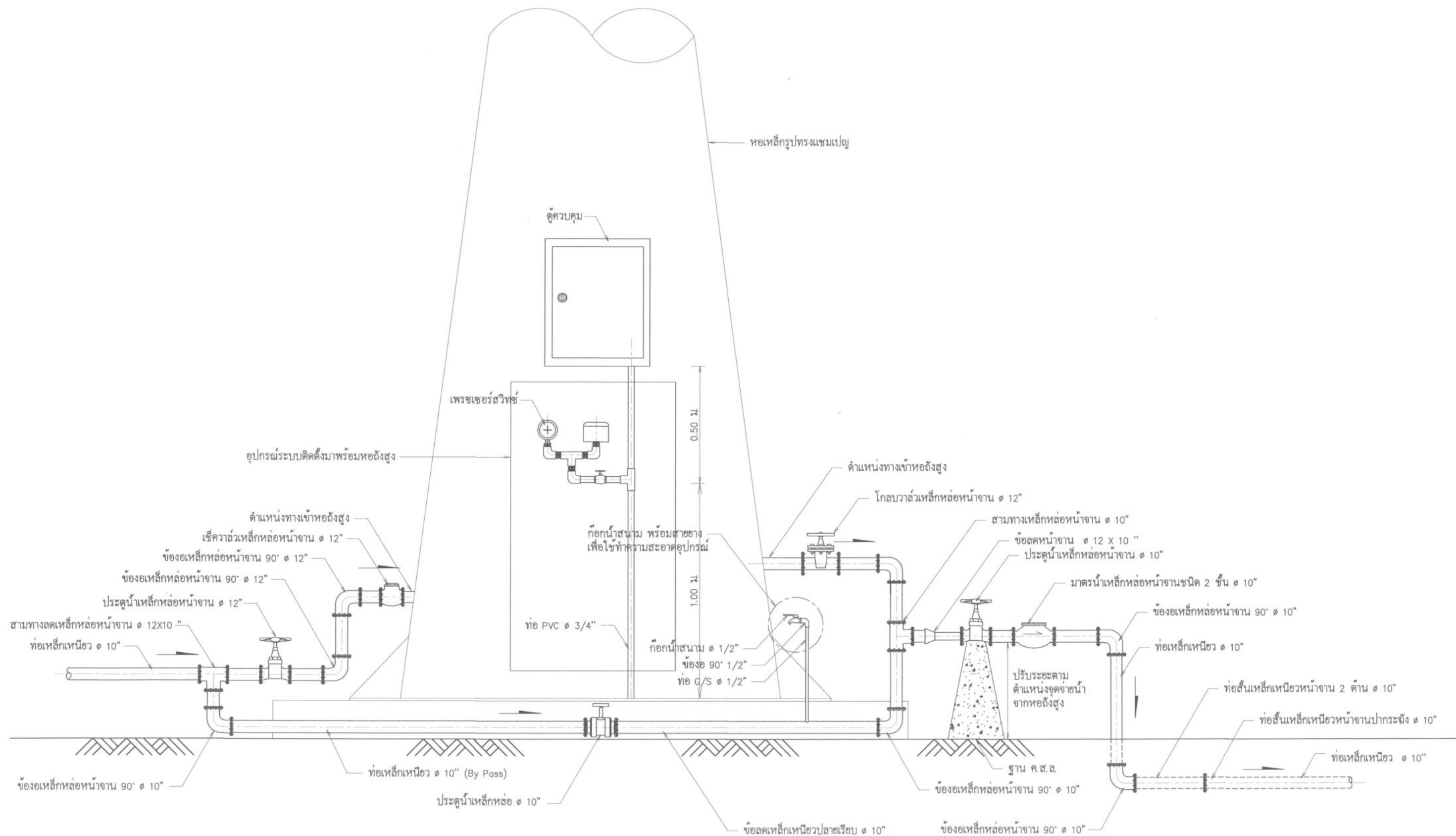
รูปแสดงรายละเอียดการต่อท่อและอุปกรณ์ออกจากถังเหล็กรูปทรงกลมแป้น ไม่แสดงมาตราส่วน
