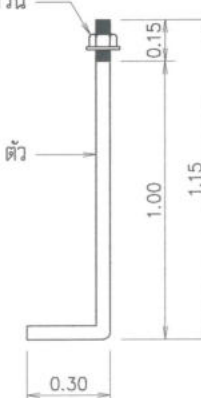
แบบขยายสลักเกลียวยึดฐาน
