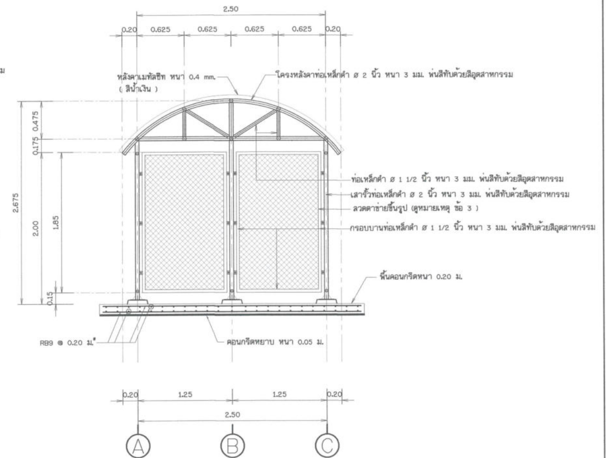
รูปตัด ข - ข ไม่แสดงขนาดบางส่วน
