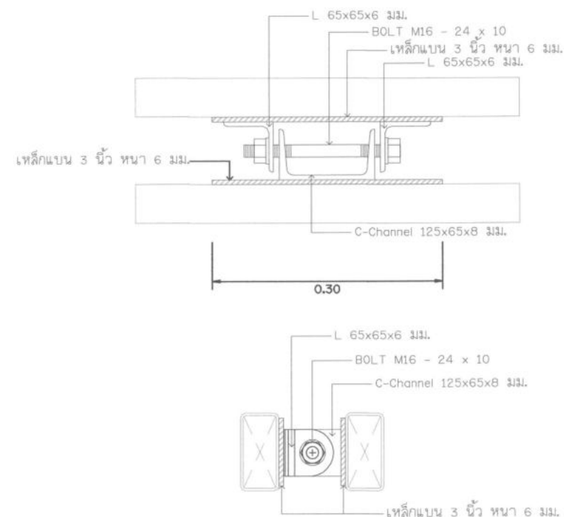
แบบขยายตัวเชื่อม มาตราส่วน 1 : 100
