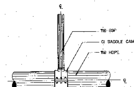
การบรรจุท่อสามทาง HDPE กับท่อ GSP แบบ CI SADDLE CLAMP (สำหรับอาคารจุดปล่อยน้ำ อาคารประสูตระบายกลิ่น อาคารระบายอากาศ กรณีท่อส่งน้ำขนาดเล็กมีขนาดเส้นผ่าศูนย์กลางน้อยกว่าหรือเท่ากับ 315 มม.)
