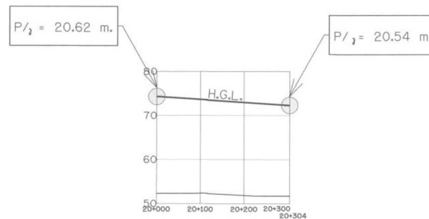
รูปตัดตามแนวยาวแสดง H.G.L. กม. 20+000
