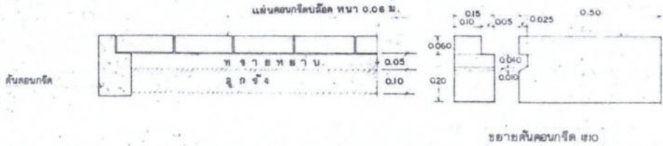
รูปขยายการเรียง I-SECTION 1:10
