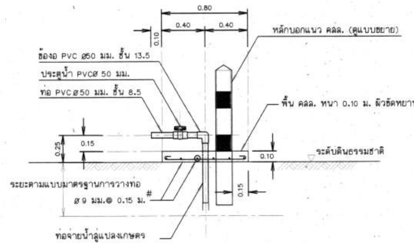
รูปตัด ก - ก แล่งการติดตั้งอาคารจุดปล่อยน้ำ มาตราส่วน 1:20
