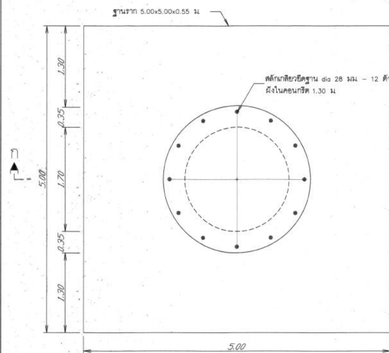
แปลน จานรากหอถึงสูง (แบบจานแผ่)
