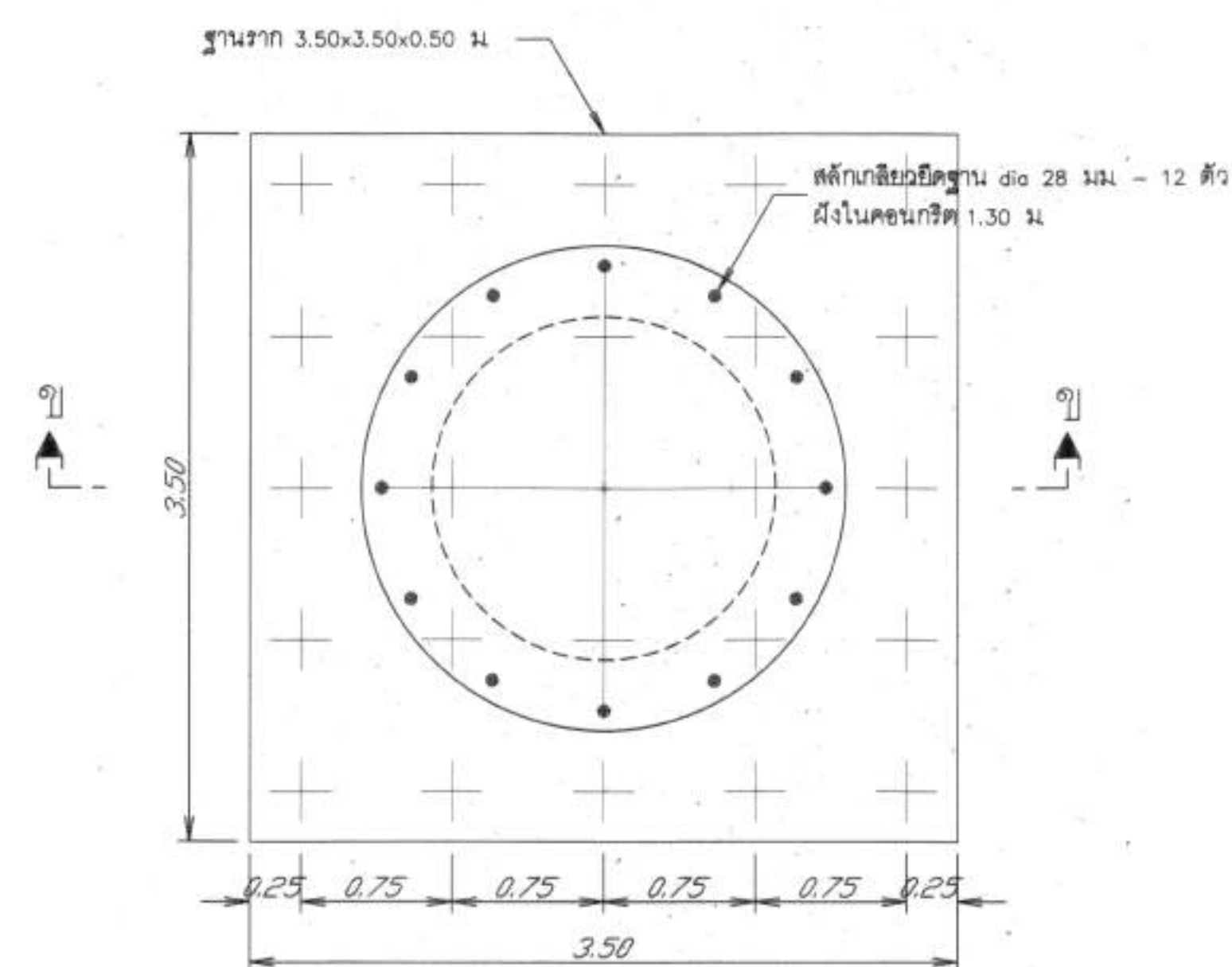
แปลน จานรากหอถึงสูง (แบบเสาเข็ม)
