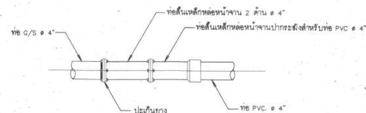
8. การบรรจุท่อเหล็กท่อน้ำจืด G/S กับท่อ PVC. ไม่แสดงมาตราส่วน
