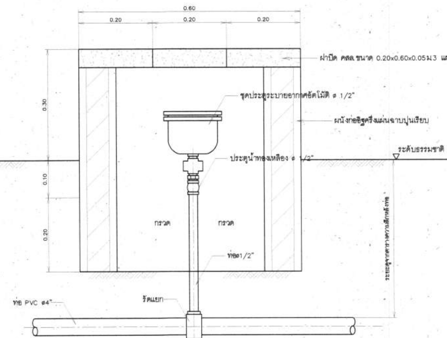
12 การติดตั้งประตูลอยอากาศอัตโนมัติ มาตราส่วน 1:5
