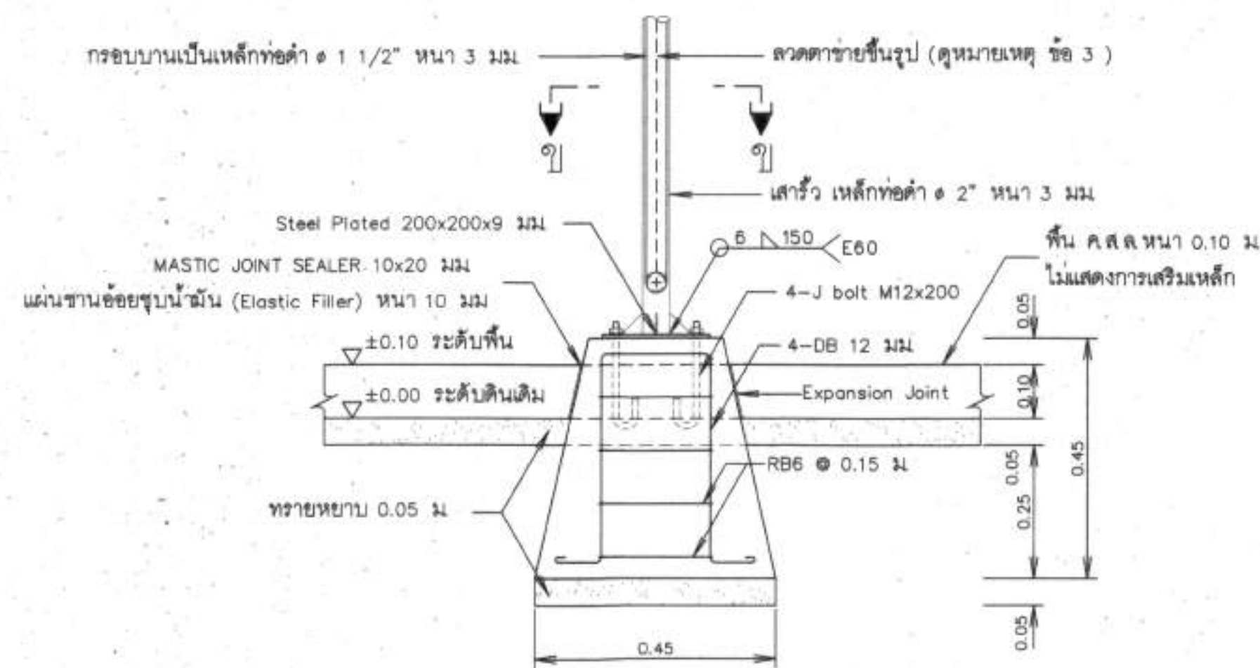
รูปขยายฐานจากโครงสร้างรับแรง F1 (ต่อม่อ คสล. หล่อสำเร็จรูปพร้อมติดตั้ง) ไม่แสดงมาตราส่วน
