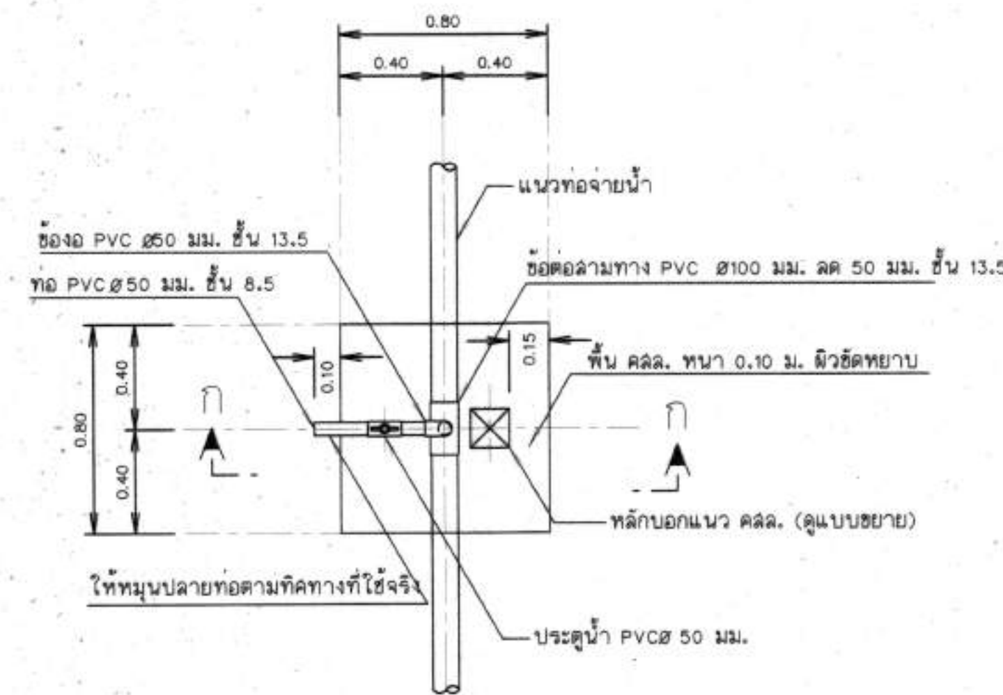
จำนวนตามใบปริมาณงาน แปลนอาคารจุดปล่อยน้ำ มาตราส่วน 1:20
