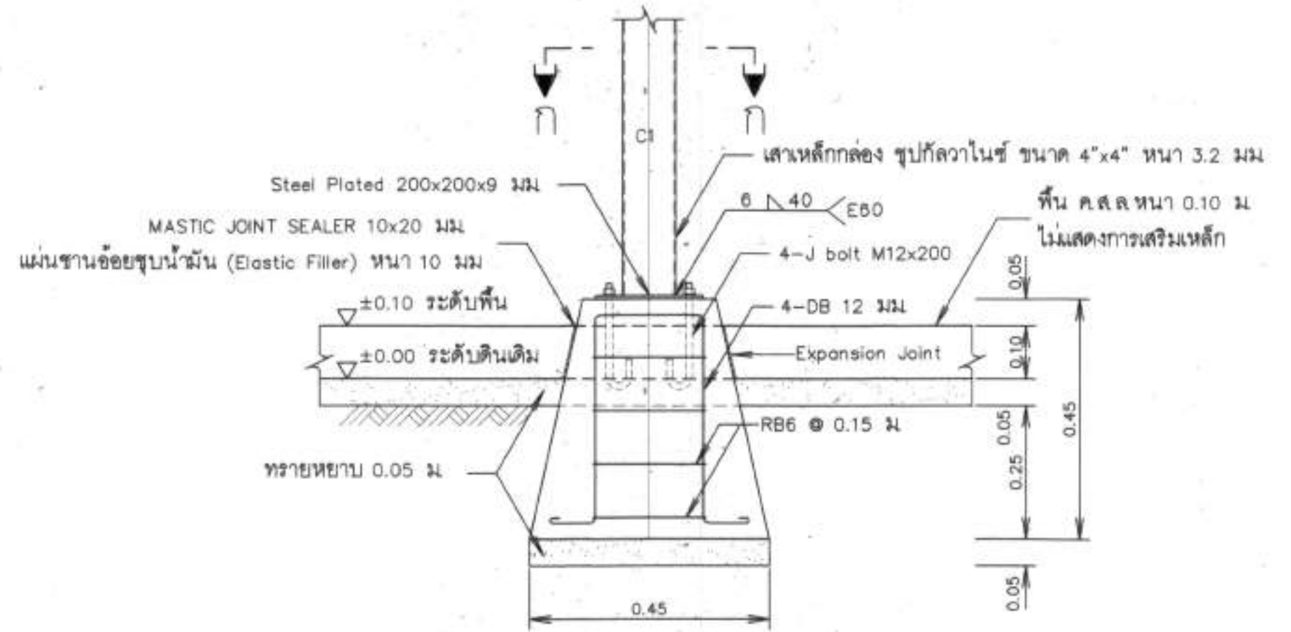
รูปขยายฐานรากโครงสร้างรับแผง F1 (ต่อหน้า คสล. หลังสำเร็จรูปพร้อมติดตั้ง) ไม่แสดงมาตราส่วน
