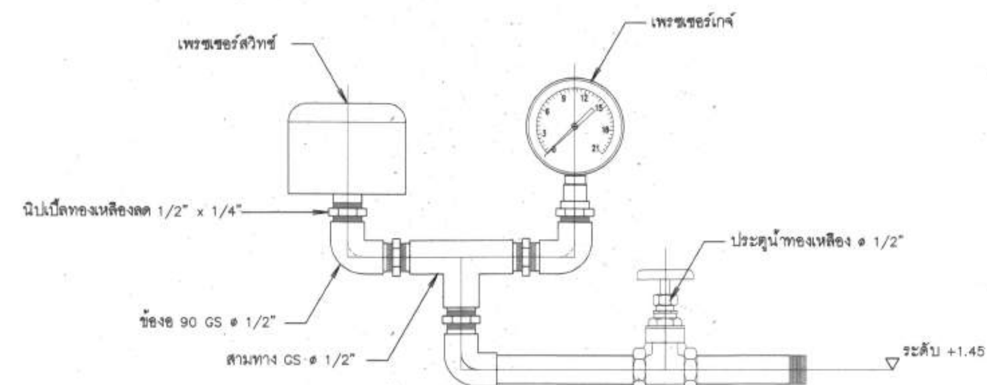
แบบขยายสวิตช์ควบคุมและเกจวัดความดัน ไม่แสดงขนาดส่วน
