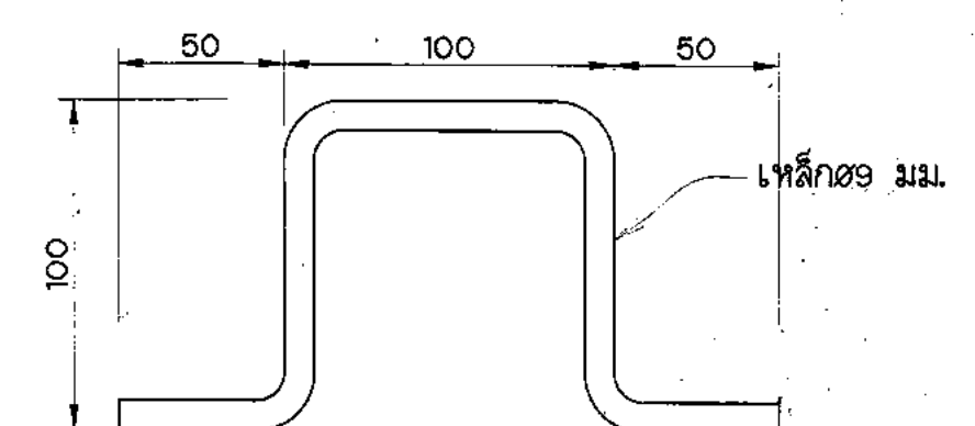
รูปขยายเหล็กหัวผ้าMANHOLE
