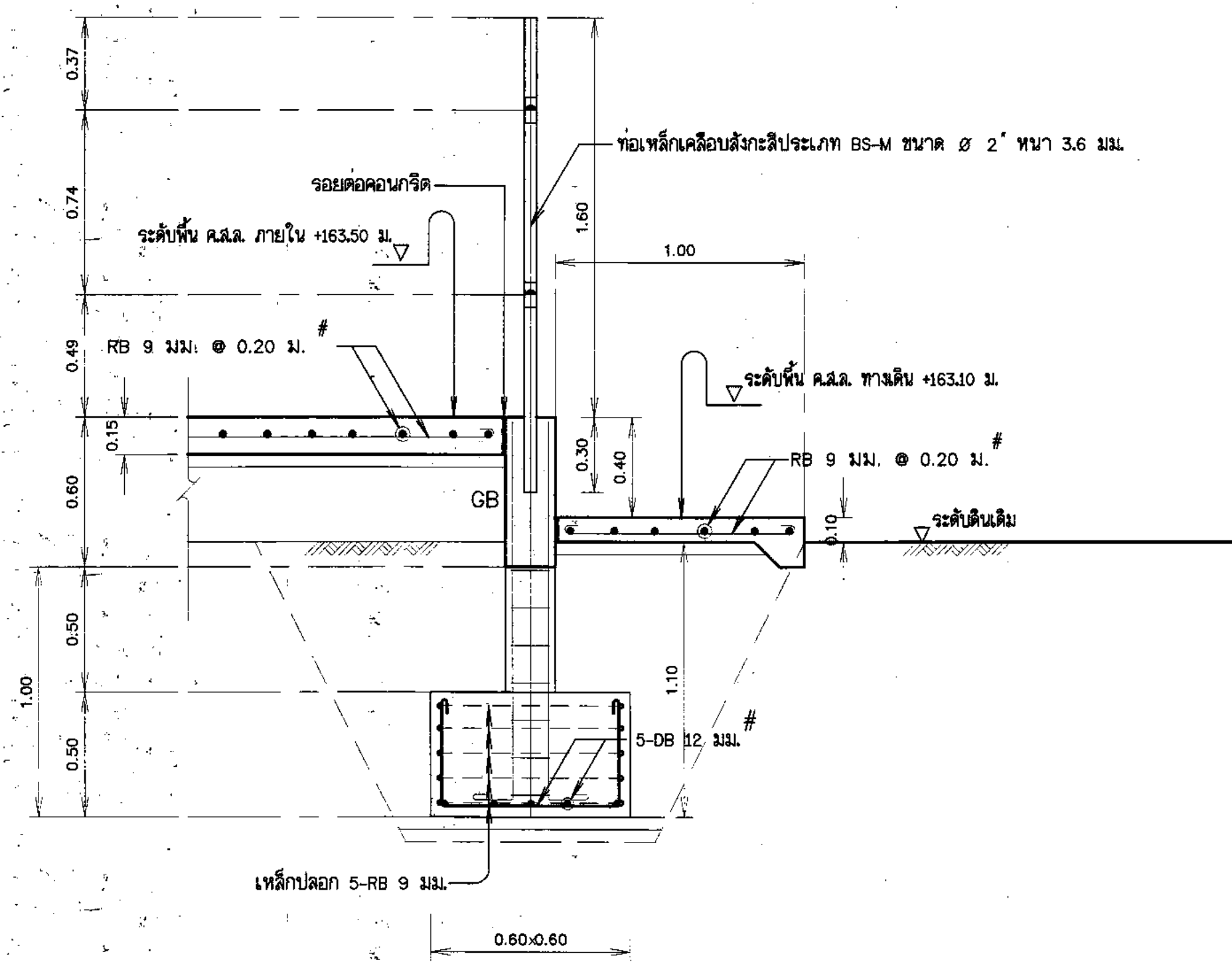
ขยายฐานรากรั้ว (F1) มาตราส่วน 1:20
