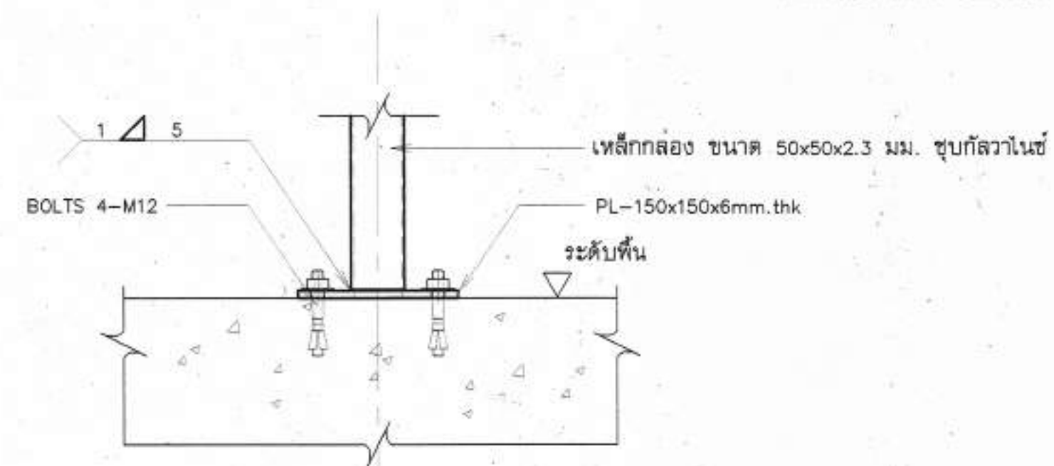
รูปตัด ข1 - ข1 มาตราส่วน 1:5
