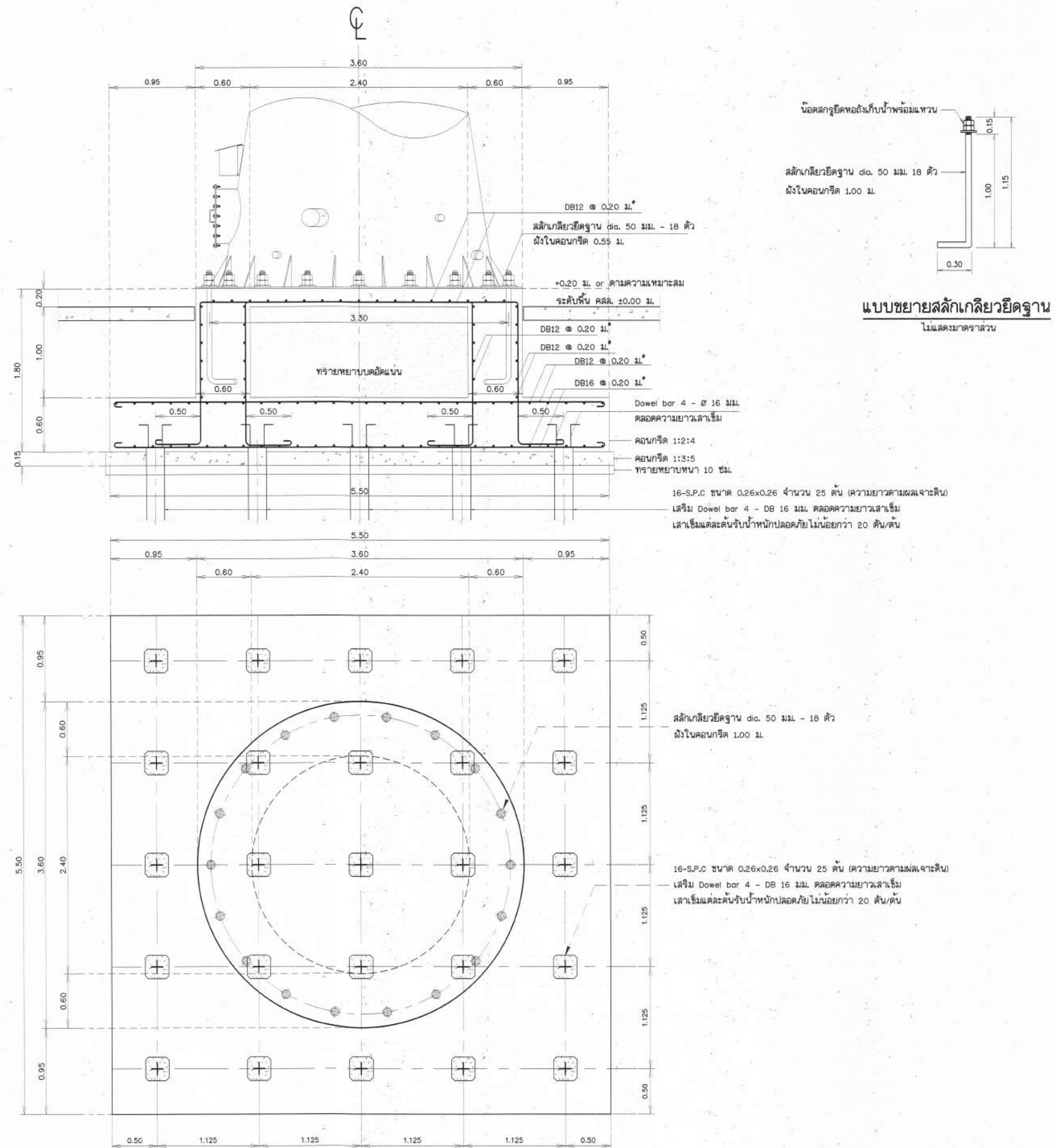
แบบขยายฐานรากท่อถึงสูง (แบบเสาเข็ม)
