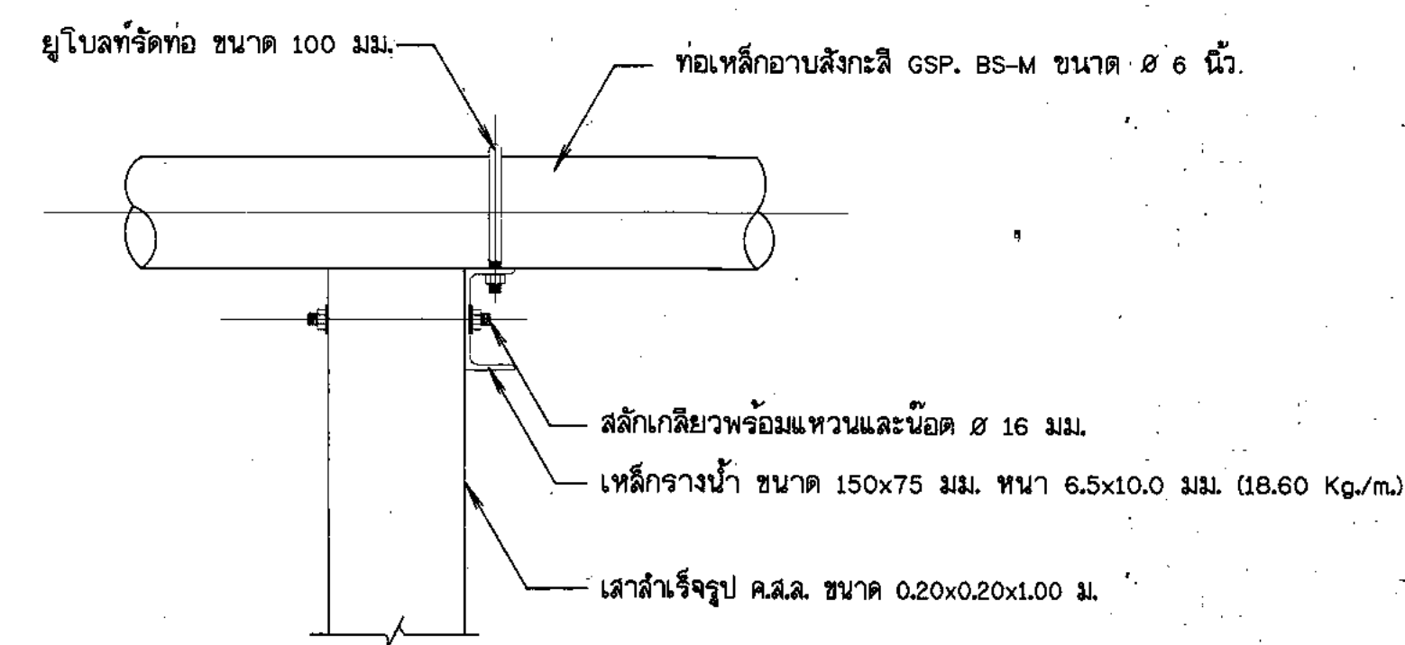
รูค้ำข้างเสาดอม่อรับท่อ และแบบขยายอุปกรณ์รับท่อ มาตราส่วน 1 : 10
