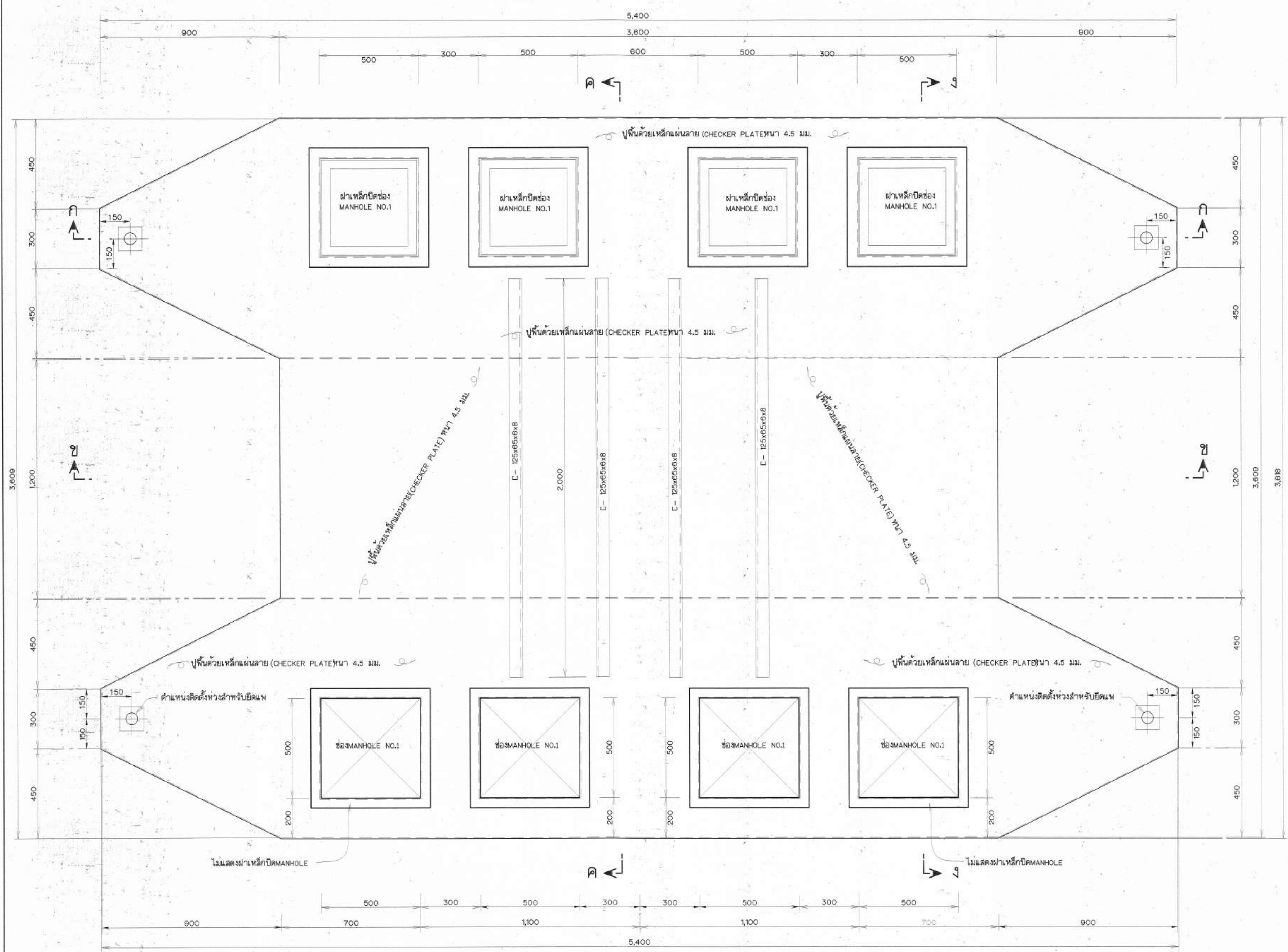
แปลนพื้นแพสูบน้ำ มาตราส่วน 1 : 10
