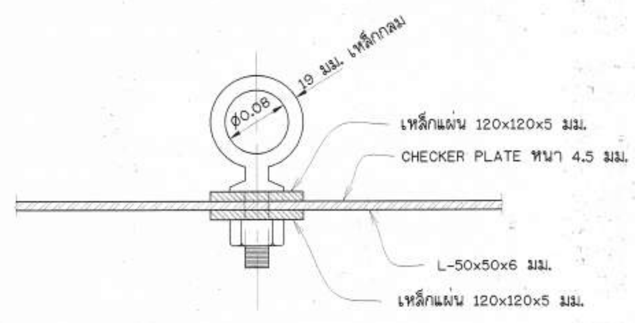
รูปขยายห่วงยึดแป้ลสูบน้ำ มาตราส่วน 1 : 5
