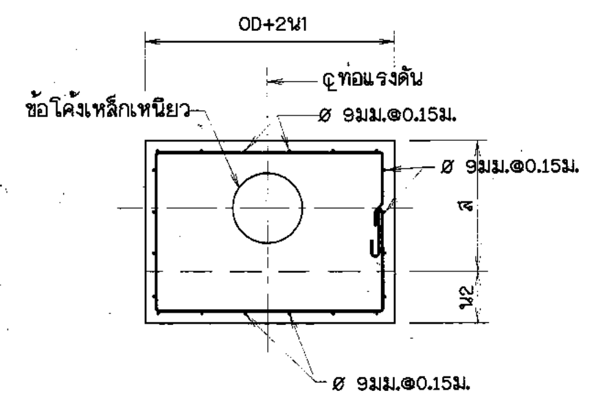
รูปตัด จ-จ
