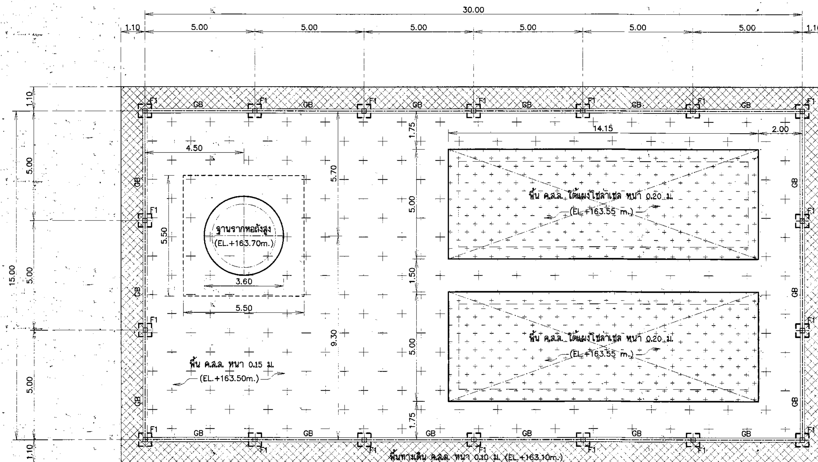
แปลนโครงสร้างอาคารสถานีสวนน้ำ มาตราส่วน 1:100
