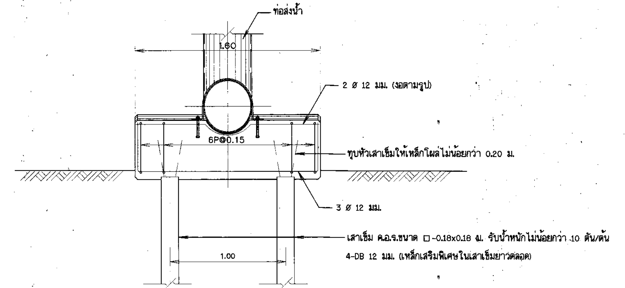
รูปตัด ก-ก
