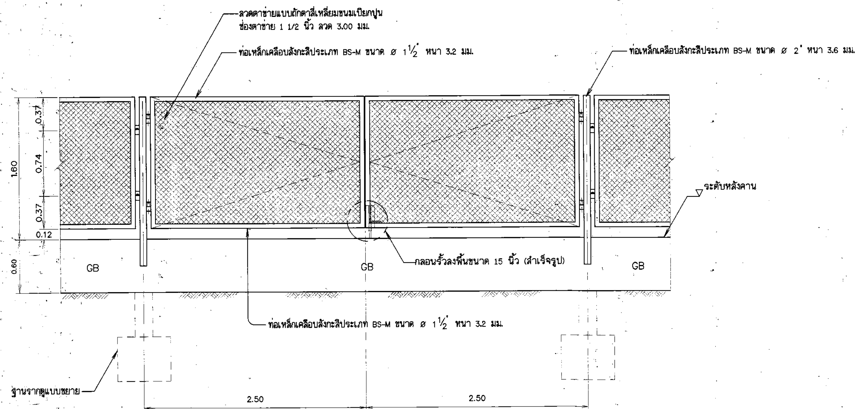
แบบขยายประตู่รั้ว มาตราส่วน 1:25
