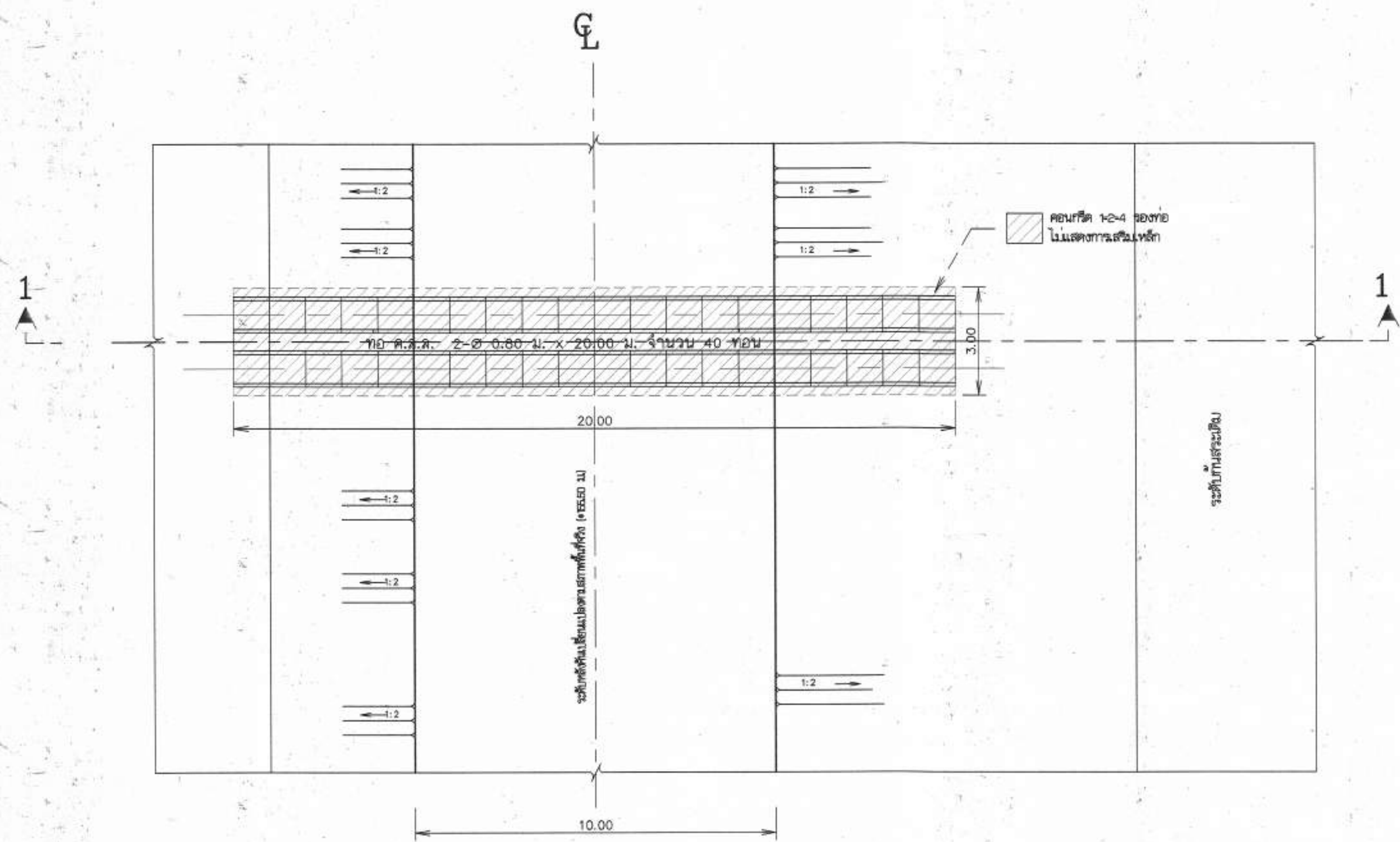
แปลนวางท่อทางน้ำเข้า คสล. ขนาด 2-Ø 0.80 ม. X 20.00 ม. มาตรฐาน 1:100
