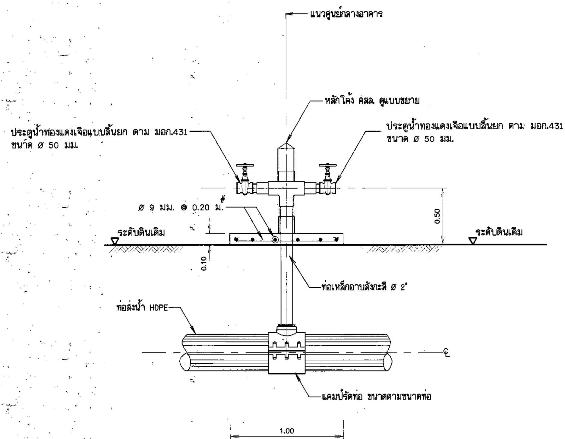
รูปตัด ก - ก (แบบที่ 1)
