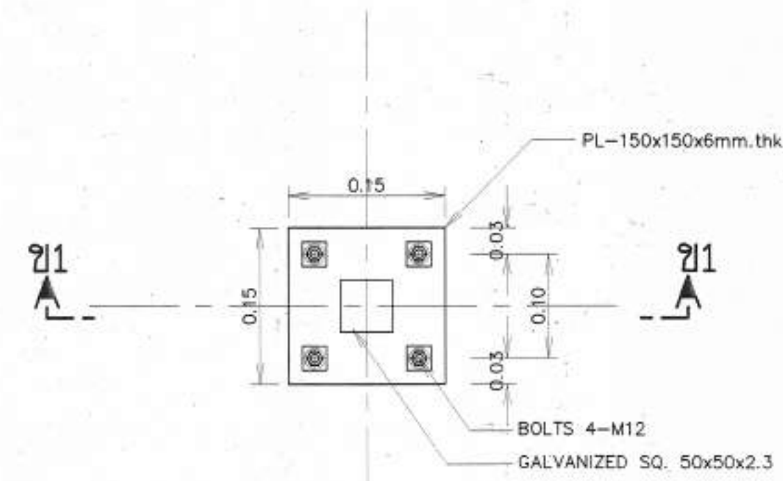
แบบขยายเสา 2 มาตราส่วน 1:5
