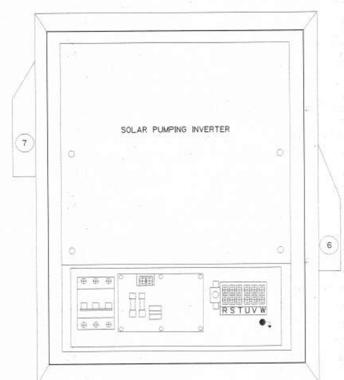
ภาพแสดงรายละเอียด แผนผังระบบไฟฟ้า และไดอะแกรมไฟฟ้า ระบบสูบน้ำด้วยพลังงานแสงอาทิตย์
