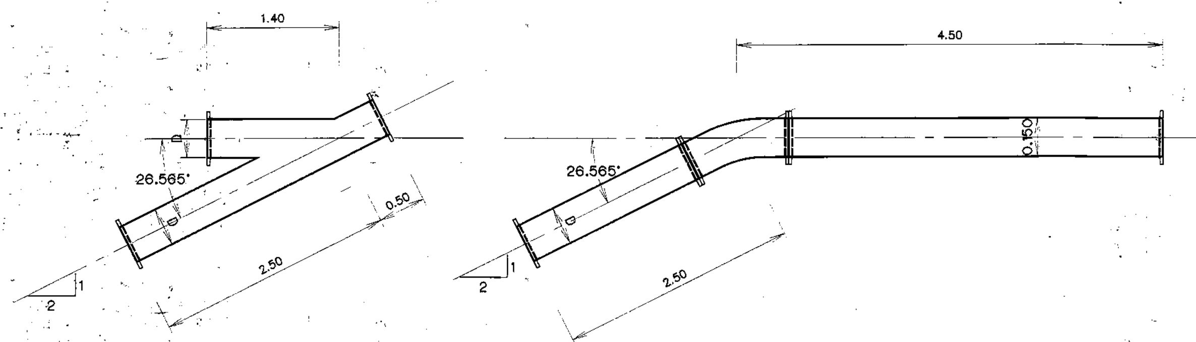
รายละเอียดท่อริมตลิ่ง ลาด 1:2
