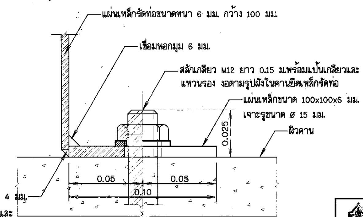
รูปตัด ง-ง
