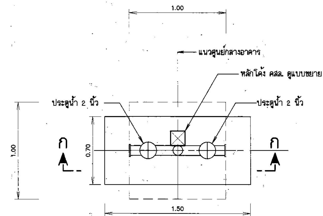
แปลนอาคารจุดปล่อยน้ำ (แบบ ข)
