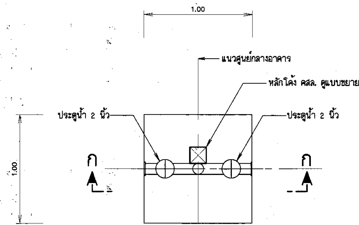
แปลนอาคารจุดปล่อยน้ำ (แบบ ก)
