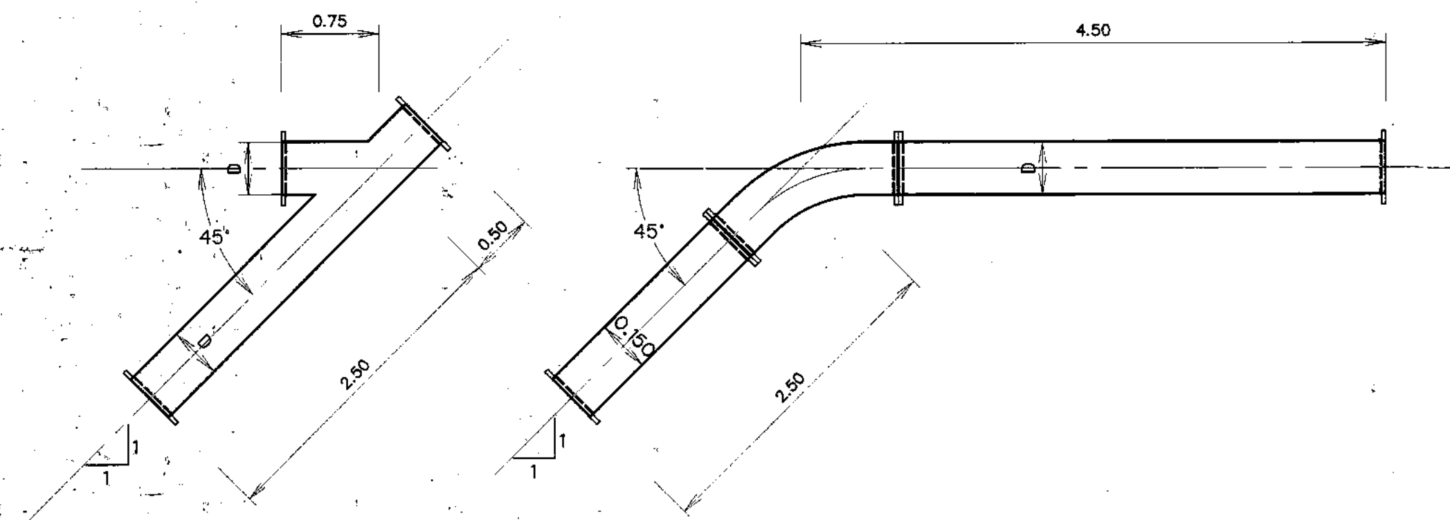
รายละเอียดท่อริมตลิ่ง ลาด 1:1
