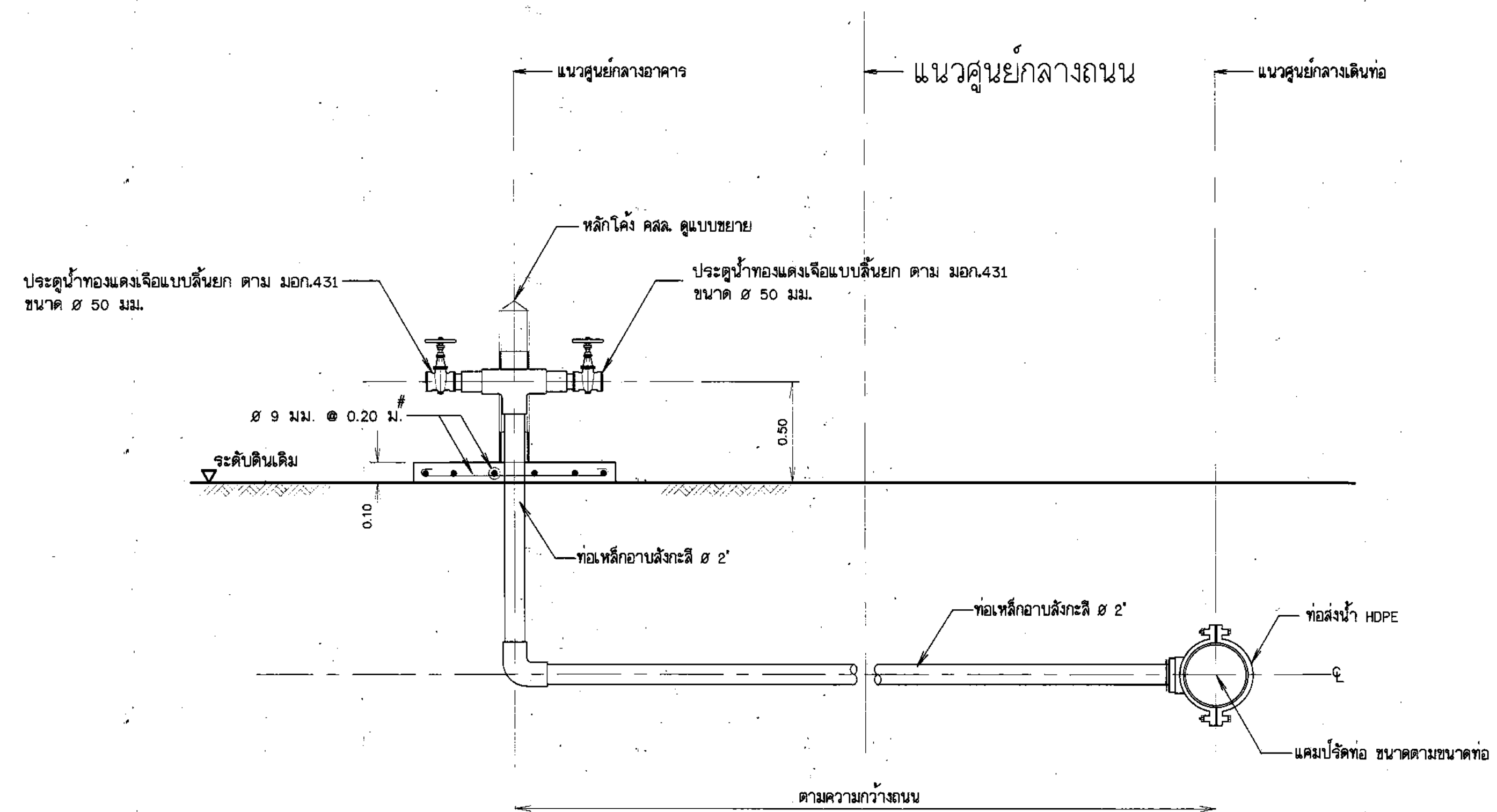
รูปตัด ก - ก (แบบที่ 2 กรณีข้ามถนน)
