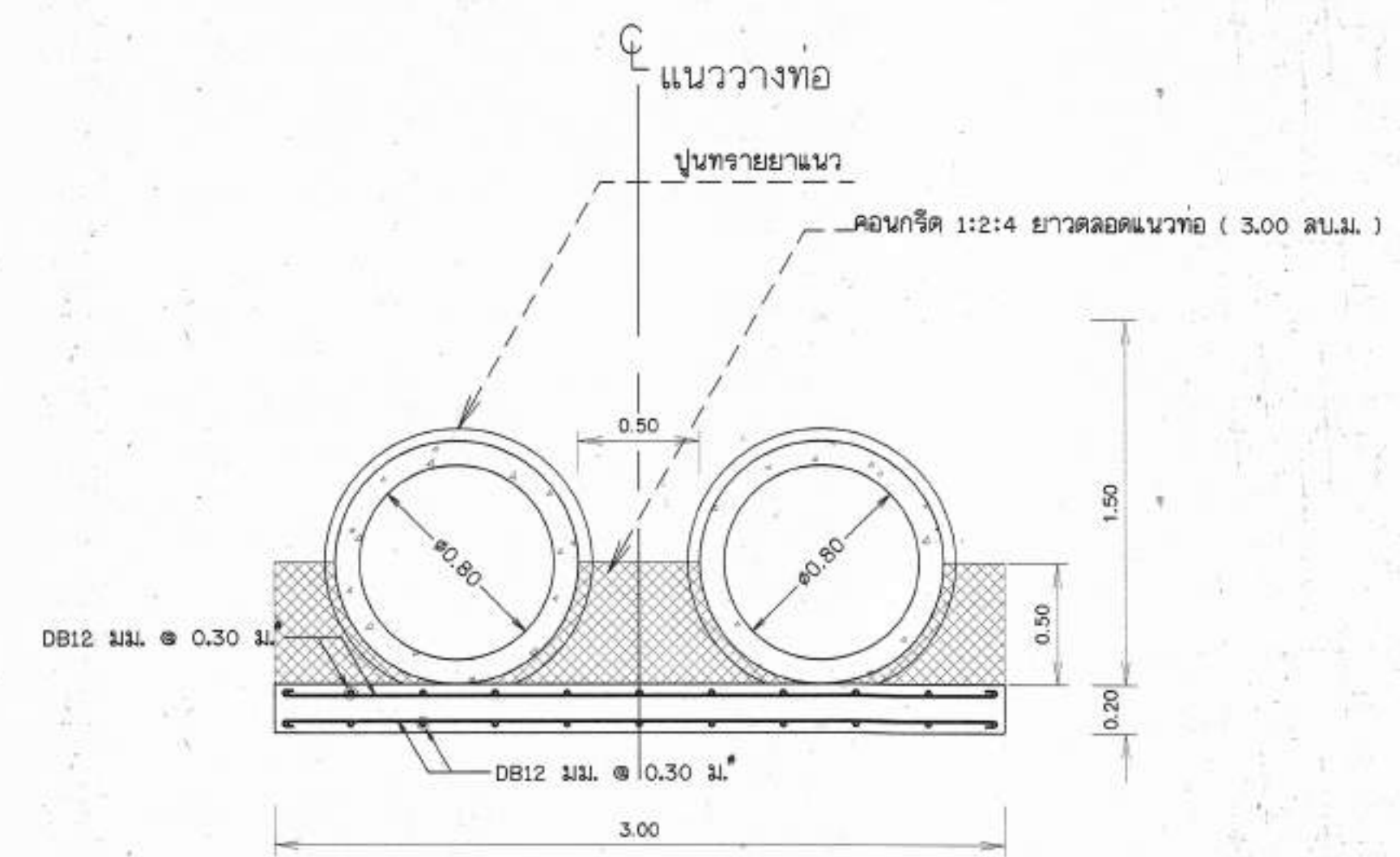
รูปตัด 2 - 2 มาตรฐาน 1:25
