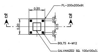
แบบขยายเสา
