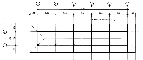
แปลนอะเส มาตราส่วน 1:100
