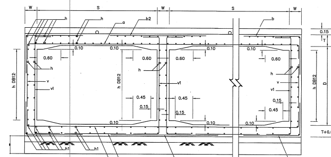
รูปตัด ①-① NOT TO SCALE
