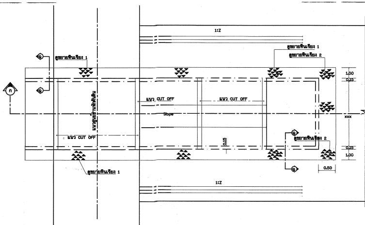
แปลนอาคารวาง Chute (กรณีพื้น Box อยู่สูงกว่าระดับชั้นพัก) ไม่แสดงขนาดส่วน
