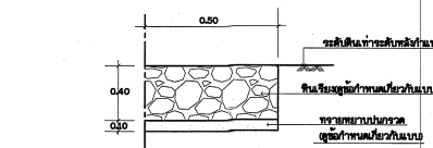
ขยายพื้นเรียบ 2 ไม่แสดงขนาดส่วน
