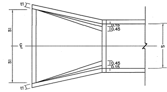
รูปตัด 1 NOT TO SCALE
