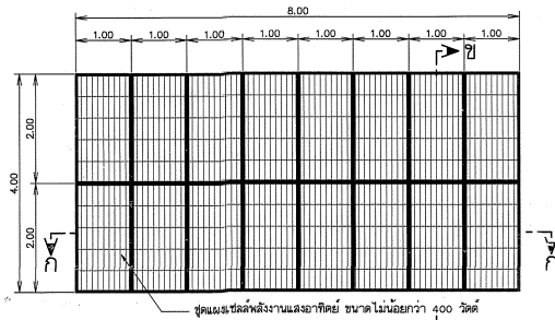
แปลนแผงเซลล์พลังงานแสงอาทิตย์ขนาดไม่น้อยกว่า 400 วัตต์ มาตราส่วน 1:50
