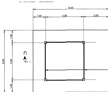
แปลนอาคารควบคุมระบบ
