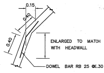
รายละเอียด 1 NOT TO SCALE
