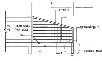
รูปตัด 2 NOT TO SCALE
