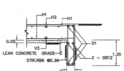
รายละเอียด 2 NOT TO SCALE
