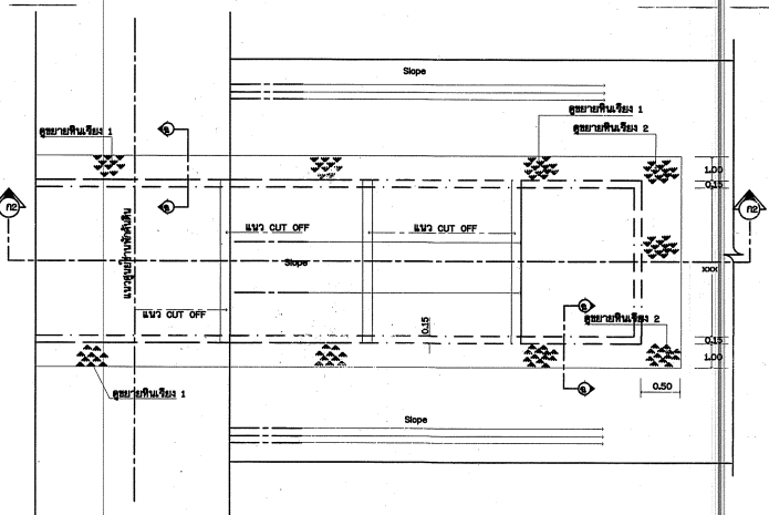
แปลนอาคารวาง Chute (กรณีพื้น Box อยู่ต่ำกว่าระดับชั้นพัก) ไม่แสดงขนาดส่วน
