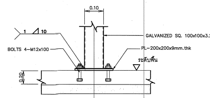
รูปตัด ข - ข
