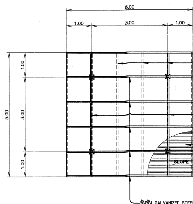
แปลนอาคารควบคุม
