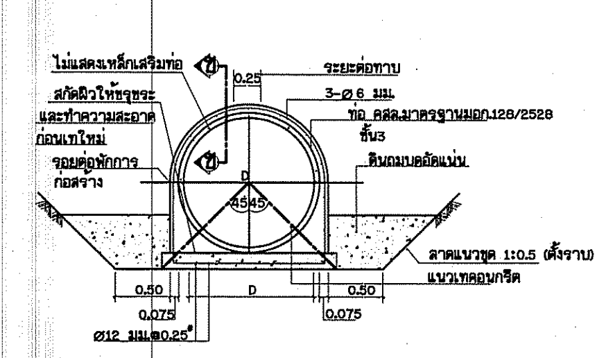
รูปตัดการวางท่อ คลส. ไม่แสดงมาตราส่วน
