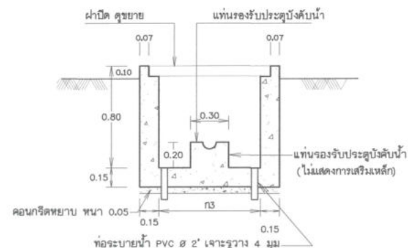
รูปตัด 1 - 1 มาตราส่วน
