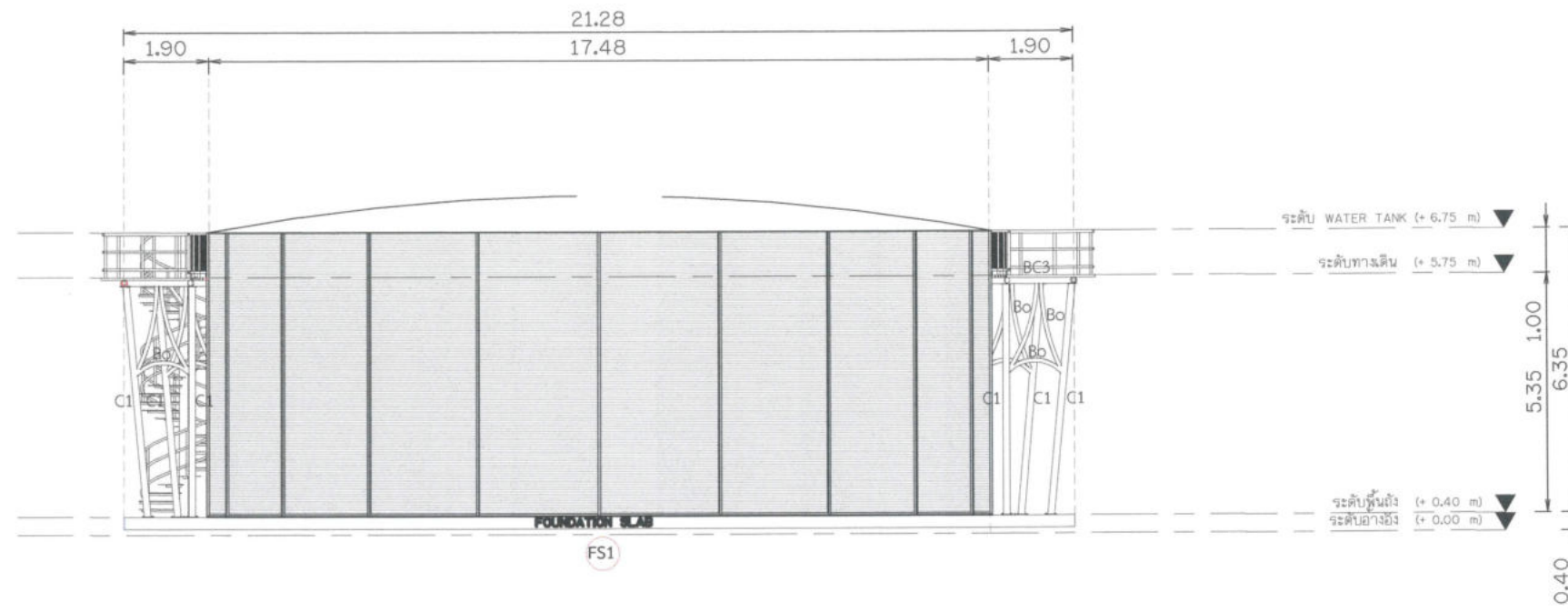
SECTION 1 - 1 มาตรฐาน 1 : 150
