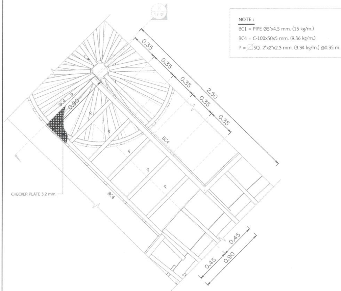
DETAIL : A
