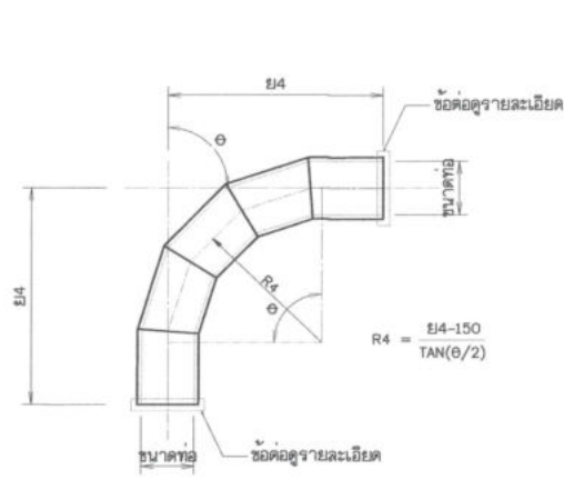
ข้ออ 5 ขึ้น \theta = 45-90 องศา ไม่แสดงมาตราส่วน
