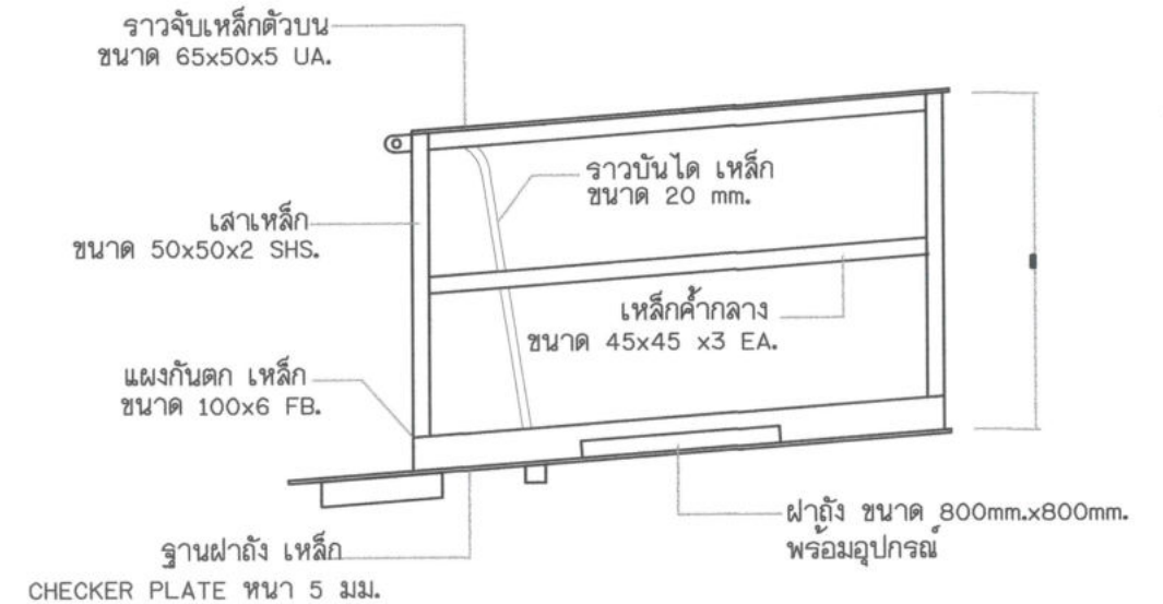
แบบขยาย 4 รูปตัดโครงเหล็กถักทั่วไป ไม่มีมาตราส่วน
