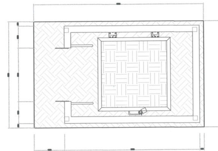
แบบขยาย 4.2 - แบบขยายแท่นทางเข้าถึง ไม่มีมาตราส่วน
