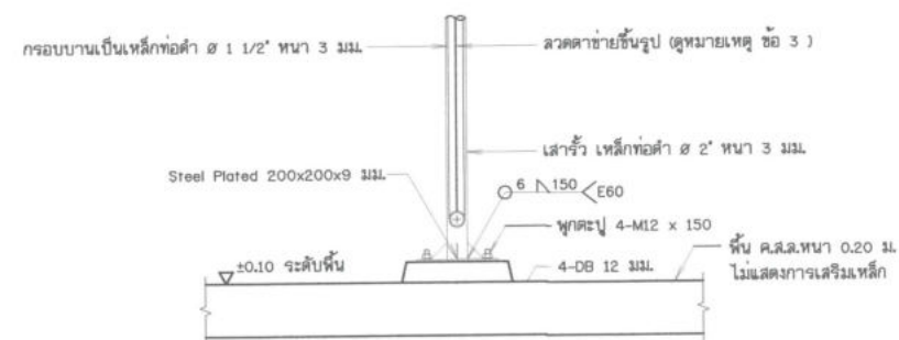
แบบขยายรายละเอียดแสดงการยึด ไม่แสดงขนาดราวล้วน
