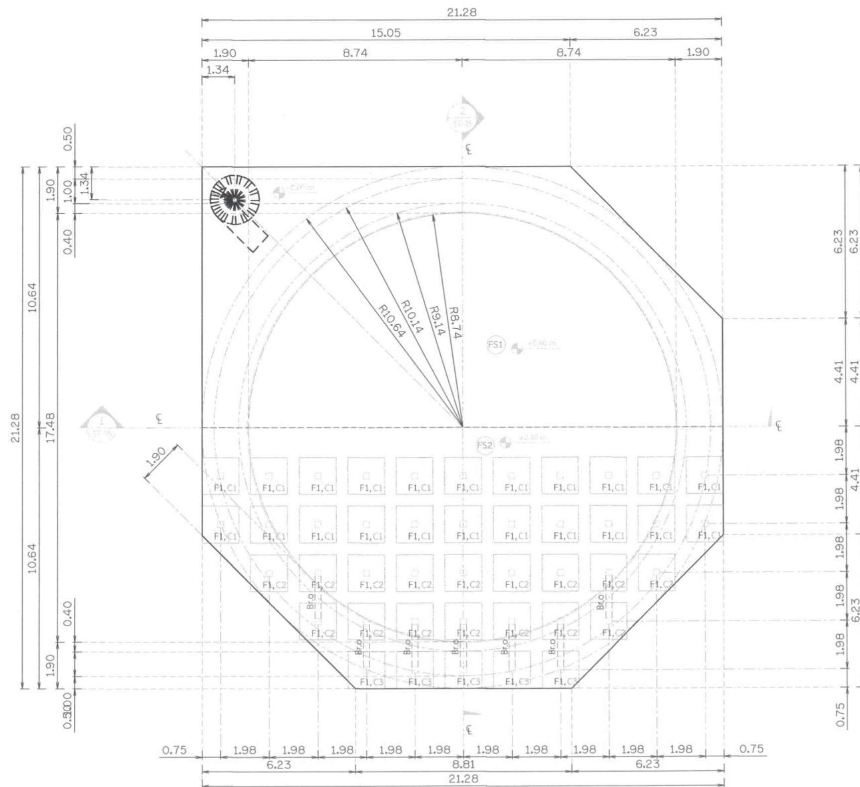
แปลน ฐานราก , พื้น มาตราส่วน 1 : 150
