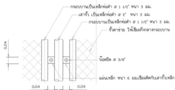
แบบขยายรายละเอียดแสดงการยึดระหว่างรั้วกับเล้า ไม่แสดงขนาดราวล้วน
