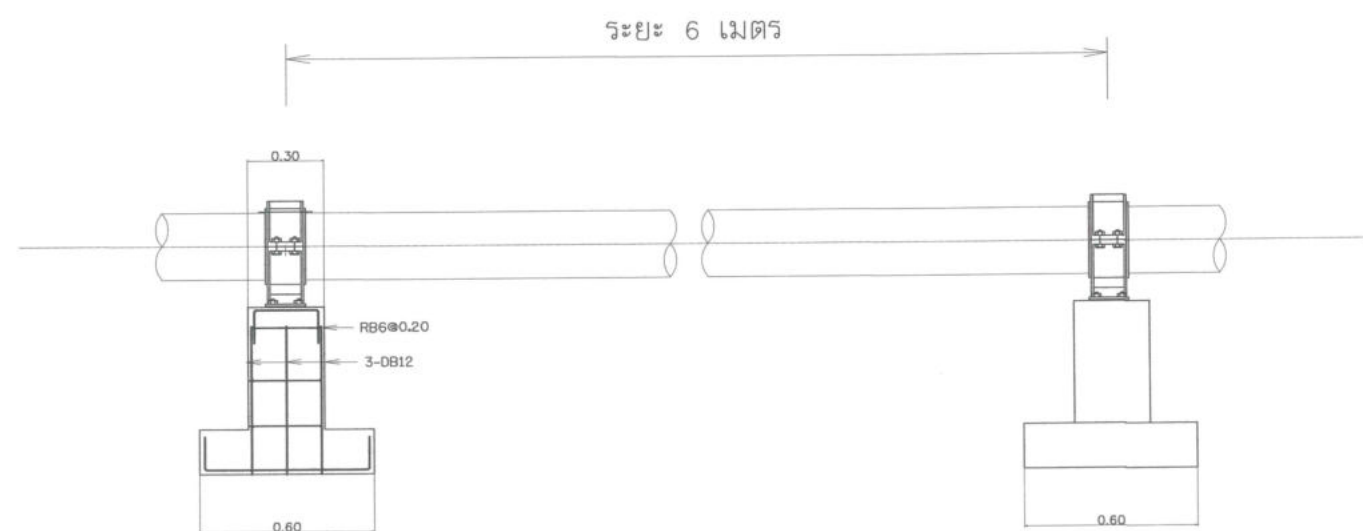
รูปด้านข้าง
