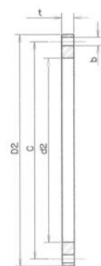
ปะเก็นยาง
