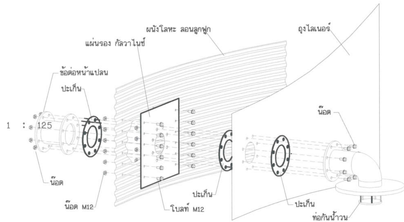
แบบท่อน้ำออกพร้อมกันน้ำวน มาตรฐาน 1 : 125
