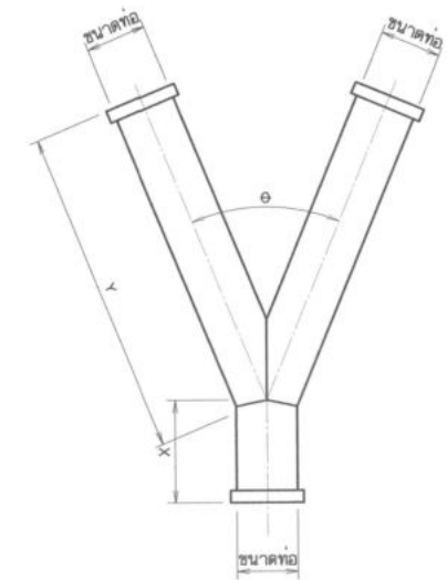
ข้อต่อ 3 ทาง รูป Y (แบบที่ 2) \theta = 45 องศา ไม่แสดงมาตราส่วน
