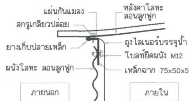
แบบขยาย 3 - จุดยึดหลังคา กับผนังถึง ไม่มีมาตราส่วน
