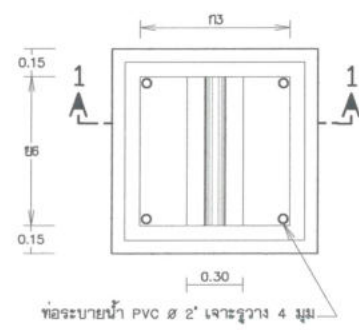
แปลนบ่อประตูปังคับน้ำ มาตราส่วน
