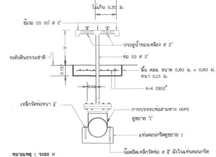
รูปตัดอาคารจุดปล่อยน้ำ 2 ด้าน (ใช้สำหรับท่อส่งน้ำที่มีขนาดไม่เกิน 6 นิ้ว) มาตราส่วน
