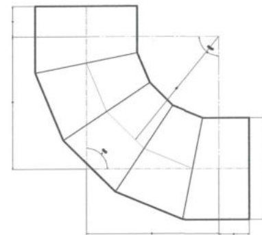
ข้อโค้ง 5 ชั้น (67.5° < 0 < 90°)
