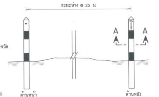
แสดงการวางหลักบ่อแก้ว มาตราส่วน
