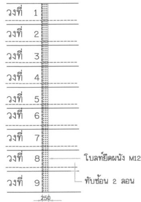
แบบขยาย 2 - รูปแบบการเจาะโบลท์ ไม่มีมาตราส่วน
