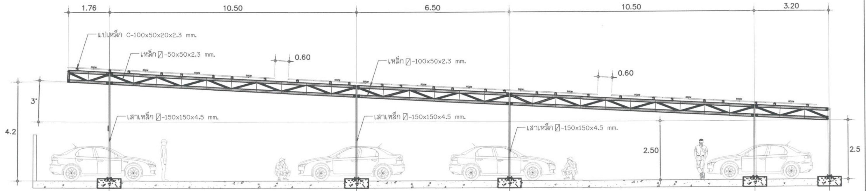
รูปด้าน โครงรับแผง (1)
