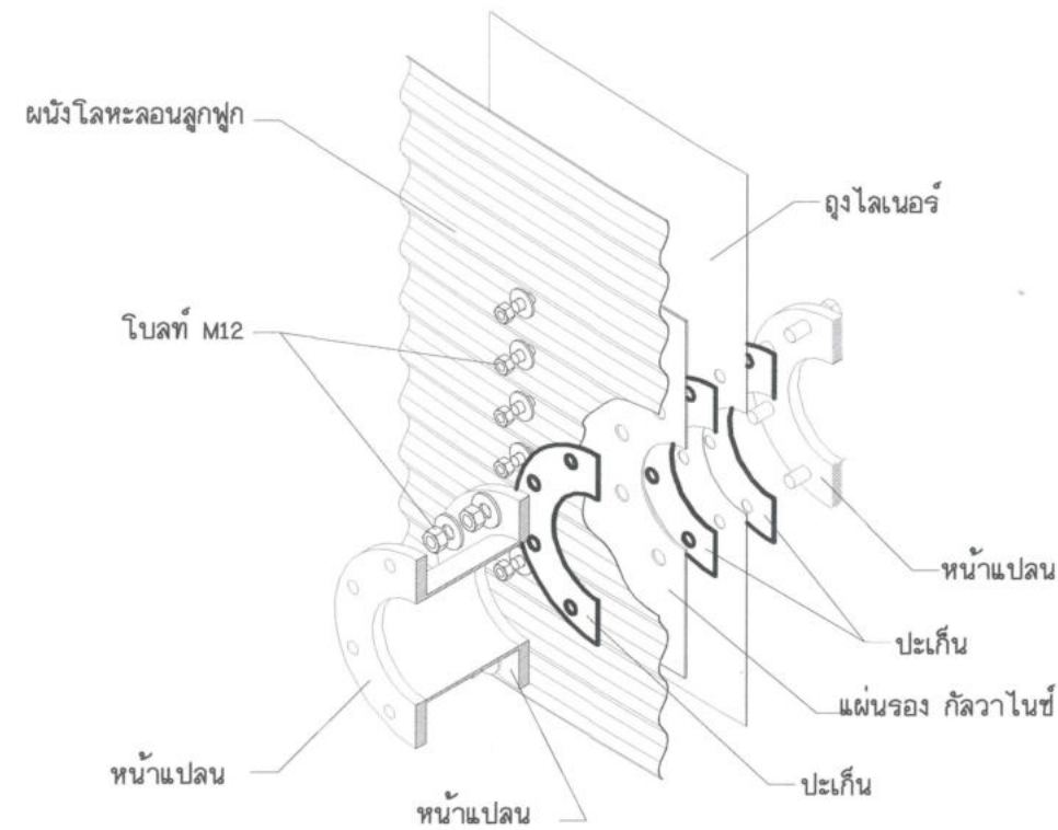
ข้อต่อท่อน้ำแบบหน้าแปลน มาตรฐาน
