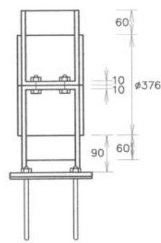
รูปด้านข้าง
