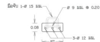
รูปตัดแนว 2 - 2 มาตราส่วน
