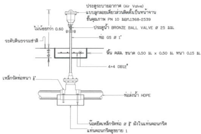
รูปตัดอาคารท่อระบายอากาศ Ø 25 มม. (ใช้สำหรับท่อส่งน้ำที่มีขนาดไม่เกิน 6 นิ้ว) มาตราส่วน
