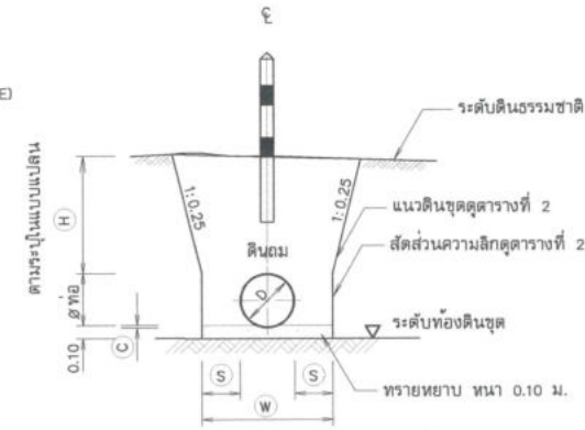
รูปตัดทั่วไปแสดงการวางท่อ มาตราส่วน
