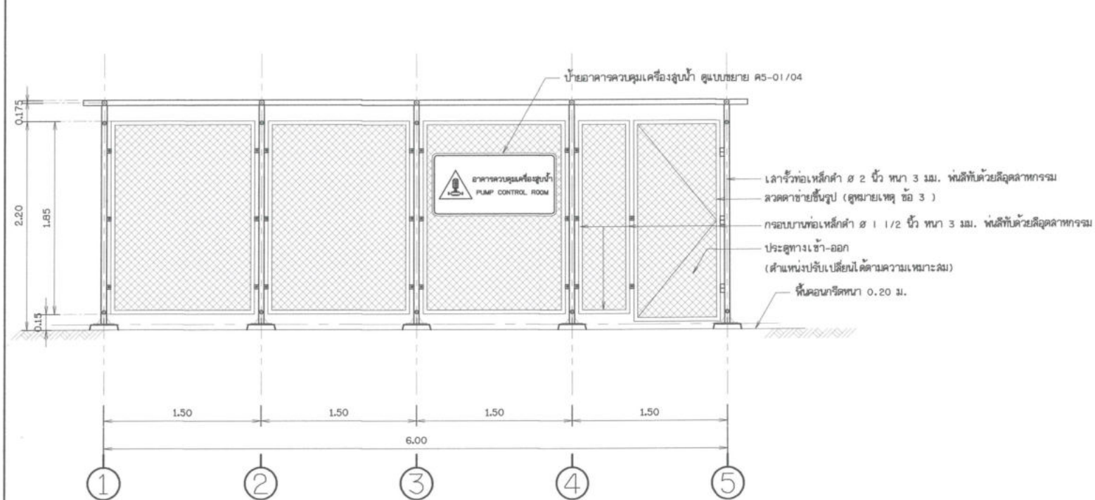
แบบขยายรั้ว 1 ไม่แสดงขนาดราวล้วน
