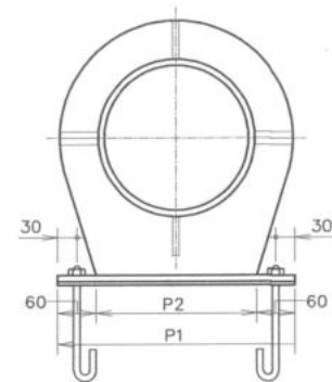
รูปด้านหน้า
