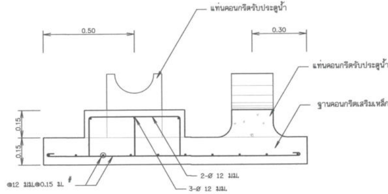
รูปตัด ก - ก
