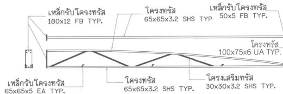
แบบขยาย 4 รูปตัดโครงเหล็กถักทั่วไป ไม่มีมาตราส่วน
