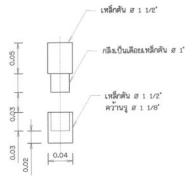
แบบขยายบานพับเหล็ก ไม่แสดงขนาดราวล้วน
