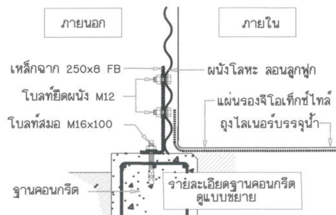
แบบขยาย 1 - จุดติดตั้งผนังถึงกับฐาน ไม่มีมาตราส่วน
