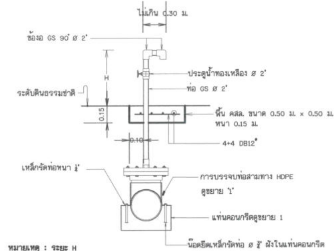
รูปตัดอาคารท่อระบายอากาศ Ø 50 มม. (ใช้สำหรับท่อส่งน้ำที่มีขนาดไม่เกิน 6 นิ้ว) มาตราส่วน
