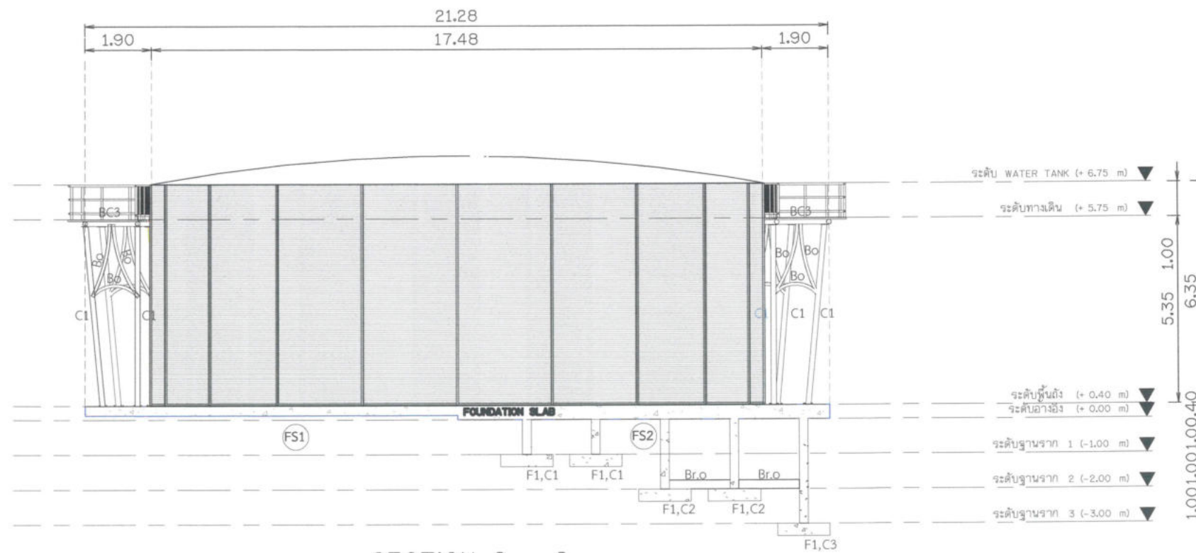
SECTION 2 - 2 มาตรฐาน 1 : 150
