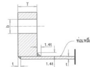
รายละเอียด "I"
