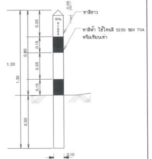
แสดงลัดส่วนหลักบ่อแก้ว มาตราส่วน
