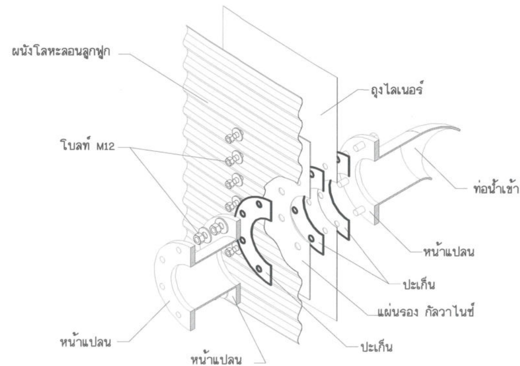
แบบท่อน้ำเข้า มาตรฐาน 1 : 125
