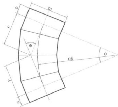
ข้อโค้ง 4 ชั้น
