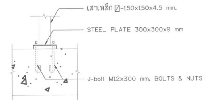
แบบขยายฐานเสาเหล็ก
