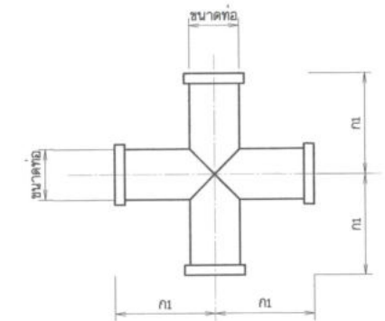
ข้อต่อ 4 ทาง ไม่แสดงมาตราส่วน
