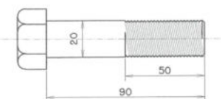
สลักเกลียวขนาด M20
