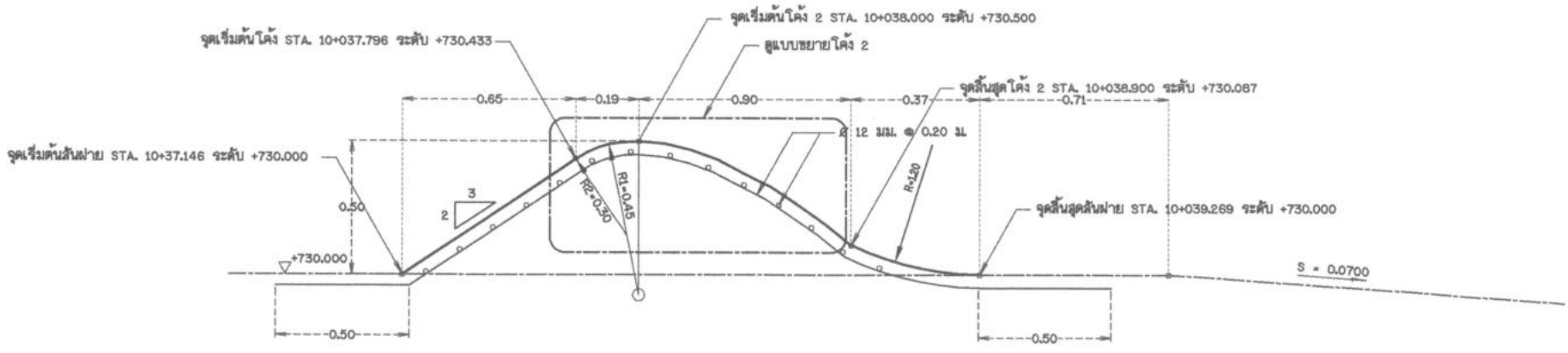
รูปขยายลัดส่วนสันฝายสูง 0.50 ม.
