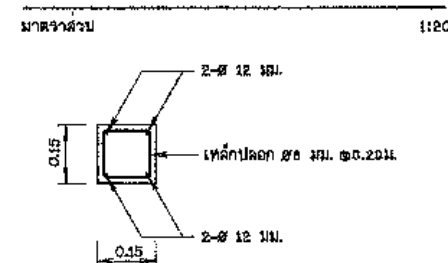
รายละเอียดเส้าป้าย คสล.
