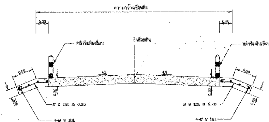
รูปขยายสันเขื่อน
