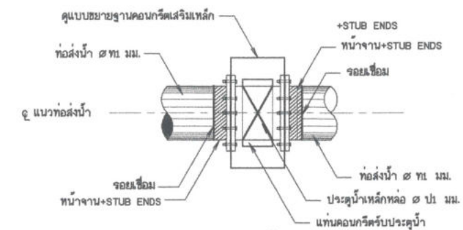
รูปขยายการติดตั้งอาคารบังคับน้ำ มาตราส่วน 1:20
