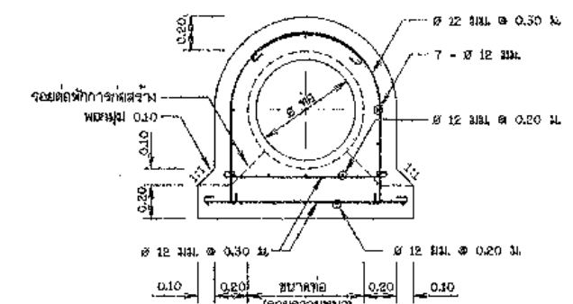
รูปตัด ง - ง
