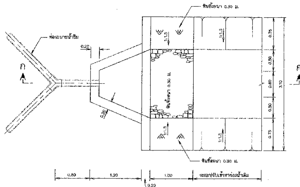
แปลนอาคารระบายน้ำซึมท้ายเขื่อน
