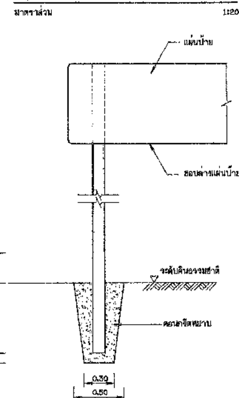
รูปแสดงการประกอบแผ่นป้าย
