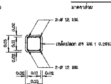
รูปตัด ข - ข
