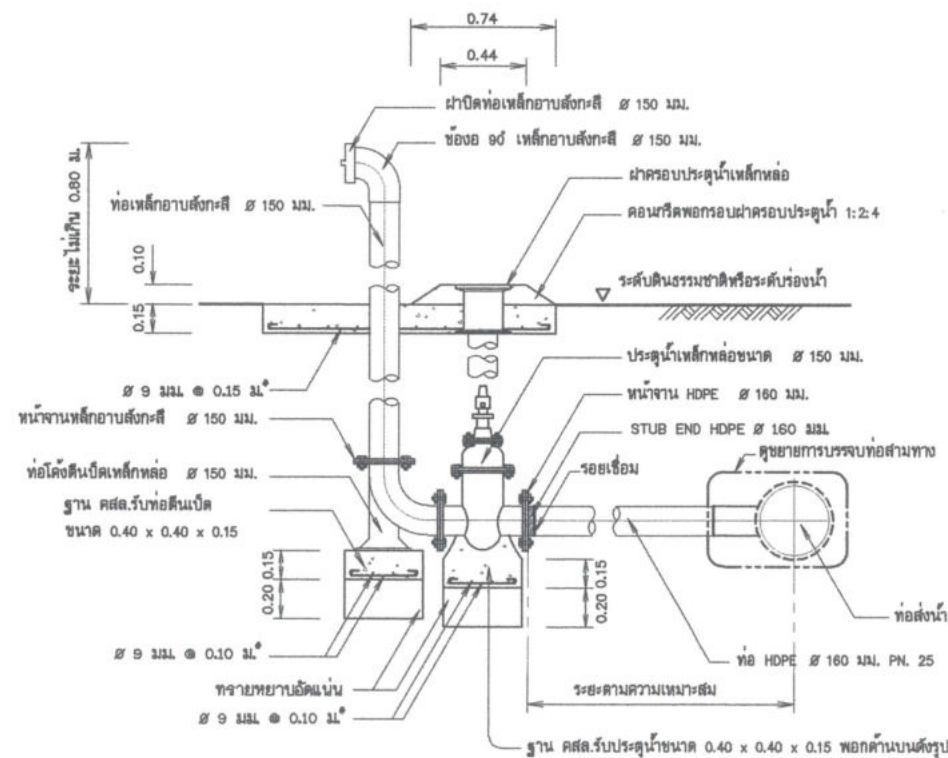
รูปตัด ก - ก แสดงการติดตั้งประตูละบายตะกอน
