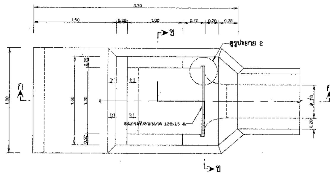
แปลนอาคารบังคับน้ำด้านเหนือ
