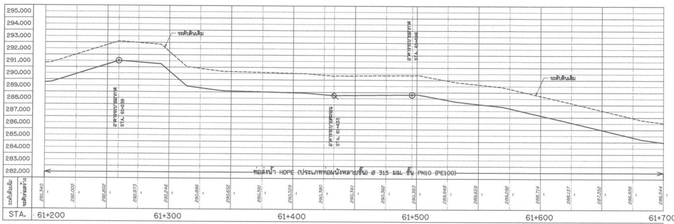
รูปตัดตามแนวยาวระบบกระจายน้ำ สาย 4R-LMP มาตราส่วน 1:1,000 แนวตั้ง 1:100
