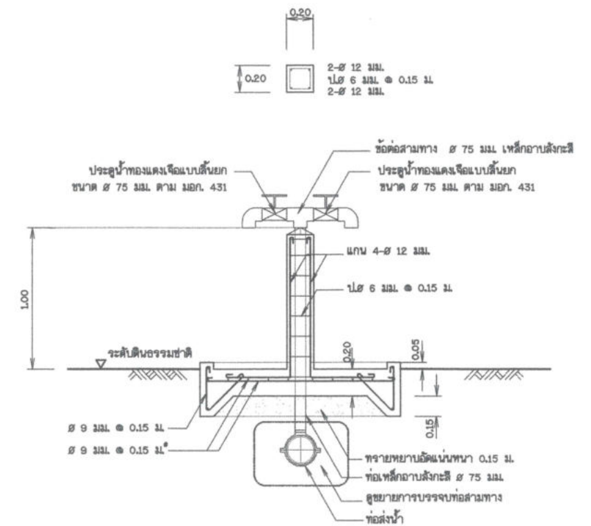
รูปตัด ค - ค
