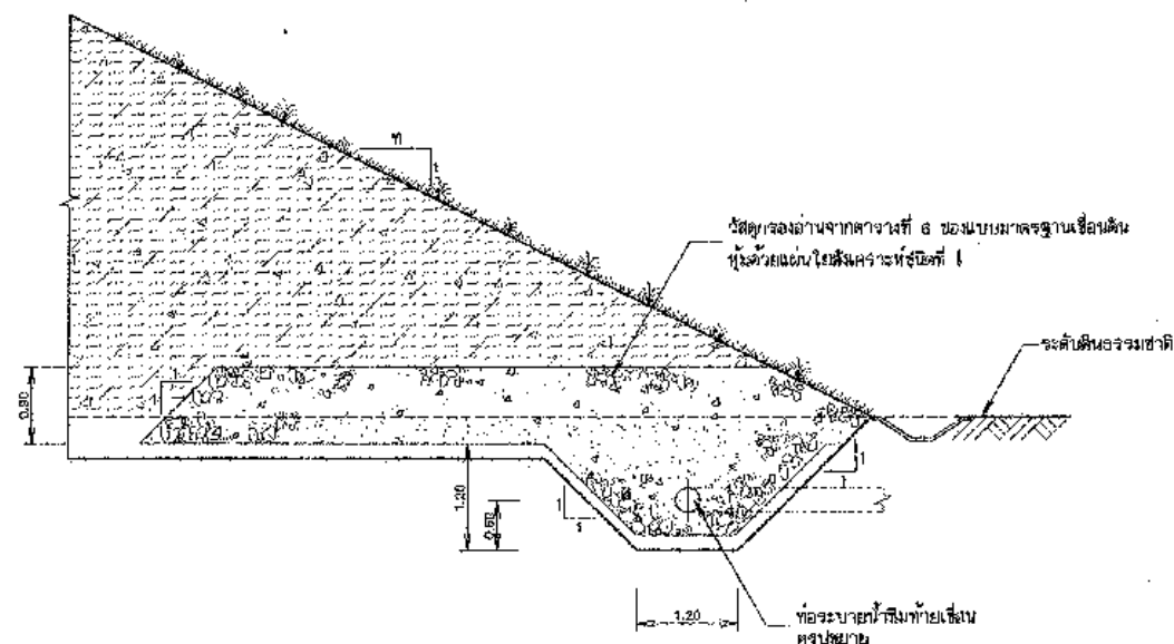
รูปขยายท่อระบายน้ำซึมท้ายเขื่อน
