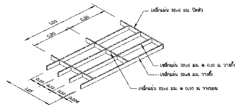
รูปขยายตะแกรงกันสวะ
