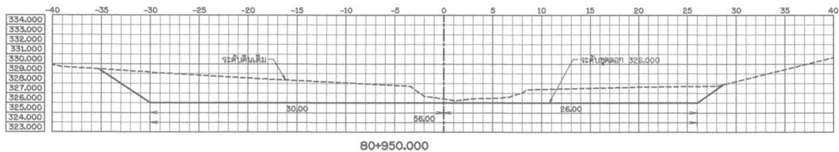
รูปตัดแสดงงานดิน มาตราส่วน 1:200
