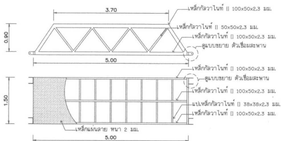
แบบขยายสพานช่วงที่ 6
