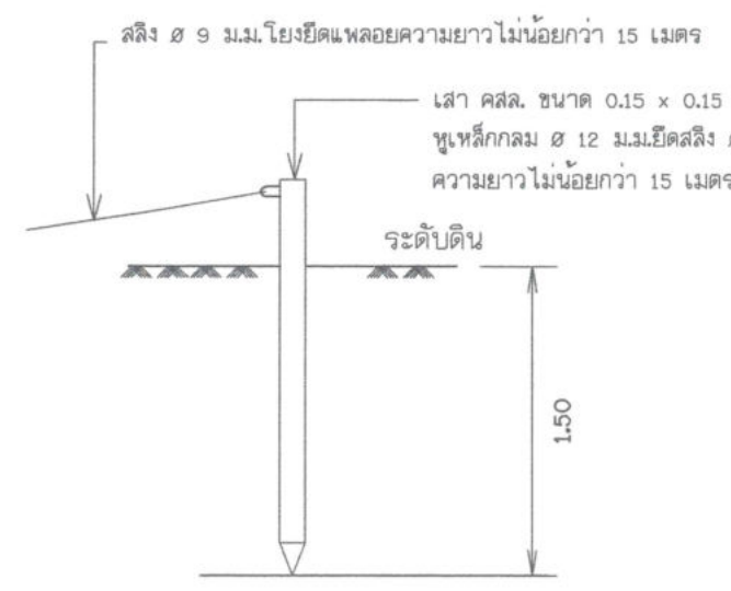
สลิงโยงยึดแพลอย
