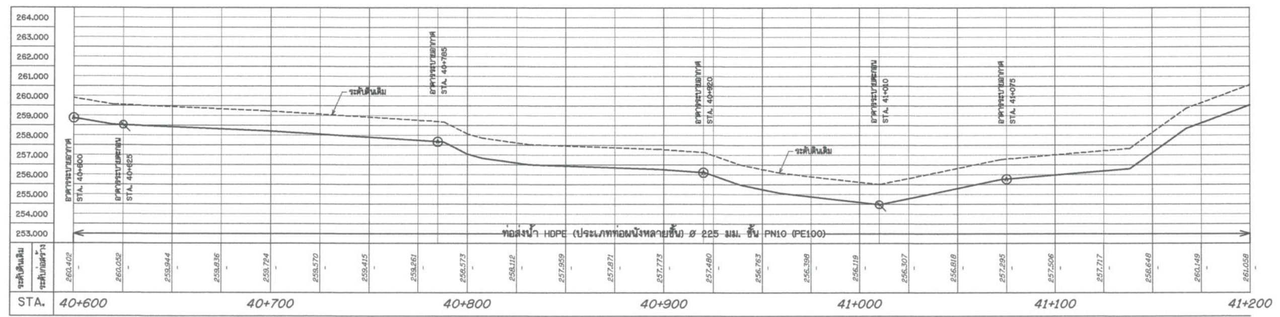
รูปตัดตามแนวยาวระบบกระจายน้ำ สาย 1-1R-RMP1 มาตรฐาน แนวยาว 1:1,000 แนวตั้ง 1:100
