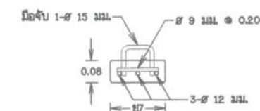
รูปตัดแนว 2 - 2
