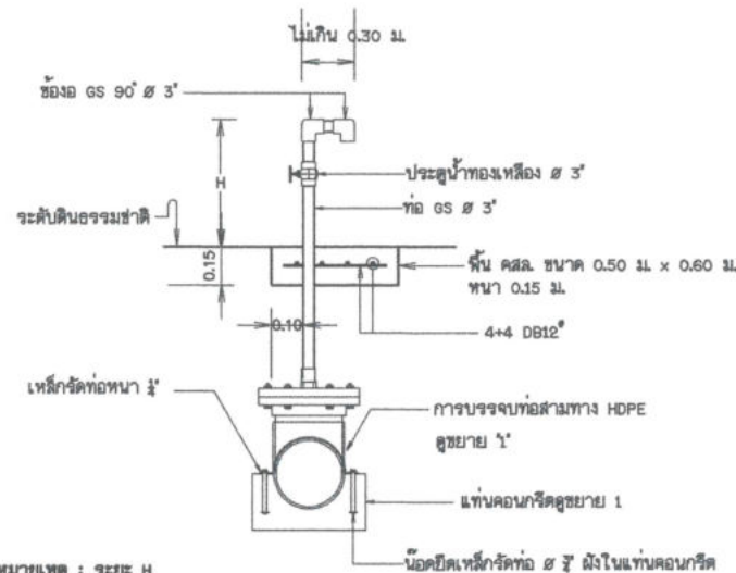
รูปตัดอาคารประตูระบายตะกอน Ø 75 มม.
