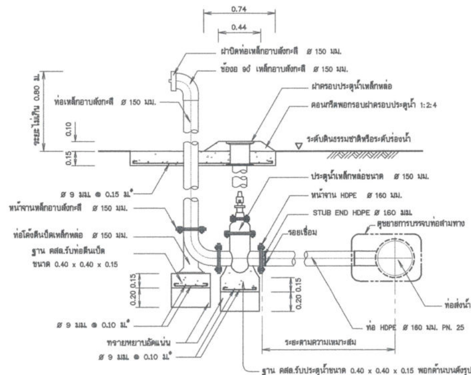
รูปตัด ก - ก แสดงการติดตั้งประตูละบายตะกอน
