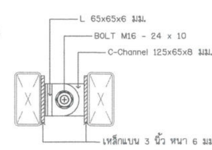
แบบขยายตัวเชื่อม
