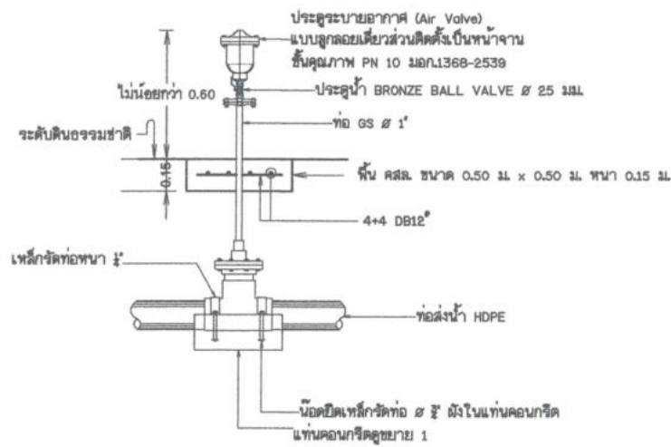
รูปตัดอาคารท่อระบายอากาศ Ø 25 มม. (ใช้สำหรับท่อส่งน้ำที่มีขนาดไม่เกิน 6 นิ้ว)
