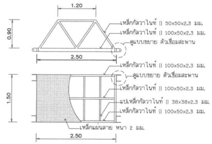
แบบขยายสพานช่วงที่ 1,3,5
