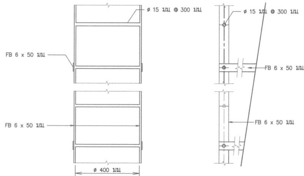
ภาพขยายบันได "1" ภายในหอดังเหล็กเก็บน้ำ
