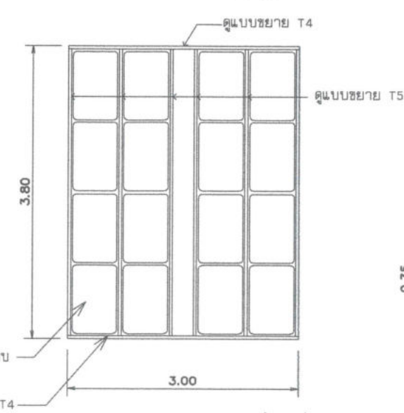
แบบขยายสพานช่วงที่ 6
