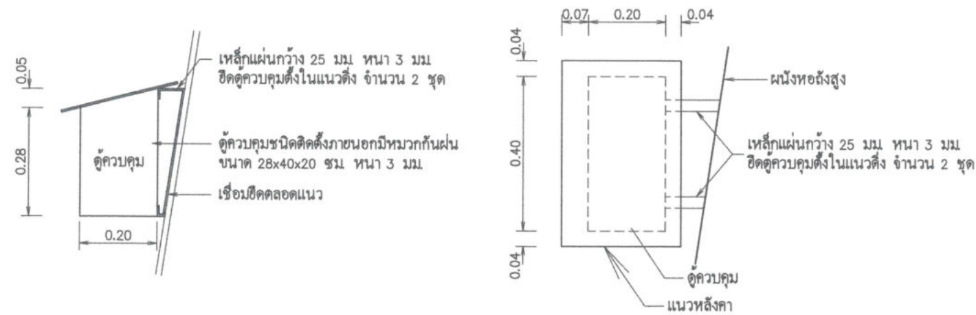
แบบขยายตู้ควบคุม
