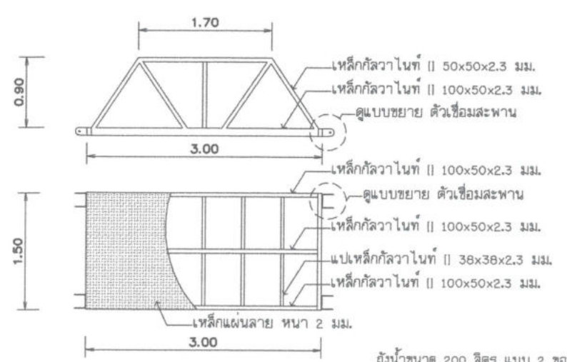
แบบขยายสพานช่วงที่ 2,4
