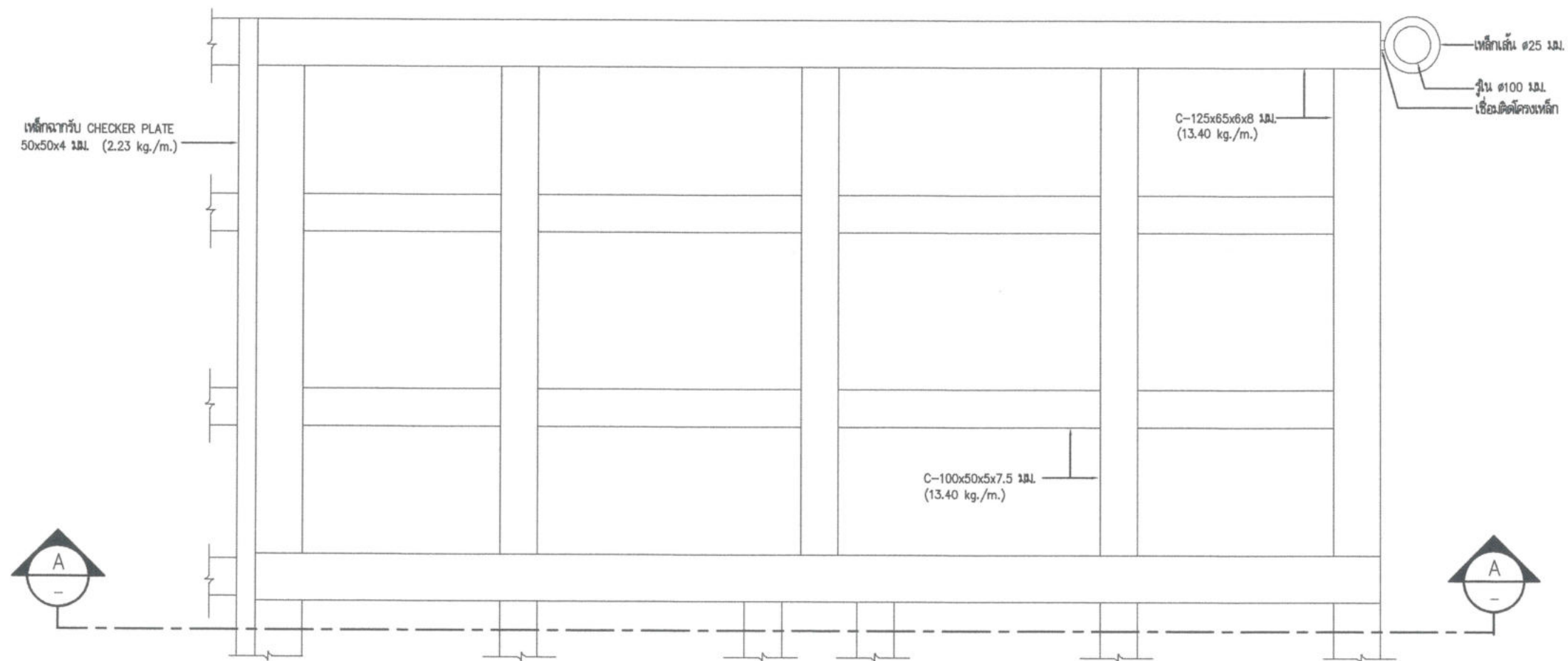
โครงสร้างรับพื้นแป้น CHECKER PLATE ทนไฟ 4.50 มม.
