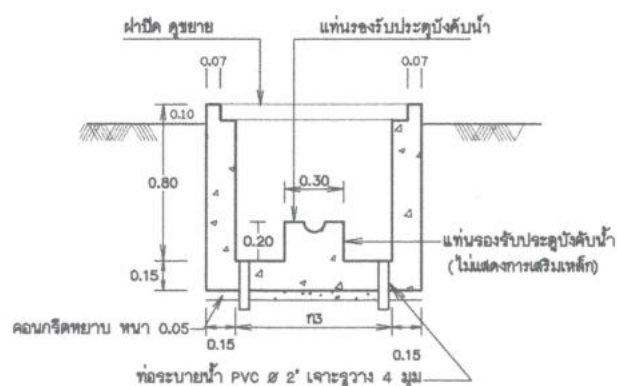
รูปตัด 1 - 1
