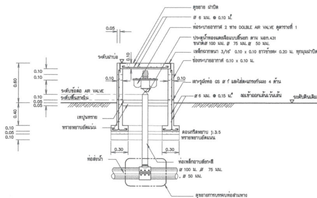
รูปตัด ข - ข แสดงการติดตั้งท่อระบายอากาศ
