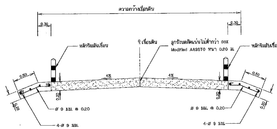
รูปขยายสันเขื่อน มาตราส่วน 1:25
