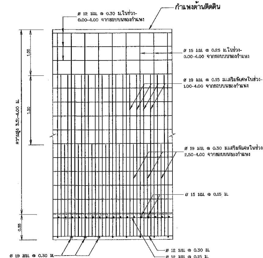
รูปขยายก้ำพังก้านตติดินความสูงระหว่าง 3.51-4.00 เมตร
