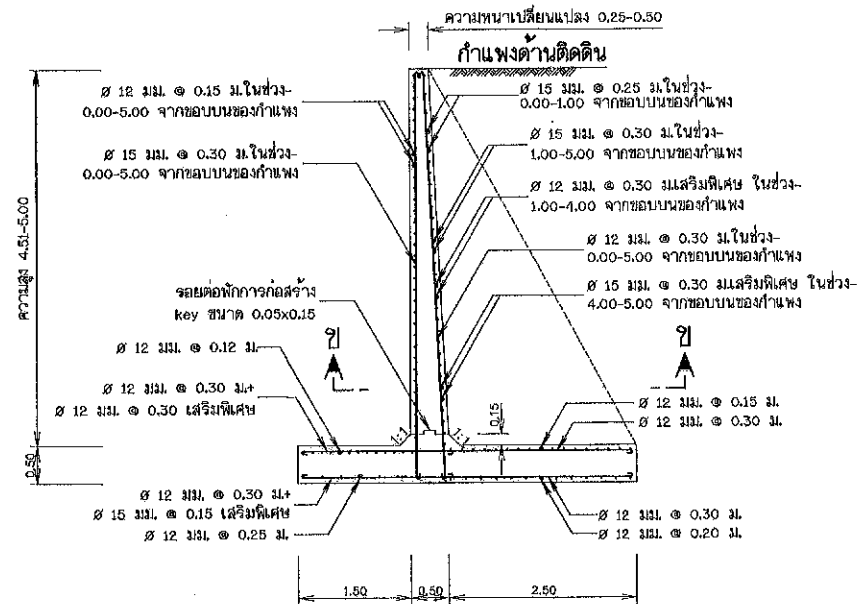
รูปตัดตามขวางของกำแพงบึงค้ำยัน
