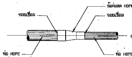
การบรรจุบดท่อ HDPE กับข้อลดท่อ HDPE
