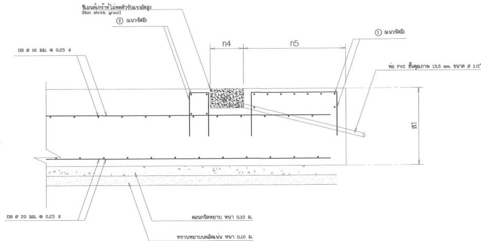
แบบขยายเหล็กเสริมรอบฐานรับดึงเค็ลอบแก้ว Fusion Bonded Epoxy (FBE) มาตราส่วน 1:25
