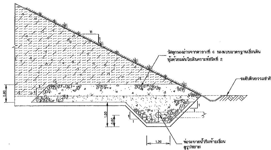
รูปขยายท่อระบายน้ำซึมท้ายเขื่อน มาตราส่วน 1:50
