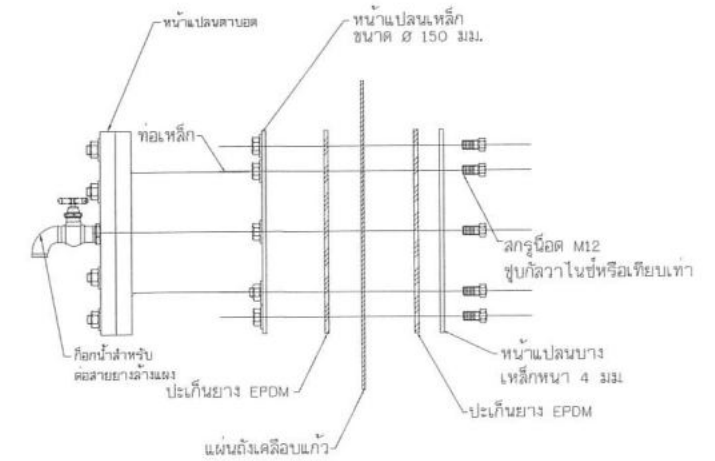
แบบขยายหน้าแปลนดาดบด scale NTC.
