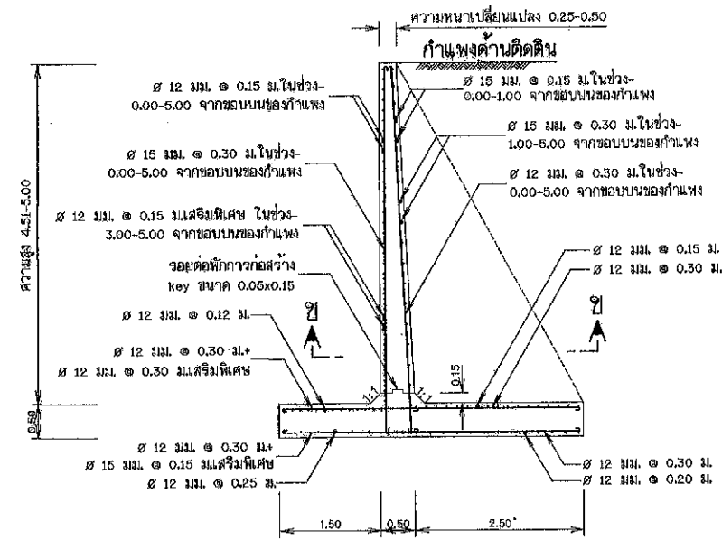
รูปตัดตามขวางของกำแพงบึงกลางช่วง
