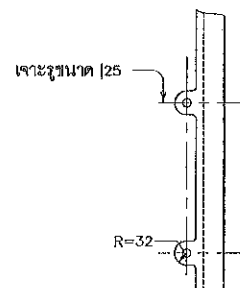
รูปขยายเหล็กนําร่อง มาตราส่วน 1:10
