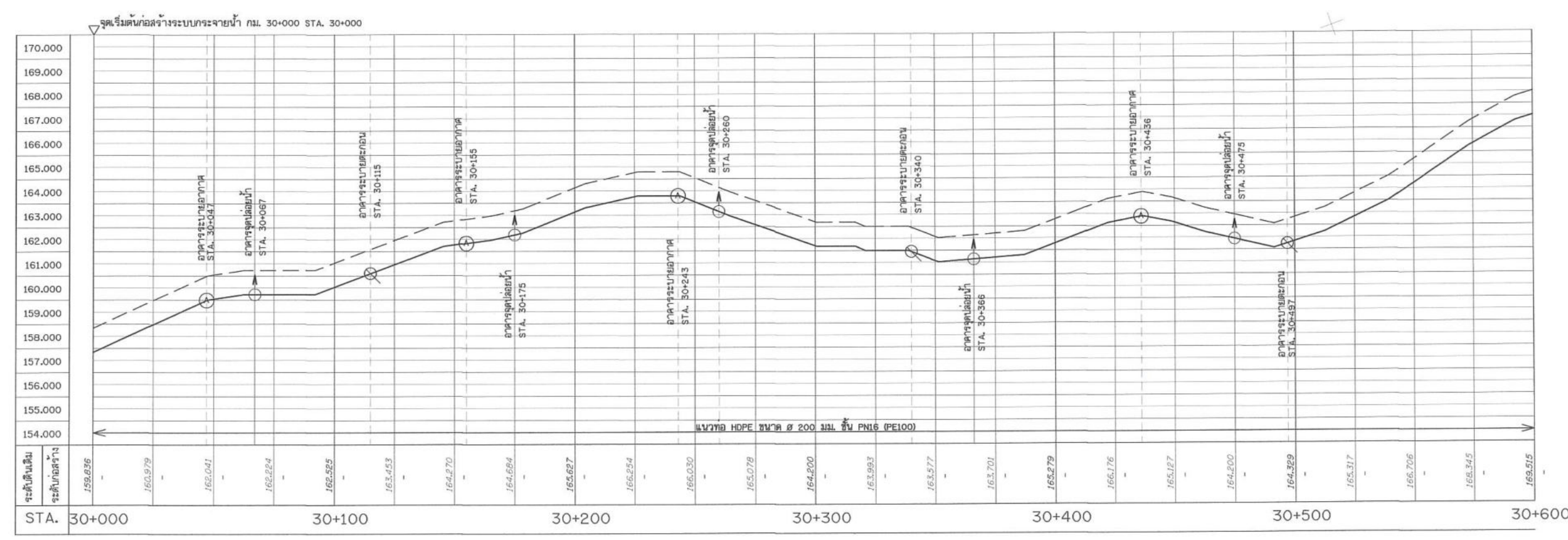
แปลนทั่วไป กม. 30+000 STA. 30+000 - 30+600 มาตรฐาน 1:1,000
