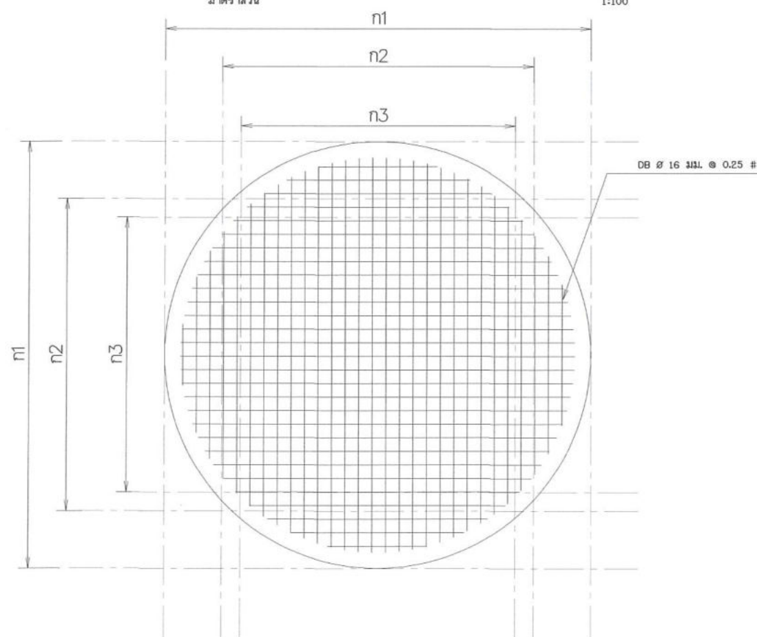
แปลนเหล็กเสริมชั้นบน รับถังเก็บน้ำ Fusion Bonded Epoxy (FBE)
