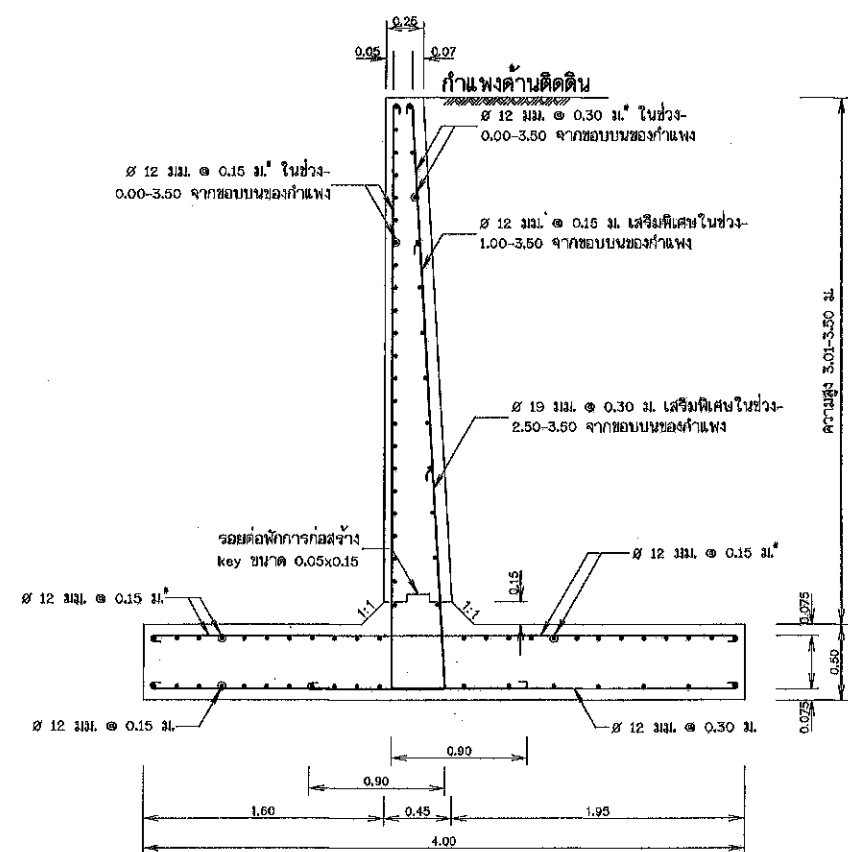
รูปขยายก้ำพังก้านตติดินความสูงระหว่าง 3.01-3.50 เมตร
