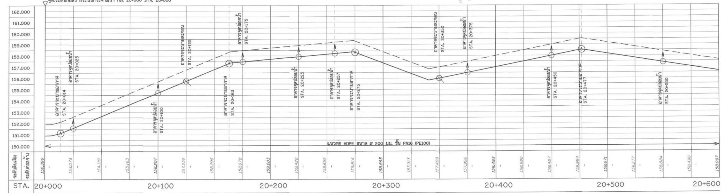
รูปตัดตามแนวยาว กม. 20+000 STA. 20+000 - 20+600 มาตราส่วน 1:1,000
