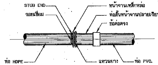
การบรรจุบดท่อ HDPE กับท่อ PVC.
