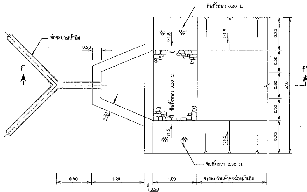
แปลนอาคารระบายน้ำซึมท้ายเขื่อน มาตราส่วน 1:25
