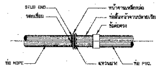
การบรรจุบดท่อ HDPE กับท่อ PVC.
