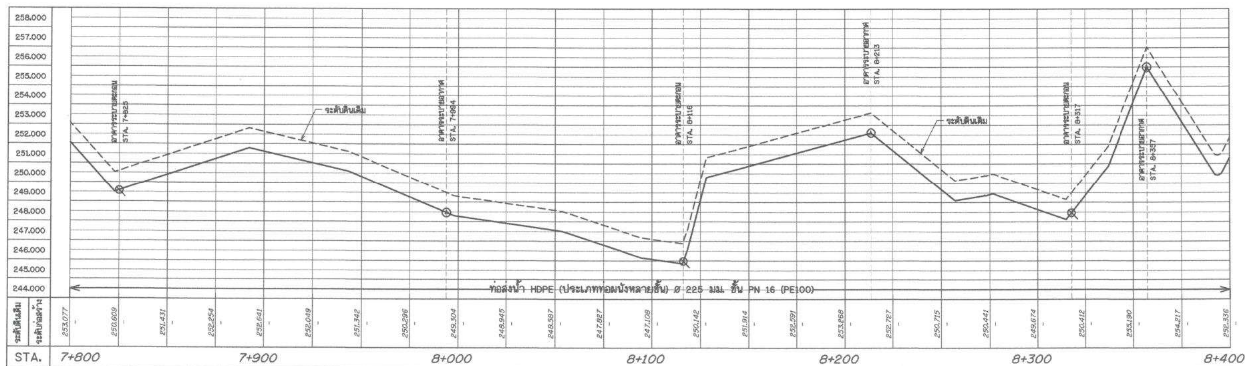
รูปตัดตามแนวยาวระบบกระจายน้ำ สาย RMP1 STA. 7+800 - 8+400
