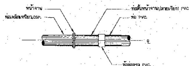
การบรรจบท่อเหล็กพินิวหรือ GSP. กับท่อ PVC.
