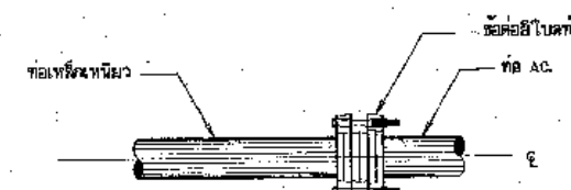
การบรรจบท่อเหล็กพินิวกับท่อ AC.
