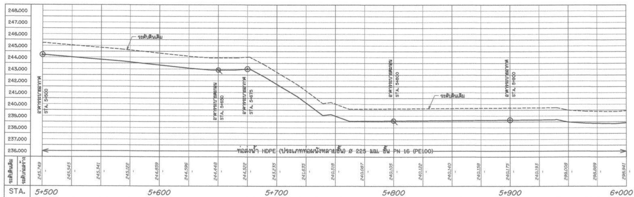
รูปตัดตามแนวยาวระบบกระจายน้ำ สาย RMP1 STA. 5+500 - 6+000
