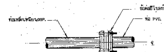
การบรรจบท่อเหล็กพินิวหรือ GSP. กับท่อ PVC.
