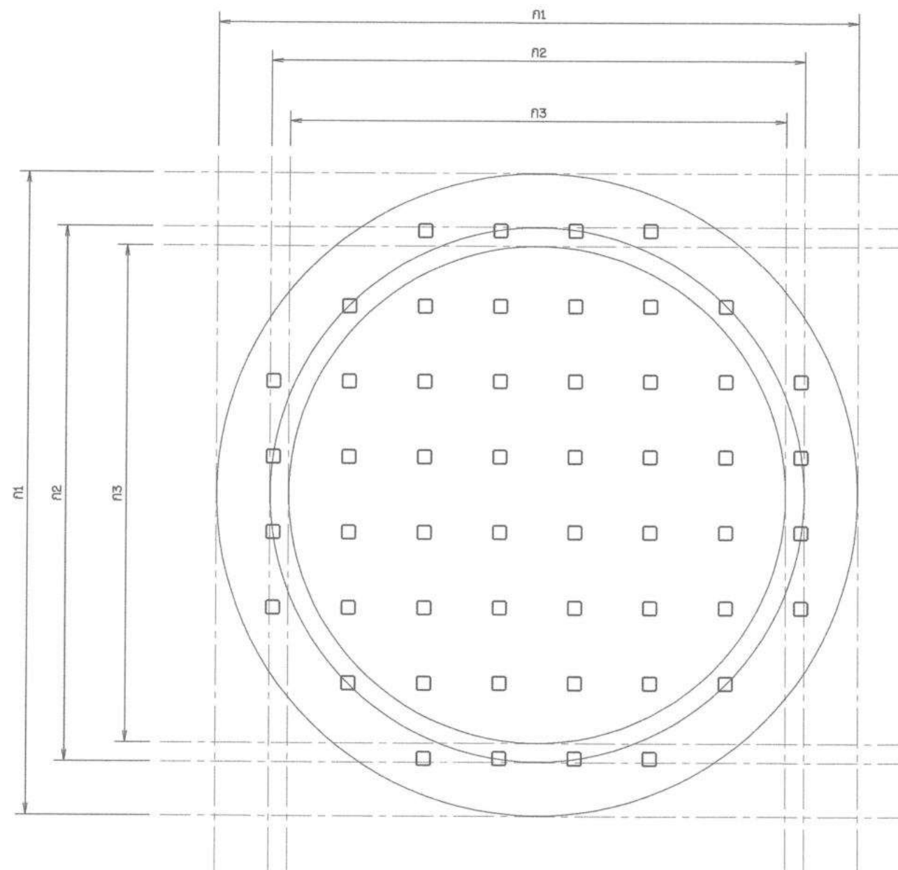
แปลนเสาสีม ถึงเก็บน้ำ Fusion Bonded Epoxy (FBE) ขนาด 1,100 ลบ.ม. มาตราส่วน 1:100
