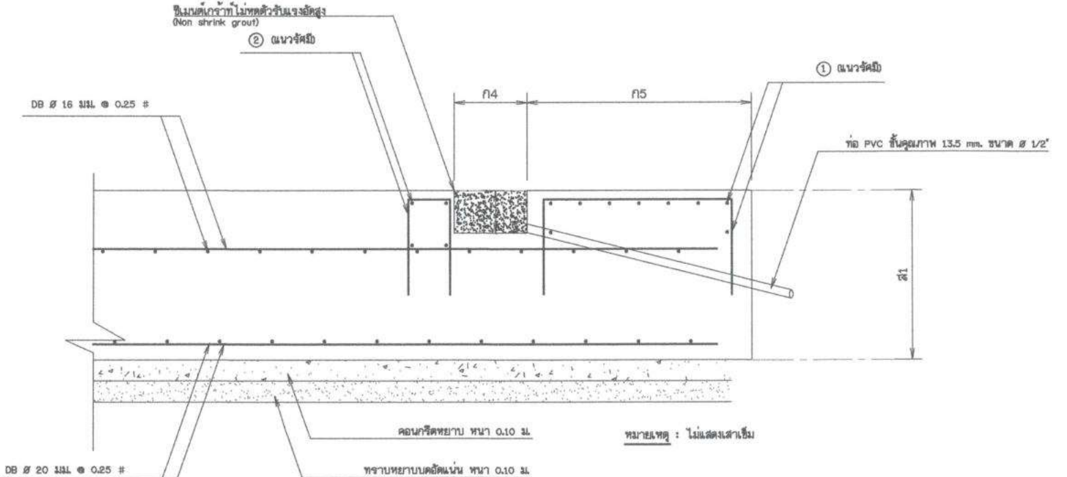
แบบขยายเหล็กเสริมรอบฐานรับถังเก็บน้ำ Fusion Bonded Epoxy (FBE) มาตราส่วน 1:25
