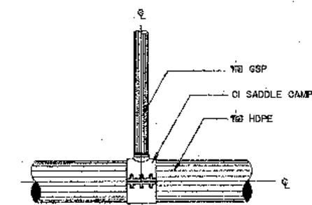
การบรรจุบดท่อสามทาง HDPE กับท่อ GSP
