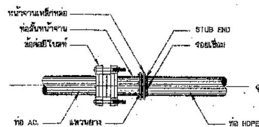
การบรรจุบดท่อ AC กับท่อ HDPE
