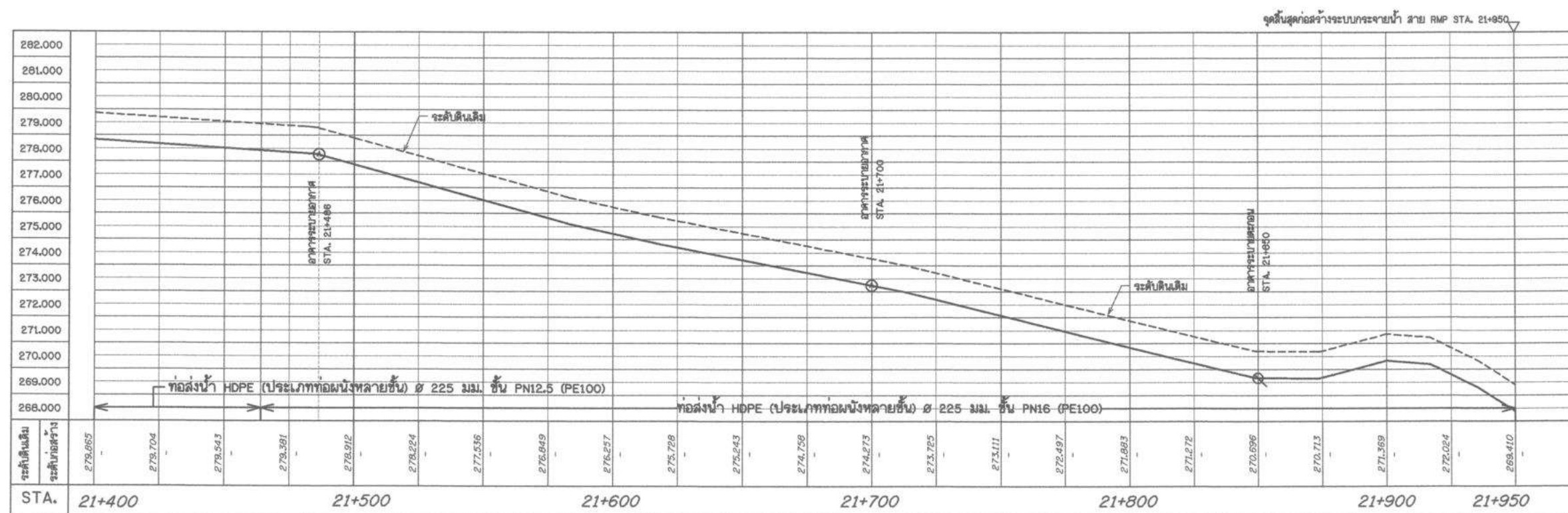
รูปตัดตามแนวยาวระบบกระจายน้ำ สาย RMP STA. 21+400 - 21+950 มาตราส่วน 1:1,000
