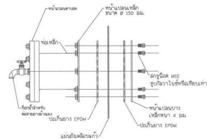
แบบขยายหน้าแปลนคานอด scale NTC.
