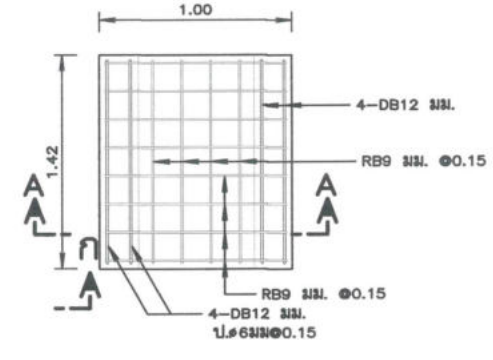
แบบขยาย พื้นสะพาน
