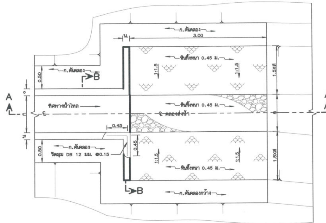
แผนจุดสิ้นสุดคลองส่งน้ำ
