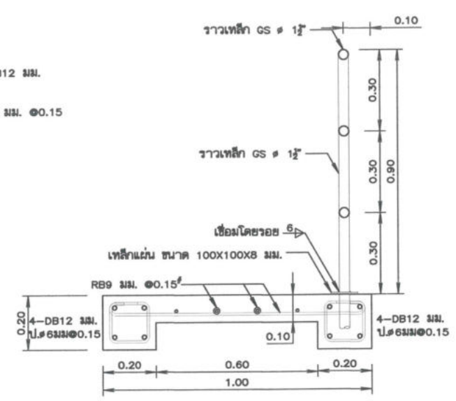
รูปตัดแนว A - A
