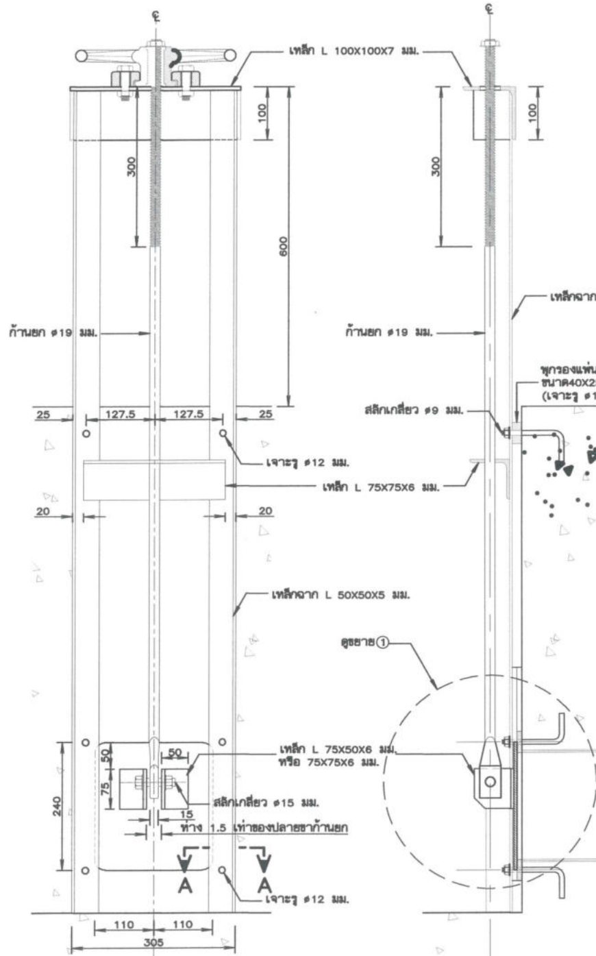
แสดงกาติดตั้ง มาตราส่วน 1:5
