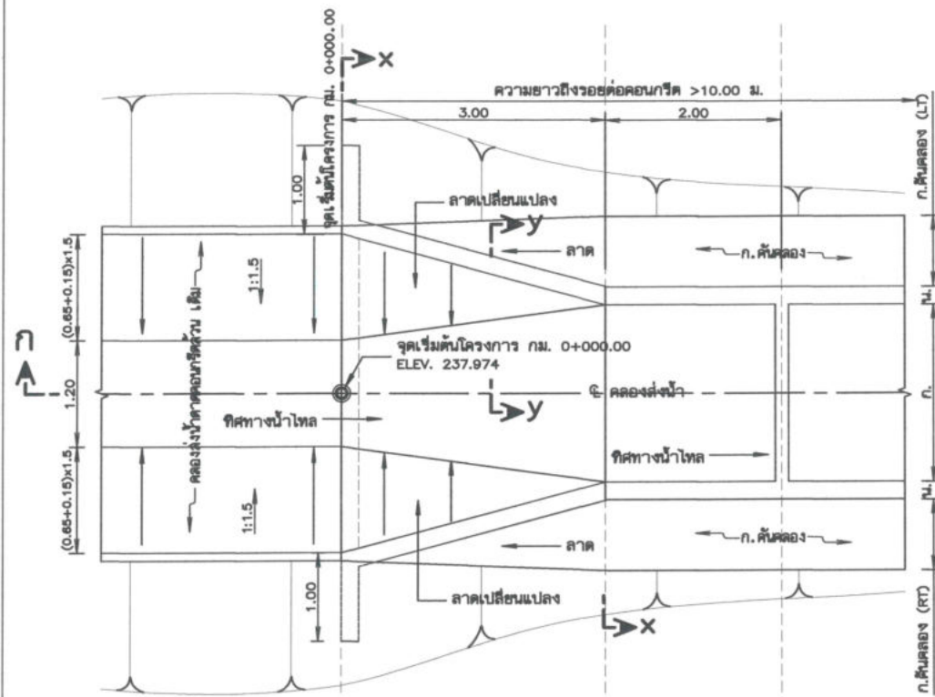
แผนจุดเริ่มต้นคลองส่งน้ำ
