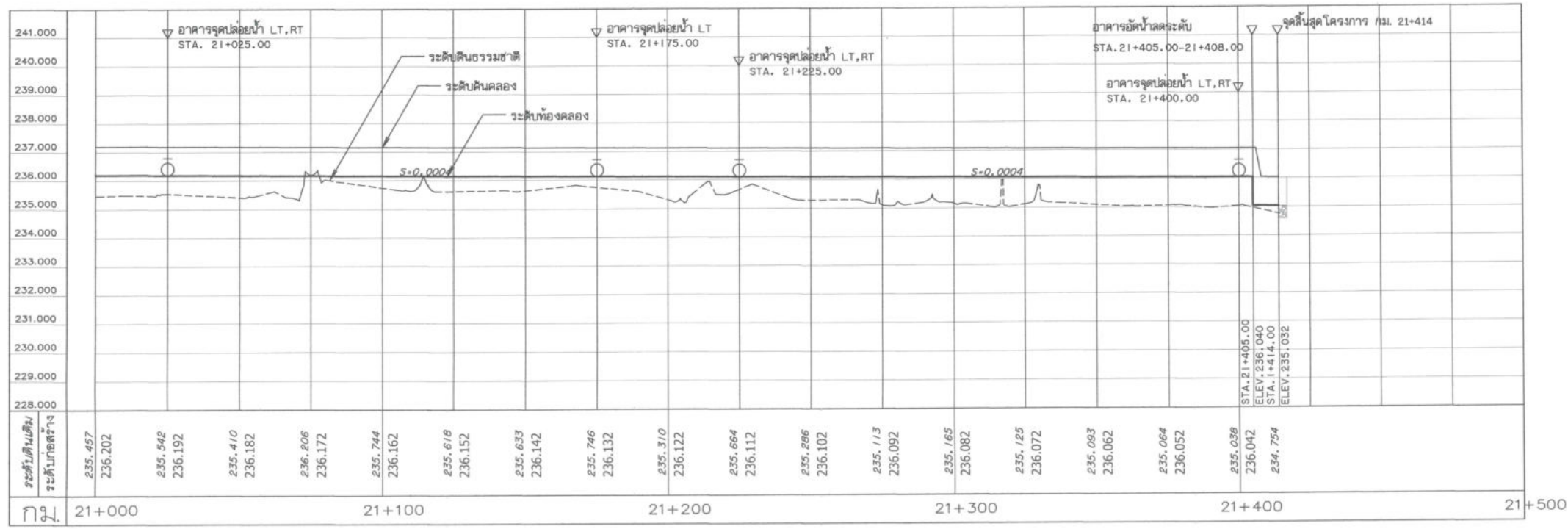
รูปตัดตามแนวยาว สาย R-RMC มาตราส่วน 1:1,000 แนวยาว 1:1,000
