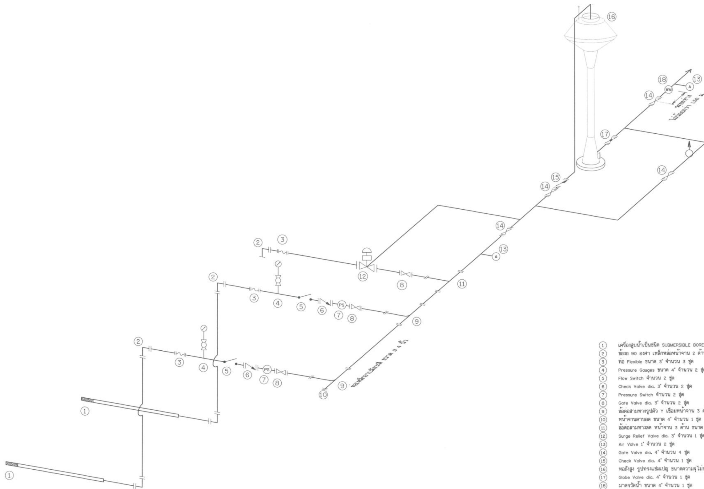
แผนผังระบบสูบน้ำด้วยพลังงานแสงอาทิตย์
