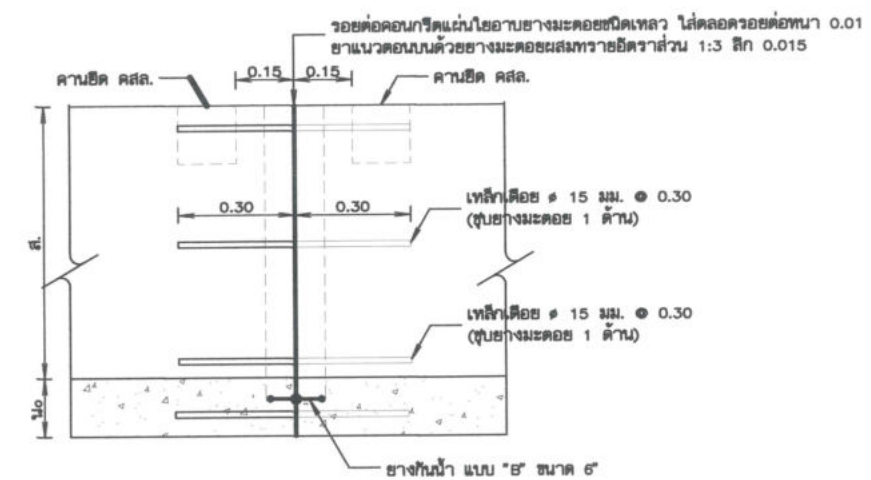
รูปตัดแสดงรอยต่อ
