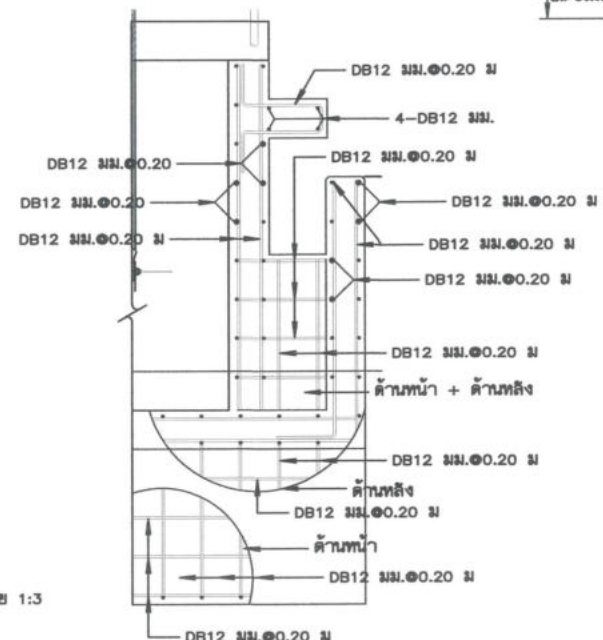
รูปตัดแนว ค - ค
