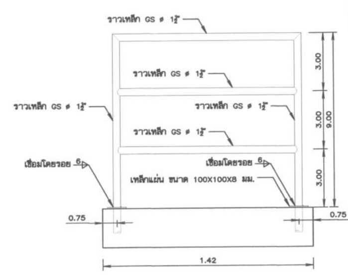
ขยายราวกันตก
