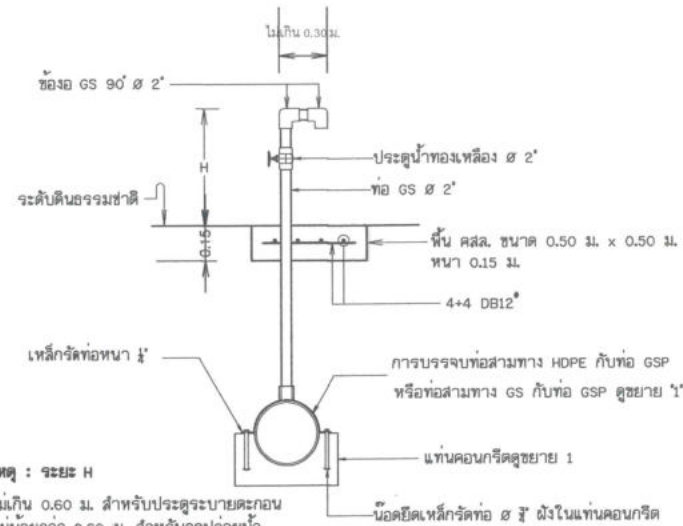
รูปตัดอาคารประตูลอยตะกอน
