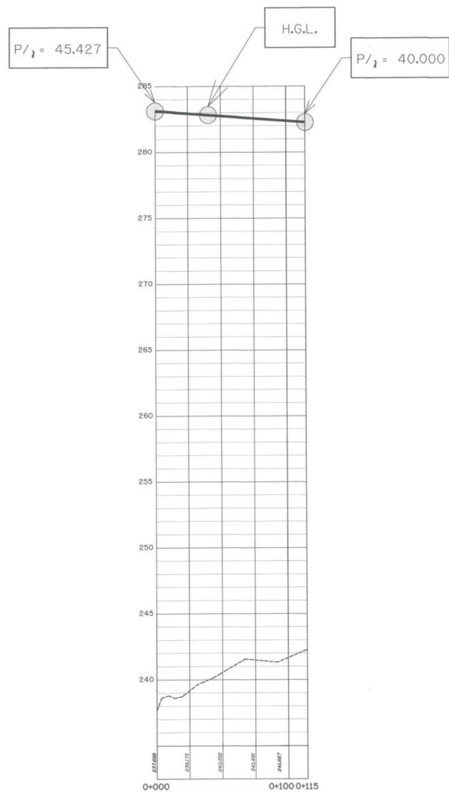
รูปตัดตามแนวยาวแสดง H.G.L. สาย RMP STA. 0+000 - 0+115 โมเดลงานมาตรฐาน
