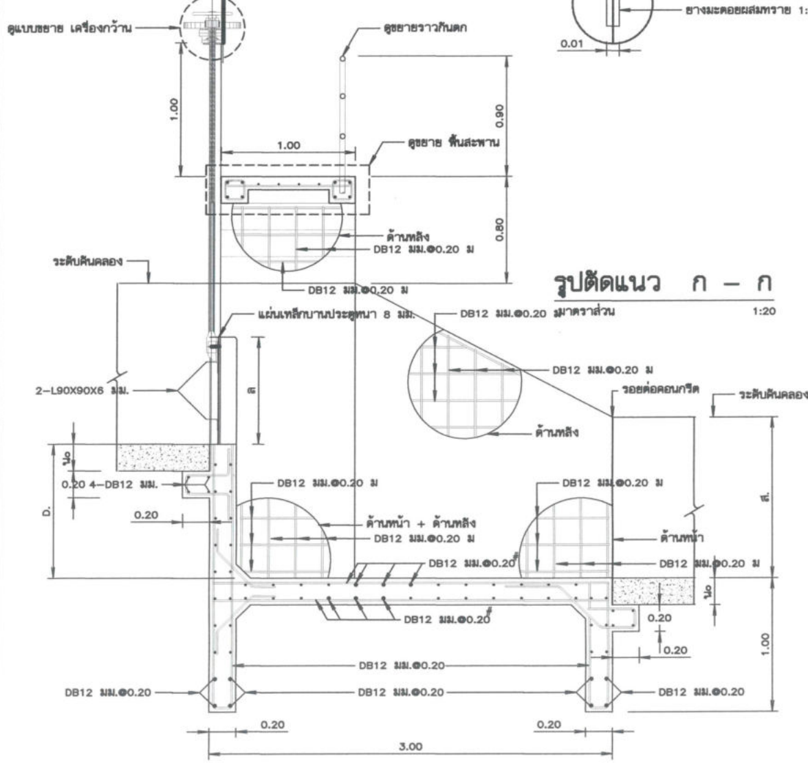
แบบอาคารยึดน้ำลดระดับ
