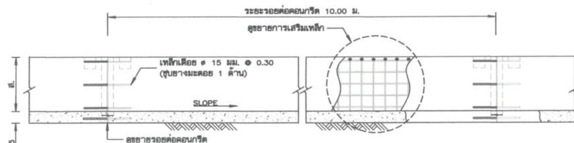
รูปตัดแนว ก - ก
