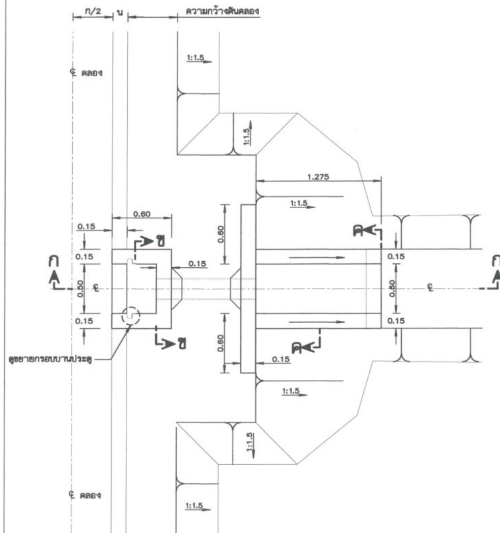
แปลนอาคารท่อส่งน้ำเข้านา มาตราส่วน 1:20
