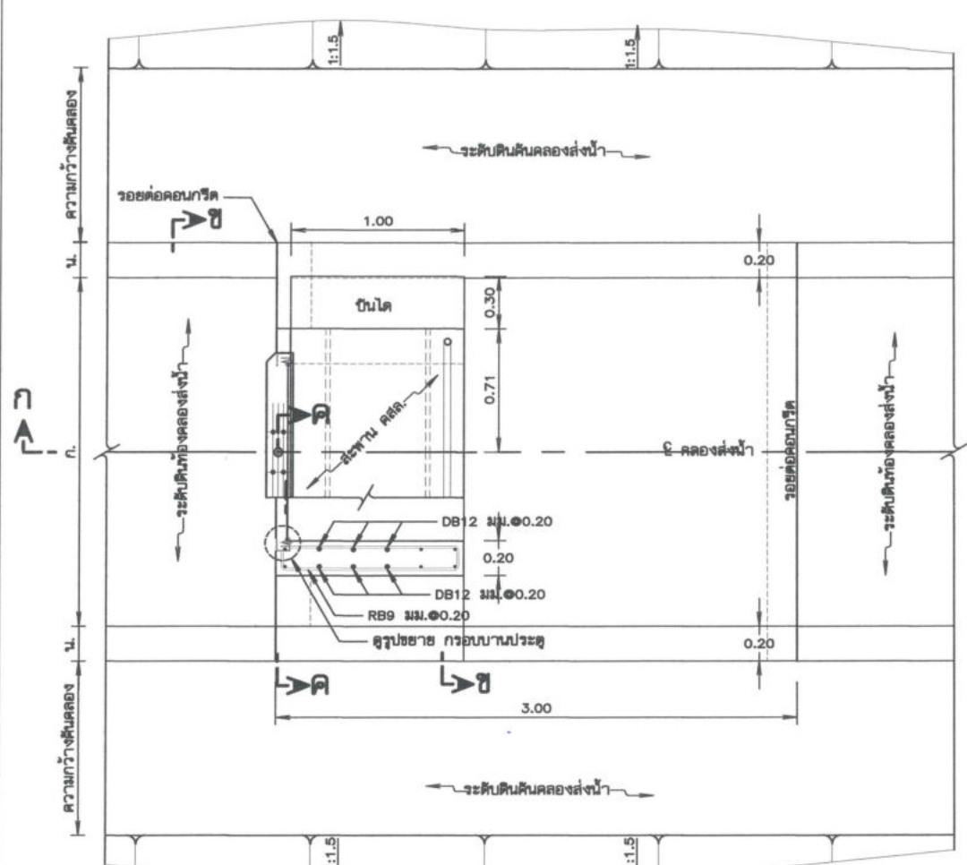
แบบอาคารยึดน้ำลดระดับ
