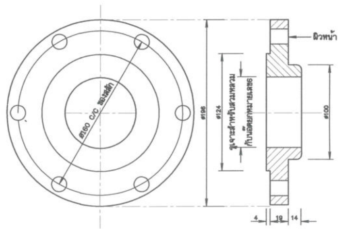
แผ่นปิดเหล็กหล่อ 4 มาตราส่วน 1:2
