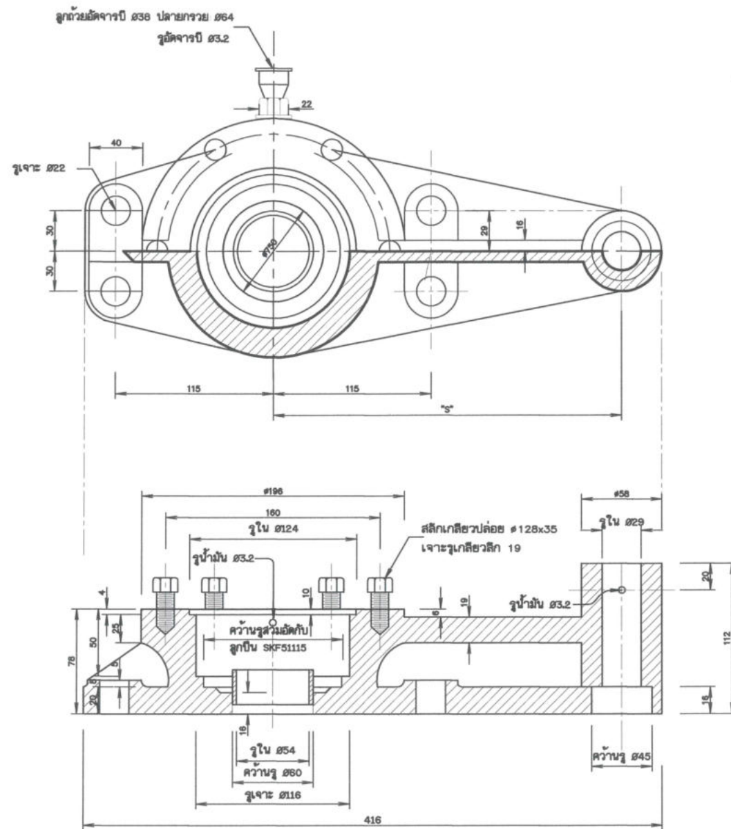
ฐานเหล็กหล่อ 5 มาตราส่วน 1:2
