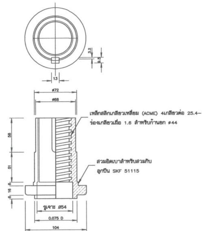
ปั๊มเกลียวยก บรอนซ์ 6 มาตราส่วน 1:2
