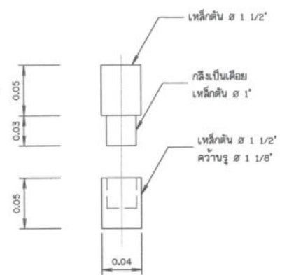
แบบขยายบานพับน๊ัทเหล็ก
