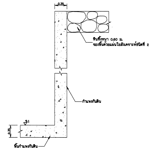
รูปตัด ค-ค
