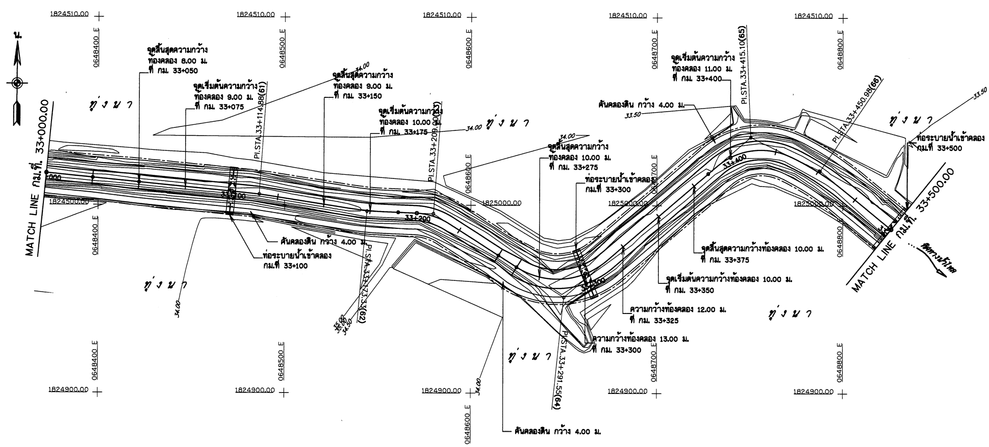
แปลนชุดลอกคลอง สาย 4MC กม.ที่ 33+000.00 - 33+500.00 มาตราส่วน 1:1,000
