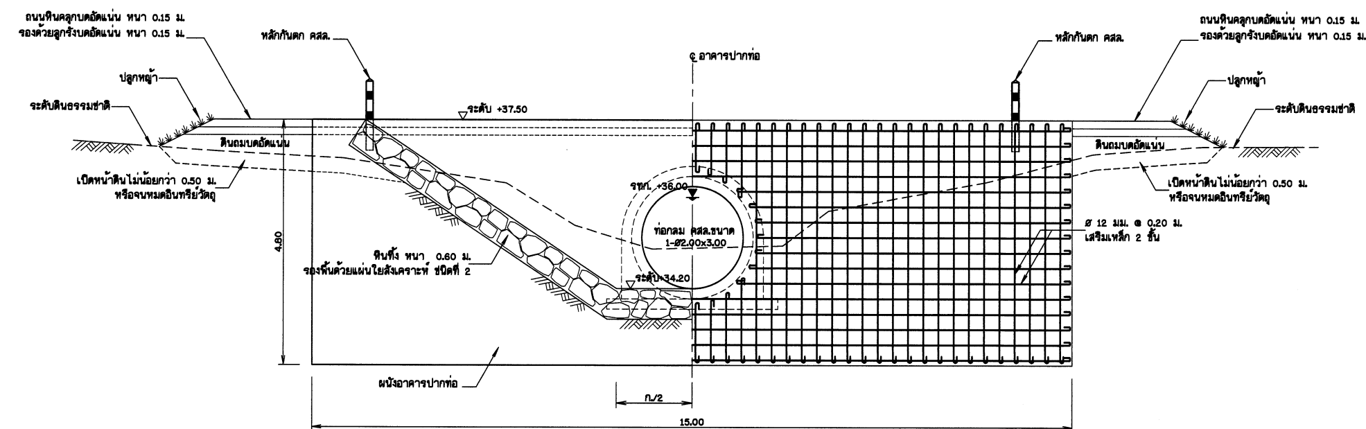
รูปตัด ค-ค มาตราส่วน 1:50
