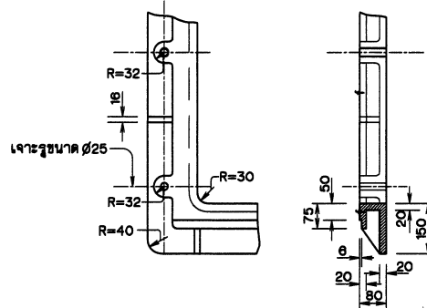
รูปขยายกรอบบาน มาตราส่วน 1:10
