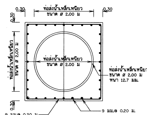
รูปขยายคอนกรีตบล็อกปิดหัว
