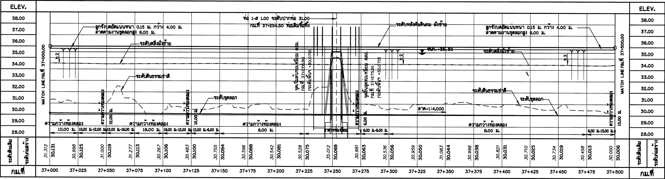
รูปตัดตามยาวชุดลอกคลอง สาย 4MC. กม.ที่ 37+000.00 - 37+500.00
