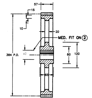
รูปตัด ค - ค
