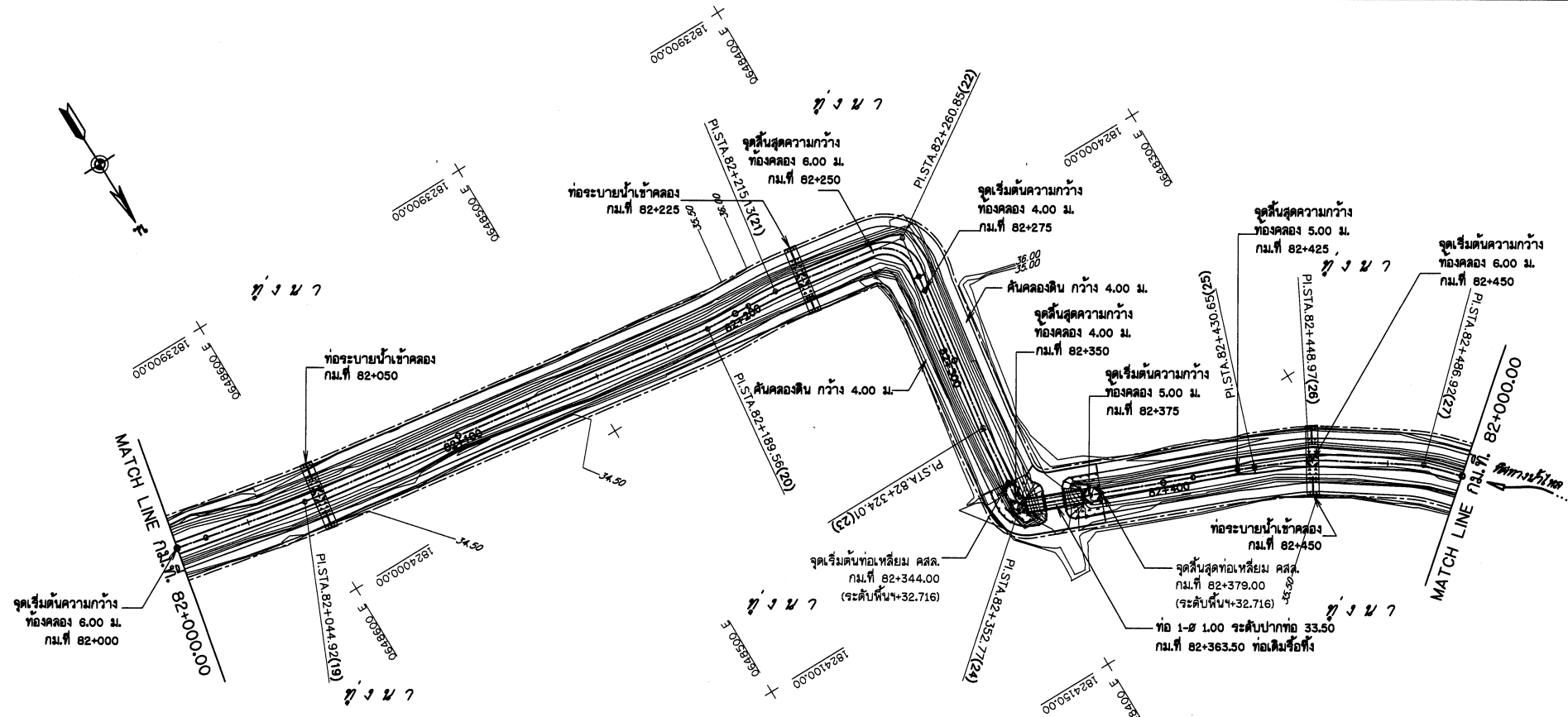
แปลนขุดลอกคลอง สาย 2R-4MC กม.ที่ 82+000.00 - 82+500.00
