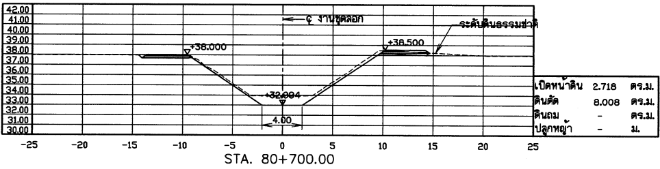
รูปตัดแสดงงานดินขุดลอกคลองสาย 1R-4MC. กม.ที่ 80+700.00-80+729.00
