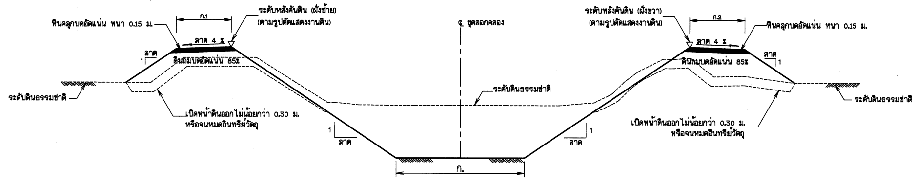
รูปตัดทั่วไปขุดลอกคลองเมื่อเป็นคันดินถม มาตราส่วน 1:50
