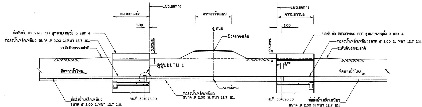
รูปตัด ก-ก
