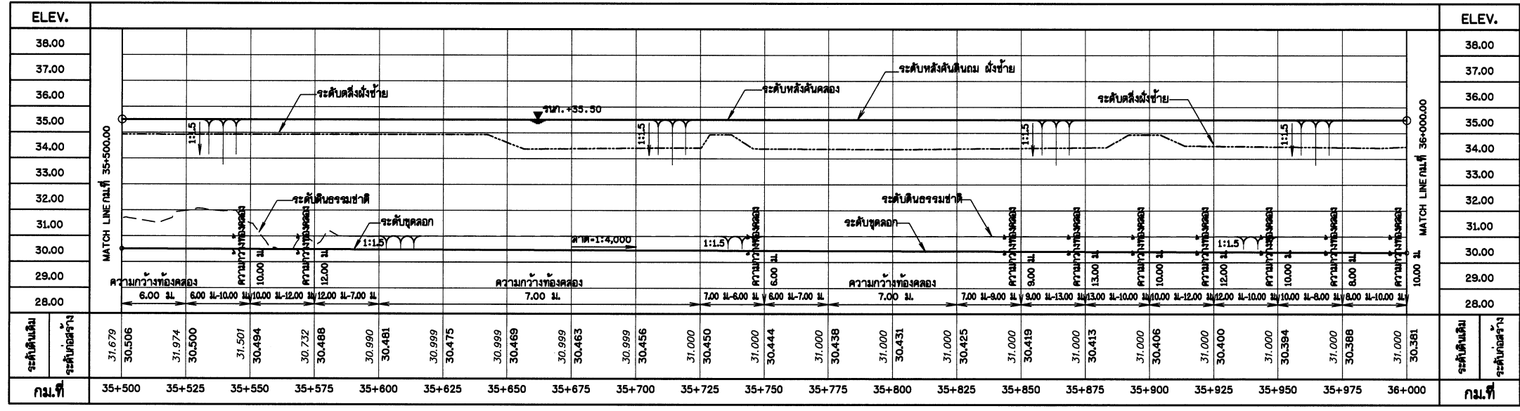
รูปตัดตามยาวขุดลอกคลอง สาย 4MC. กม.ที่ 35+500.00 - 36+000.00 มาตรฐาน 1:100 แนวตั้ง 1:100 แนวนอน 1:1,000
