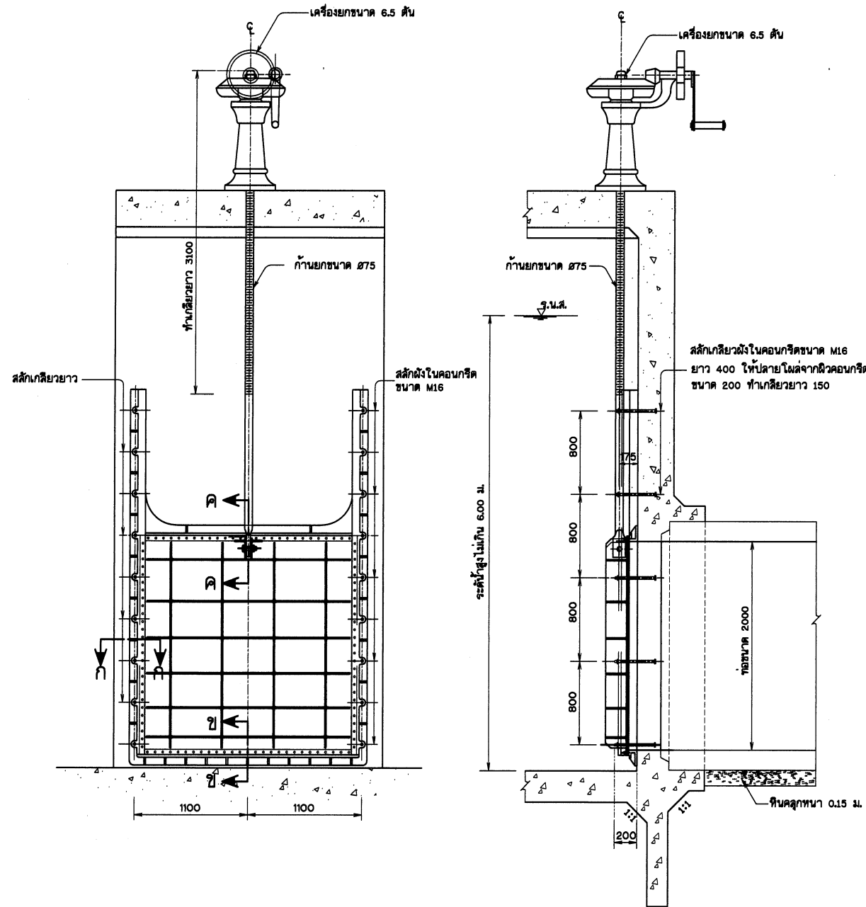
การประกอบและติดตั้งงาน มาตรฐาน 1:25
