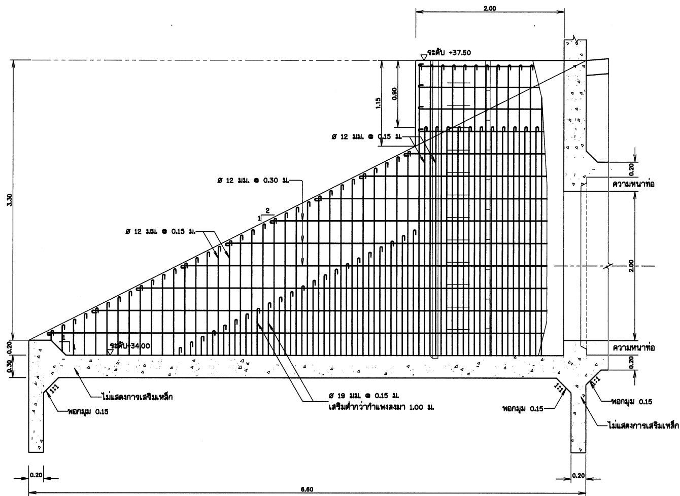
การเสริมเหล็กกำแพงอาคารอัดน้ำ
