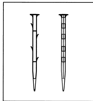
รูปที่ 4 หมุดยึด (Pin) ทำจาก POLYPROPYLENE มีขนาดความยาวไม่น้อยกว่า 240 mm. ความกว้างของหมุดทั้งสองด้านไม่น้อยกว่า 14 mm. หัวหมุดเส้นผ่าศูนย์กลางไม่น้อยกว่า 28.00 mm. ลำตัวของหมุดมีก้าน 4 ก้าน และระบุชื่อผู้ผลิตอย่างชัดเจนบนตัวหมุด
