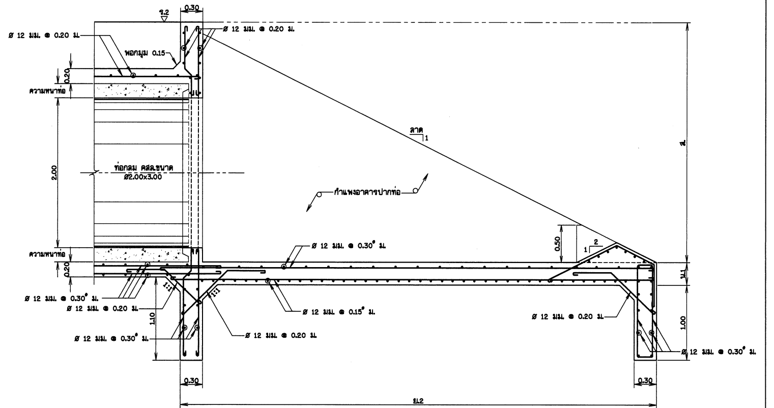
การเสริมเหล็กพื้นอาคารปากท่อ มาตราส่วน 1:25
