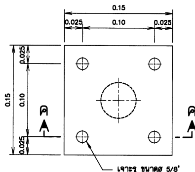
รูปขยายแผ่นเหล็กหน้าแปลน มาตราส่วน 1:10
