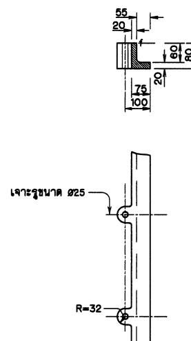
รูปขยายเหล็กนาร่อง มาตราส่วน 1:10
