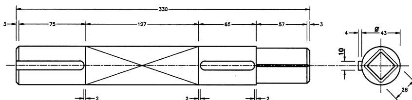
เพลาชัก (เหล็กเหล็กรีดเย็น)
