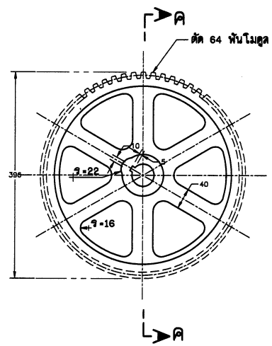
เฟืองใหญ่ (เหล็กหล่อ)
