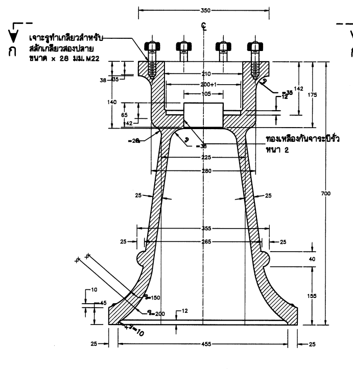
แท่น (เหล็กหล่อ)
