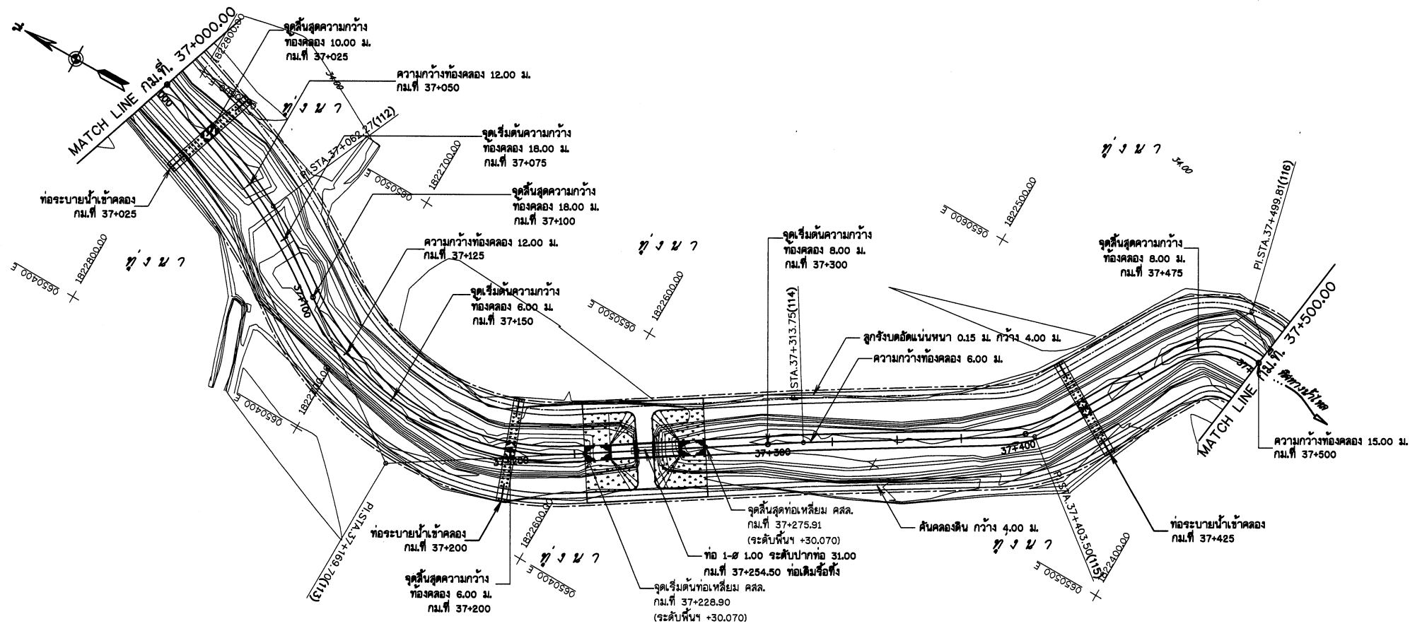
แปลนชุดลอกคลอง สาย 4MC กม.ที่ 37+000.00 - 37+500.00
