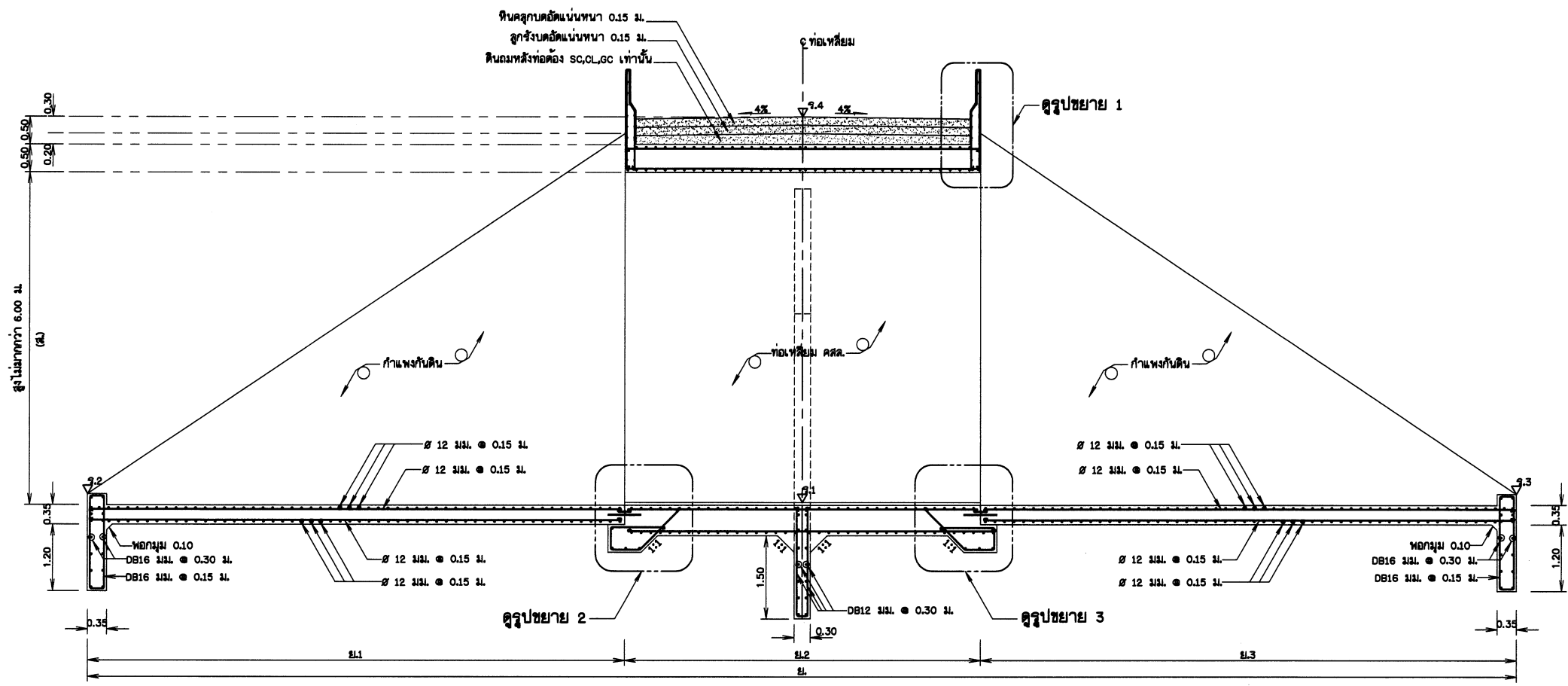
รูปตัดตามยาวแสดงการเสริมเหล็ก
