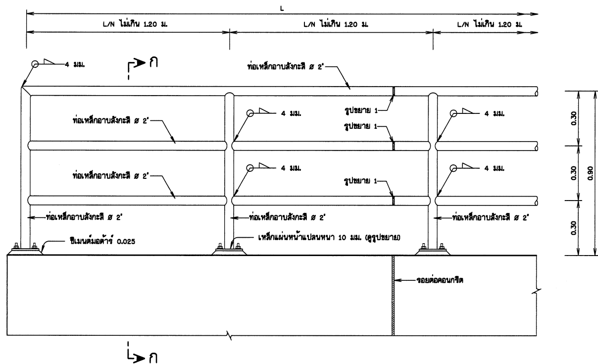
จาวเหล็กกันตก มาตราส่วน 1:10
