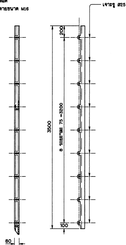
เหล็กนำร่องเหล็กเหนียว มาตราส่วน 1:20
