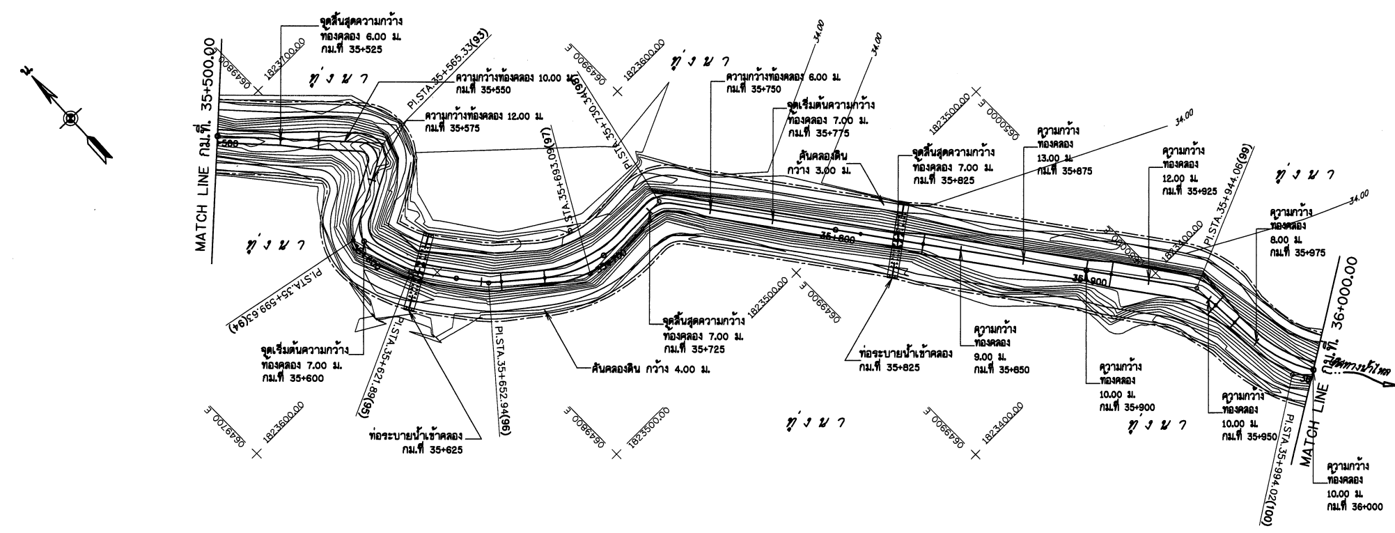
แปลนขุดลอกคลอง สาย 4MC กม.ที่ 35+500.00 - 36+000.00 มาตรฐาน 1:1,000
