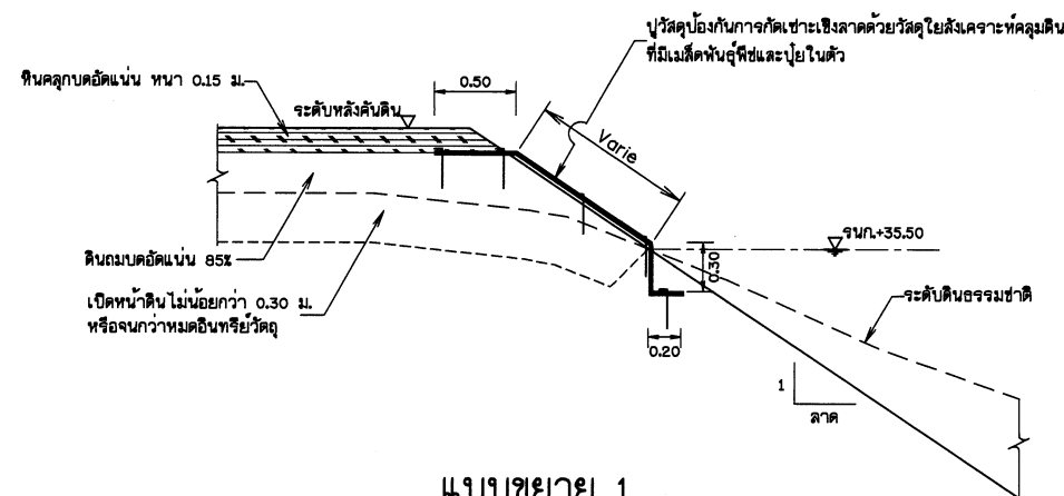
แบบขยาย 1 ไม่แสดงมาตราส่วน
