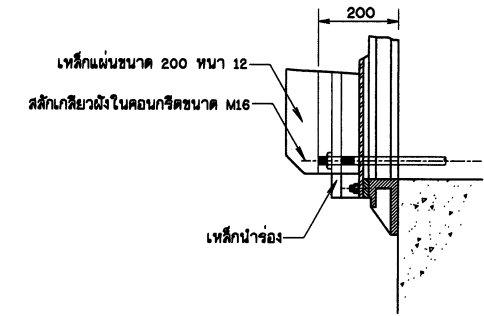
รูปตัด ข - ข มาตรฐาน 1:10
