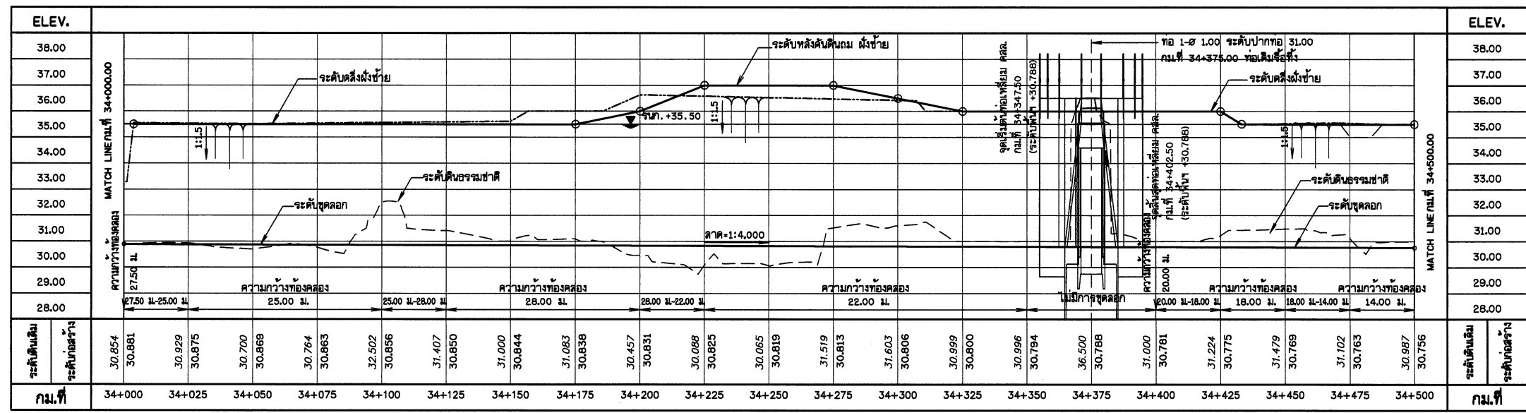
แปลนชุดลอกคลอง สาย 4MC กม.ที่ 34+000.00 - 34+500.00 มาตรฐาน 1:1,000
