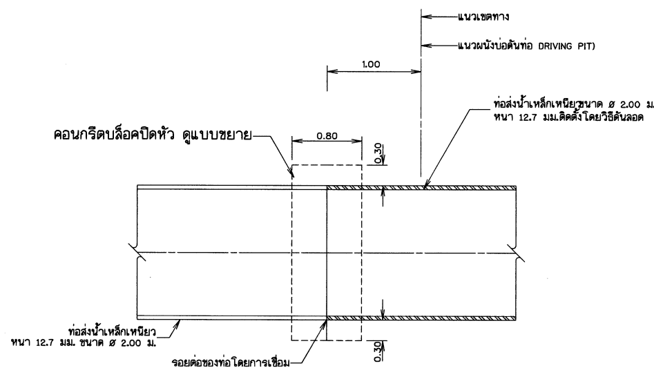
รูปขยาย 1
