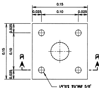
รูปขยายแผ่นเหล็กหน้าแปลน มาตราส่วน 1:10
