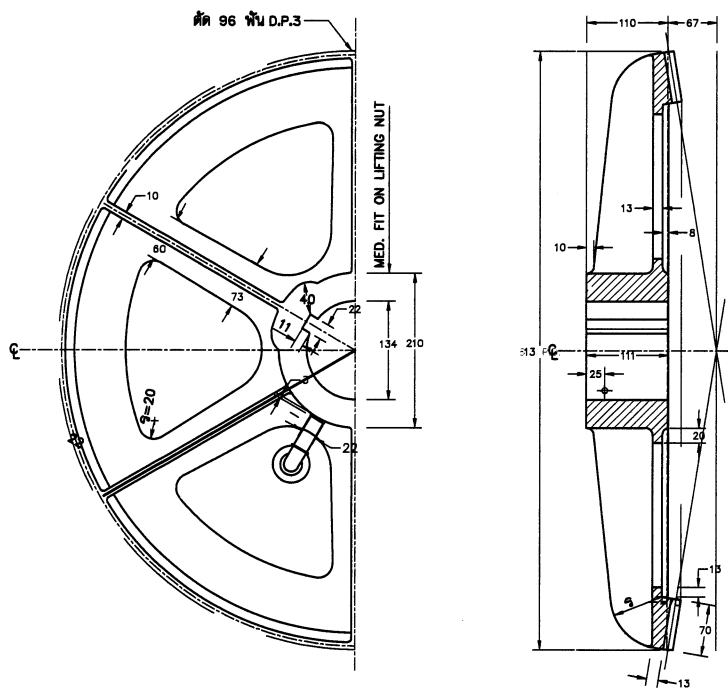
เพื่องดอกจอกใหญ่ (เหล็กหล่อ)
