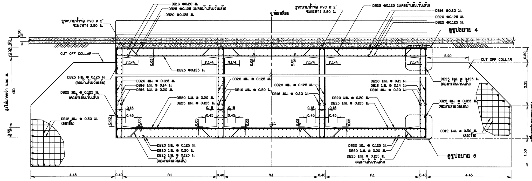
รูปตัดตามขวางแสดงการเสริมเหล็ก
