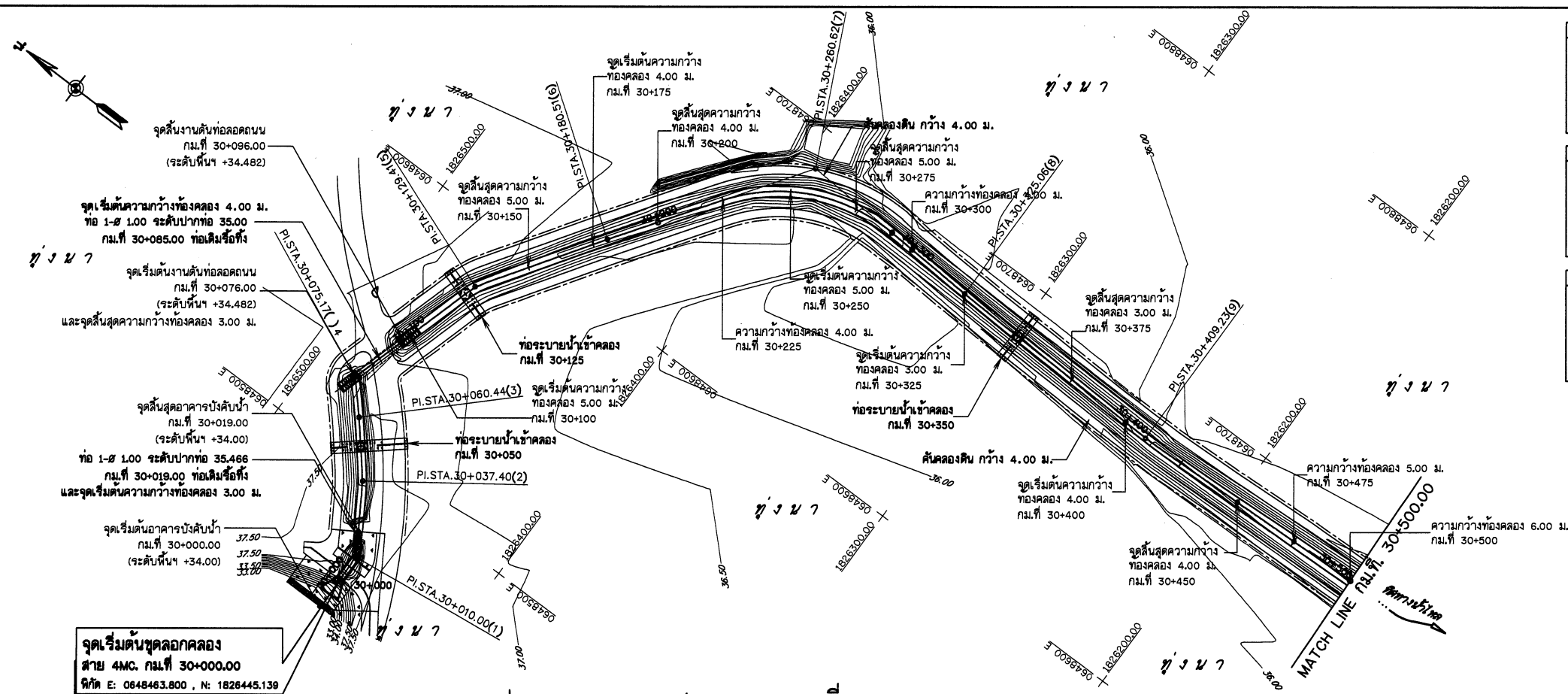
แปลนขุดลอกคลอง สาย 4MC กม.ที่ 30+000.00 - 30+500.00
