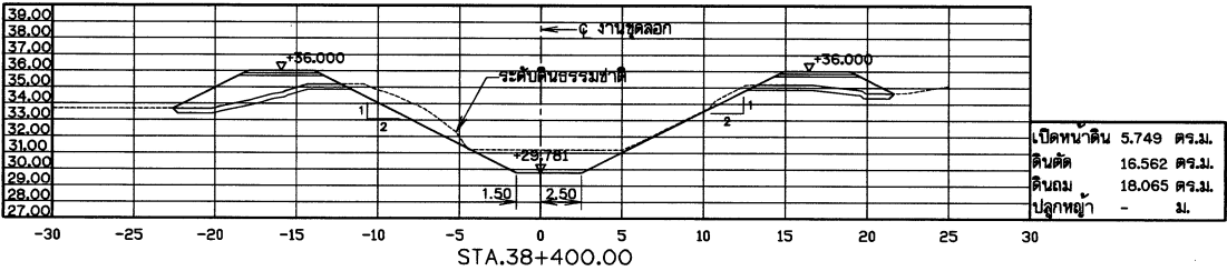
รูปตัดแสดงงานดินขุดลอกคลองสาย 4MC. กม.ที่ 38+400.00-38+420.76
