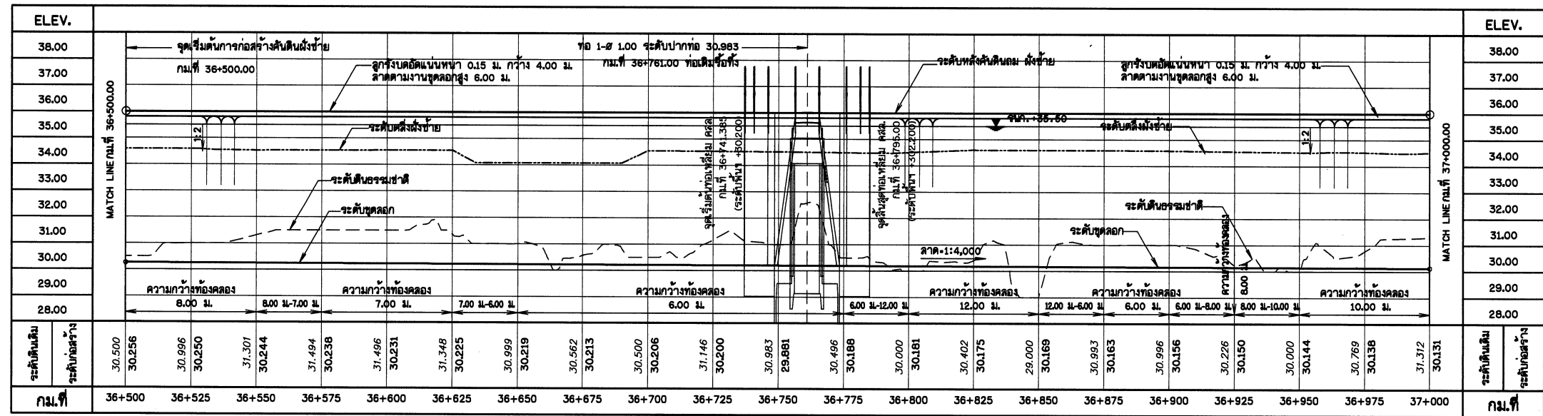
แปลนชุดลอกคลอง สาย 4MC กม.ที่ 36+500.00 - 37+000.00 มาตราส่วน 1:1,000
