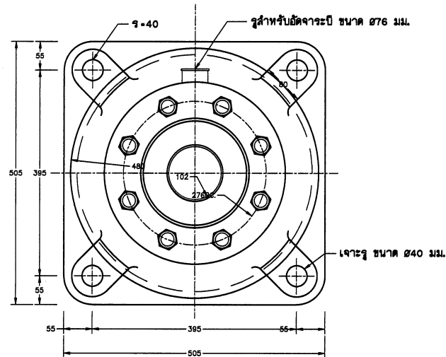
รูปตัด ก - ก
