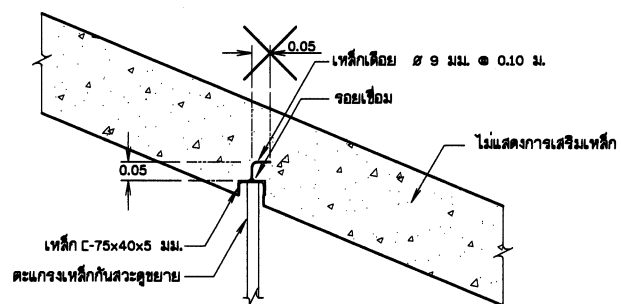
รูปขยายร่องใส่ตะแกรงกันสวะ มาตราส่วน 1:10
