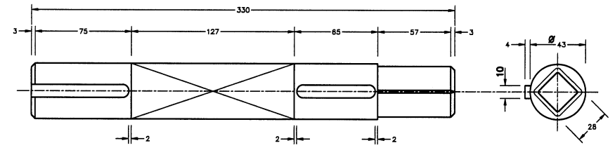
เพลากลางเฟืองดอกจอกเล็ก
