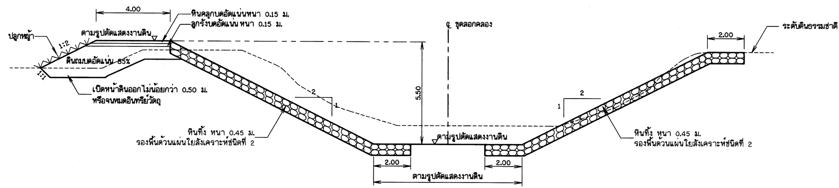
รูปตัดทั่วไปขุดลอกคลองช่วงเป็นหินทิ้ง หนา 0.45 ม. มาตราส่วน กม.ที่ 26+305.00 - 26+505.00 และ กม.ที่ 26+835.00 - 26+890.00 1:100
