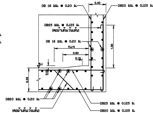
รูปขยาย 5 มาตราส่วน 1:20
