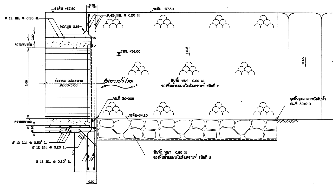
การเสริมเหล็กผนังอาคารปากท่อ มาตราส่วน 1:25
