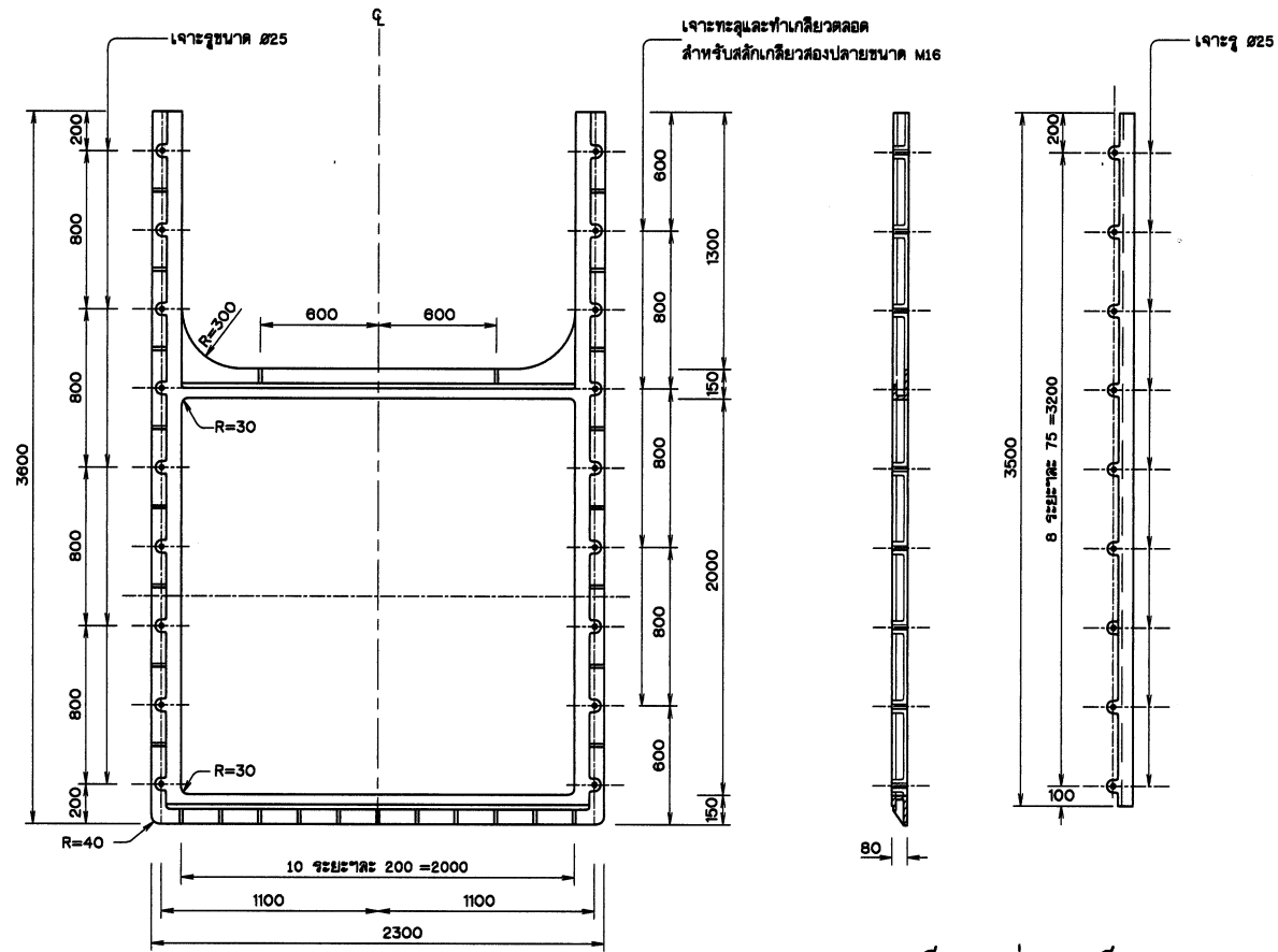
เหล็กนำร่องเหล็กเหล็ย มาตราส่วน 1:20
