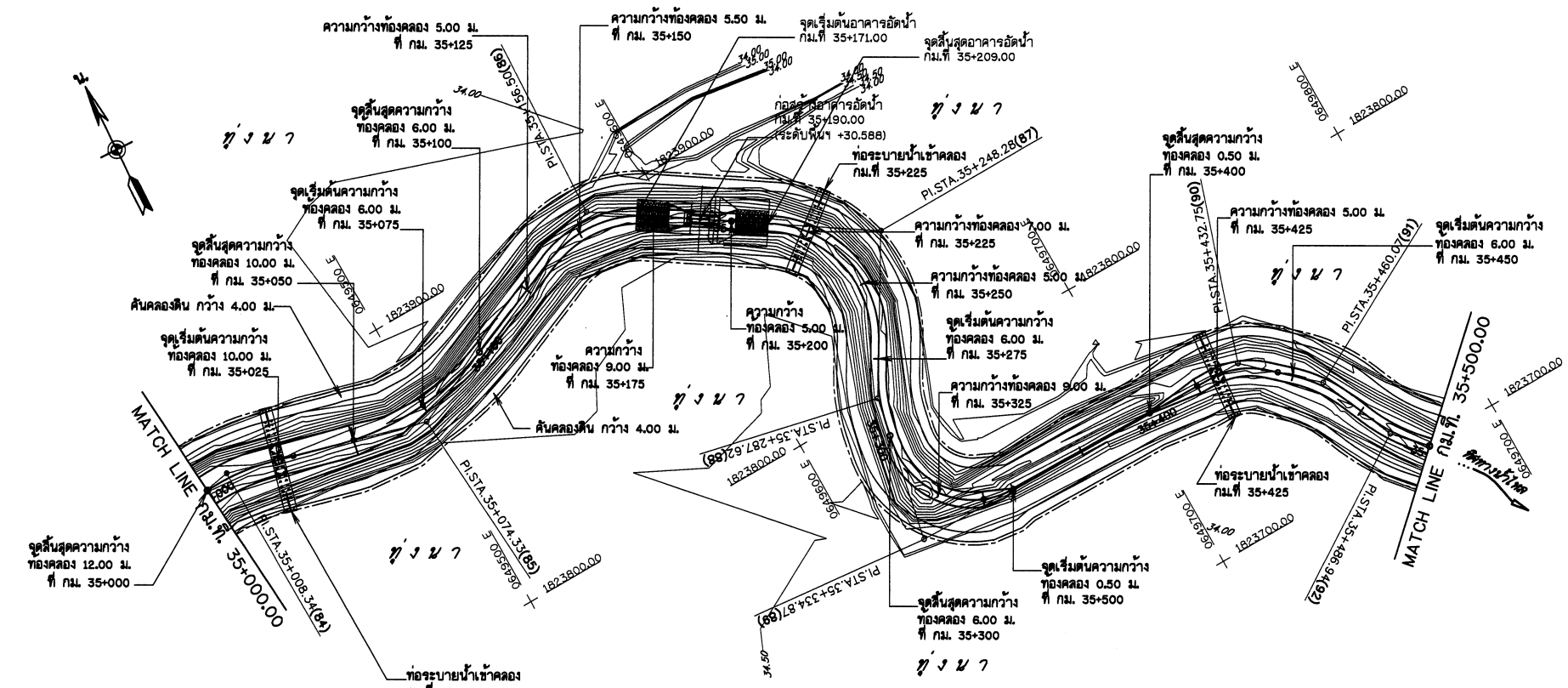
แปลนชุดลอกคลอง สาย 4MC กม.ที่ 35+000.00 - 35+500.00 1:1,000
