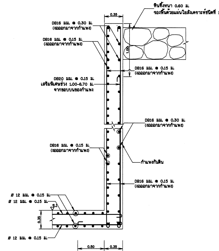
การเสริมเหล็กกำแพง มาตราส่วน (รูปตัด 3-3) 1:20
