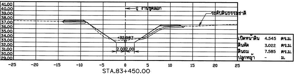
รูปตัดแสดงงานดินขุดลอกคลองสาย 2R-4MC. กม.ที่ 83+450.00-83+515.00
