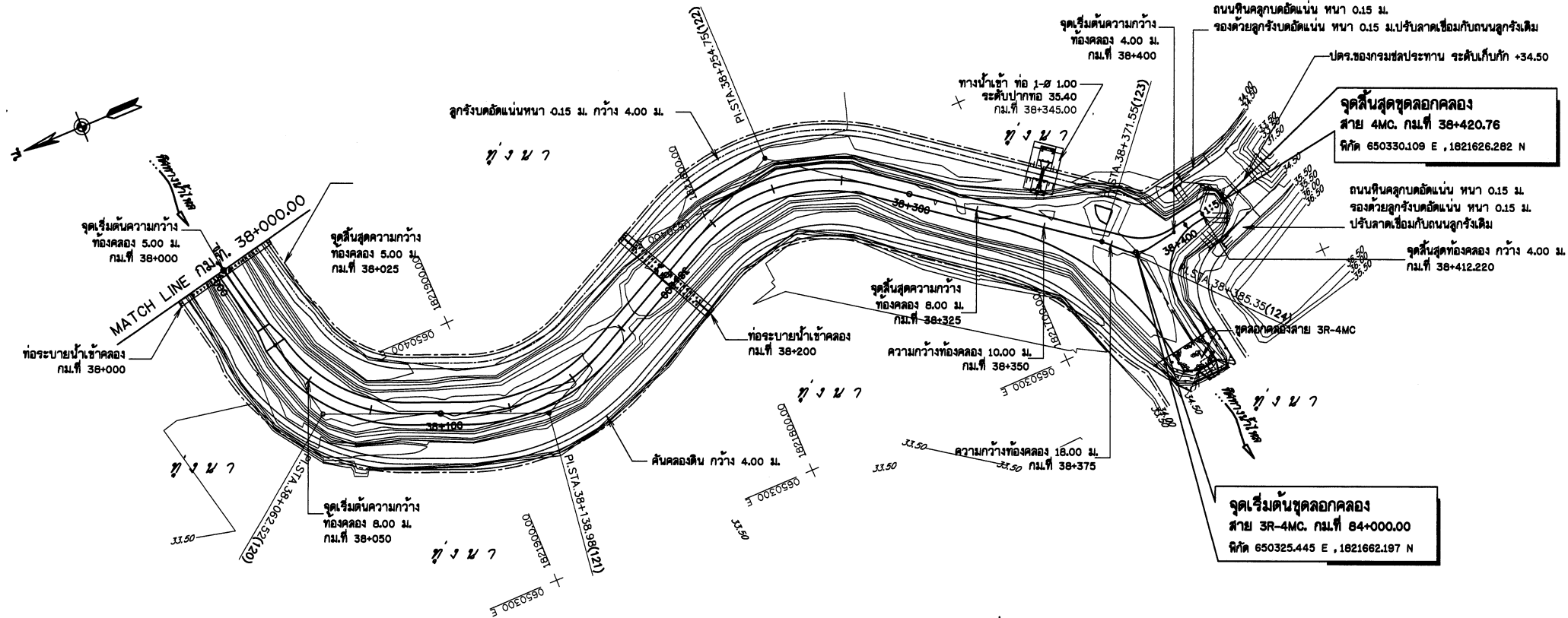
แปลนจุดดอกลอง สาย 4MC กม.ที่ 38+000.00 - 38+420.76
