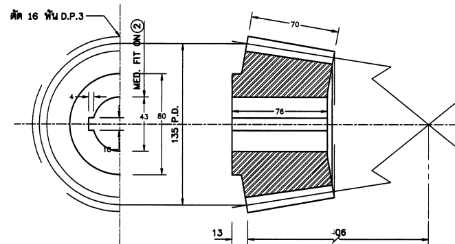
เพื่องดอกจอกเล็ก (เหล็กเหนียว)
