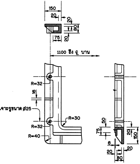
รูปขยายกรอบบาน มาตราส่วน 1:10
