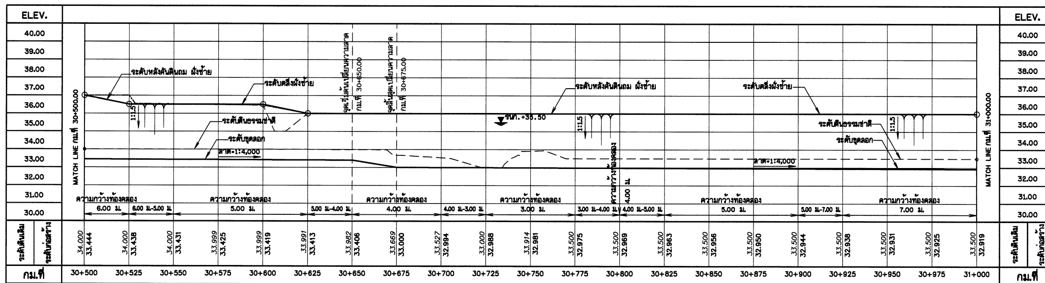
รูปตัดตามยาวขุดลอกคลอง สาย 4MC. กม.ที่ 30+500.00 - 31+000.00 มาตราส่วน 1:1,000
