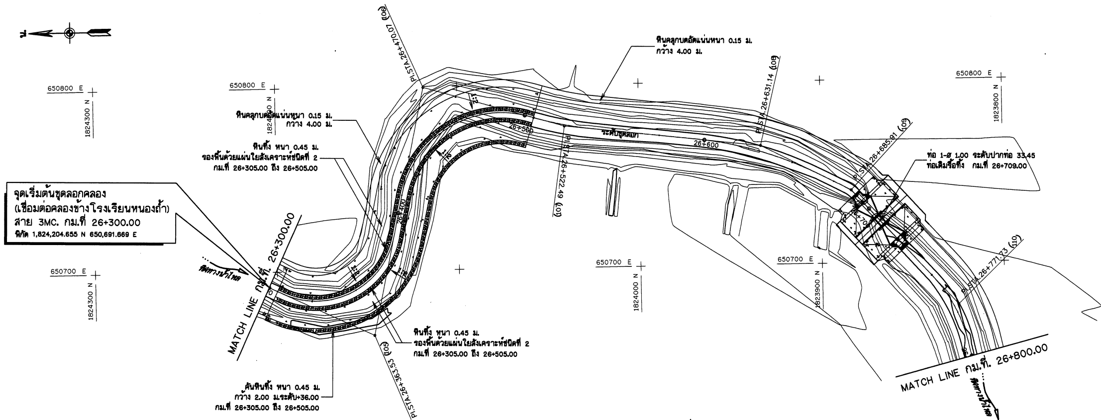
แปลนขุดลอกคลอง สาย 3MC กม.ที่ 26+300.00 - 26+800.00 มาตราส่วน 1:1,000
