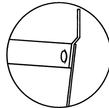
แบบขยาย A: ข้อนทับรอยต่อแผ่นบนทับแผ่นล่าง 0.05 – 0.10 ม.
