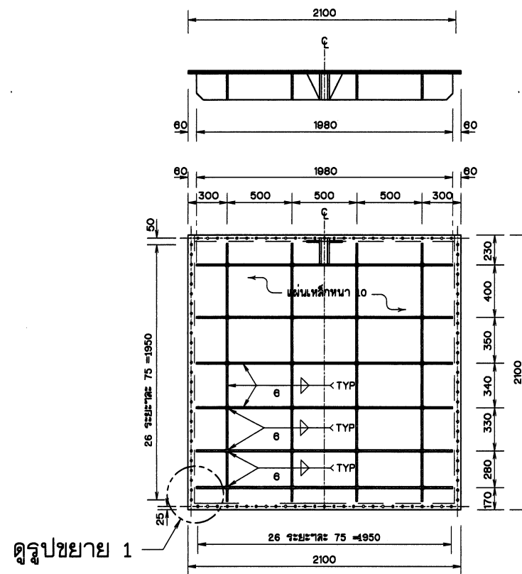
บานเหล็กเหนียว มาตราส่วน 1:20
