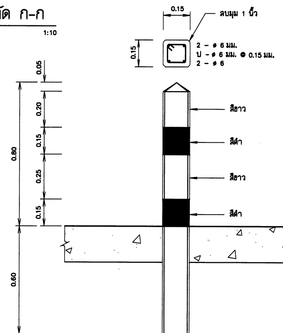
รูปขยายหลักกันตก คสล. มาตราส่วน 1:10
