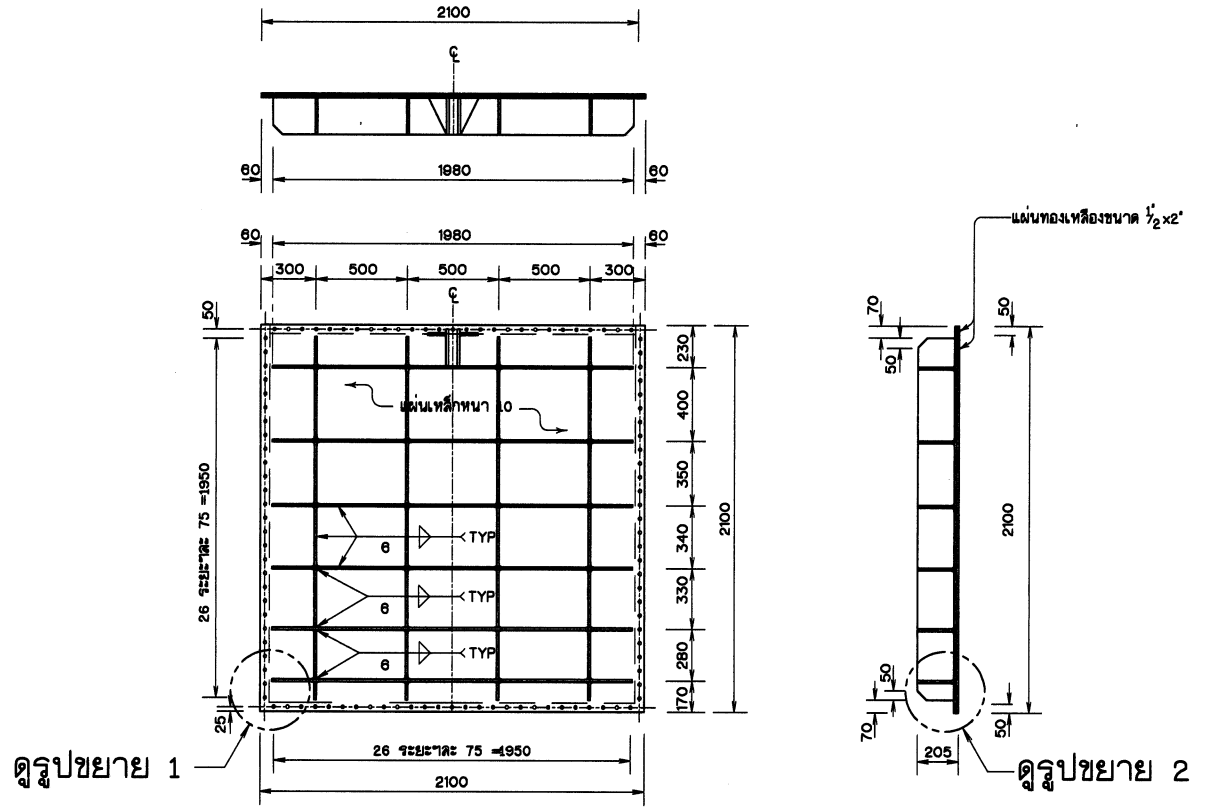
บานเหล็กเหล็ย มาตราส่วน 1:20
