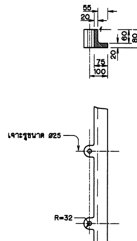
รูปขยายเหล็กนำร่อง มาตรฐาน 1:10
