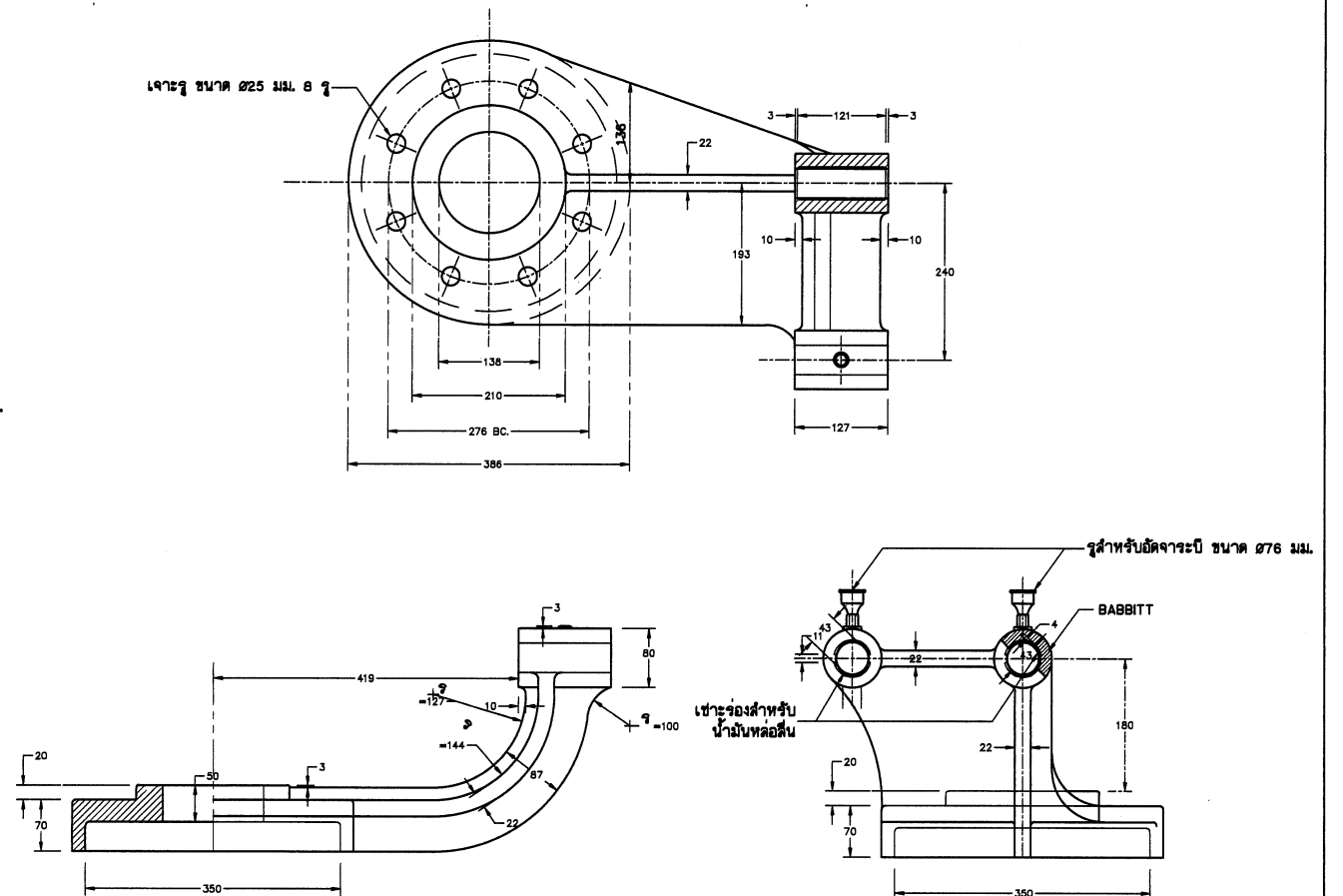
ฝาคกรอบและตุ้กดตา (เหล็กหล่อ)
