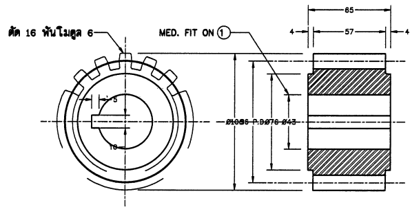
เพื่องเล็ก (เหล็กเหนียว)
