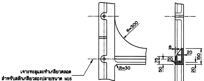
กรอบบานเหล็กหล่อ มาตราส่วน 1:20
