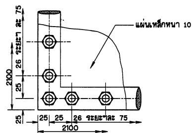
รูปขยาย 1 มาตราส่วน 1:4
