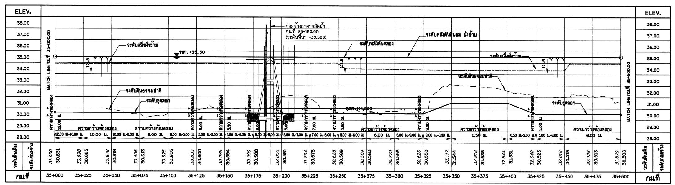
รูปตัดตามยาวชุดลอกคลอง สาย 4MC. กม.ที่ 35+000.00 - 35+500.00 1:100
