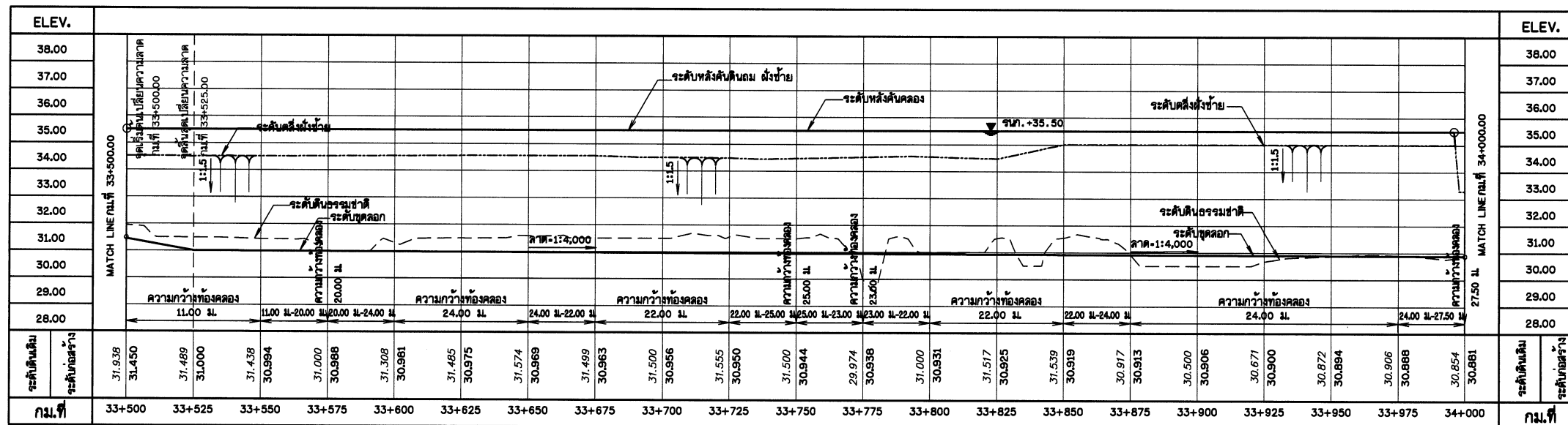
รูปตัดตามยาวชุดลอกคลอง สาย 4MC. กม.ที่ 33+500.00 - 34+000.00
