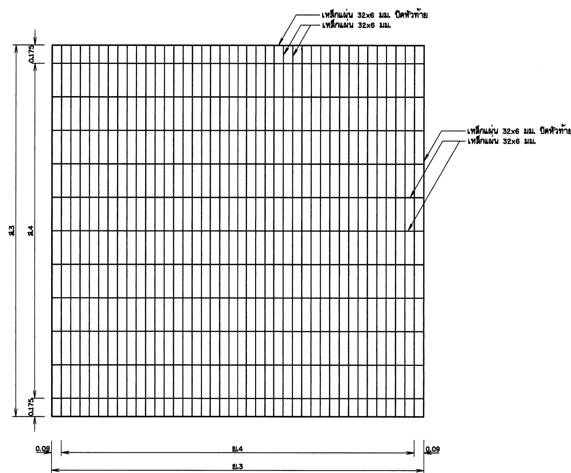
แบบขยายตะแกรงกันสวะ มาตราส่วน 1:20
