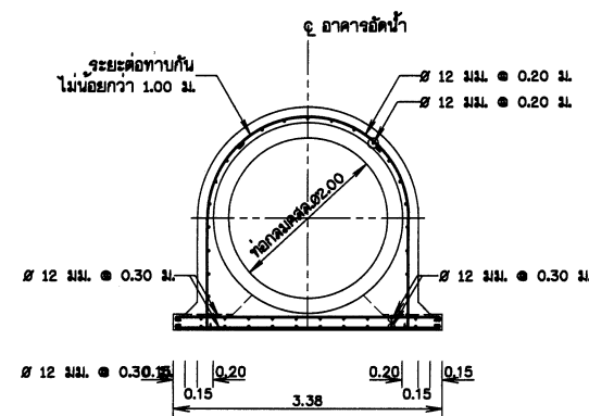
รูปแสดงการเสริมเหล็กคอนกรีตหุ้มท่อ มาตราส่วน 1:50
