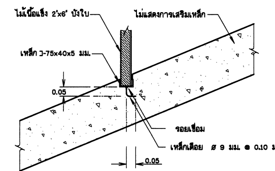
รูปขยายร่องใส่บาน มาตราส่วน 1:10
