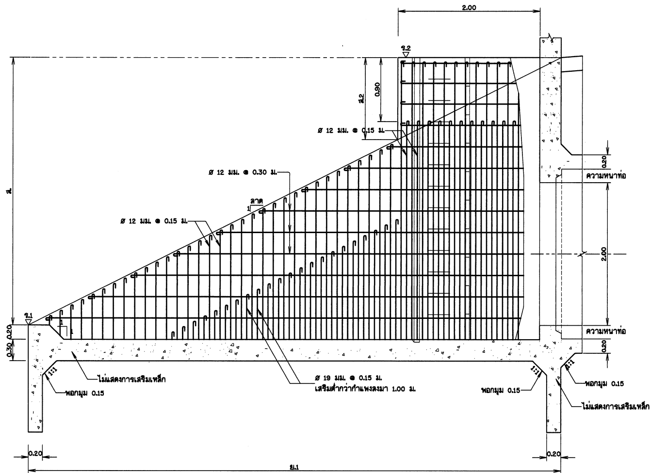
การเสริมเหล็กกำแพงอาคารอัดน้ำ มาตราส่วน 1:25
