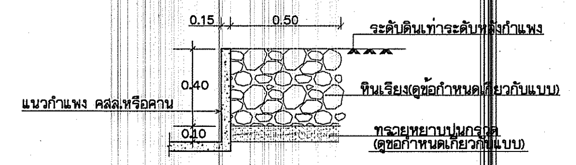
ขยายพื้นเรียง 1 ไม่แสดงมาตราส่วน
