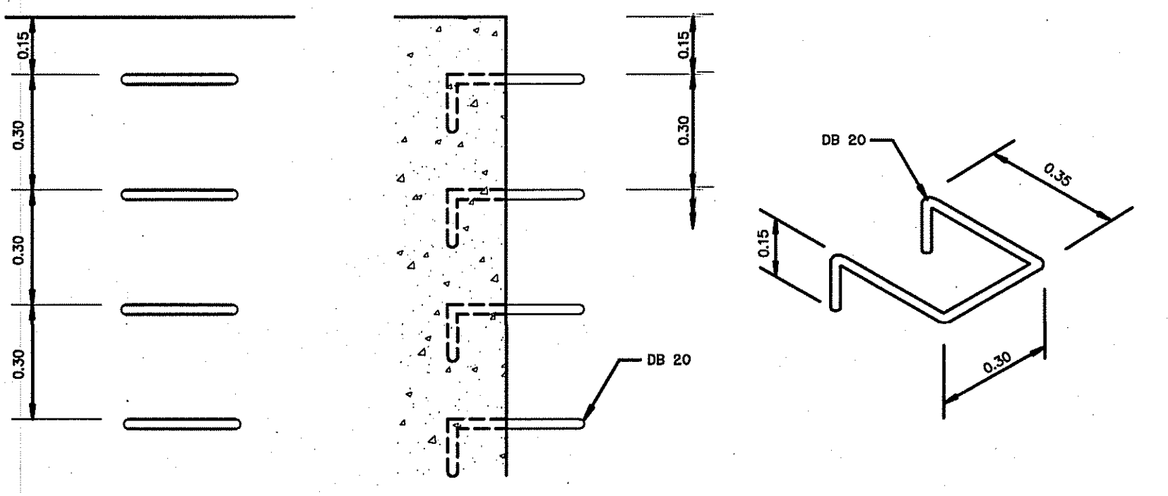
รูปขยายบันไดลงหลัก ไม่แสดงมาตราส่วน
