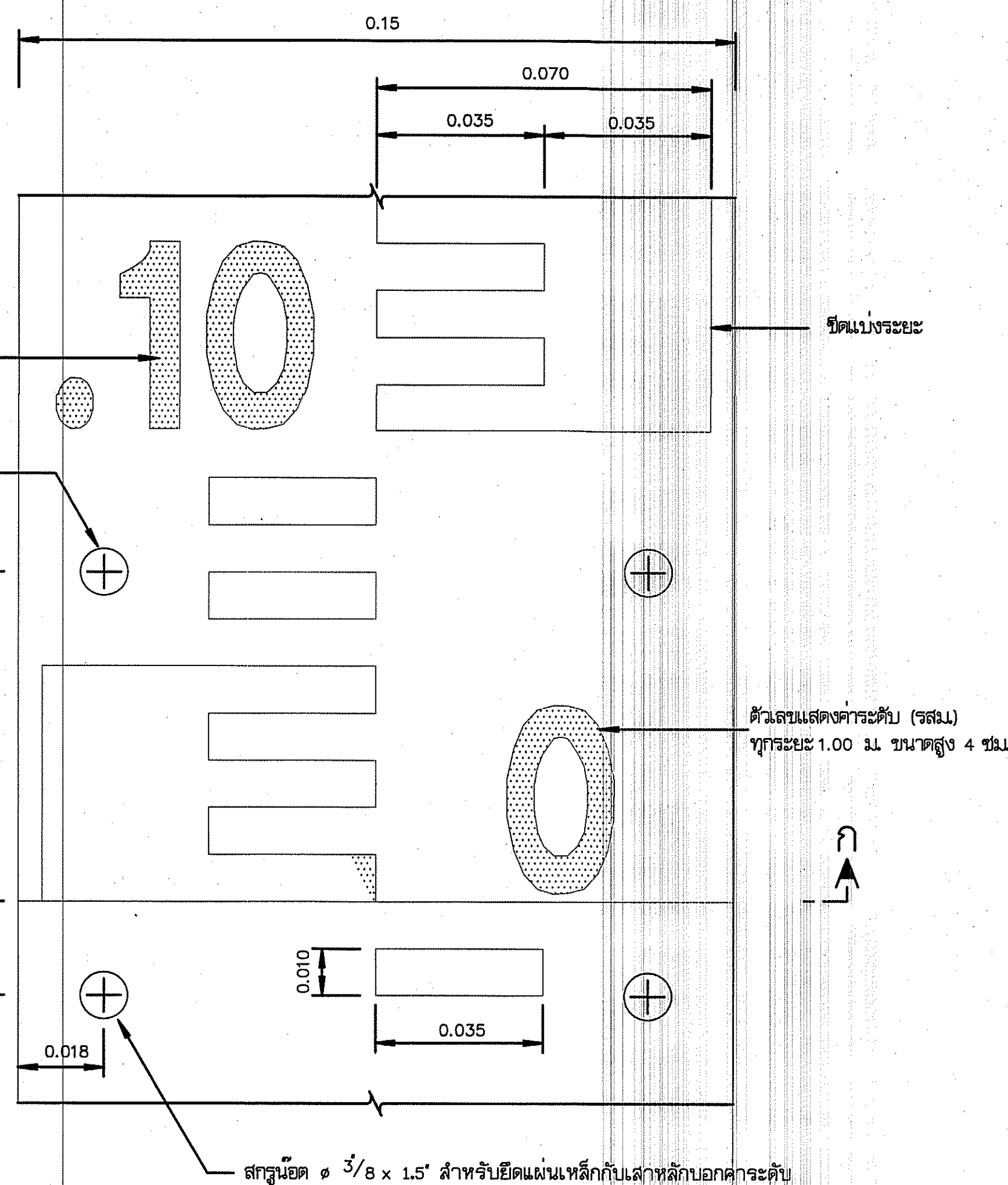
ขยายแผ่นหลักบอกระดับ
