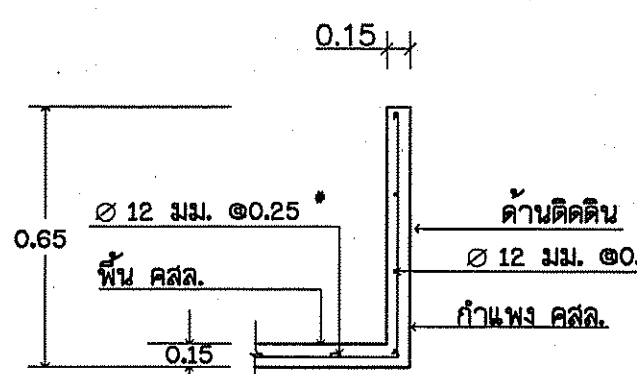
รูปตัด ค-ค (ความหนาพื้น 0.15 ม.) ไม่แสดงมาตราส่วน
