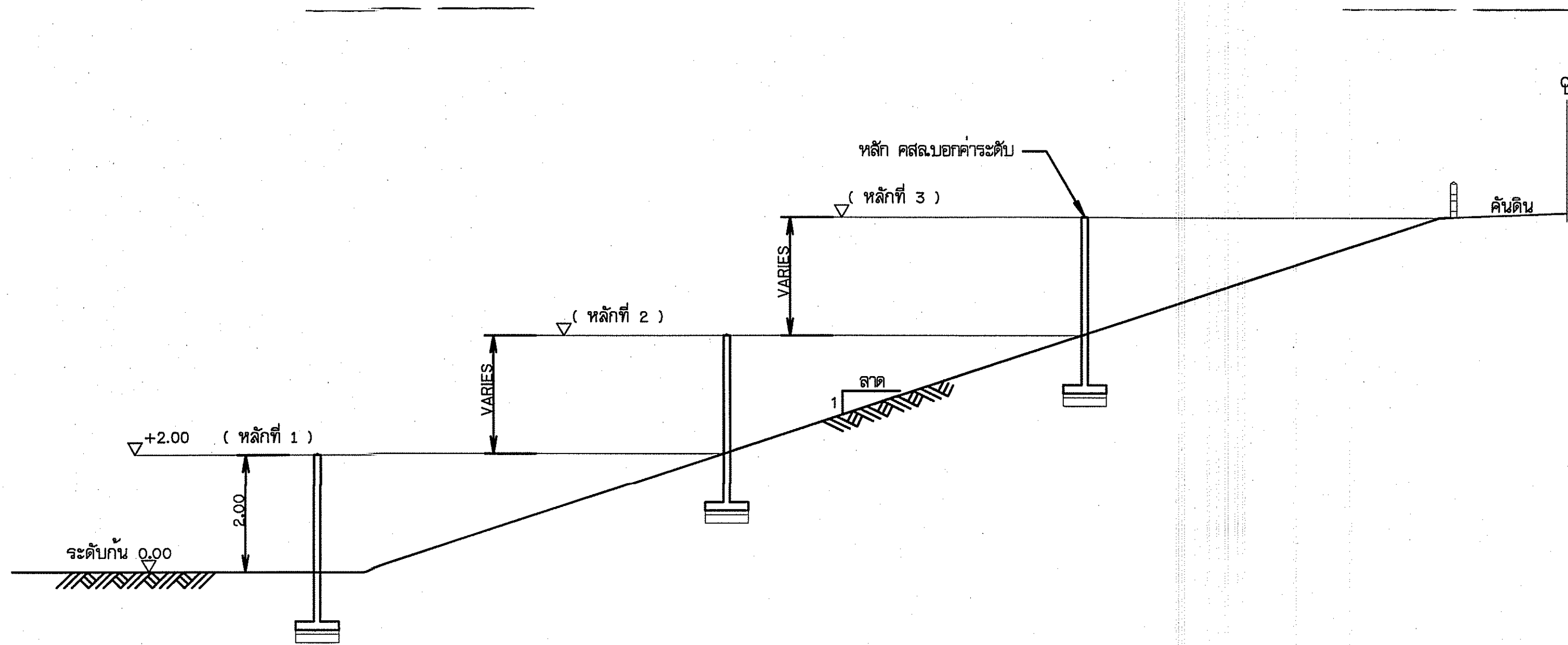
รูปตัดทั่วไปแสดงตำแหน่งหลักบอกระดับน้ำ
