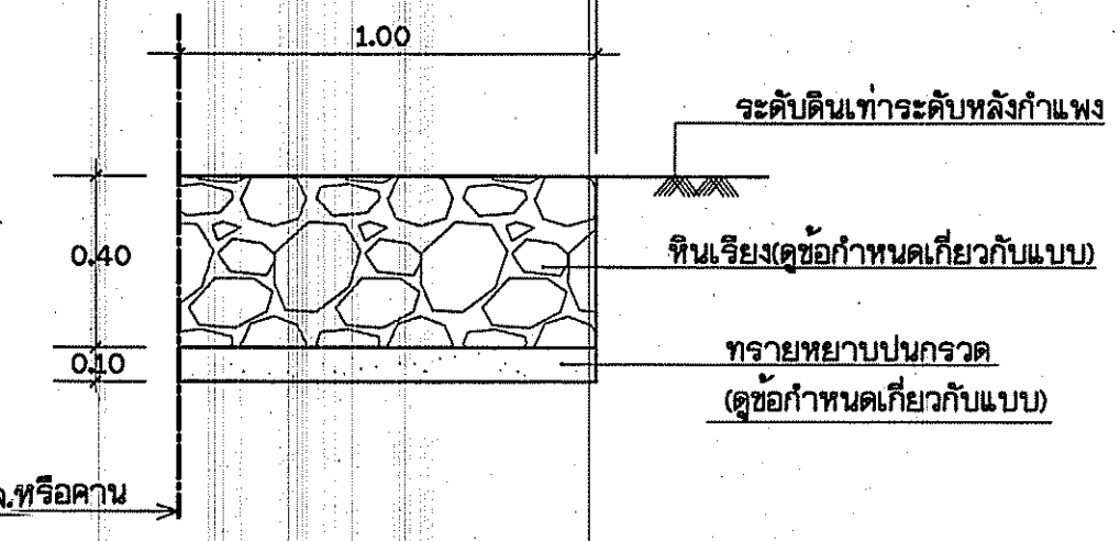
ขยายพื้นเรียง 2 ไม่แสดงมาตราส่วน
