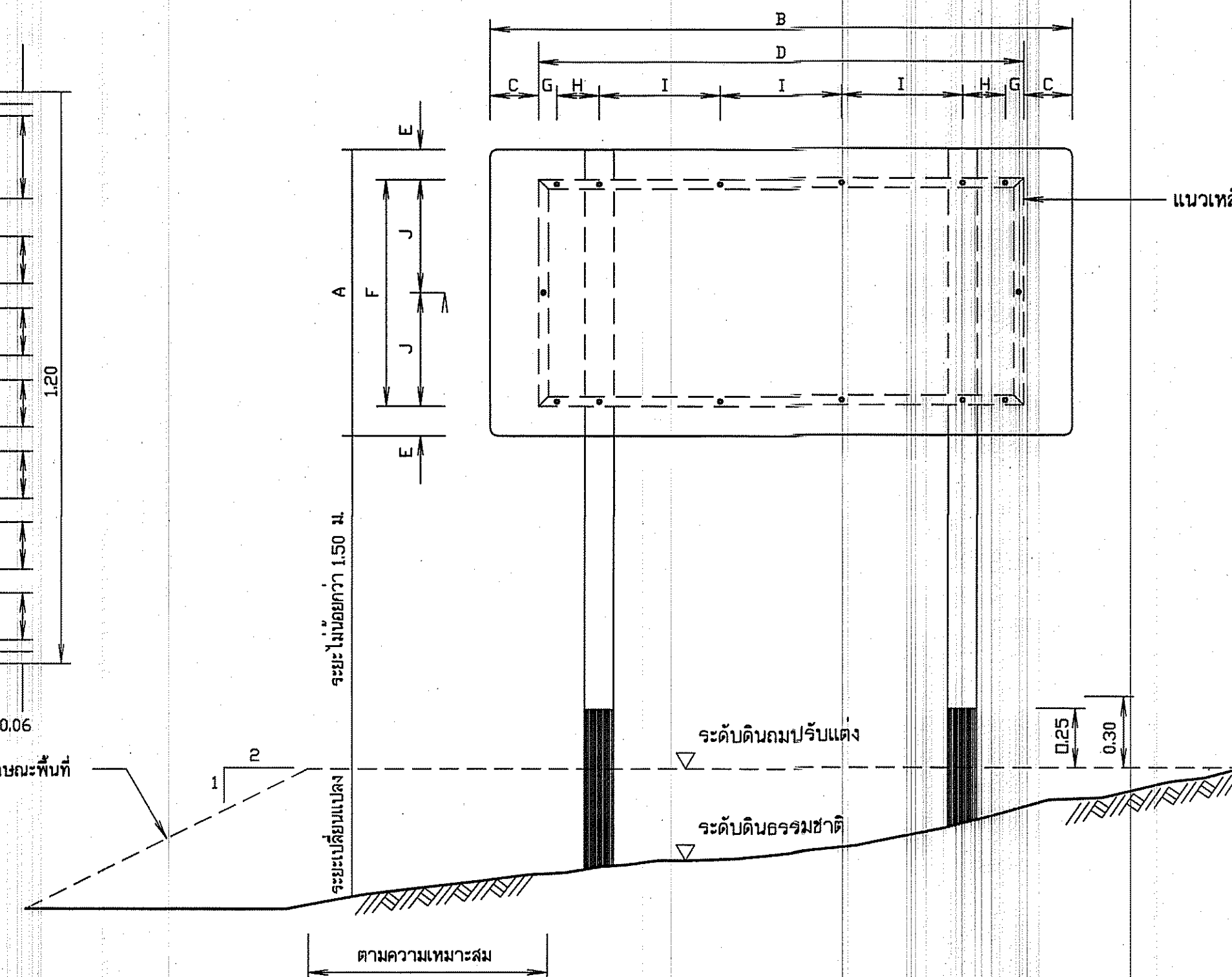
รูปแสดงการประกอบแผ่นบ้าย มาตราส่วน 1:20
