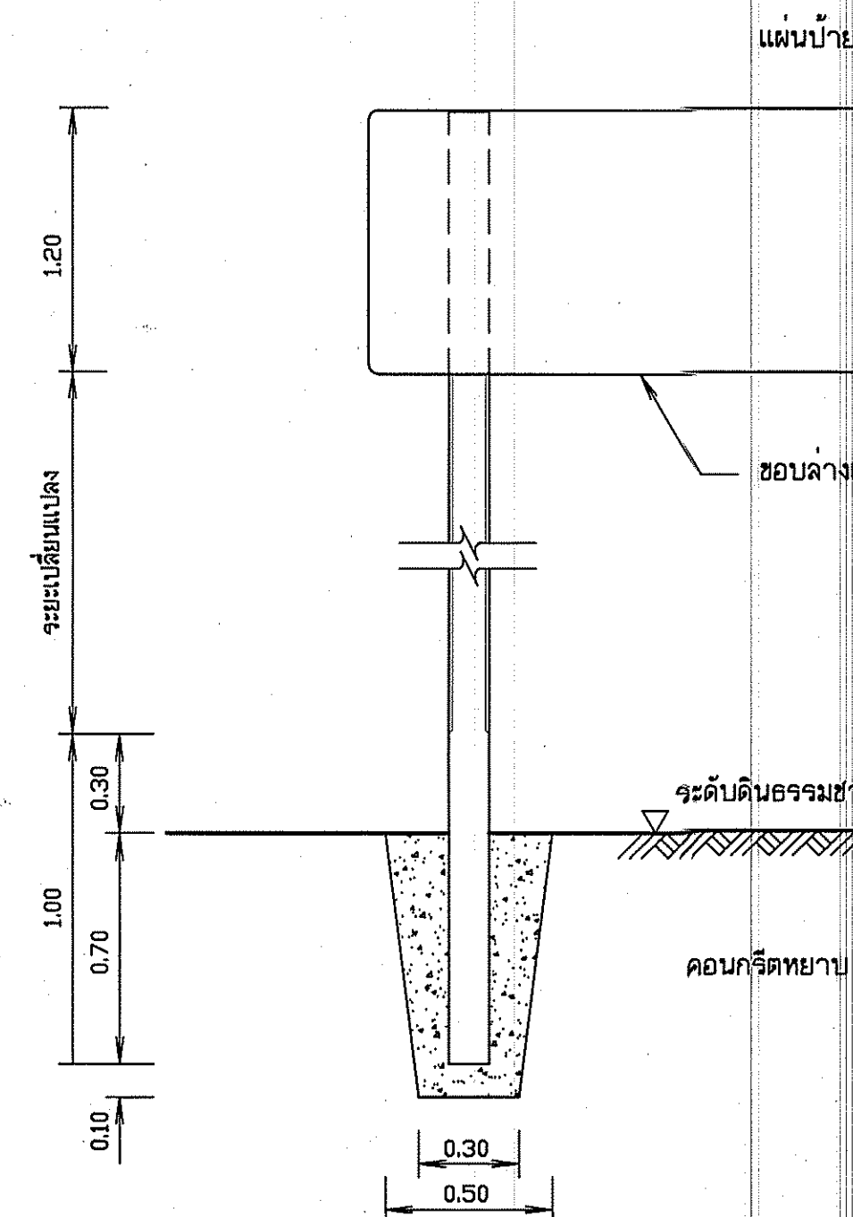
รายละเอียดการติดตั้งเสาบ้าย มาตราส่วน 1:20
