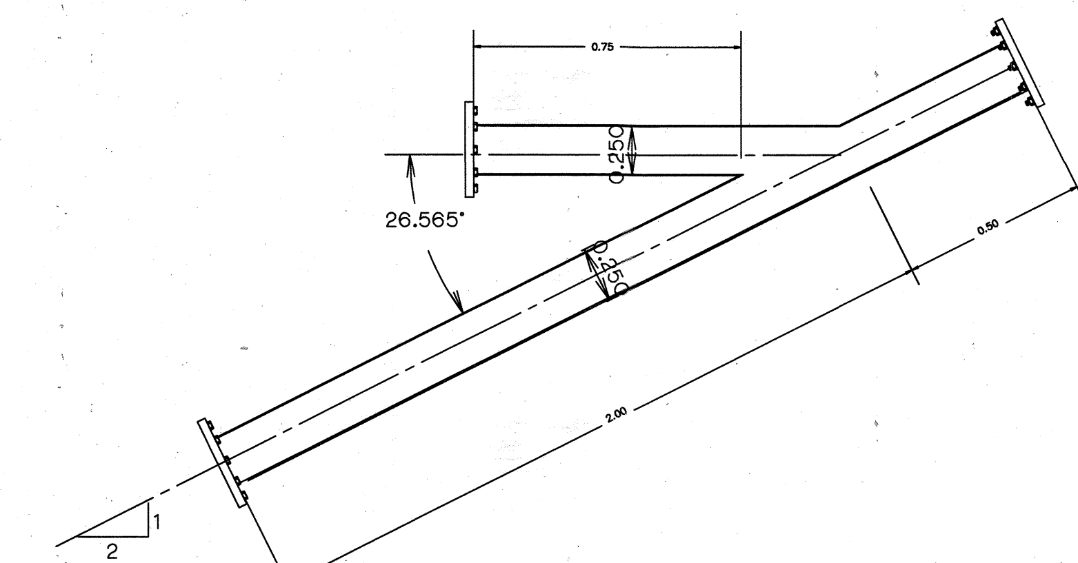
รายละเอียดทอริมดลิง ลาด 1:2 มาตราส่วน 1 : 100
