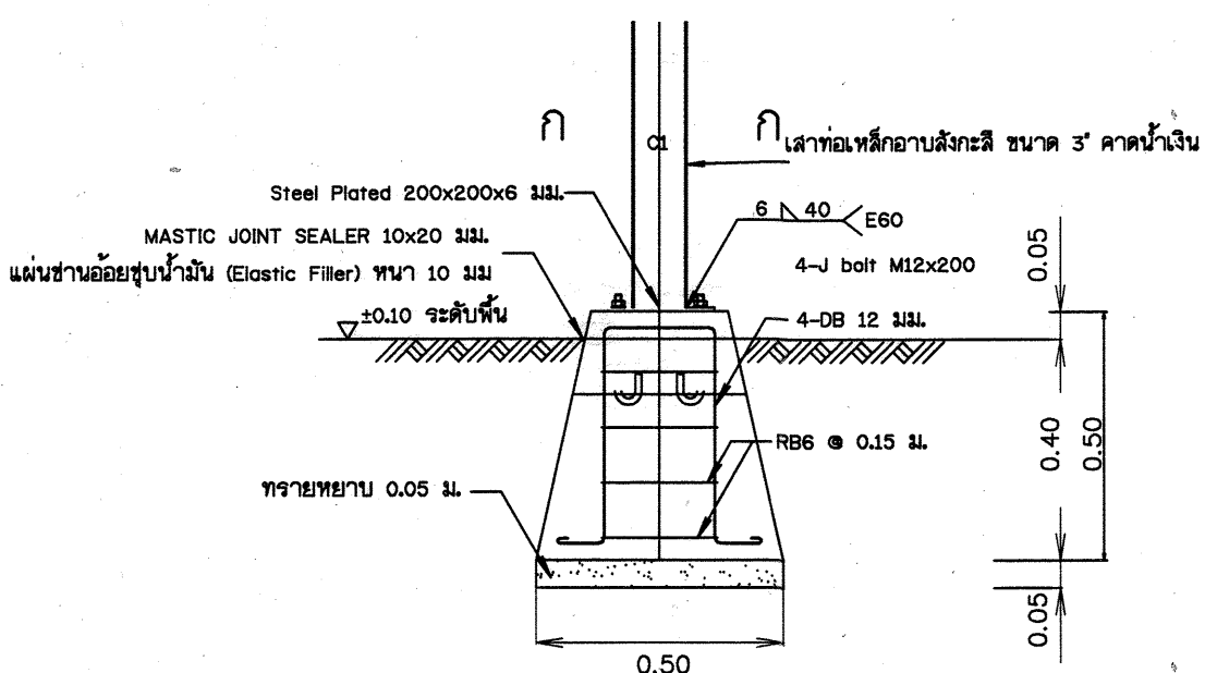
รูปขยายต่อม่อชุดกล้องวงจรปิด (ต่อม่อ ครอบ, หลอดไฟ, ครอบหลอดไฟ)
