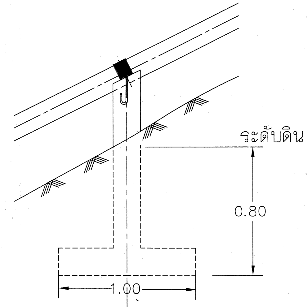
รูปขยายเลารับท่อส่งน้ำ
