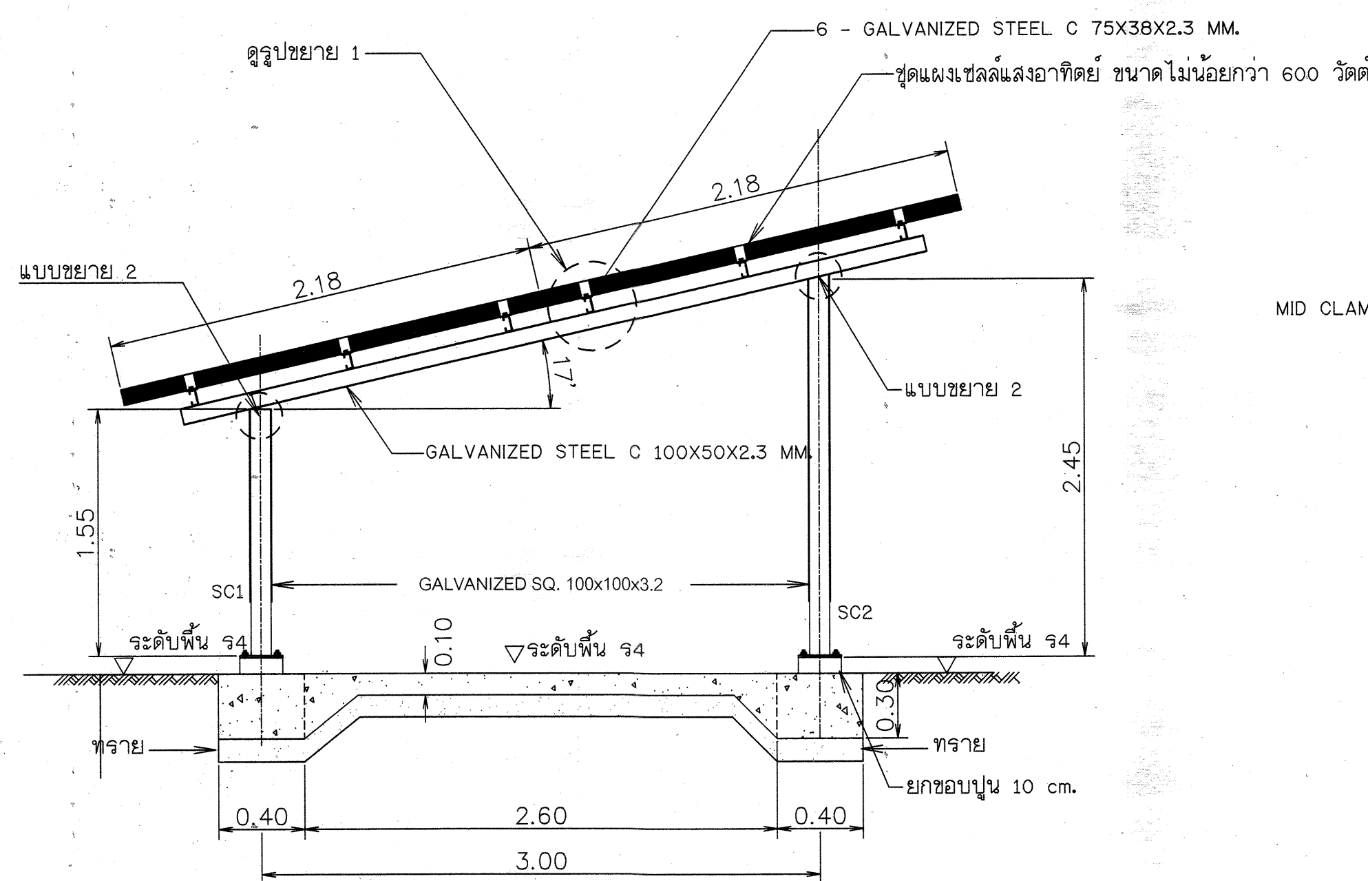
รูปตัด ป - ป มาตราส่วน 1:25
