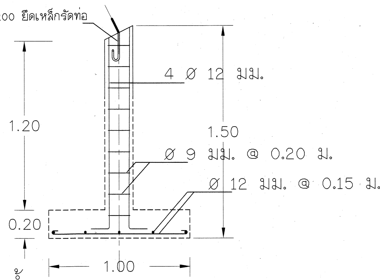
ทอส่งน้ำ GS. Ø 6" เหล็กแบนรัดทอตัดขึ้นรูป ขนาด 0.10 ม.หนา 10 มม.
