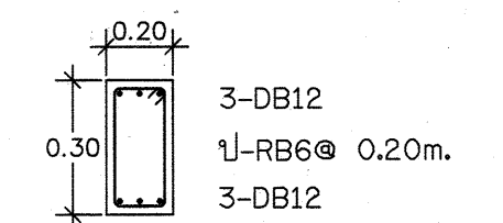
แบบขยายโครงสร้างคานรั้ว (BE) SCALE 1:100
