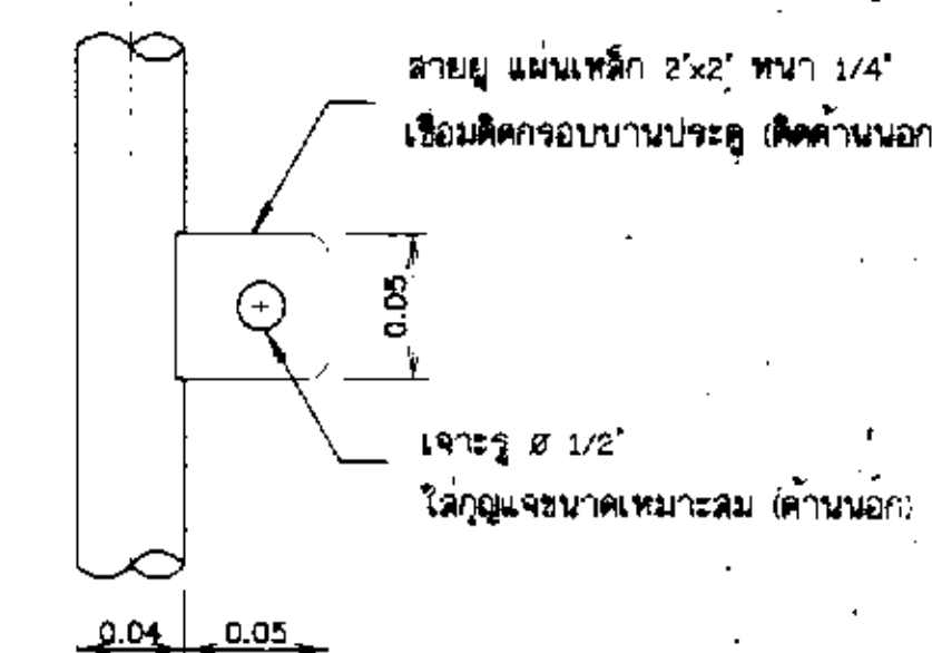
แบบขยายลายปู ไม่แสดงมาตราส่วน
