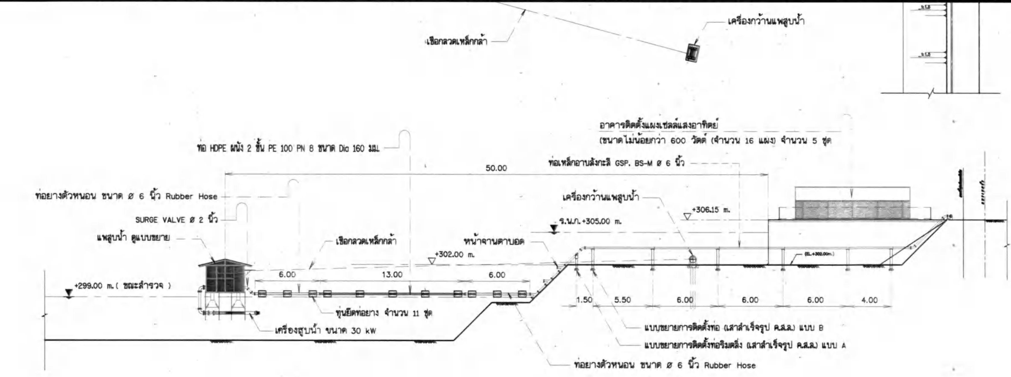
รูปตัด ก-ก อาคารสถานีสูบน้ำ มาตราส่วน 1:200
