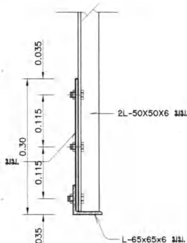
รูปตัด ข - ข
