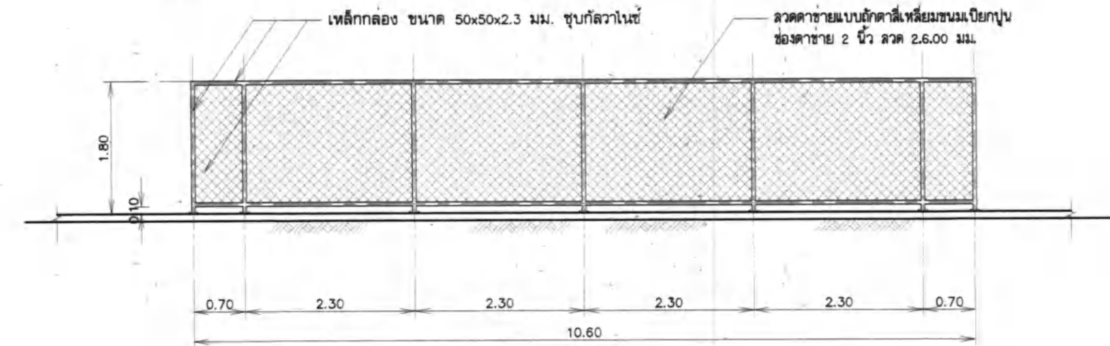
รูปด้าน 3
