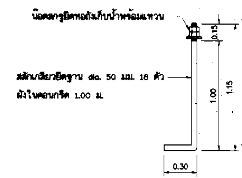
แบบขยายสลักเกลียวยึดฐาน ไม่แสดงขนาดฐาน
