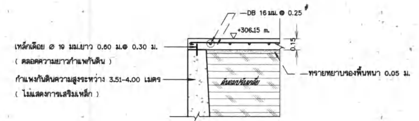
รูปขยาย ② มาตราส่วน 1:25
