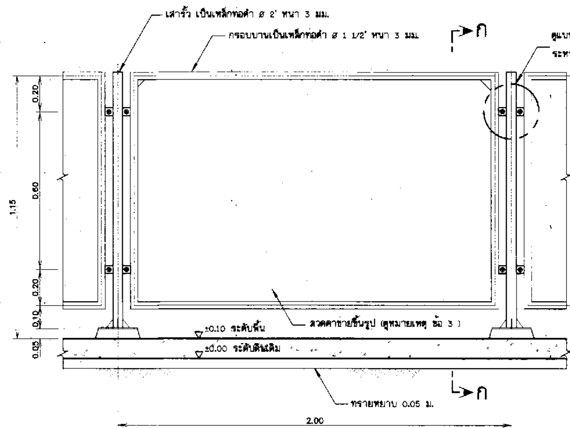
แบบขยายรั้วลวดค้ำยัน ไม่แสดงมาตราส่วน
