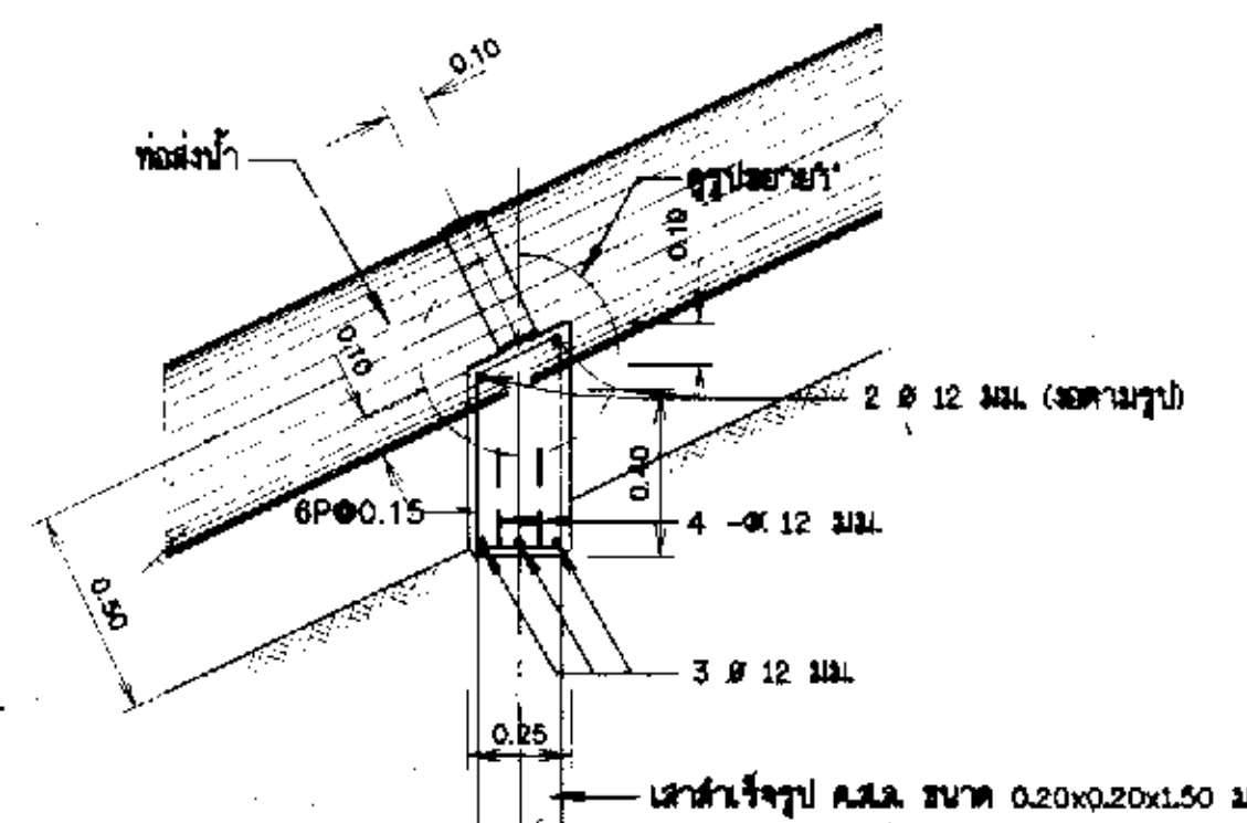
รูปตัด ค-ค
