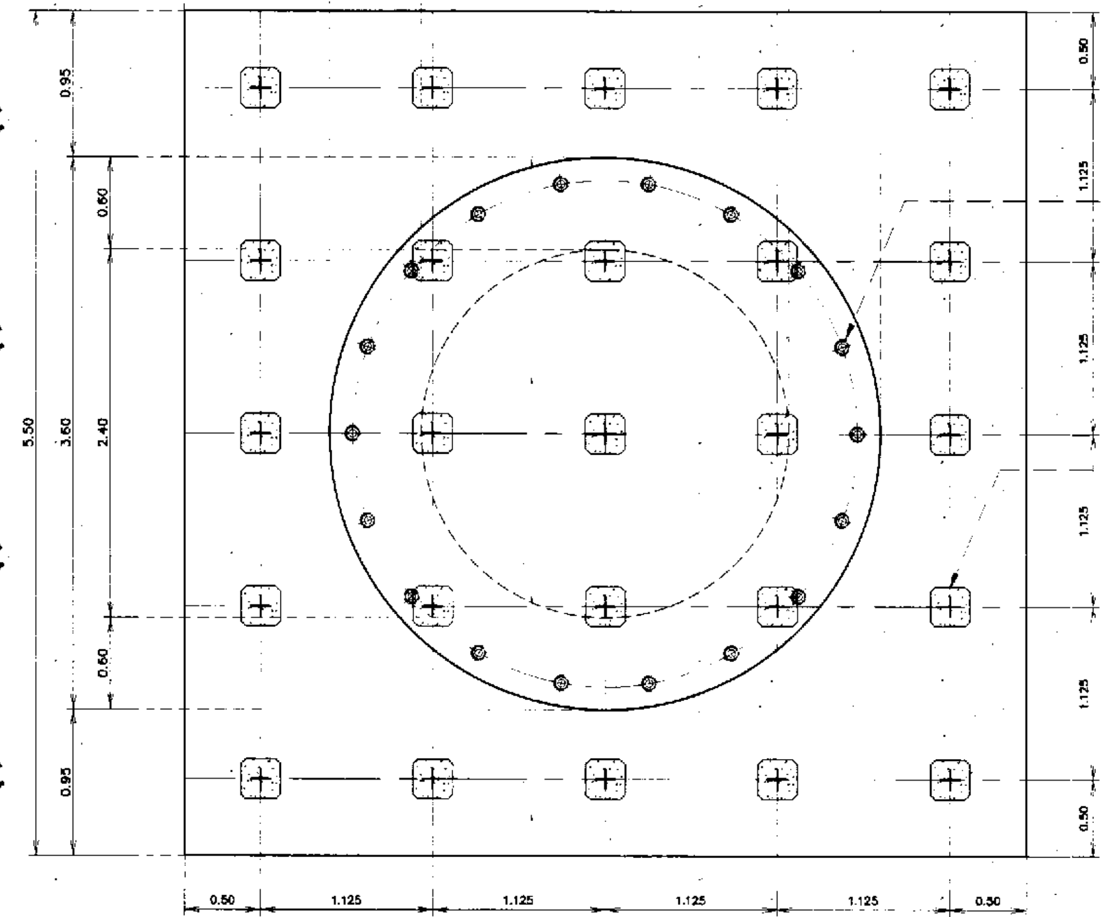
แบบขยายฐานรากทอถังสูง (แบบเสาเข็ม)
