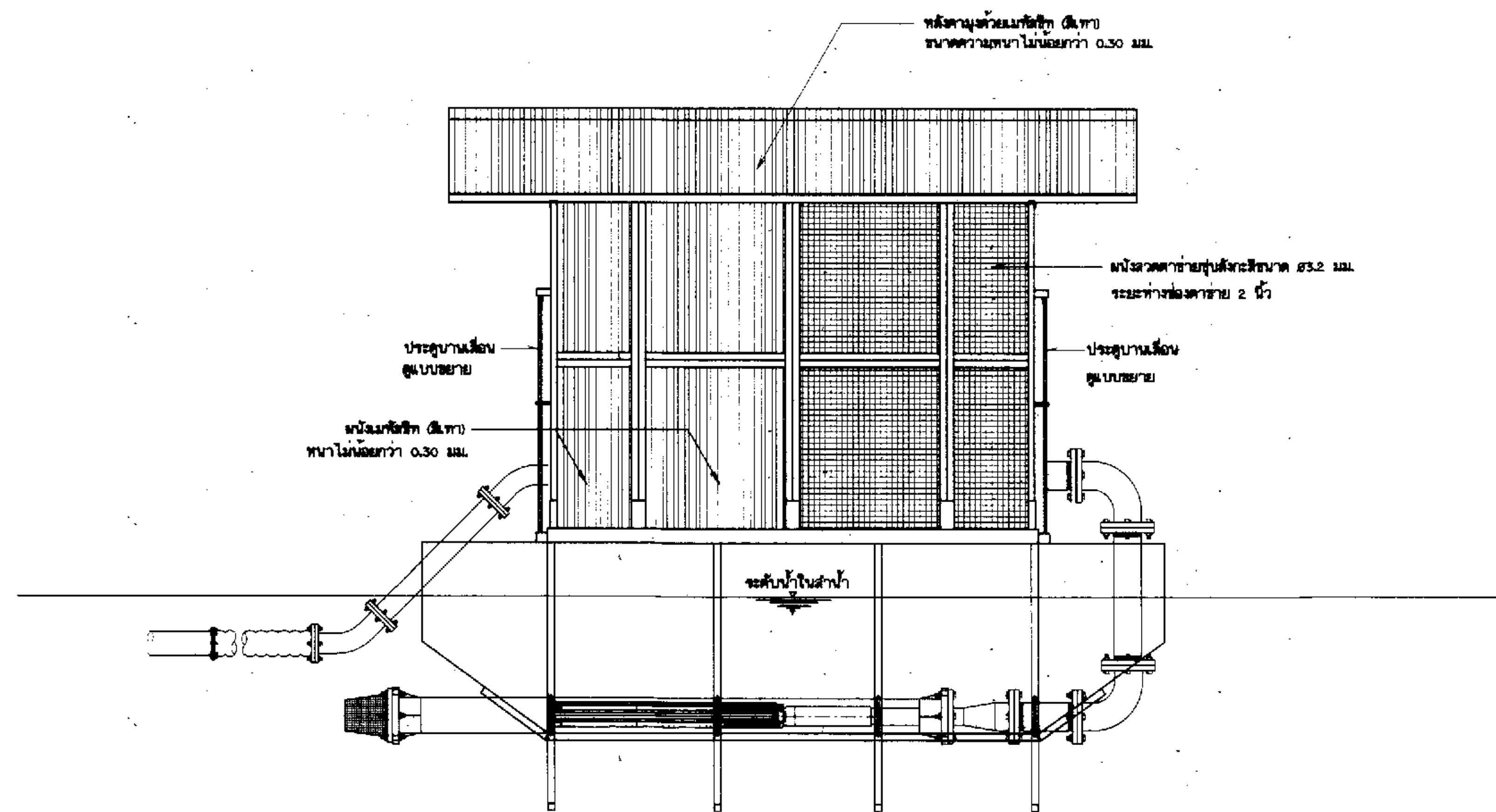
รูปด้าน 3
