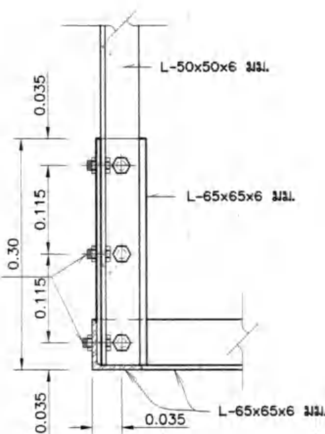
รูปตัด ก - ก
