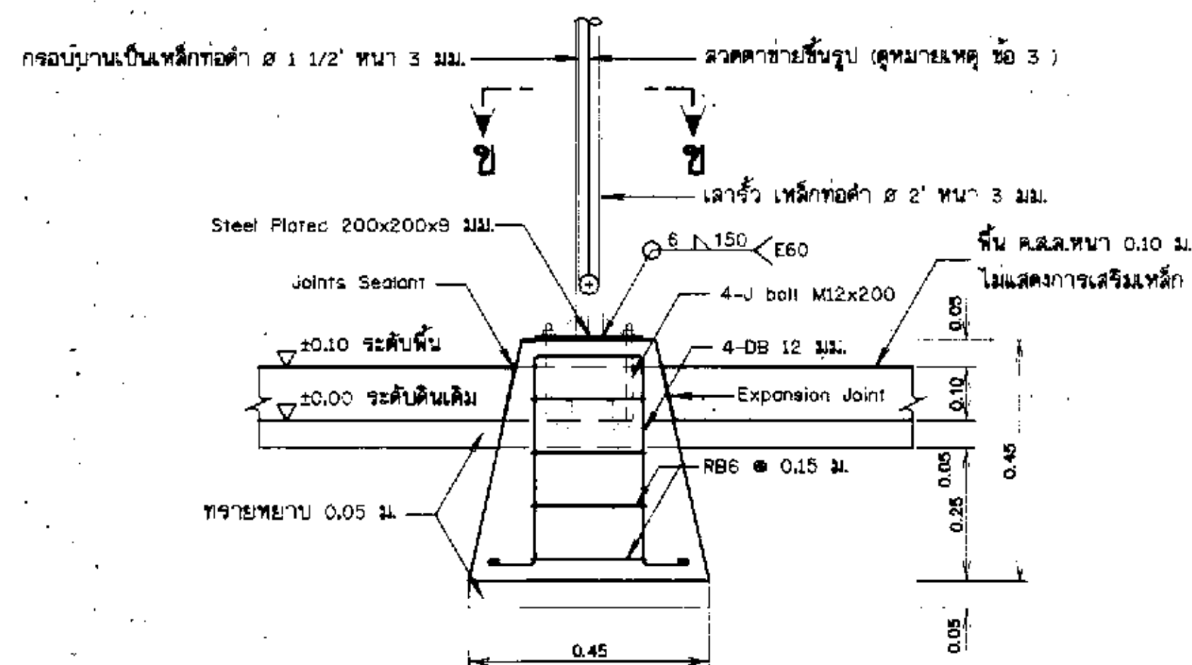
รูปขยายฐานรากโครงสร้างรับแผง F1 (คอม. คสล. หล่อสำเร็จรูปพร้อมติดตั้ง) ไม่แสดงมาตราส่วน
