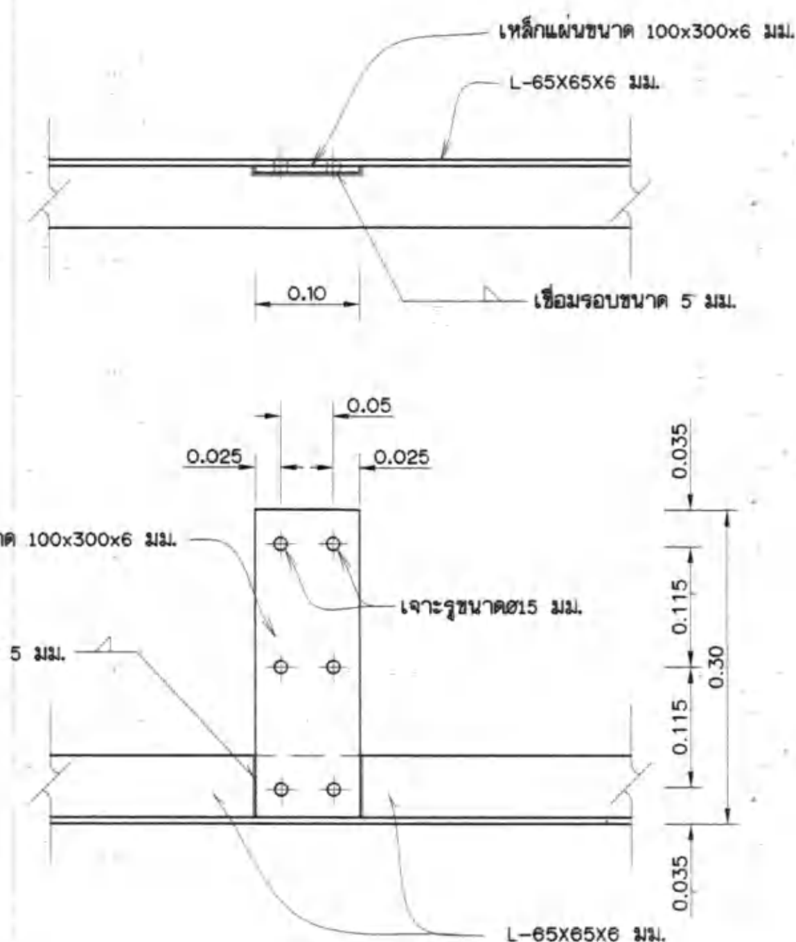
รูปด้านตั้ง (ไม่แสดงเหล็กจาก)
