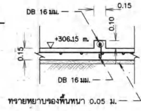
รูปขยาย CURB มาตราส่วน 1:25
