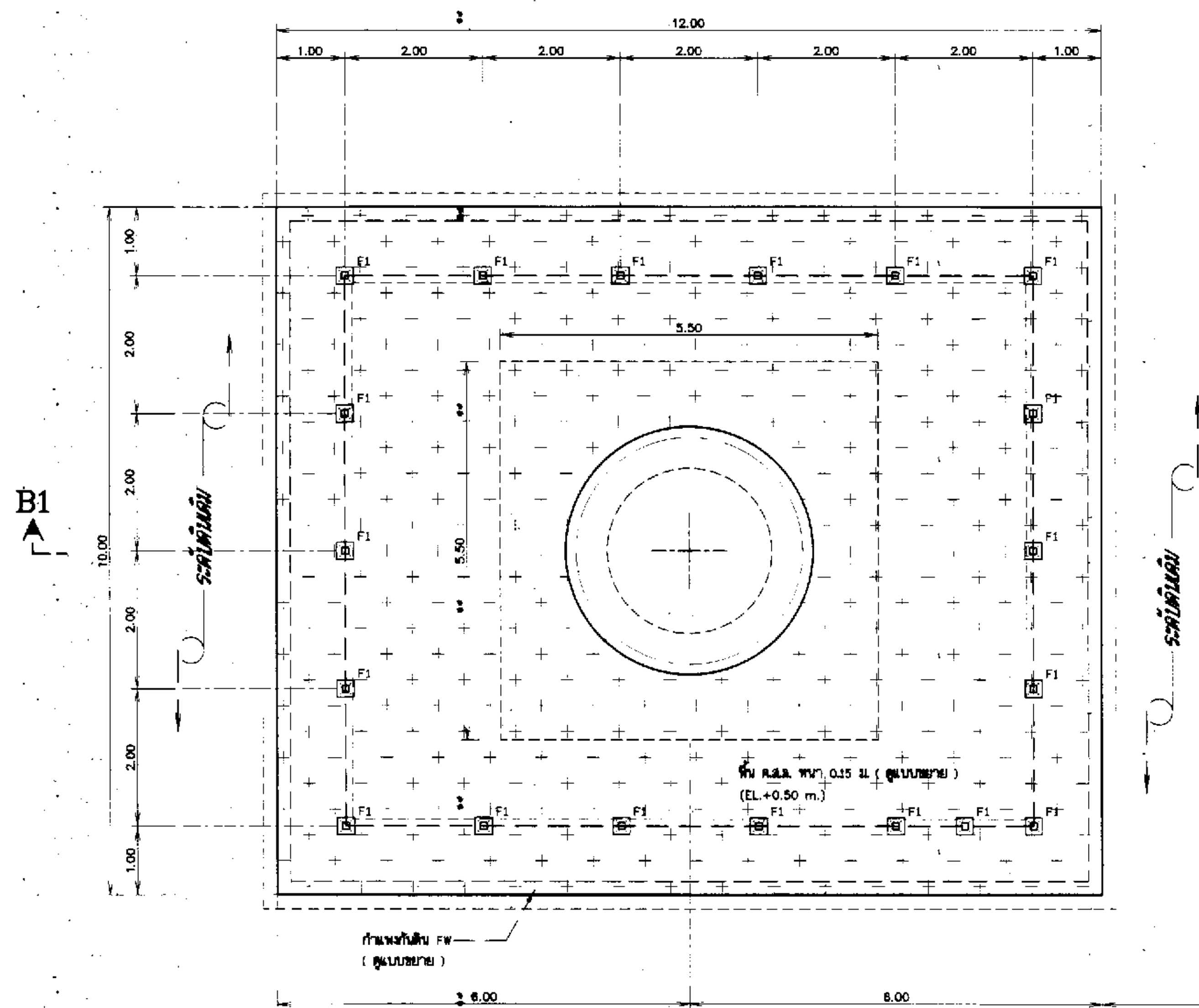
แปลนที่ติดตั้งเก็บน้ำ
