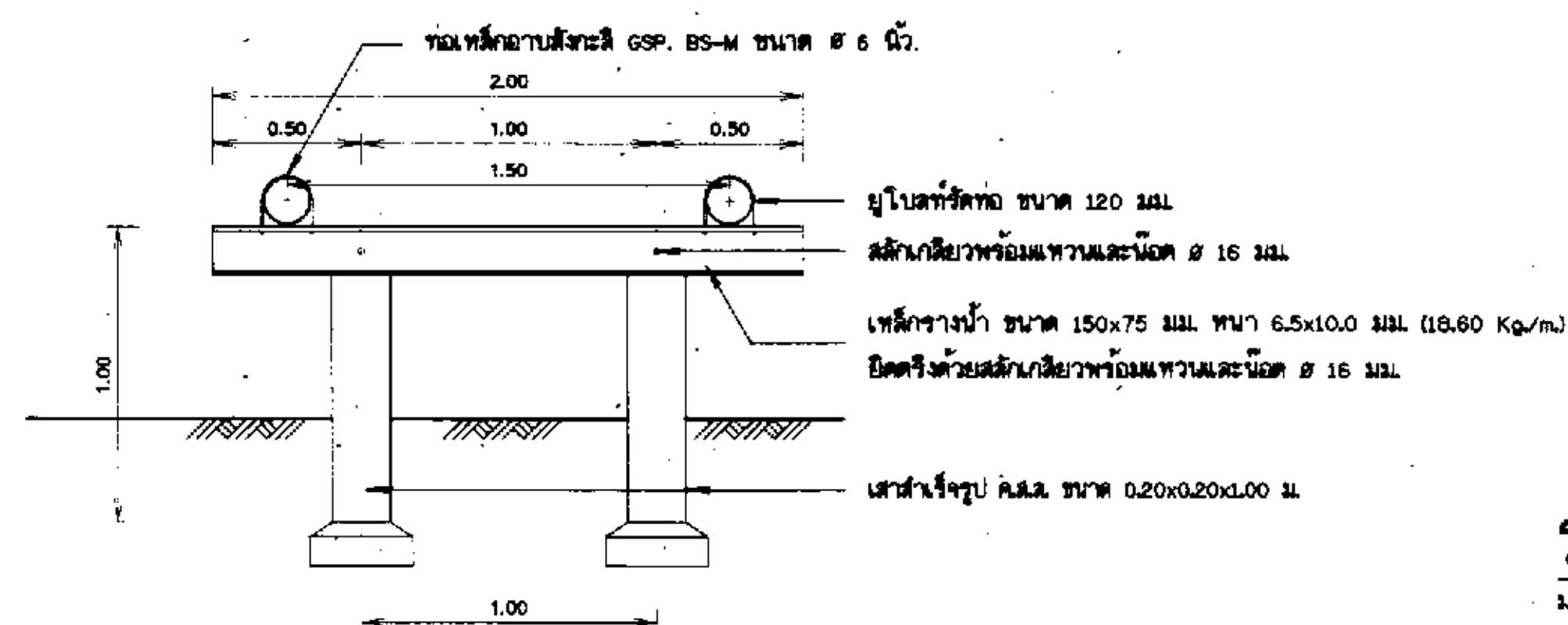
แบบขยายการติดตั้งแบบ C
