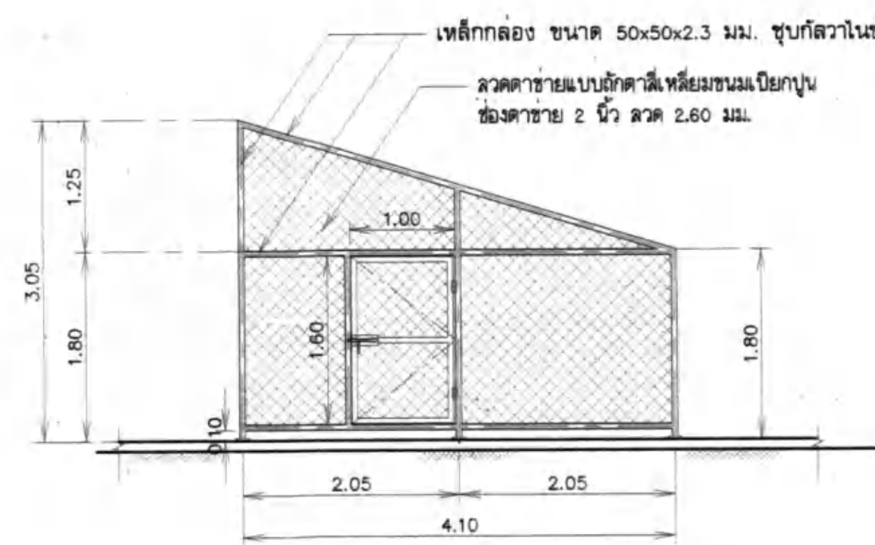
รูปด้าน 2
