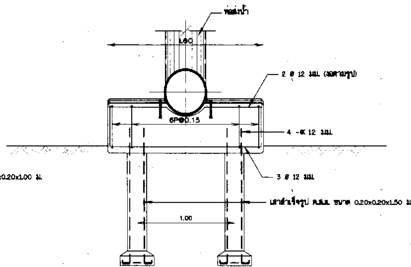
รูปตัด ก-ก
