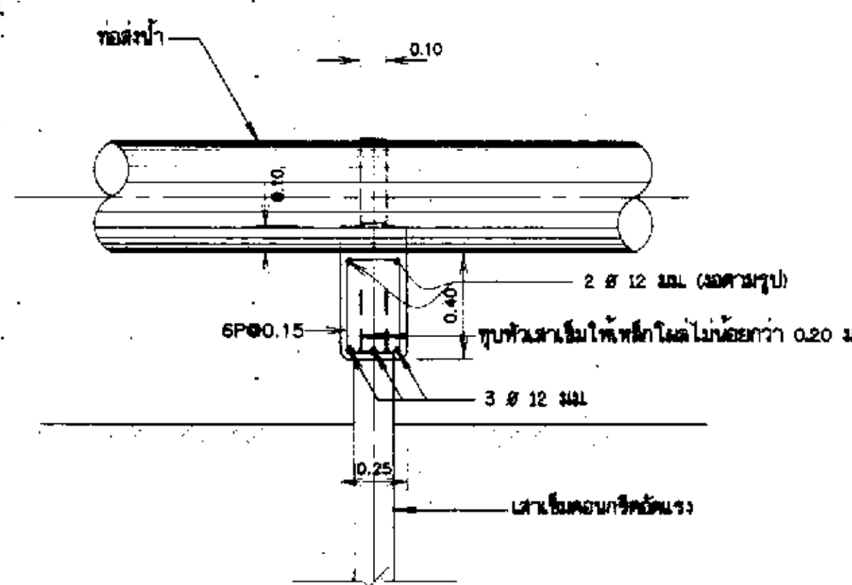
รูปตัด ข-ข
