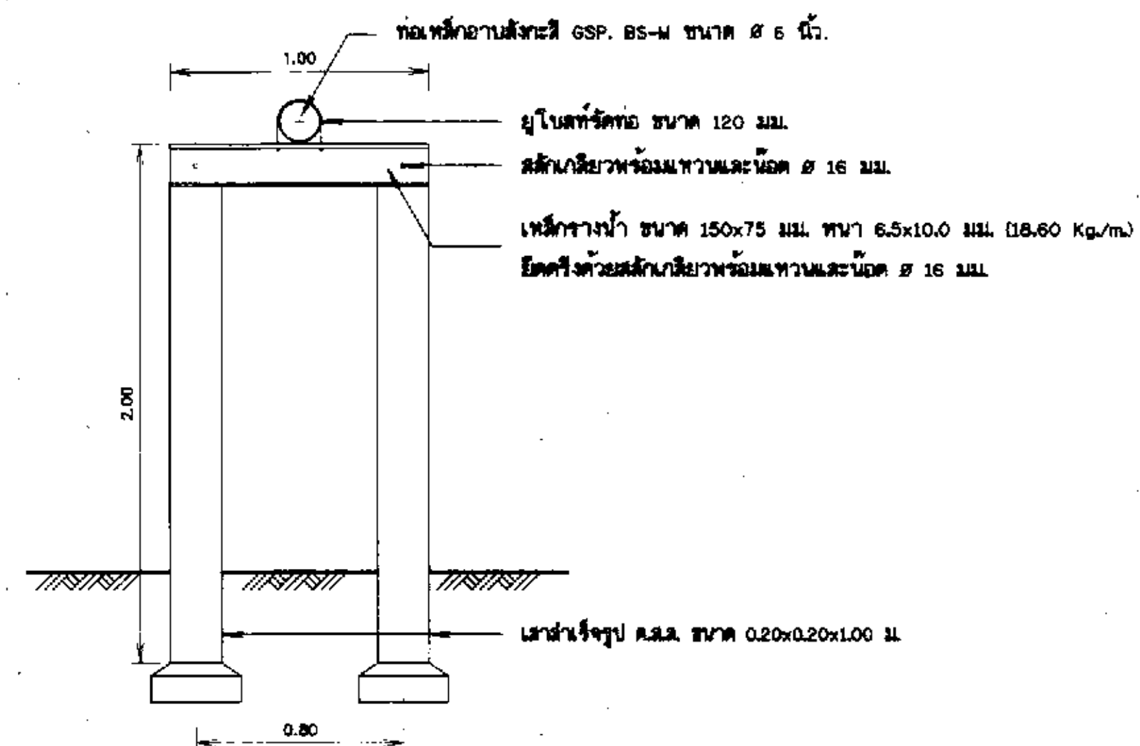
แบบขยายการติดตั้งแบบ B
