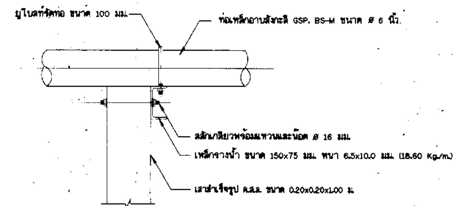
รูค่าน้ำข้างเสาตอม่อรับท่อ และแบบขยายอุปกรณ์รัดท่อ มาตราส่วน 1 : 10
