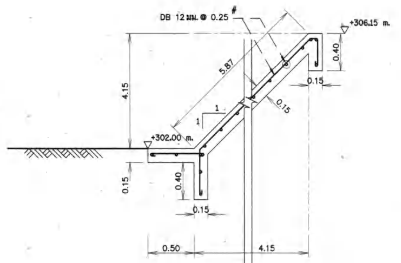
แบบขยาย ตาด ค.ส.ล. ป้องกันการกัดเซาะ ลาด 1 : 1 มาตราส่วน 1:25
