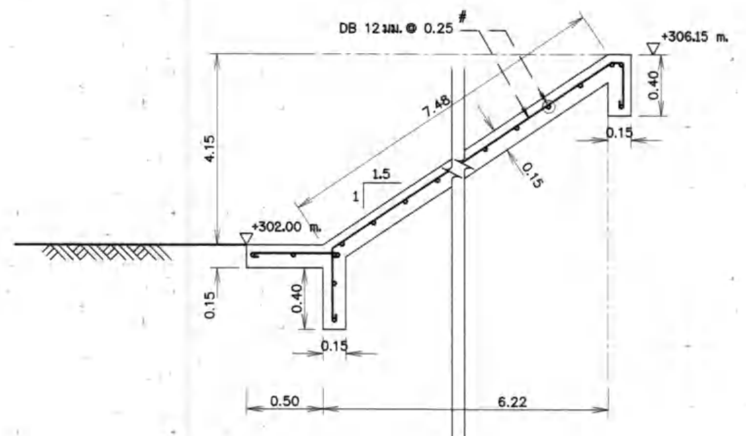
แบบขยาย ตาด ค.ส.ล. ป้องกันการกัดเซาะ ลาด 1 : 1.5 มาตราส่วน 1:25
