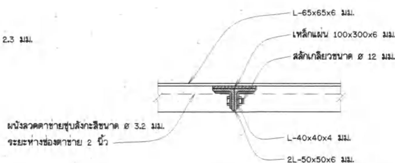
รูปตัด ค-ค
