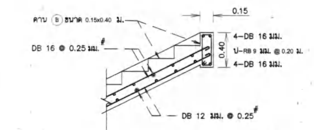
รูปขยาย 1 มาตราส่วน 1:25
