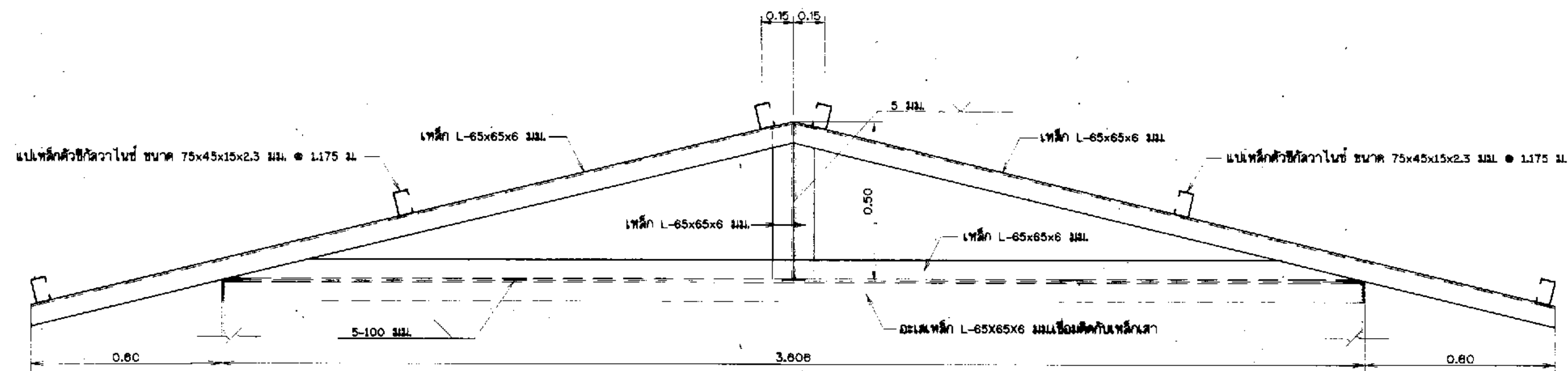
รูปขยายโครงหลังคา
