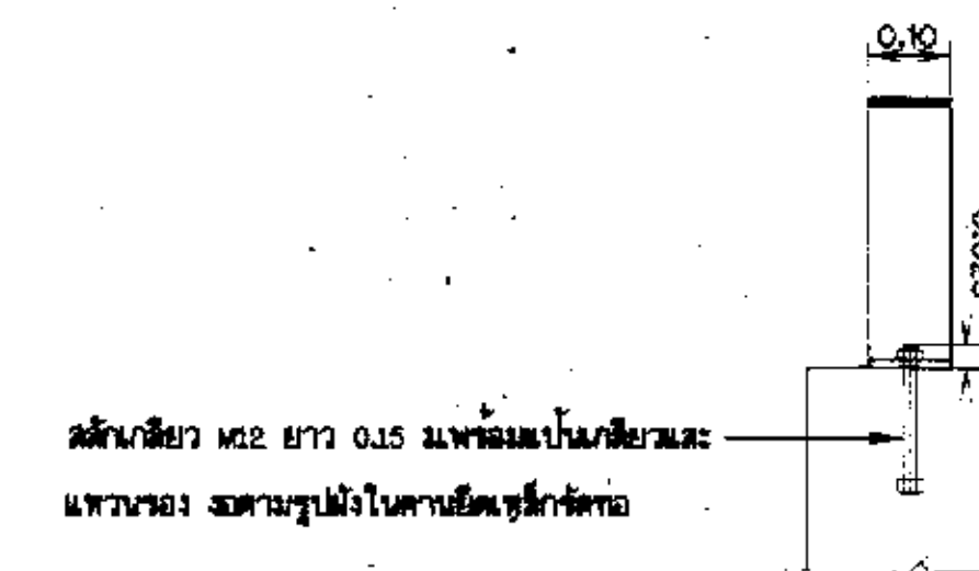
รูปขยาย 1
