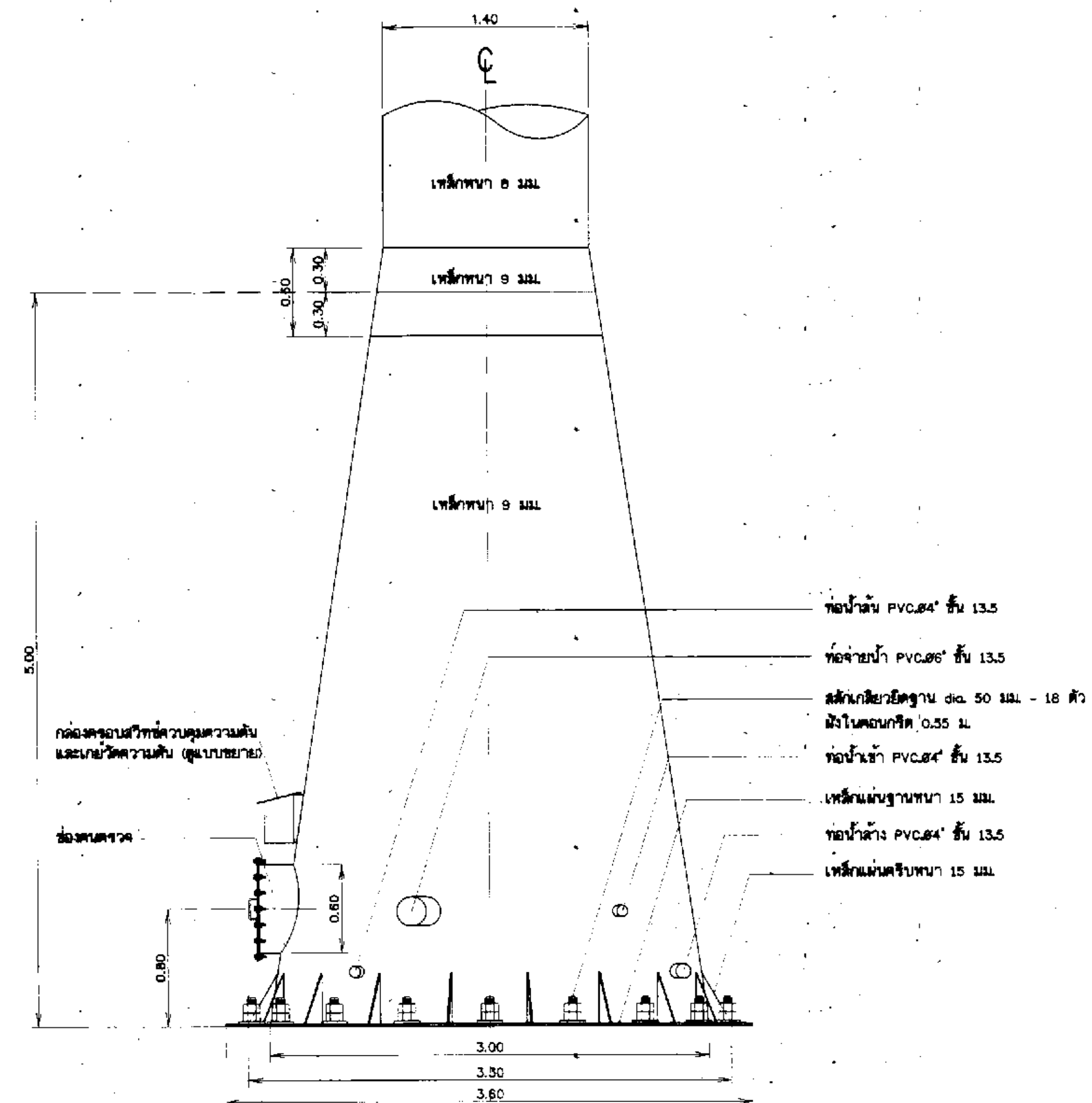
แบบขยายแมนโฮลล่างถึงชมพู
