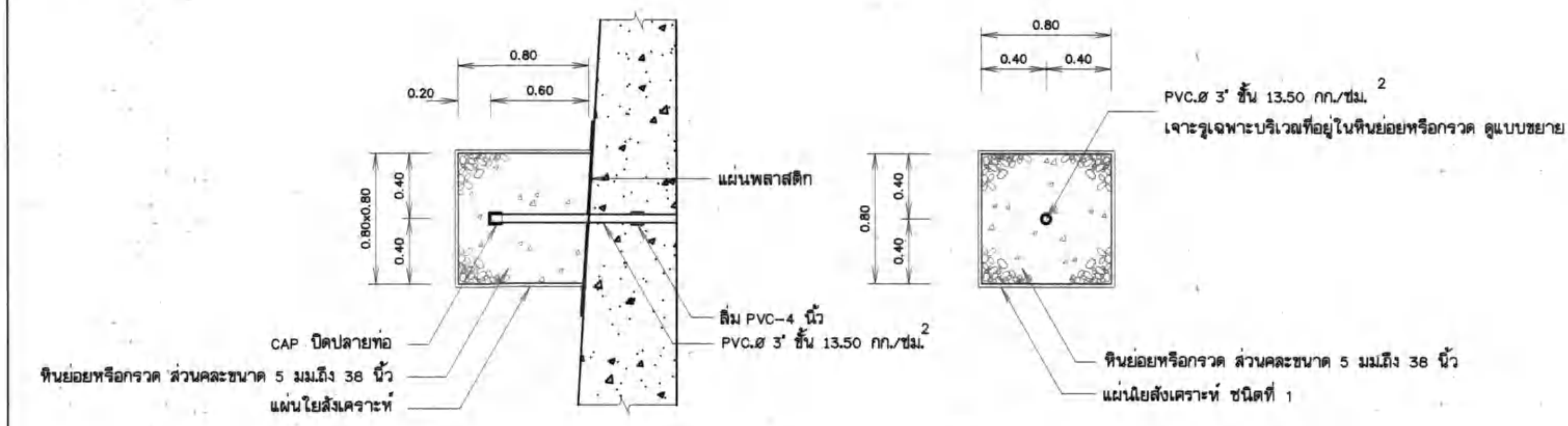
แบบขยาย รุระบายน้ำกำแพง มาตราส่วน 1:25
