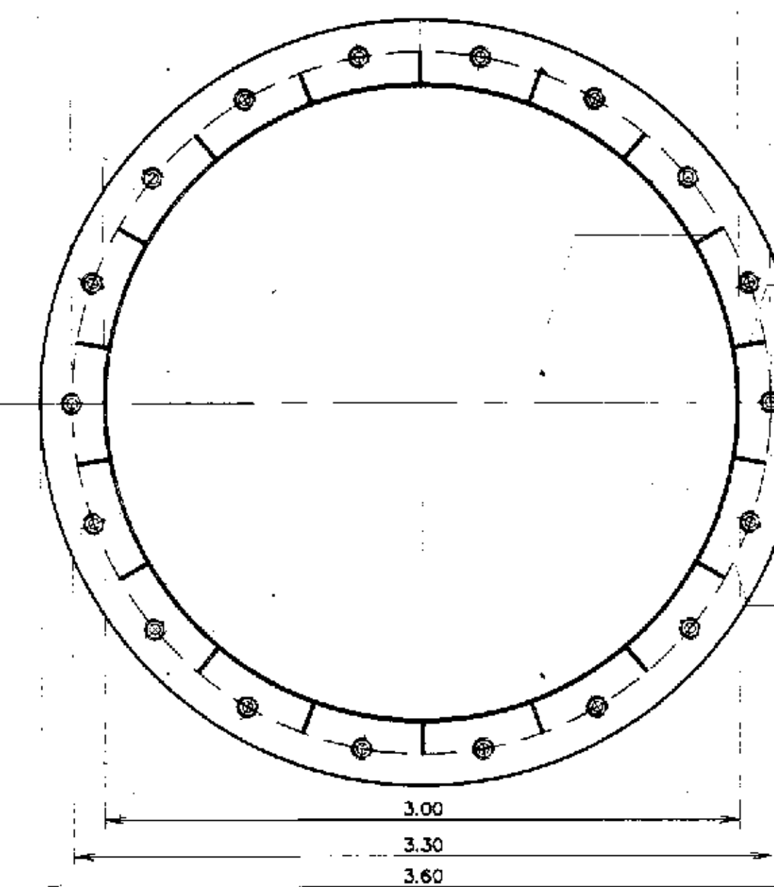
แบบขยายหลักผ่านฐาน
