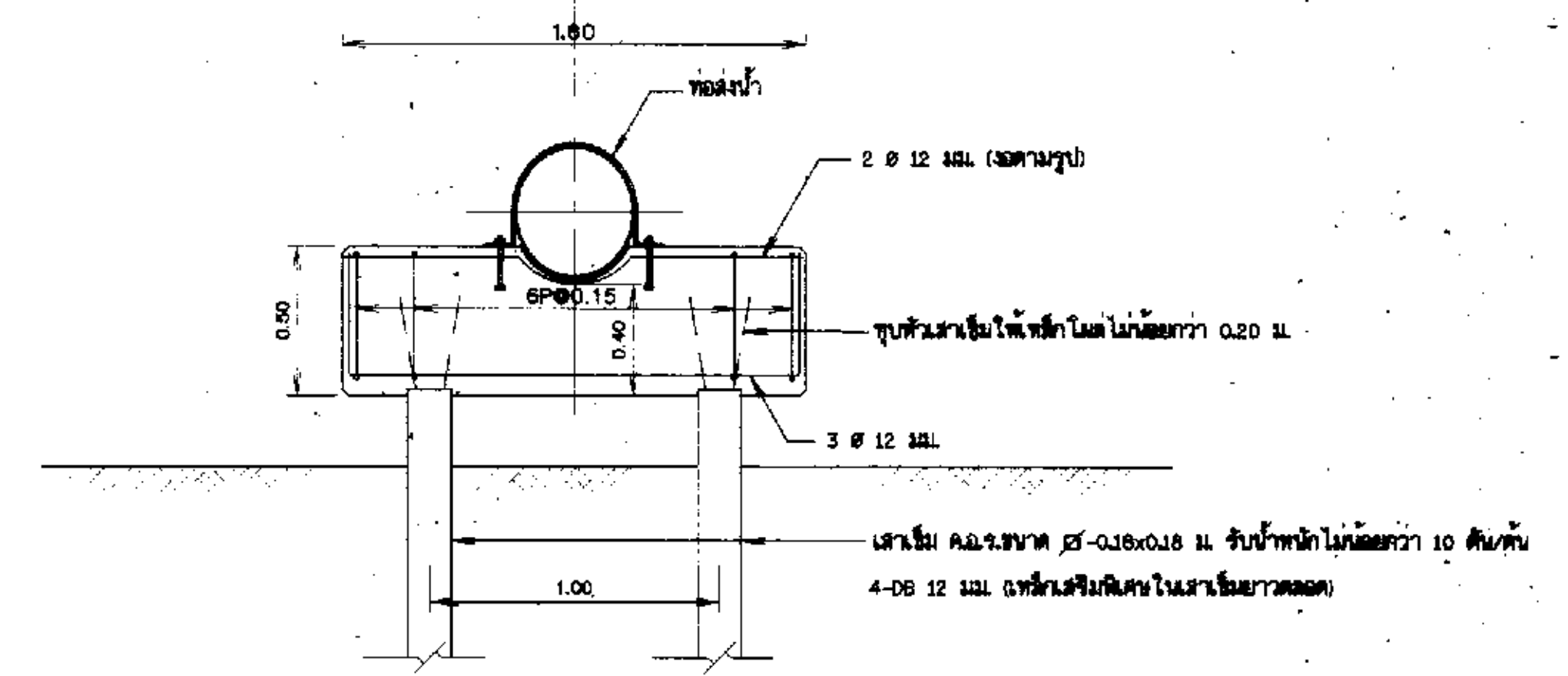
รูปตัด ก-ก
