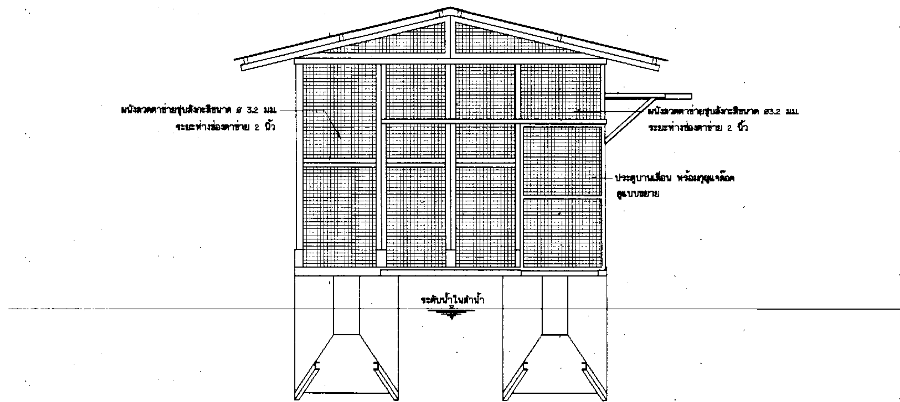
รูปด้าน 4 มาตราส่วน 1 : 25
