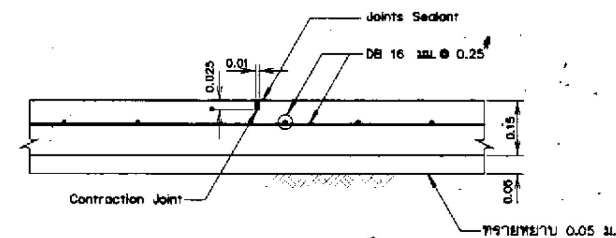
แบบขยายรอยต่อพื้น
