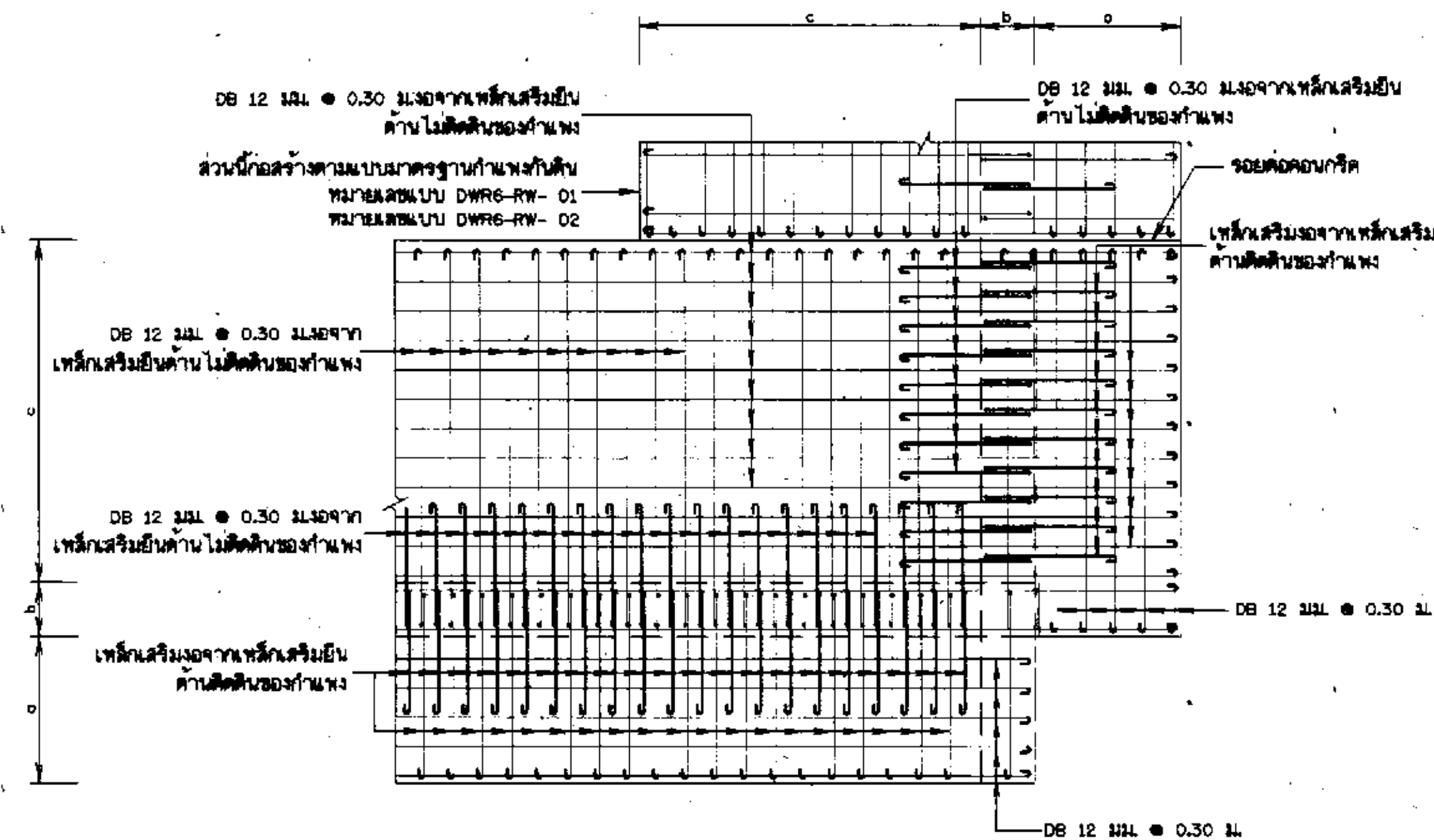
แปลนแสดงการเสริมเหล็กพื้นคานล่าง
