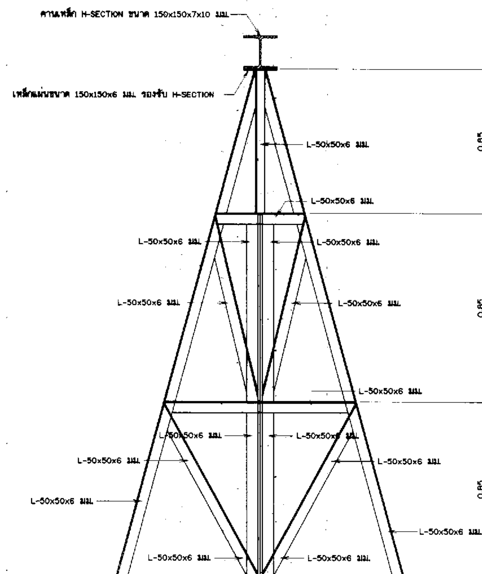
รูปขยายชาดั่งรูปตัว A รับคานเหล็ก
