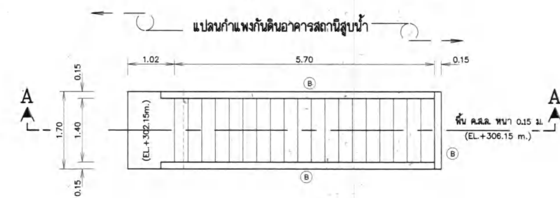
แปลนบันได มาตราส่วน 1:50
