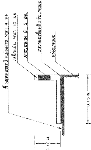
รูปตัดเหล็กยึดสลิง 1:5
