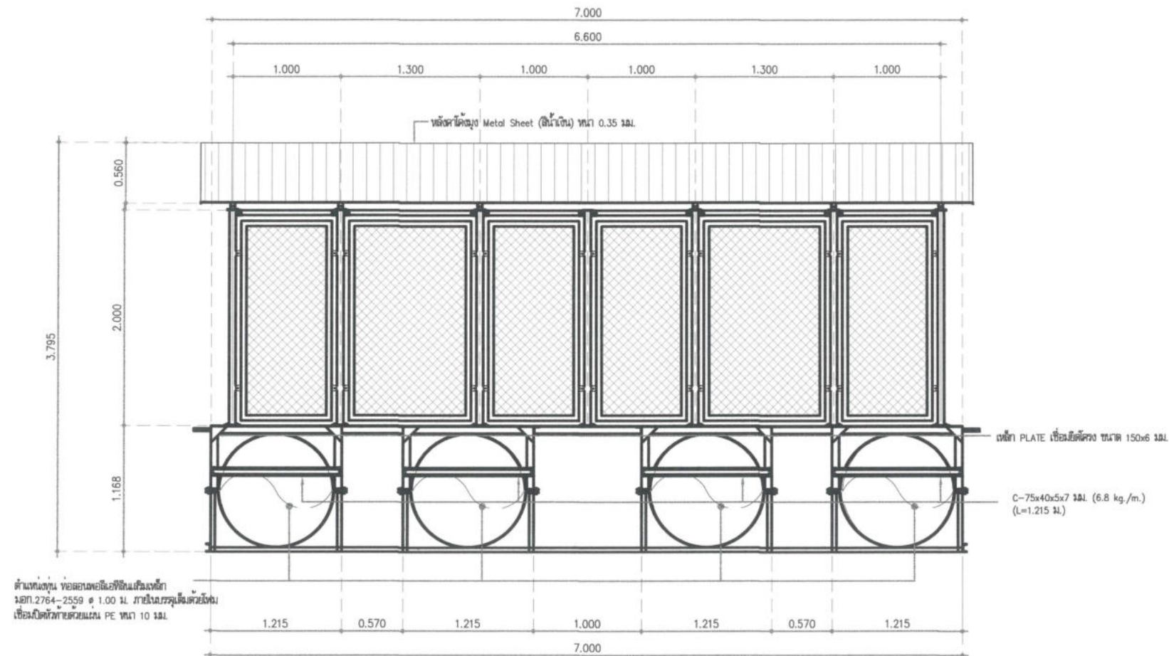
รูปด้าน 3 SCALE 1:50
