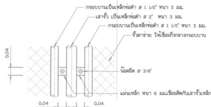
แบบขยายรายละเอียดแสดงการยึดระหว่างรื้อกับเสา ไม่แสดงขนาดราวล้วน
