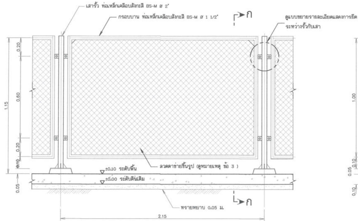
แบบขยายรั้วลวดตาข่าย ไม่แสดงมาตราส่วน
