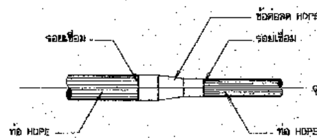
การบรรจุท่อ HDPE กับข้อต่อตรง HDPE
