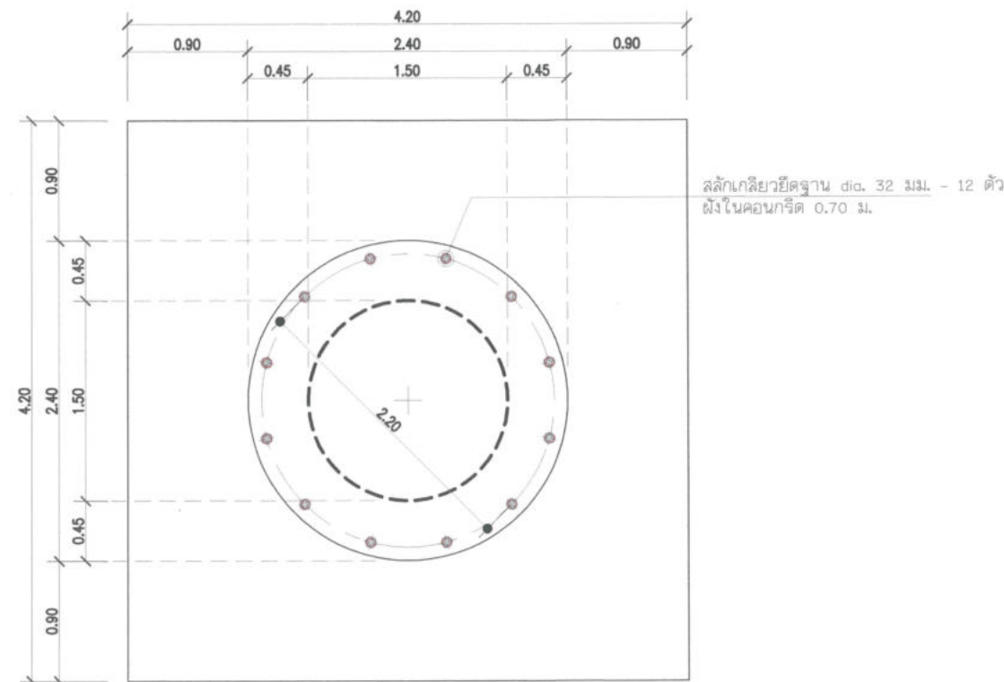
แบบขยายฐานรากห่อถังสูง (แบบฐานแฉก) มาตราส่วน 1 : 50
