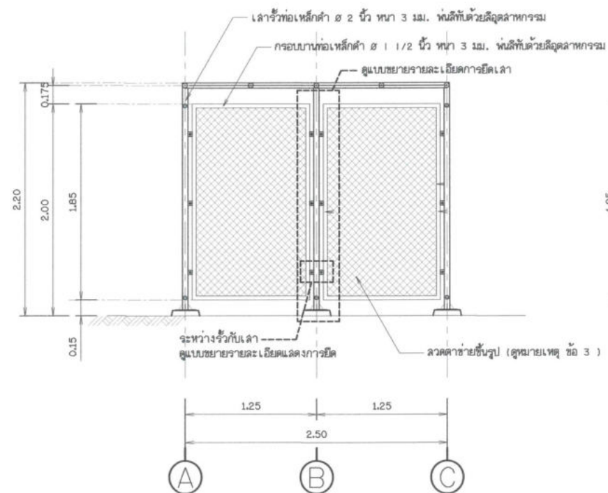
แบบขยาย ๒ ไม่แสดงขนาดราวล้วน
