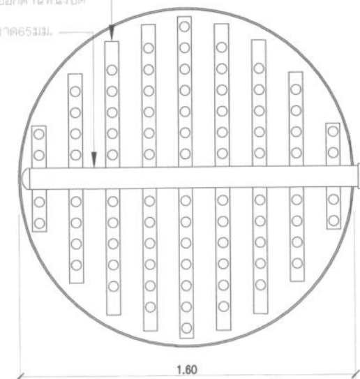
แบบขยายการวางท่อน้ำ มาตราส่วน 1 : 25
