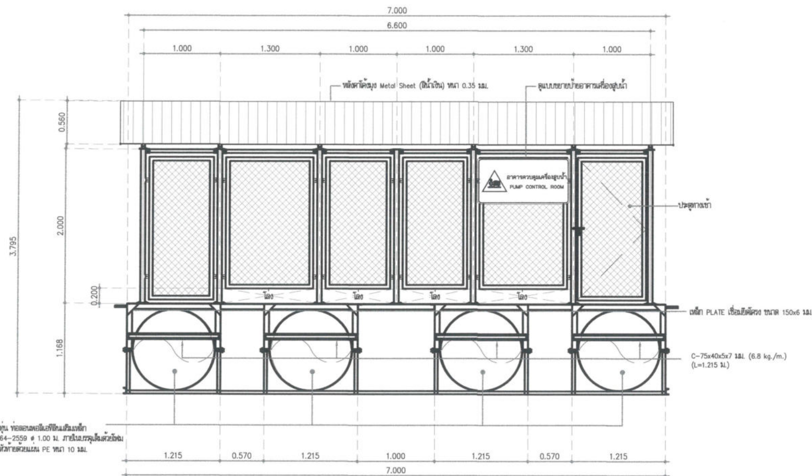
รูปด้าน 1
