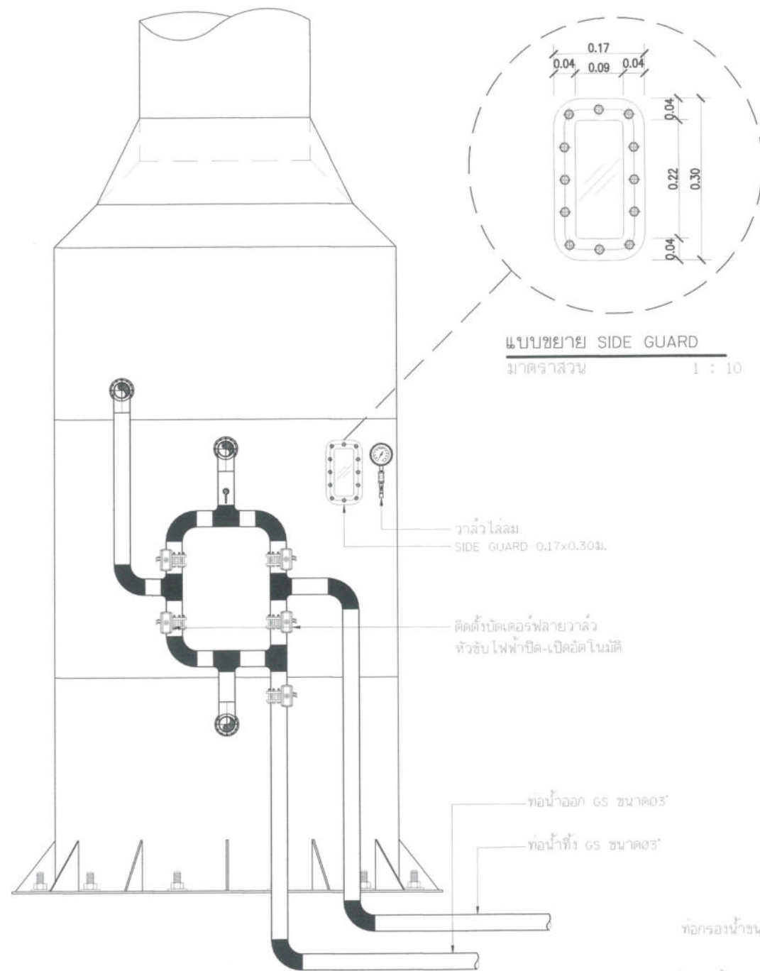
แบบขยายรูปด้านหน้าวาล์วกรอง มาตราส่วน 1 : 25
