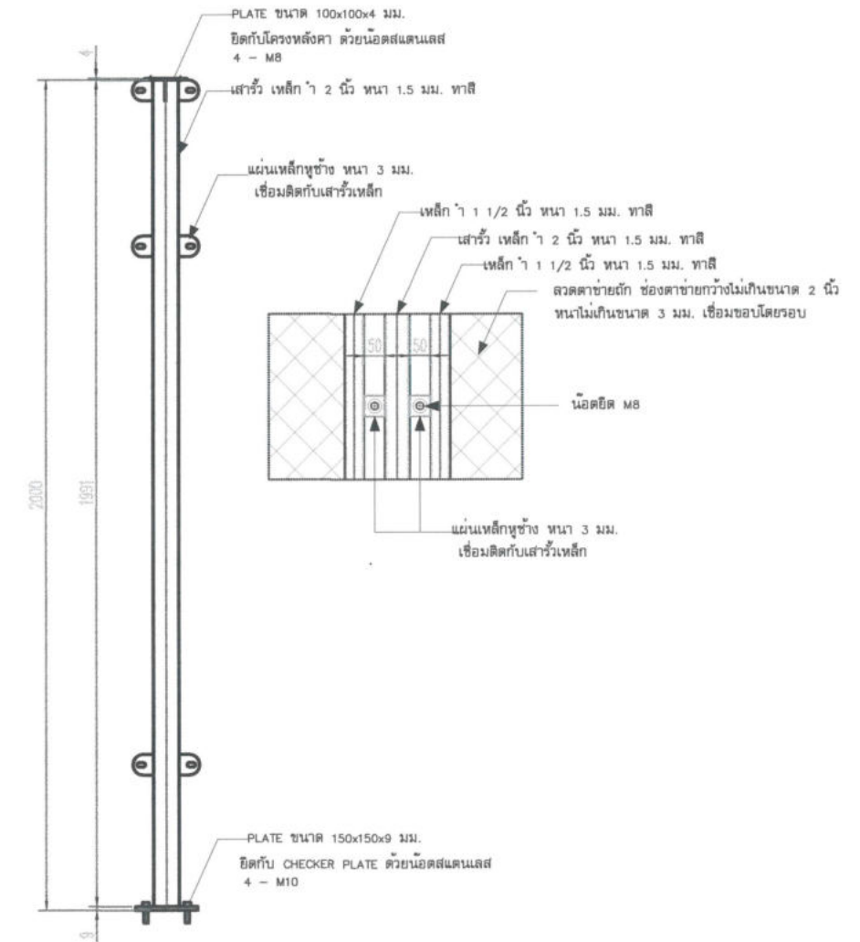
แบบขยายรายละเอียดแสดงการยึดรั้ว
