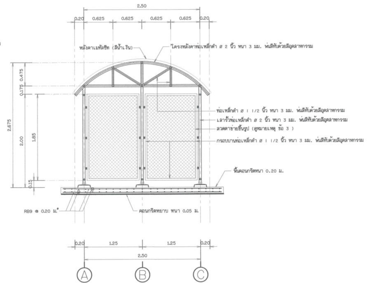
รูปตัด ข - ข ไม่แสดงขนาดราวล้วน
