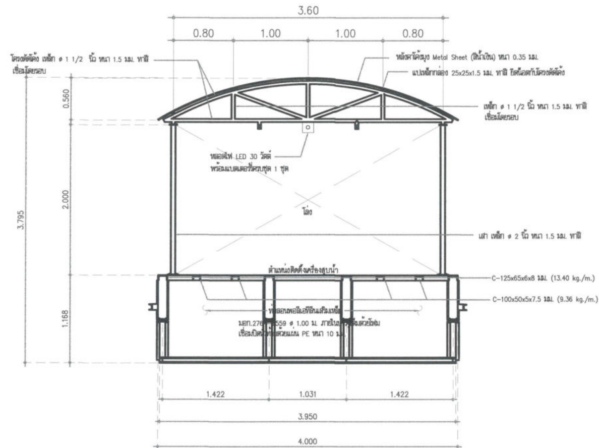
รูปตัด X - X SCALE 1:50
