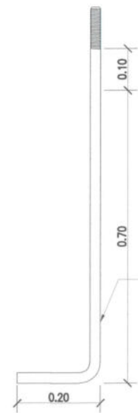
แบบขยายสลักเกลียวยึดฐาน มาตราส่วน 1 : 12.5
