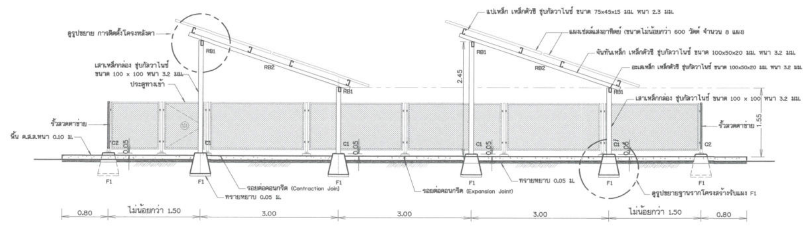
รูปด้านข้าง ไม่แสดงมาตราส่วน
