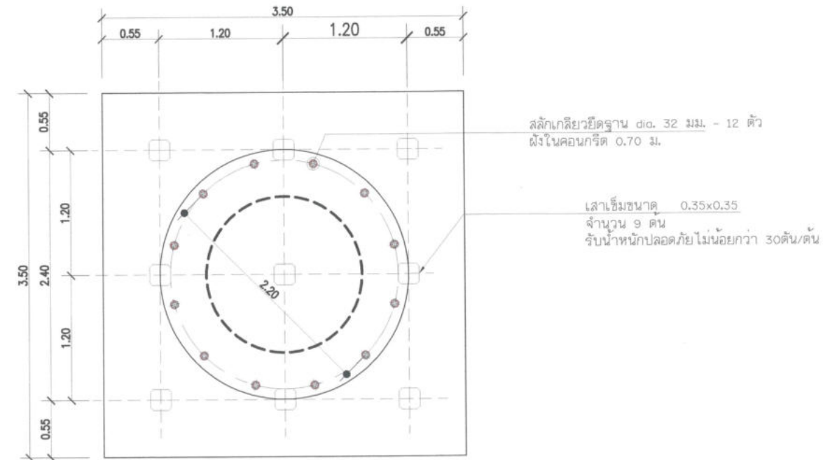
แบบขยายฐานรากห่อถังสูง (แบบเสาเข็ม) มาตราส่วน 1 : 50
