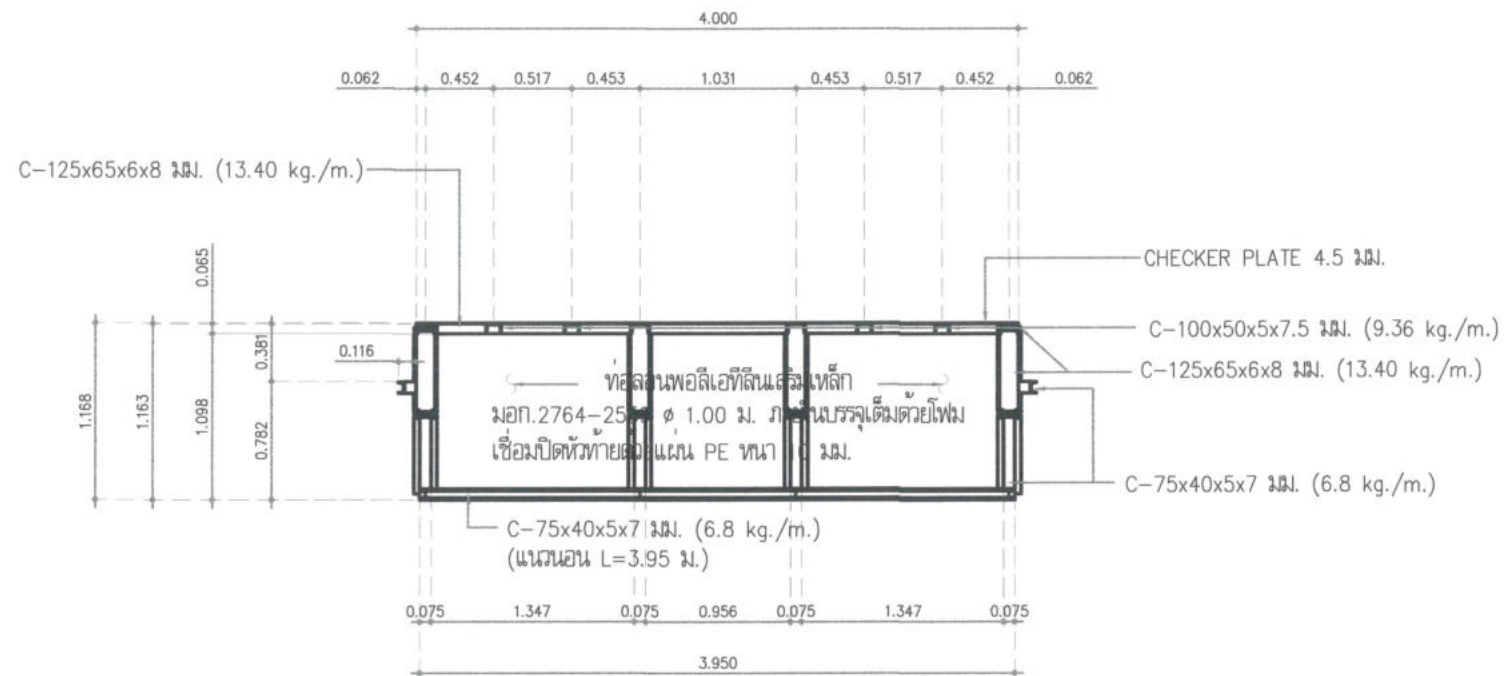
รูปตัด ก - ก SCALE 1:50
