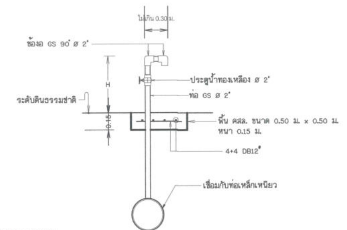
ก๊อกน้ำสำหรับล้างแ่ง มาตรฐาน 1 : 20
