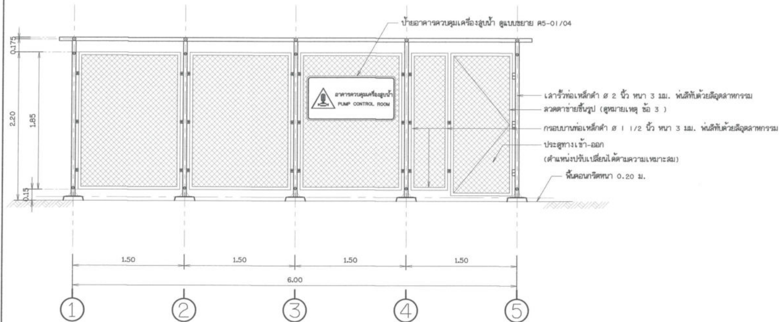
แบบขยาย ๑ ไม่แสดงขนาดราวล้วน
