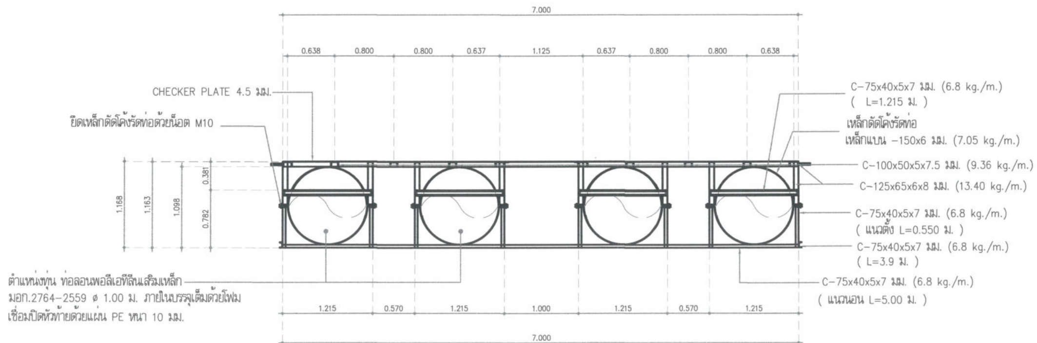
รูปตัด ข - ข SCALE 1:50
