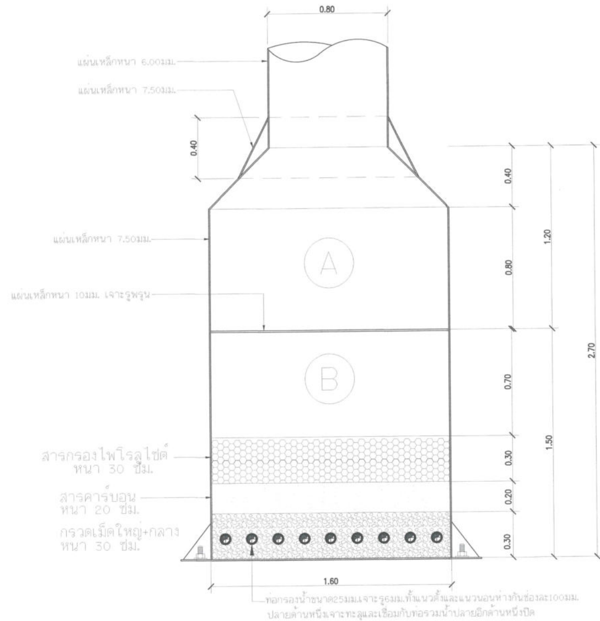
แบบขยายรูปตัดแสดงสารกรอง มาตราส่วน 1 : 25
