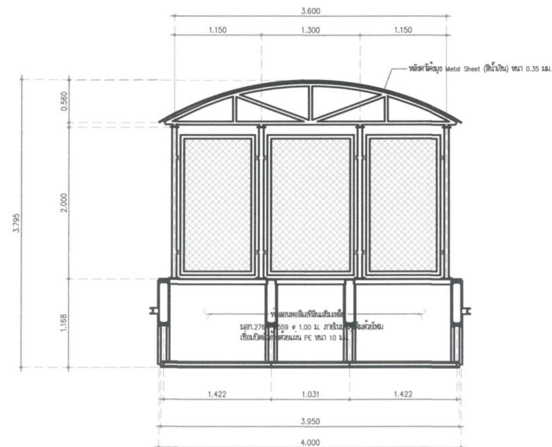
รูปด้าน 4 SCALE 1:50
