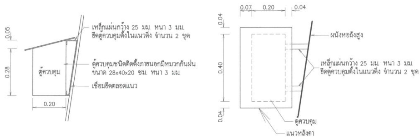
แบบขยายตู้ควบคุม ไม่แสดงมาตราส่วน
