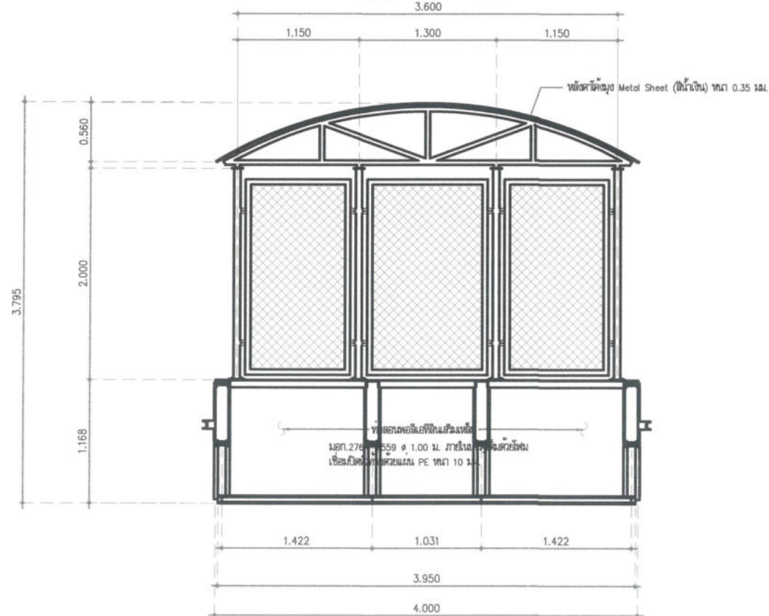
รูปด้าน 2
