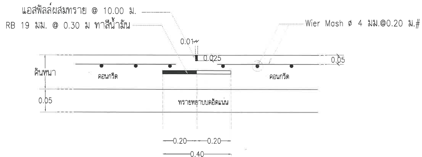
[CONTRACTION JOINT] ทูกระยะ 10.00 ม.
