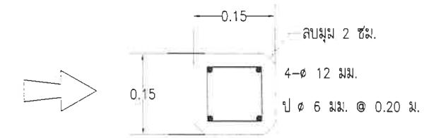
ขยายเสาป้ายฐานเสา - ตัวแผ่นป้าย SCALE 1:10
