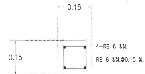
แบบขยายเหล็กเสริมหลักบ่อแนว มาตราส่วน 1:10
