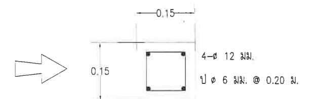
ขยายเสาป้ายได้ป้าย - หัวเสา SCALE 1:10
