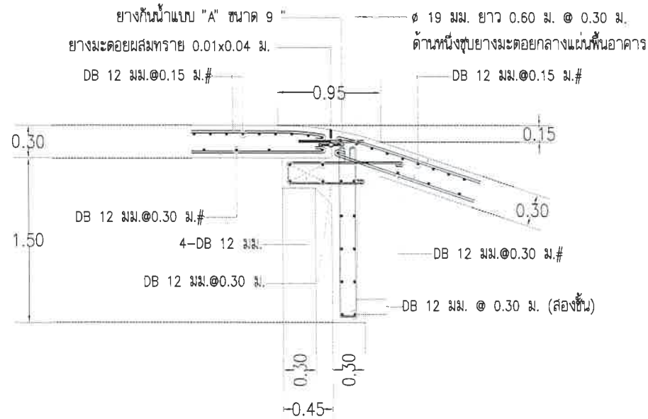
แบบขยาย 5 มาตราส่วน 1:50
