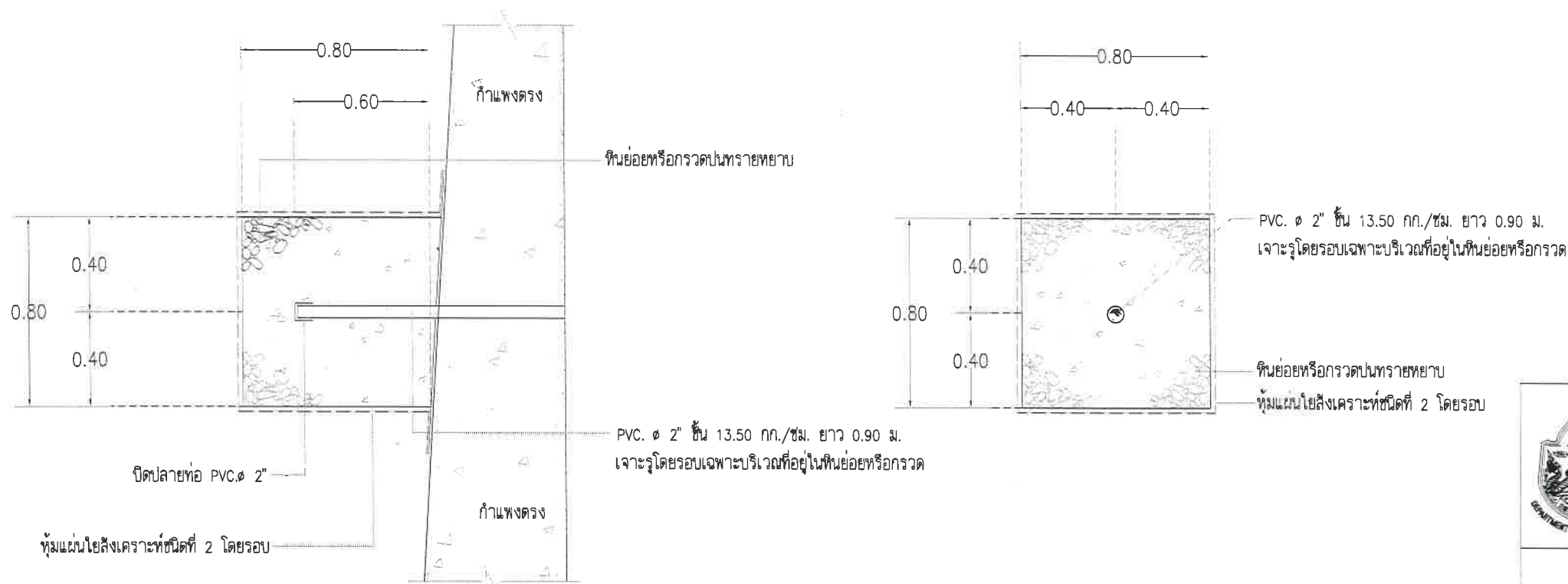
ขยายท่อลดแรงดันด้านข้างกำแพงแบบที่ 1 [กำแพงตรง] SCALE 1:25
