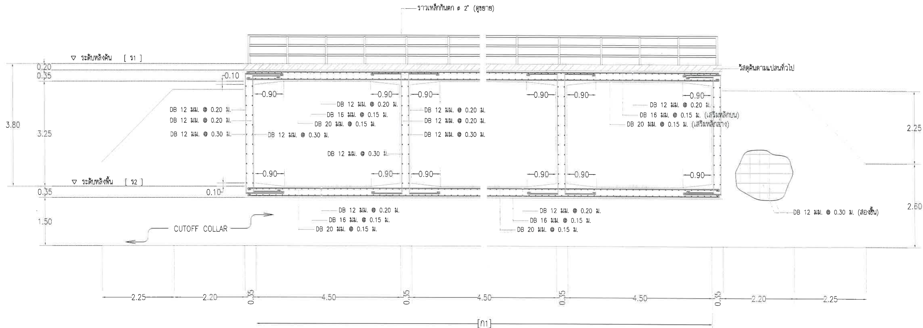
รูปตัดตามขวางท่อเหลี่ยม คลล. มาตราส่วน 1:50
