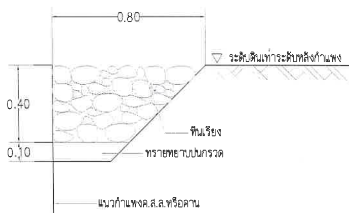
ขยายรูปตัด 2 หินเรียงสำหรับกว้าง 0.80 ม. มาตราส่วน 1:20
