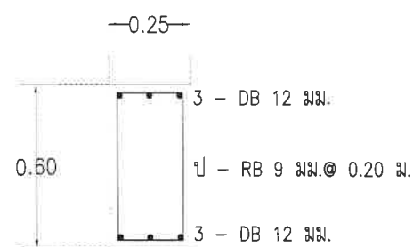
ขยายคานขอบโดยรอบบันได SCALE 1:25
