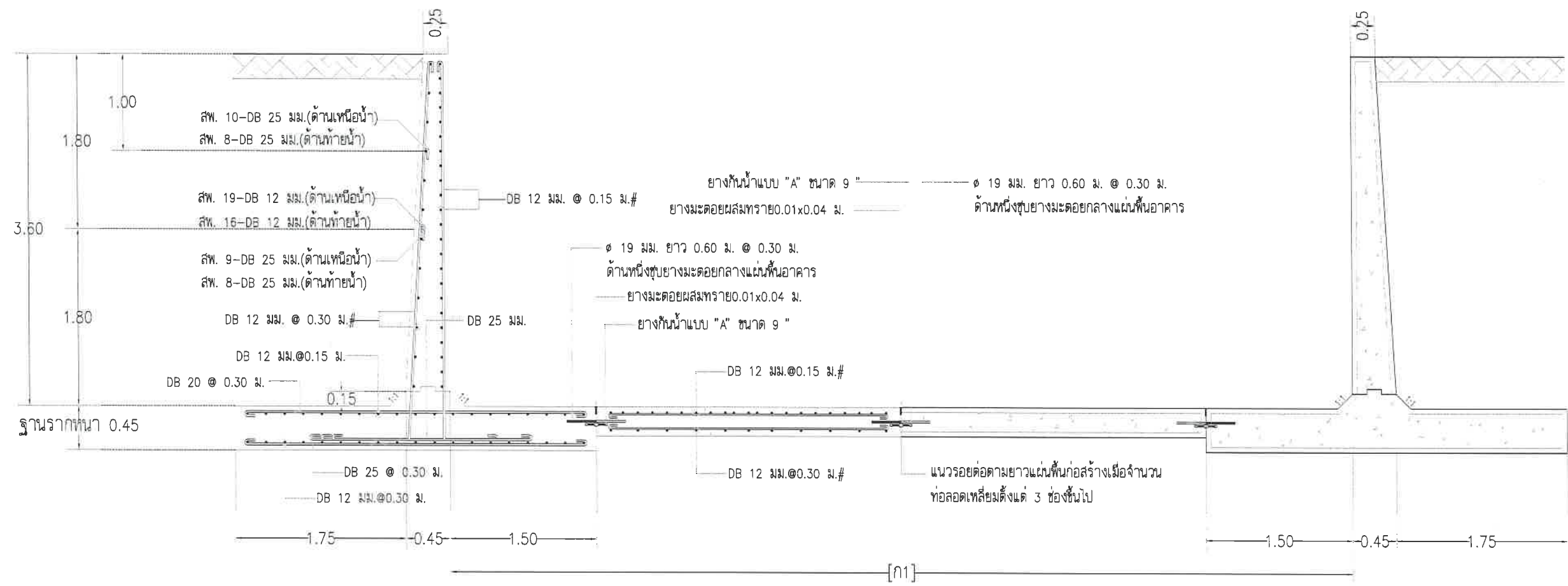
รูปตัดแสดงการเสริมเหล็ก ช่วงกำแพงสูง 1.80-3.60 ม. พื้น รอยต่อ อาคารระบายน้ำ มาตราส่วน 1:50
