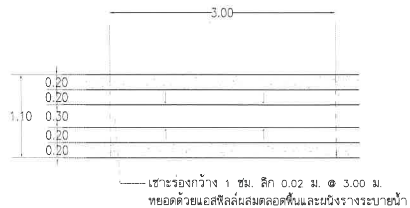
แปลนรางระบายน้ำ มาตราส่วน 1:50
