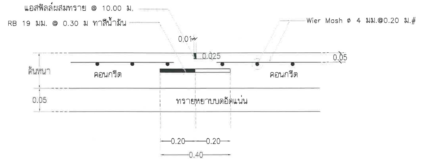
[CONTRACTION JOINT] ทกระยะ 10.00 ม.
