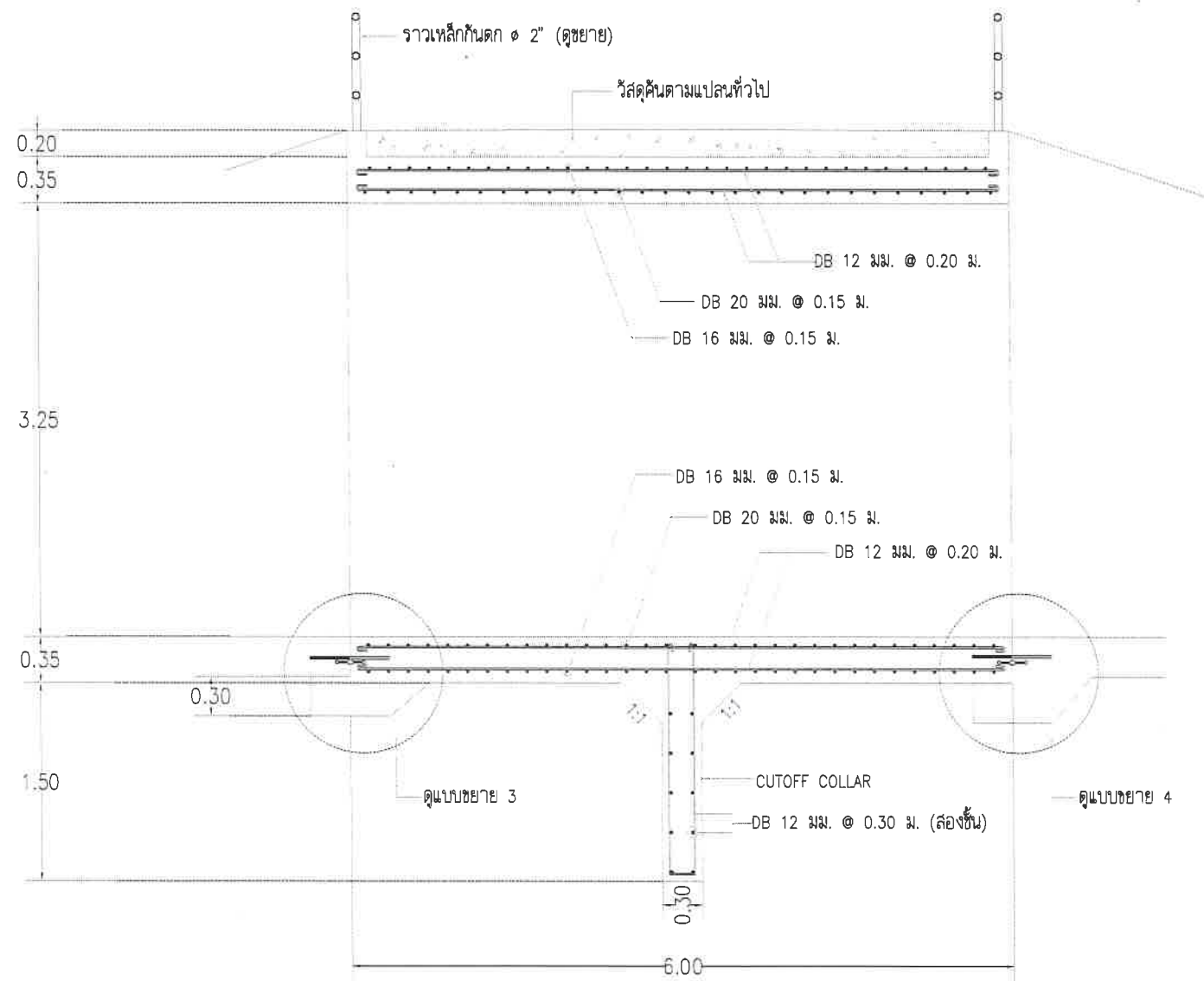
รูปตัดตามยาวท่อเหลี่ยม คลล. มาตราส่วน 1:50
