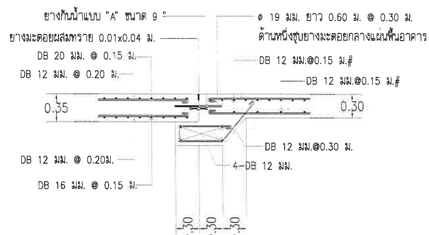
แบบขยาย 4 มาตราส่วน 1:50
