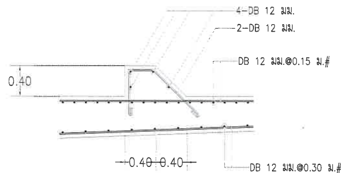
แบบขยาย 9 มาตราส่วน 1:50
