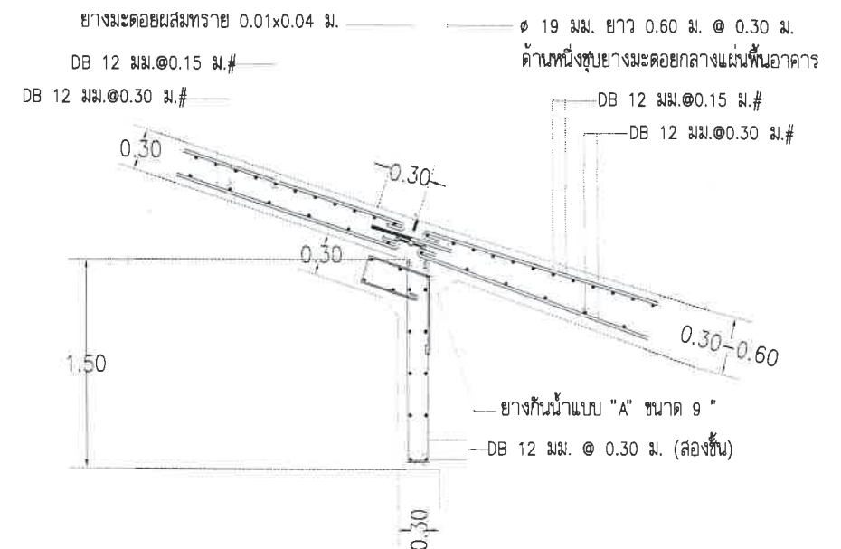
แบบขยาย 7 มาตราส่วน 1:50
