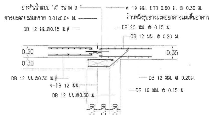
แบบขยาย 3 มาตราส่วน 1:50
