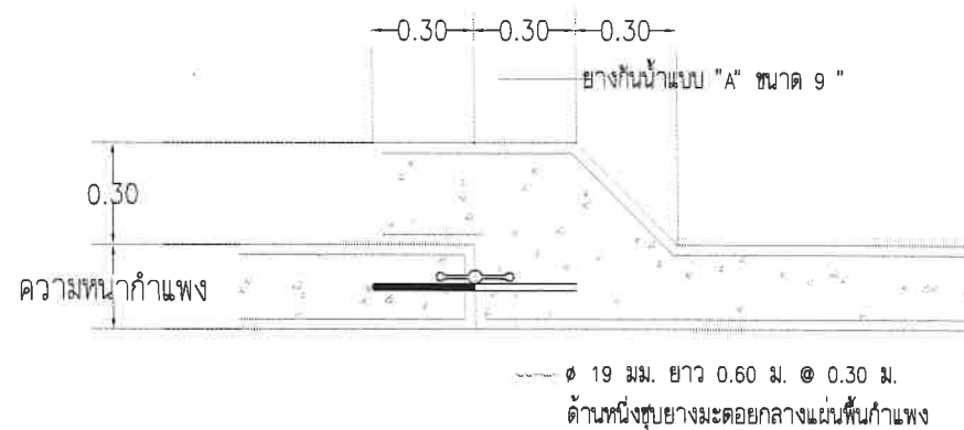
แบบขยายรอยต่อกำแพง มาตราส่วน 1:25
