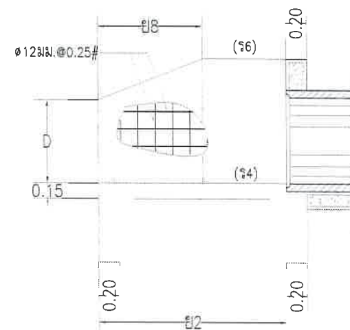
แบบขยายเหล็กเสริมกำแพงปากทางน้ำเข้า มาตราส่วน 1:25
