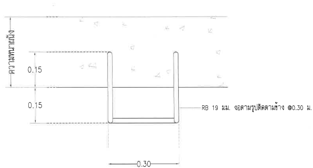
แปลนบันไดลิง
