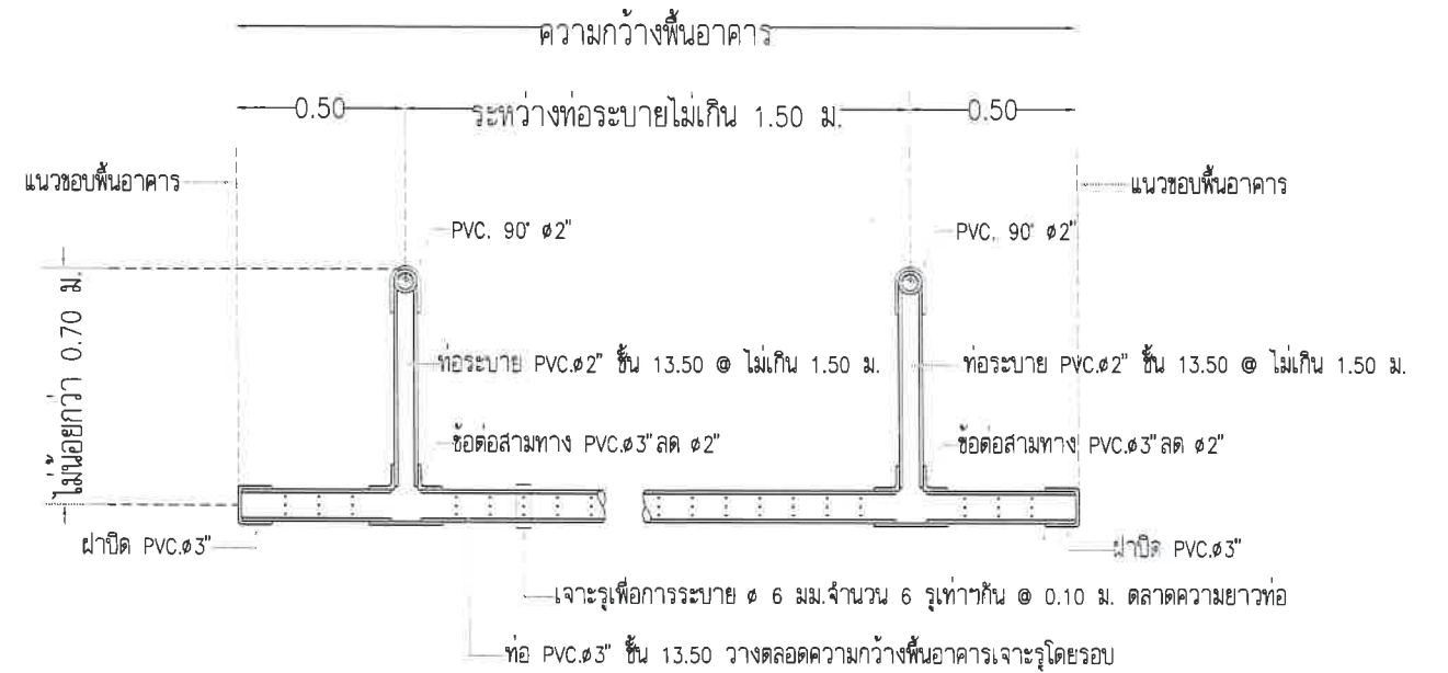
ขยายท่อลดแรงดันน้ำที่พื้นแบบที่ 2 [ห้องพื้นเอียง] SCALE 1:25
