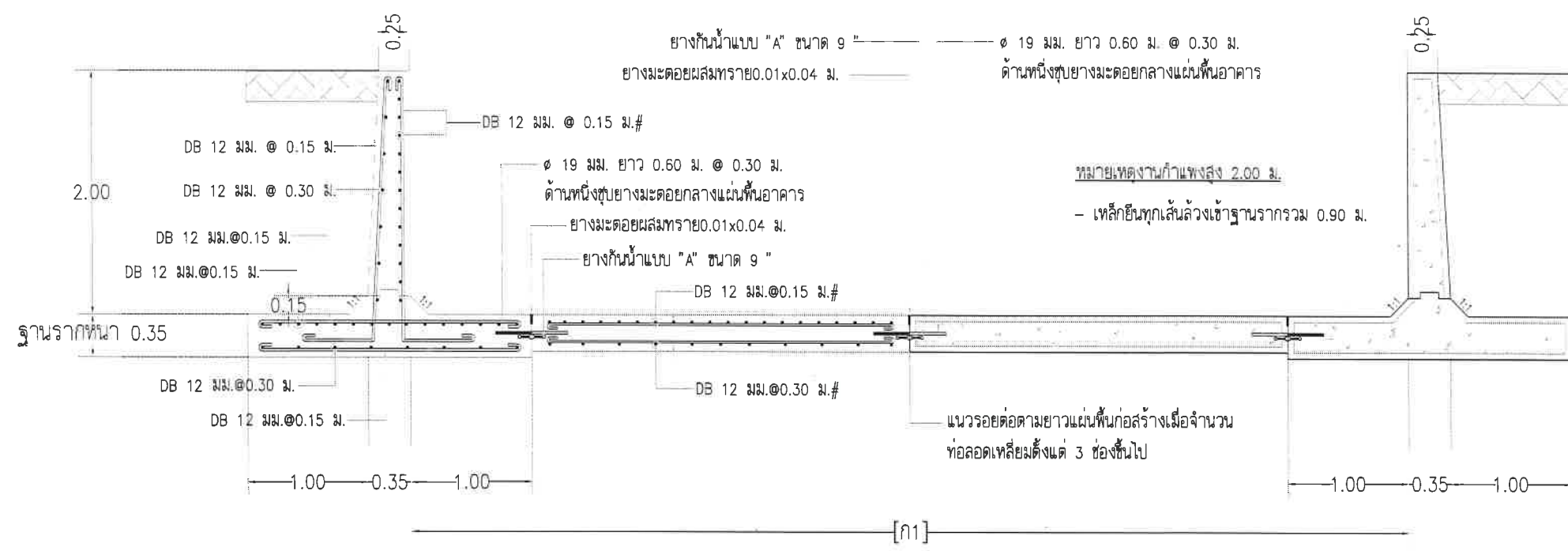
รูปตัดแสดงการเสริมเหล็ก ช่วงกำแพงสูง 2.00 ม. พื้น รอยต่อ อาคารระบายน้ำ มาตราส่วน 1:50
