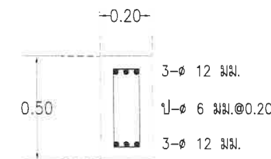
ขยายคานช่วงใน มาตราส่วน 1:25
