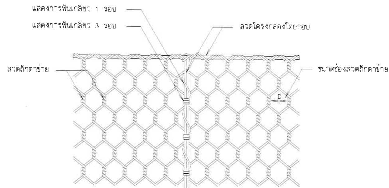
รูปแสดงการพันลวดระหว่างกล่องลวดตาข่ายและฝาบปิด
