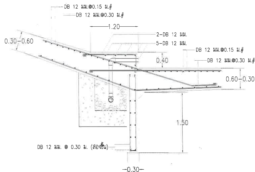
แบบขยาย 8 มาตราส่วน 1:50
