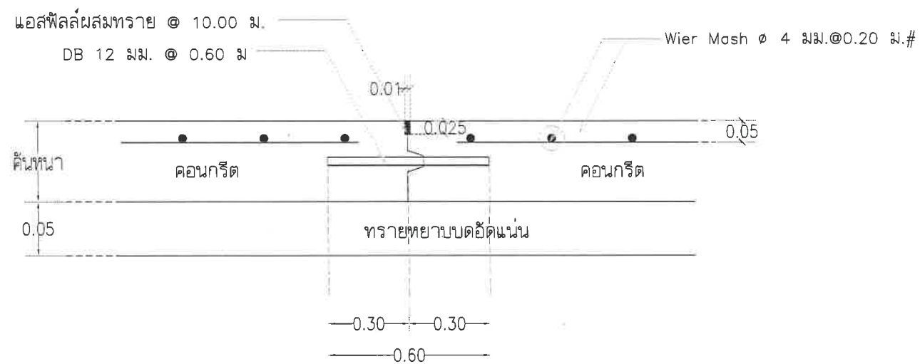
[LONGITUDINAL JOINT] เมื่อความกว้างคั่นมากกว่า 5.00 ม.
