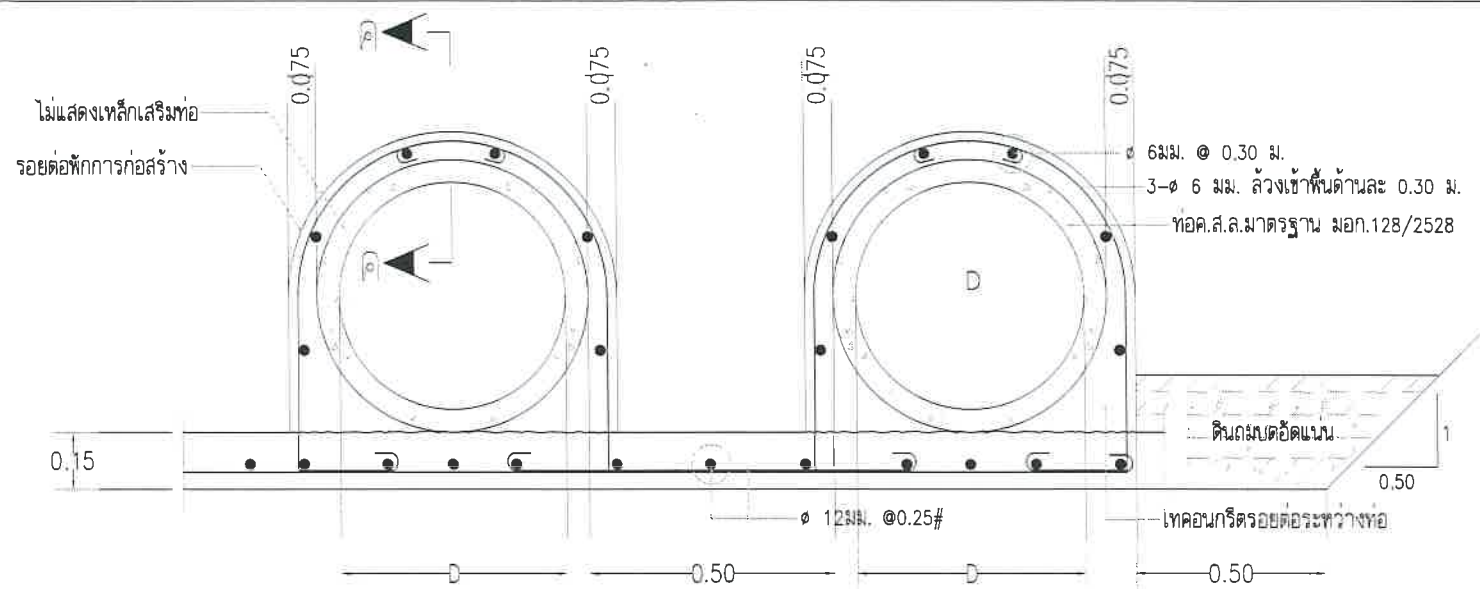
รูปตัดการวางท่อ ค.ส.ล. มาตราส่วน 1:20
