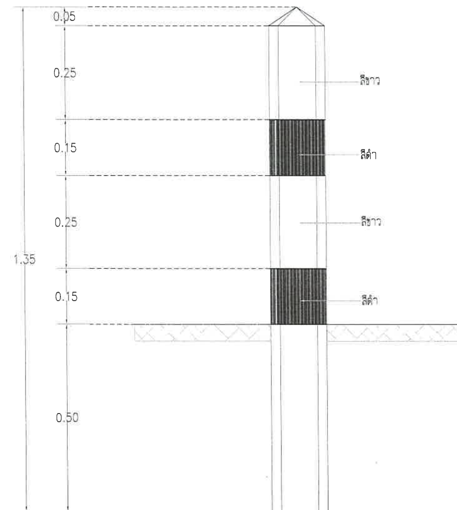
แบบขยายเหล็กเสริมหลักบ่อแนว มาตราส่วน 1:10
