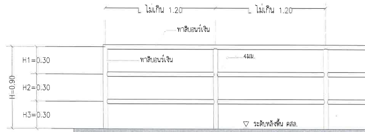
แสดงรูปด้านราวกันตก มาตราส่วน 1:25
