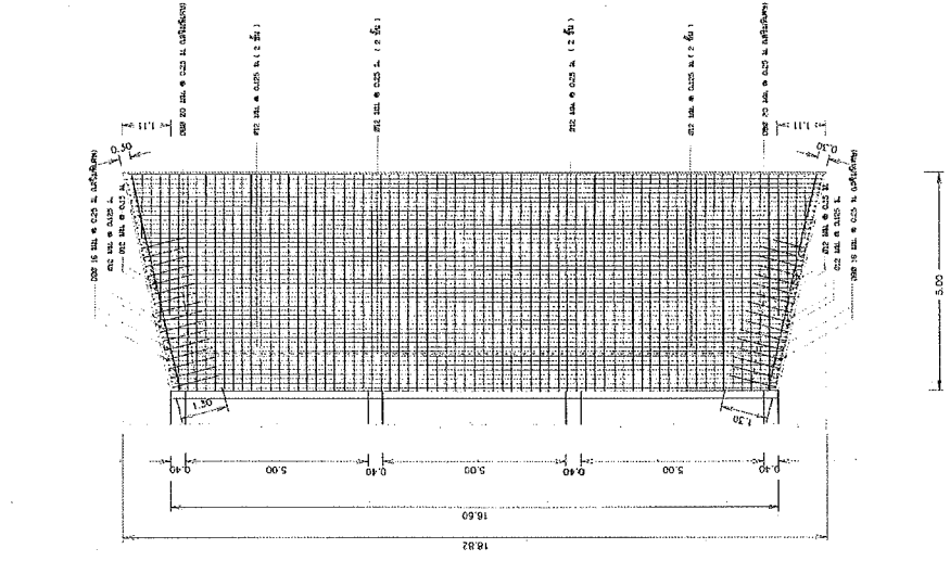
แบบขยายการเสริมเหล็กพื้นทางขึ้น
