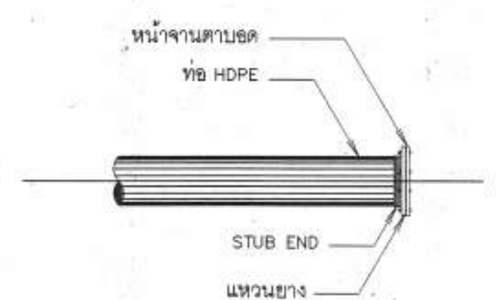
การปิดปลายท่อ
