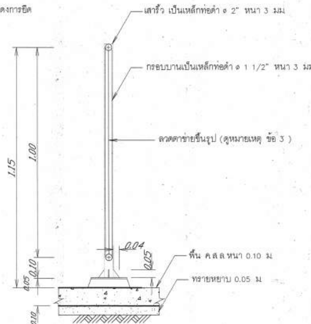
รูปตัด ก-ก
