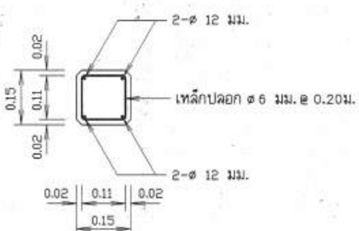
รูปตัด 2 - 2 มาตรฐาน 1:10
