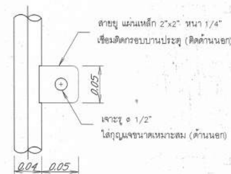
แบบขยายสายยู
