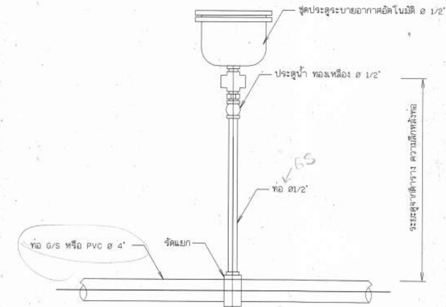
12. การติดตั้งประตูปะบายอากาศอัตโนมัติ
