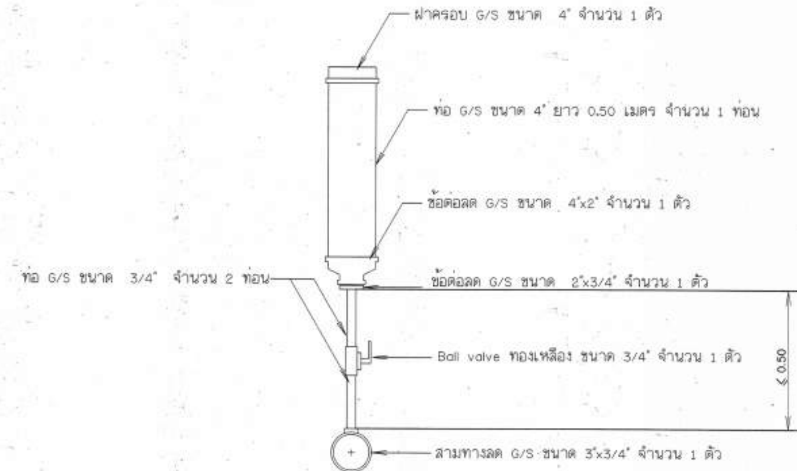
11. ช่องเติมน้ำ
