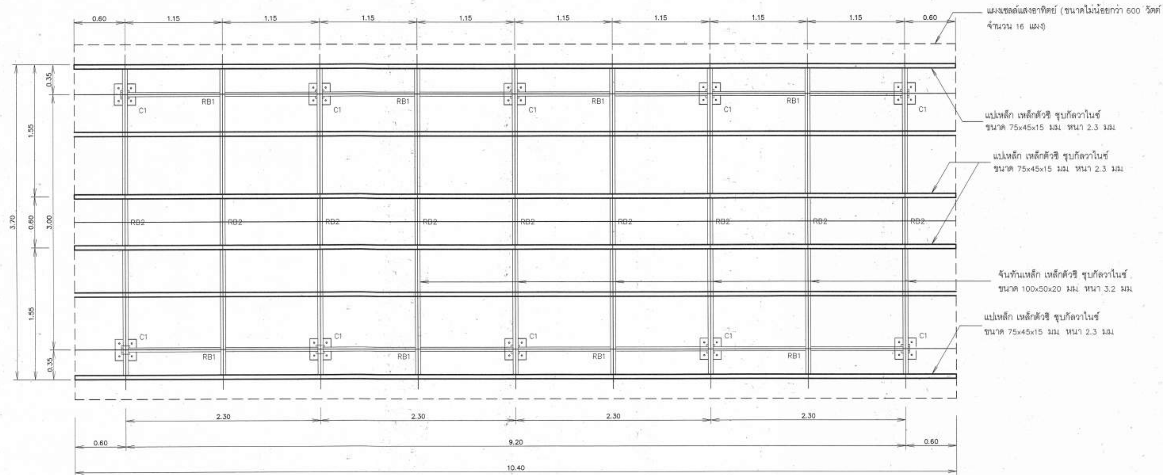
แปลนฐานรากและโครงหลังคา ไม่แสดงขนาดส่วน
