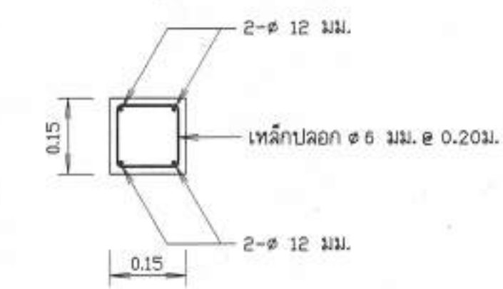
รูปตัด 1 - 1 มาตรฐาน 1:10
