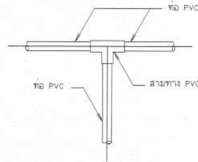
10. แบบการต่อสามทาง PVC
