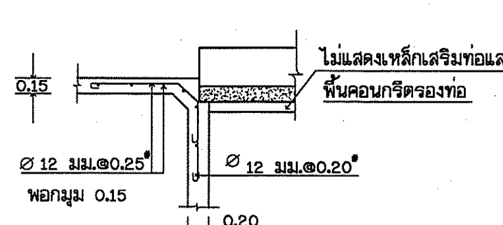
ขยาย (4) ไม่แสดงมาตราส่วน
