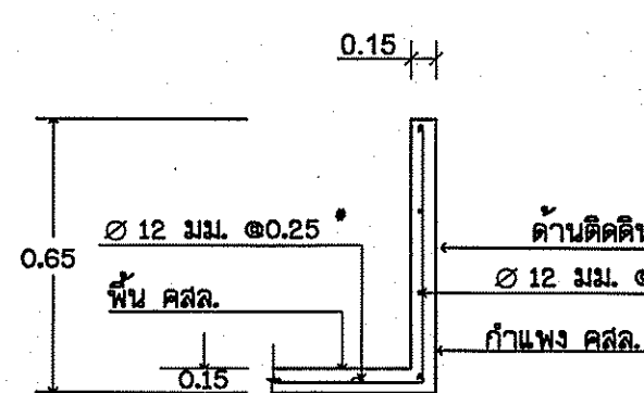
รูปตัด (ข) - (ข) (ความหนาพื้น 0.15 ม.) ไม่แสดงมาตราส่วน
