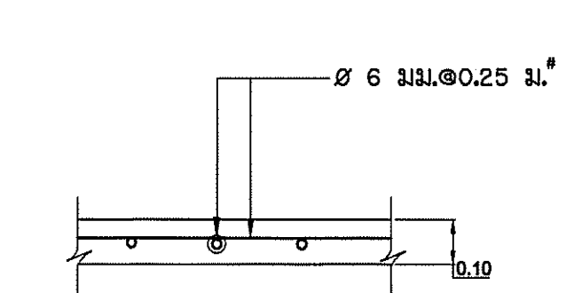
แบบขยาย 2
