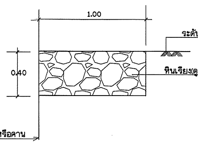
ขยายหินเรียง 2 ไม่แสดงมาตราส่วน
