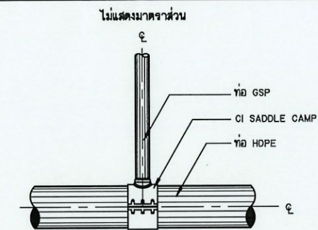
การบรรจุท่อสามทาง HDPE กับท่อ GSP แบบ CI SADDLE CLAMP (สำหรับอาคารจุดปล่อยน้ำ อาคารประจําขยะบดก่อน อาคารท่อระบายอากาศ กรณีที่ท่อส่งน้ำขนาดเส้นผ่านศูนย์กลางน้อยกว่าหรือเท่ากับ 315 มม.)
