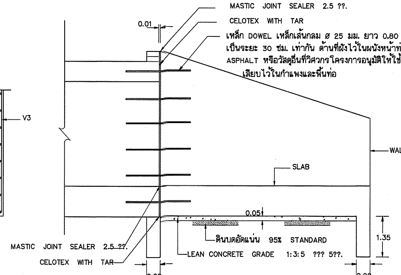
รายละเอียดรอยต่อเพื่อการขยายตัว NOT TO SCALE
