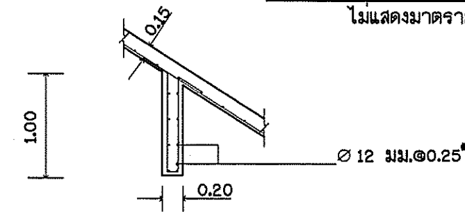
ขยาย CUT OFF ไม่แสดงมาตราส่วน
