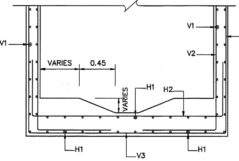
รูปตัด ๑๔ NOT TO SCALE
