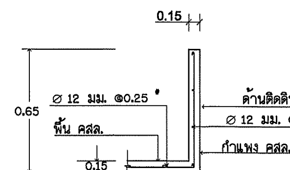
รูปตัด ก-ก (ความหนาพื้น 0.15 ม.) ไม่แสดงมาตราส่วน
