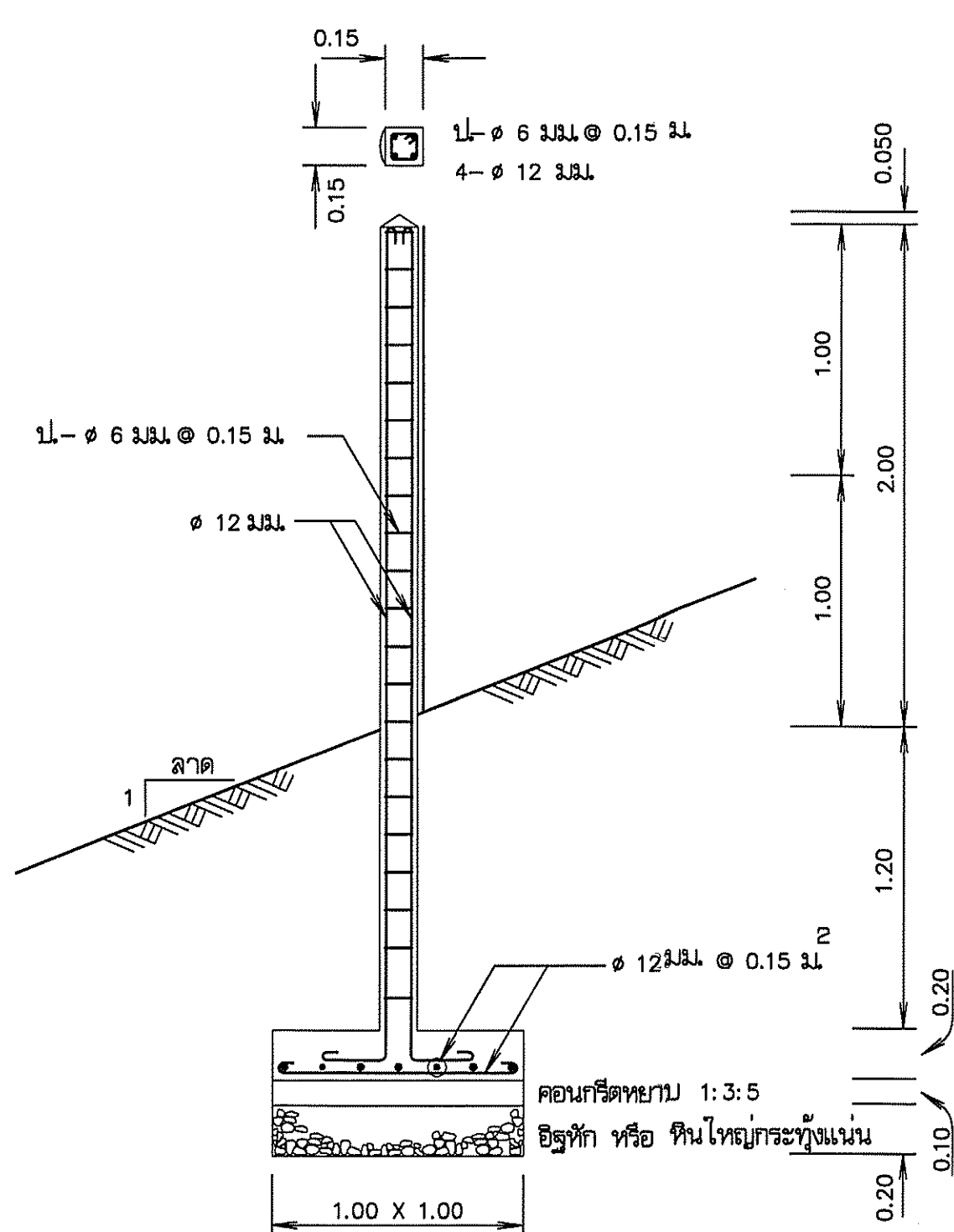
ขยายหลัก คส.บอกระดับน้ำ
