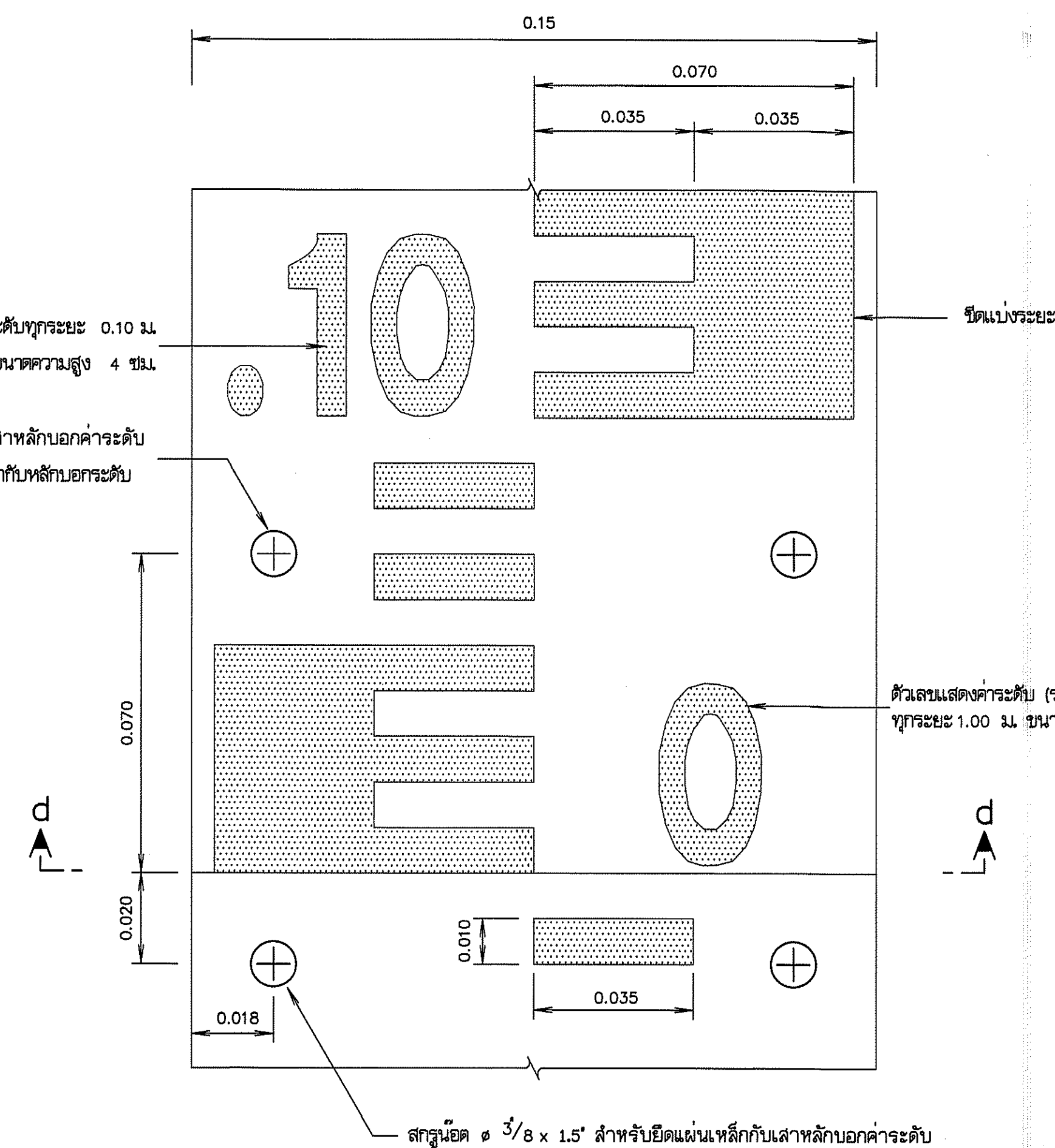
ขยายแผ่นหลักบอกระดับน้ำ
