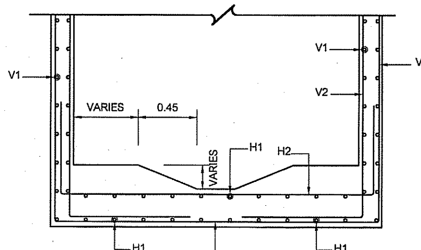
รูปตัด ③ NOT TO SCALE
