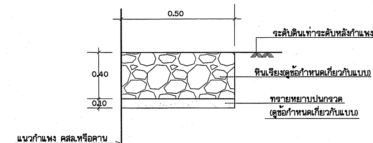
ขยายพื้นเรียบ 2 ไม่แสดงมาตราส่วน
