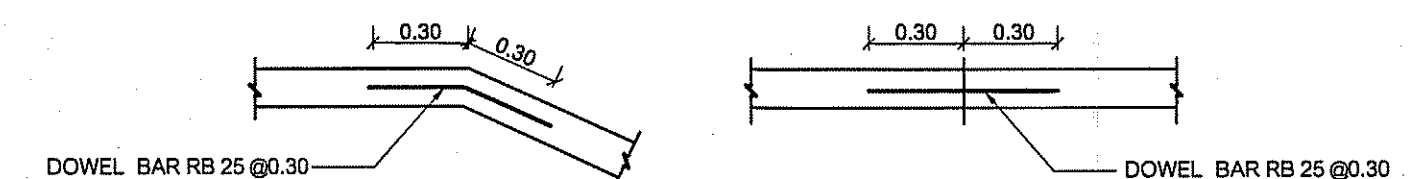
รายละเอียด ① ไม่แสดงมาตราส่วน
