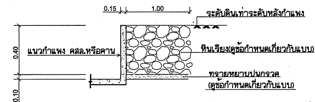
ขยายพื้นเรียบ 1 ไม่แสดงมาตราส่วน
