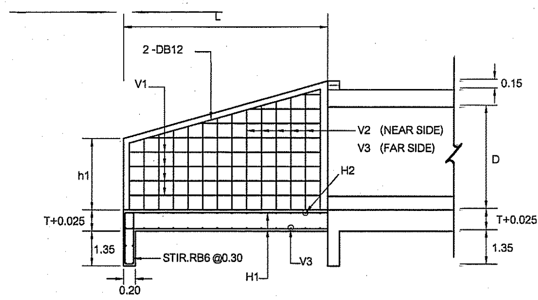
รูปตัด ① NOT TO SCALE
