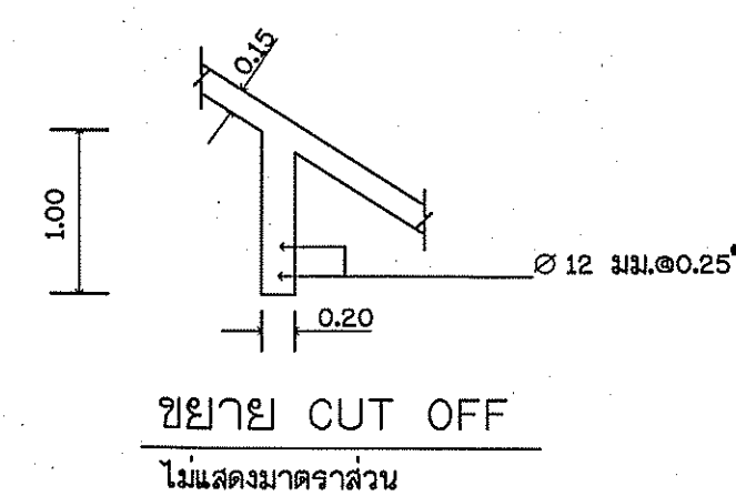
รูปตัด (ค) - (ค) (ความหนาพื้น 0.15 ม.) ไม่แสดงมาตราส่วน
