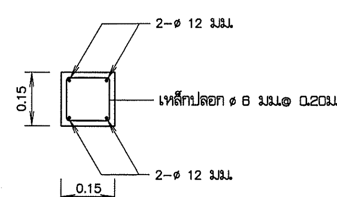
รูปตัด ก - ก
