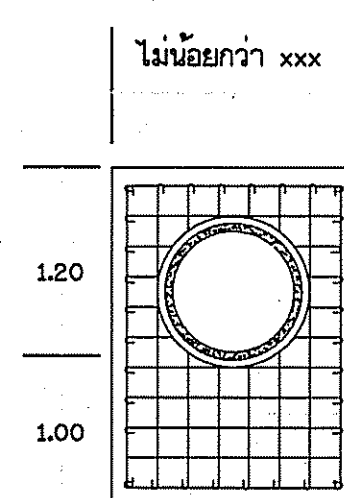
ขยายการเสริมเหล็กกำแพงปากท่อและท้ายท่อ (HEAD WALLS)
