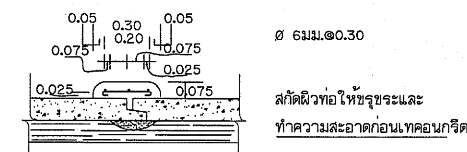
รูปตัด ก-ก ไม่แสดงขนาดบางส่วน
