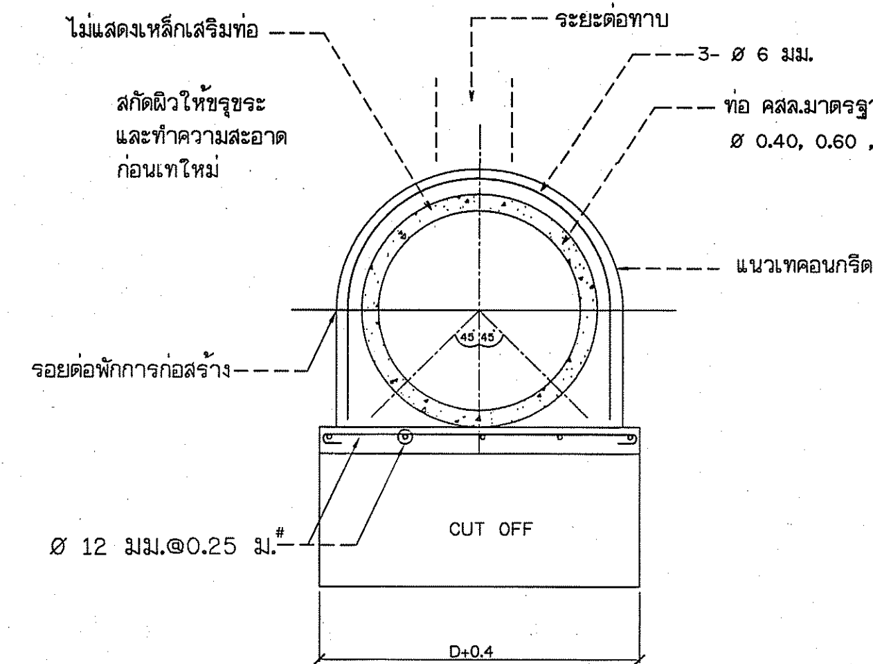
รูปตัด ก-ก ไม่แสดงขนาดบางส่วน
