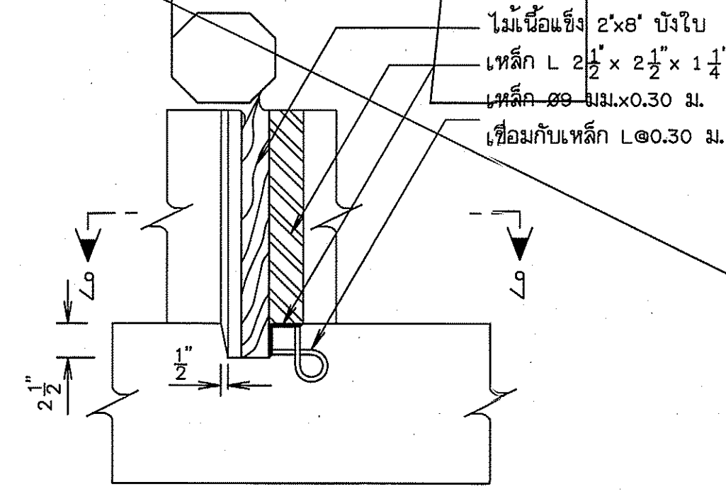
รูปขยายช่องใส่บานไม้ มาตราส่วน 1:10
