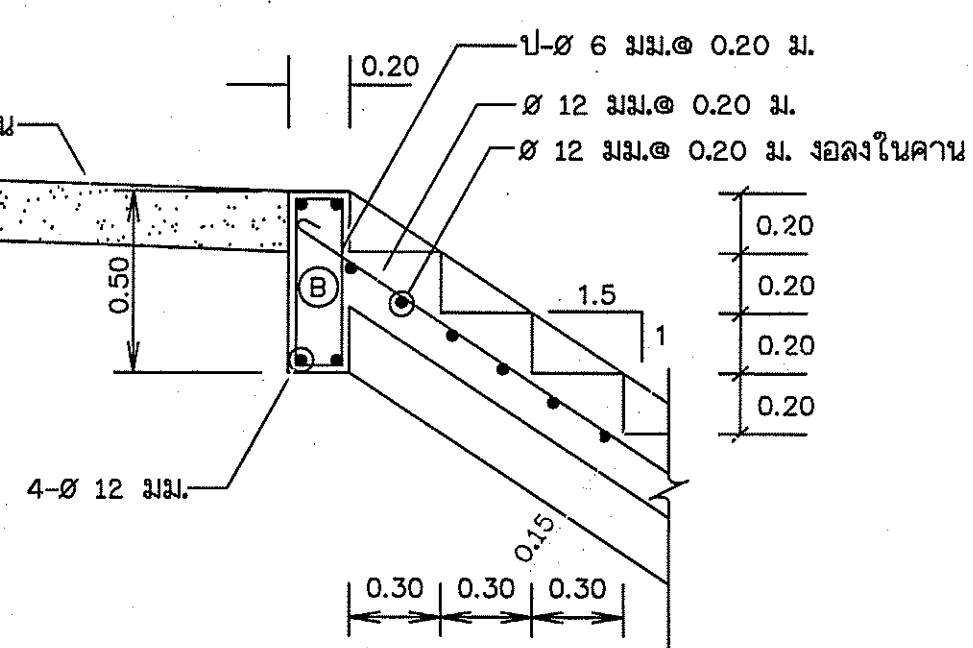
รูปตัด ค - ค ไม่แสดงมาตราส่วน
