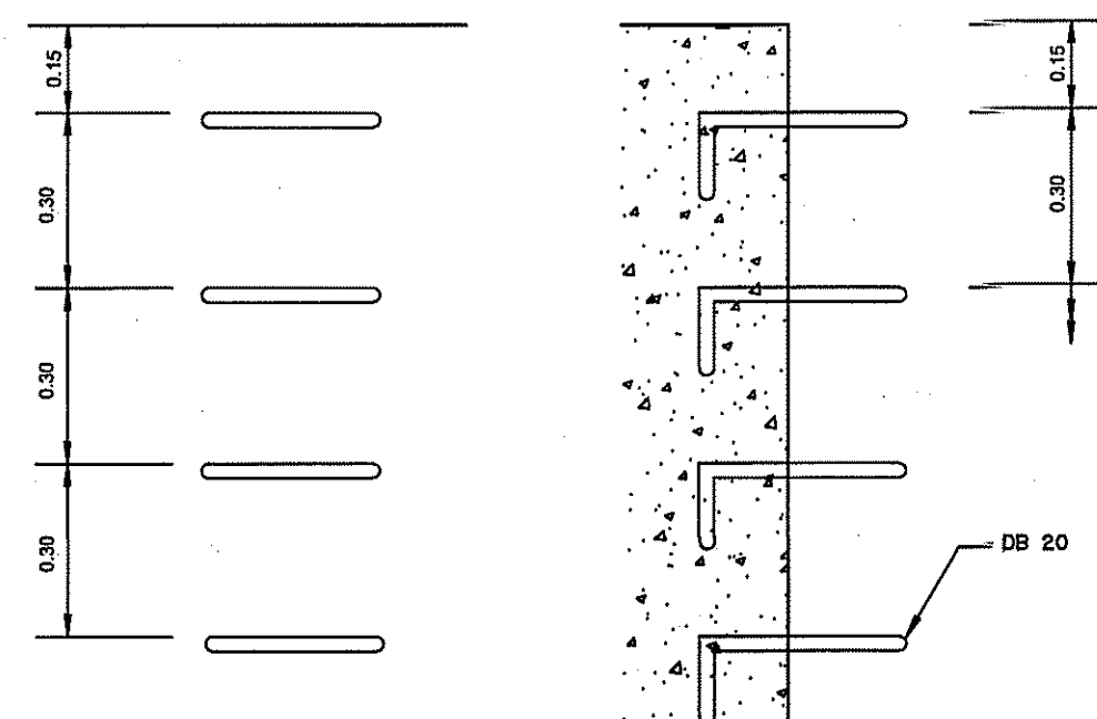
รูปขยายบันไดลิ้น ไม่แสดงมาตราส่วน
