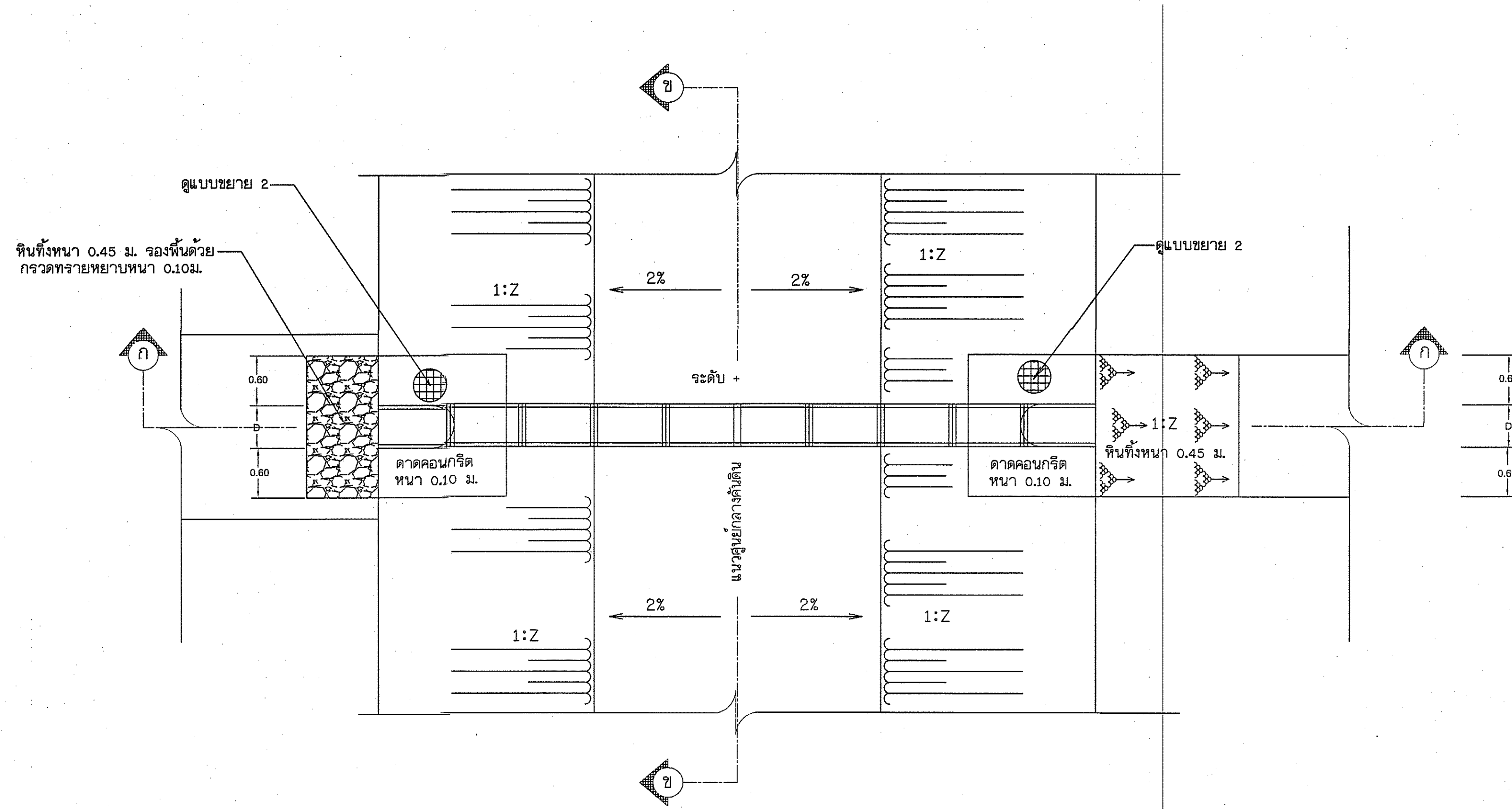
แปลนอาคารทางน้ำเข้า ไม่แสดงขนาดบางส่วน
