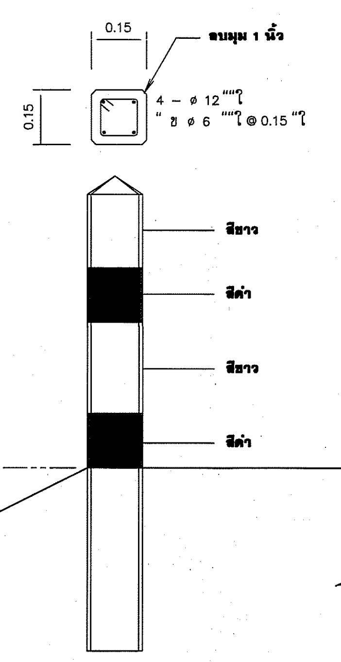
แบบขยายหลักริมคันดิน ไม่แสดงมาตราส่วน
