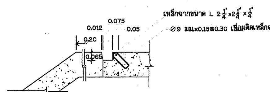
ขยายช่องใต้ประตูไม้ ไม่แสดงมาตราส่วน
