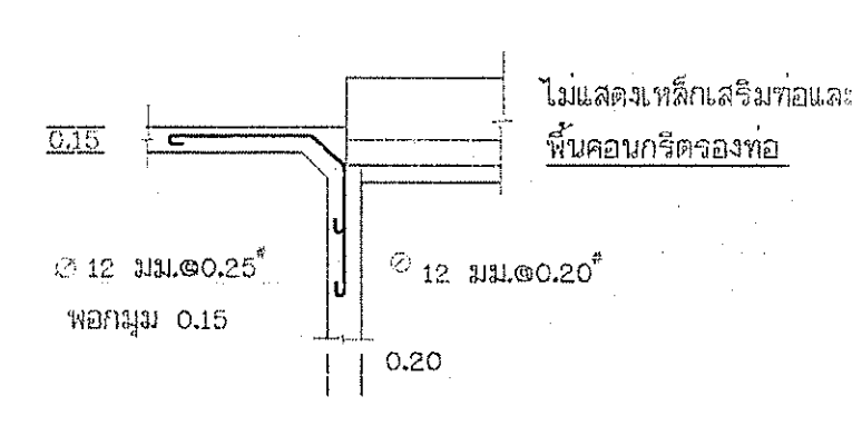
ขยาย ④ ไม่แสดงมาตราส่วน
