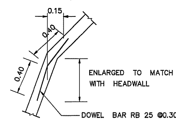
รายละเอียด ① NOT TO SCALE
