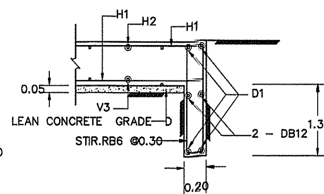
ຈາຍລະເວີຍດ ② NOT TO SCALE
