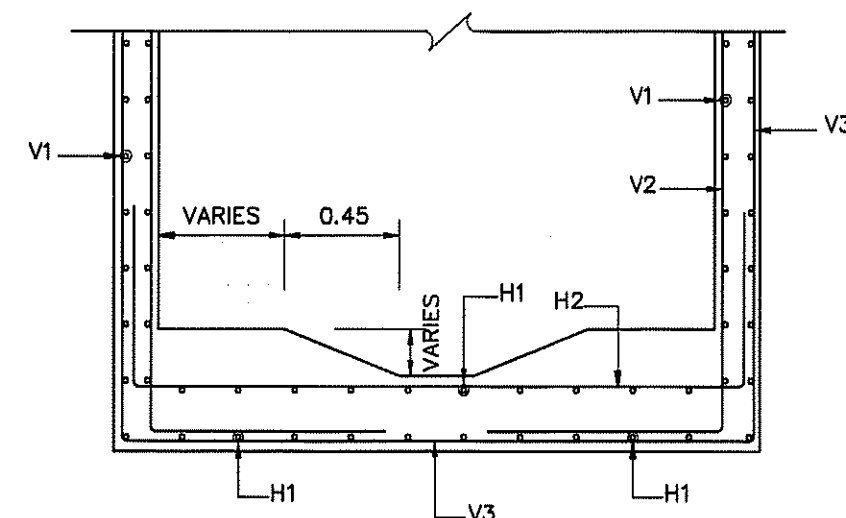
รูปตัด ๑๒ NOT TO SCALE
