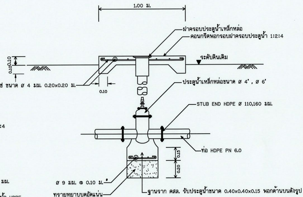
รูปตัด ค - ค แสดงการติดตั้งประติรูปใต้ดิน มาตราส่วน No Scale
