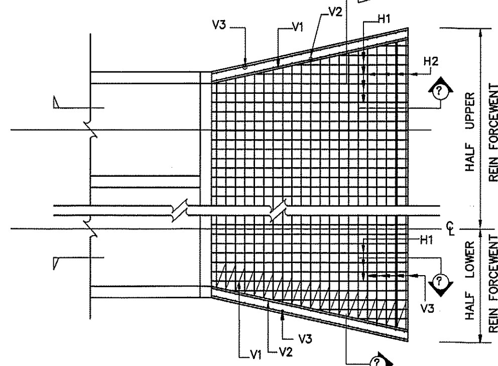
รายละเอียดสำหรับ MULTIPLE BOX
