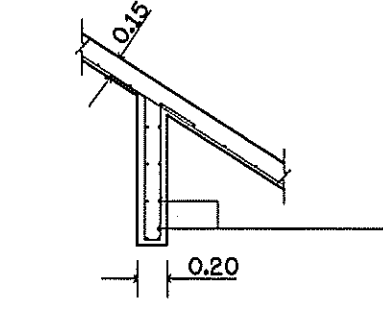
ขยาย CUT OFF ไม่แสดงมาตราส่วน
