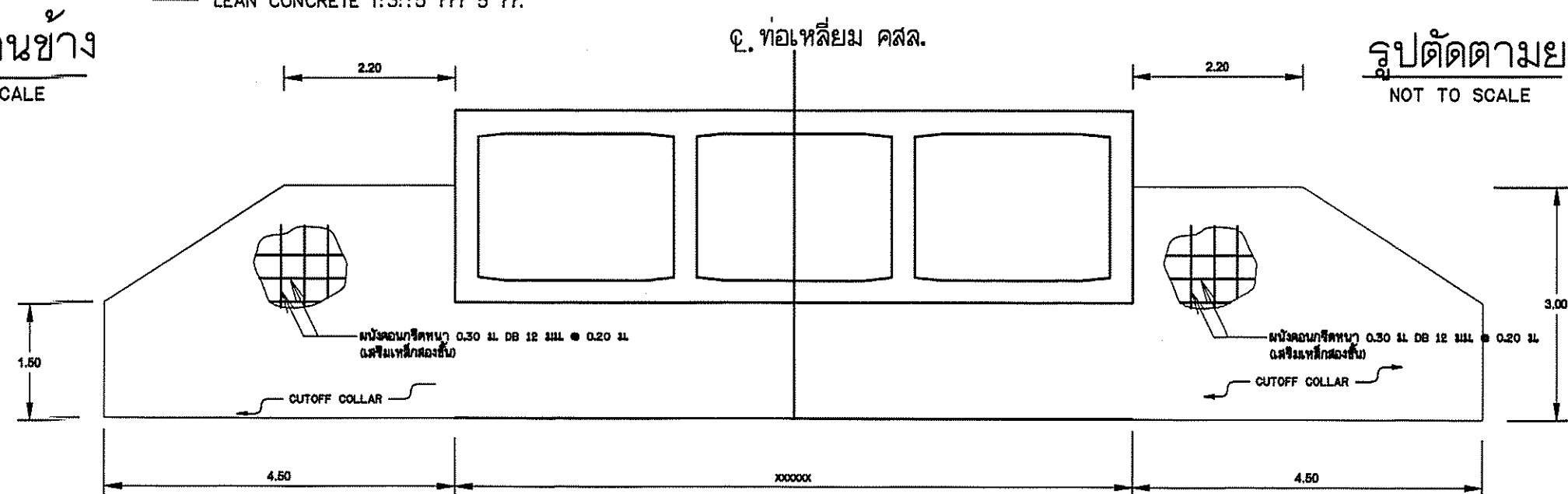
รูปตัดขยาย CUTOFF COLLAR
