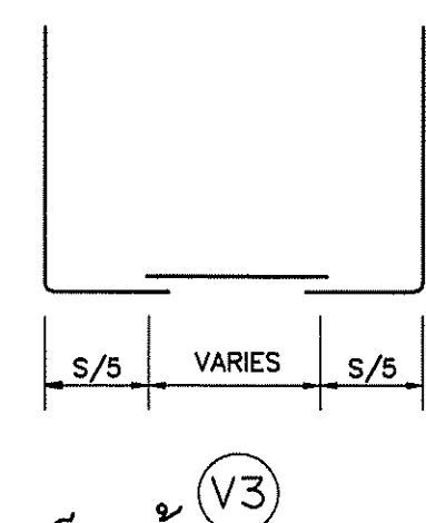
รายละเอียดหลักเส้น NOT TO SCALE
