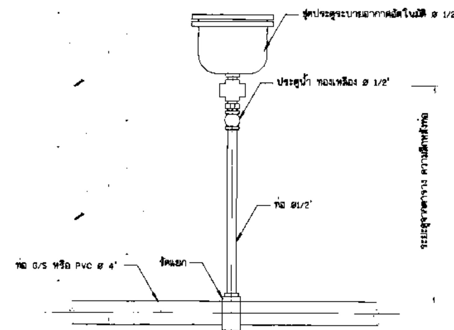
12. การติดตั้งประตูประบายอากาศอัตโนมัติ ไม่แสดงมาตราส่วน
