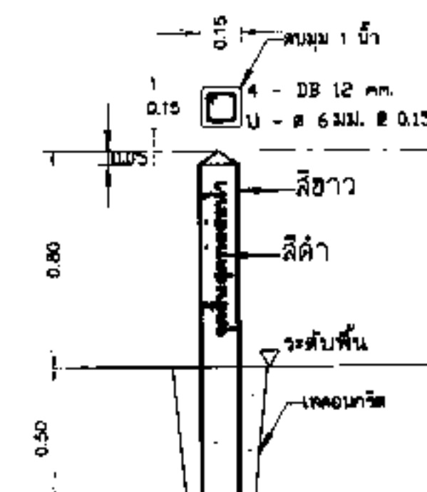
แบบขยายหลักสิ้นสุดท่อส่งน้ำ มาตราส่วน 1:20
