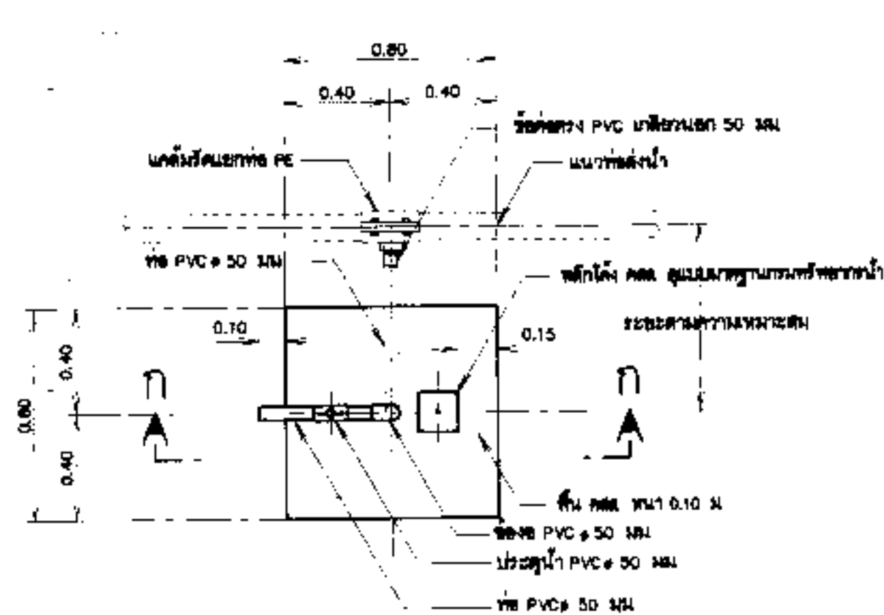
แปลนอาคารจุดปล่อยน้ำ มาตราส่วน 1:20
