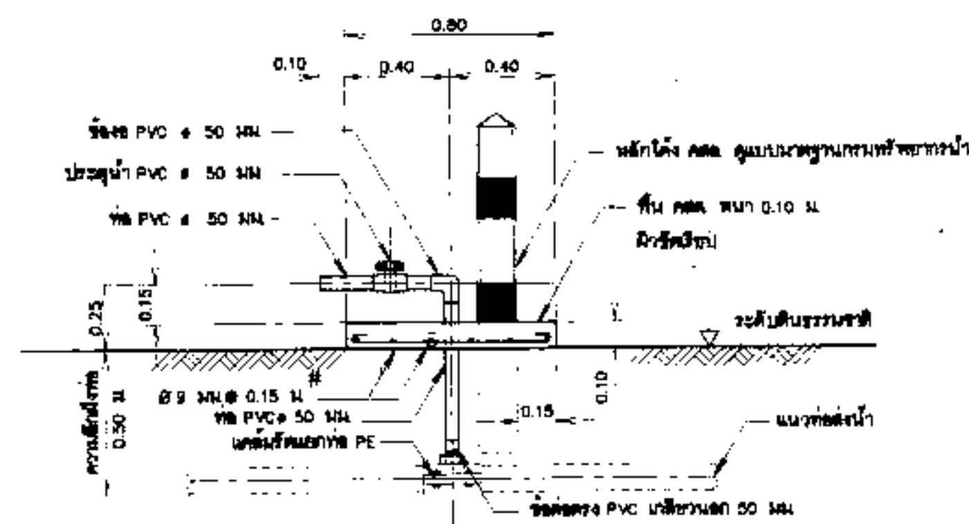
รูปตัด ก - ก แสดงการติดตั้งประจุดปล่อยน้ำ มาตราส่วน 1:20
