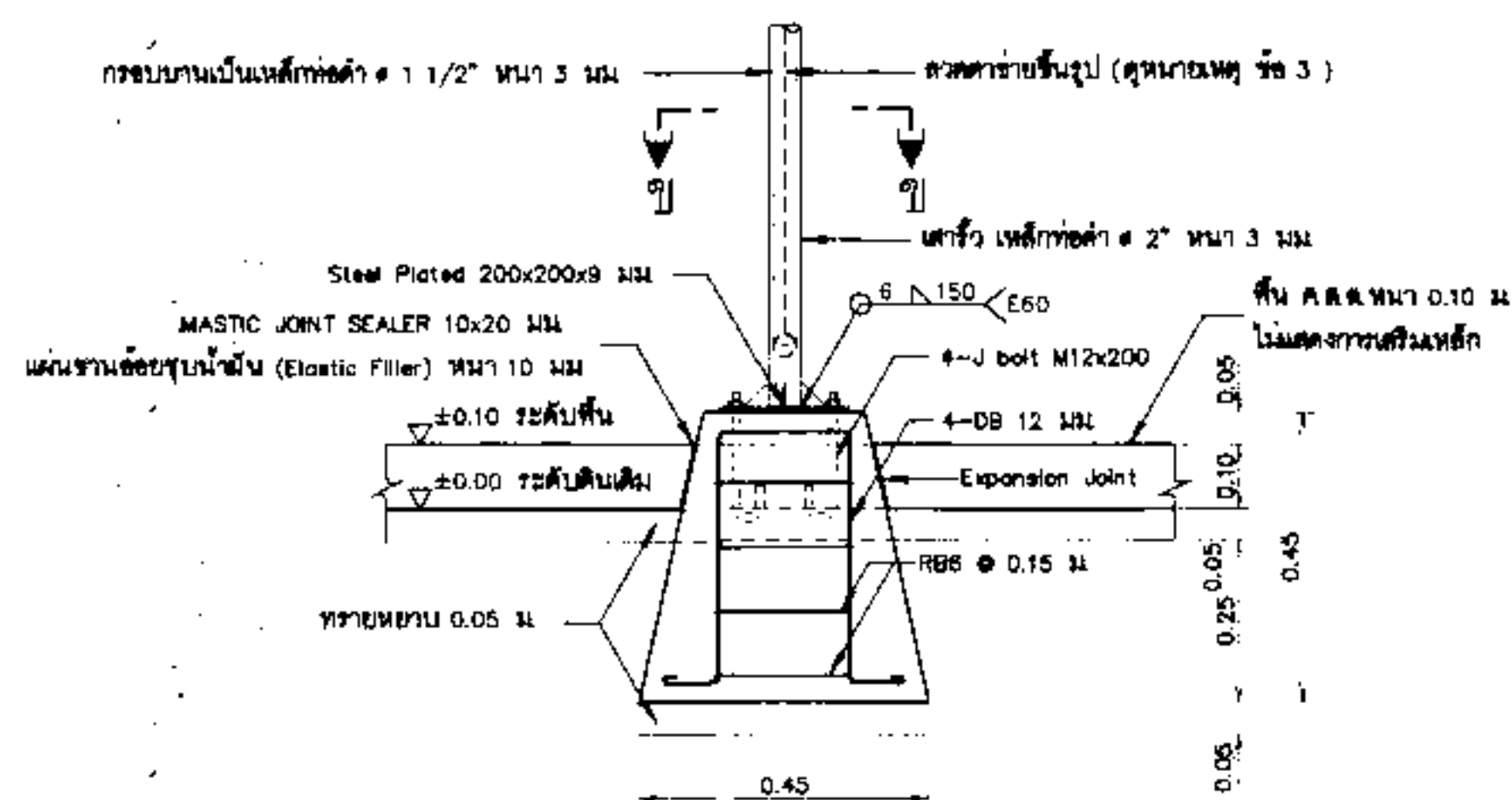
รูปขยายฐานรากโครงสร้างรับแรง F1 (กรณี คสล. ห่อด้วยปูนหรือฉาบฉวย) มาตราส่วน 1:10
