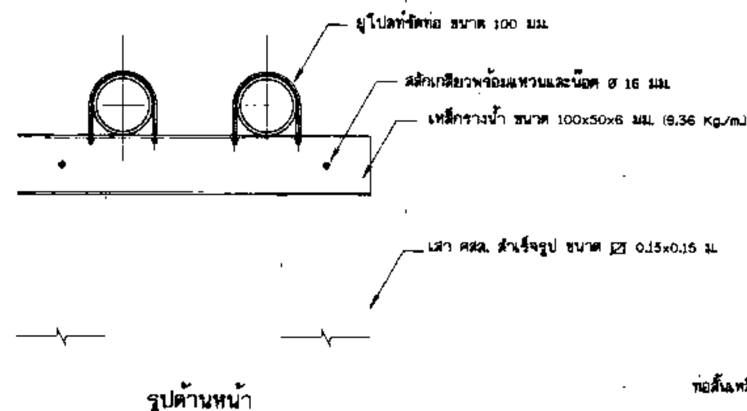
13. เสาคอมมูริบท่อชุด และแบบขยายอุปกรณ์วัดท่อ ไม่แสดงมาตราส่วน
