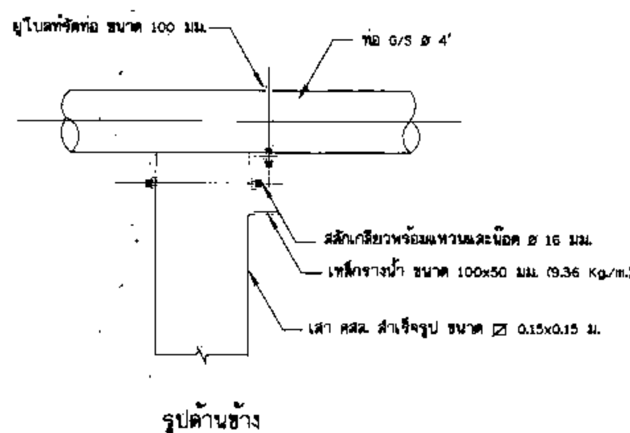
13. เสาคอมมูริบท่อชุด และแบบขยายอุปกรณ์วัดท่อ ไม่แสดงมาตราส่วน
