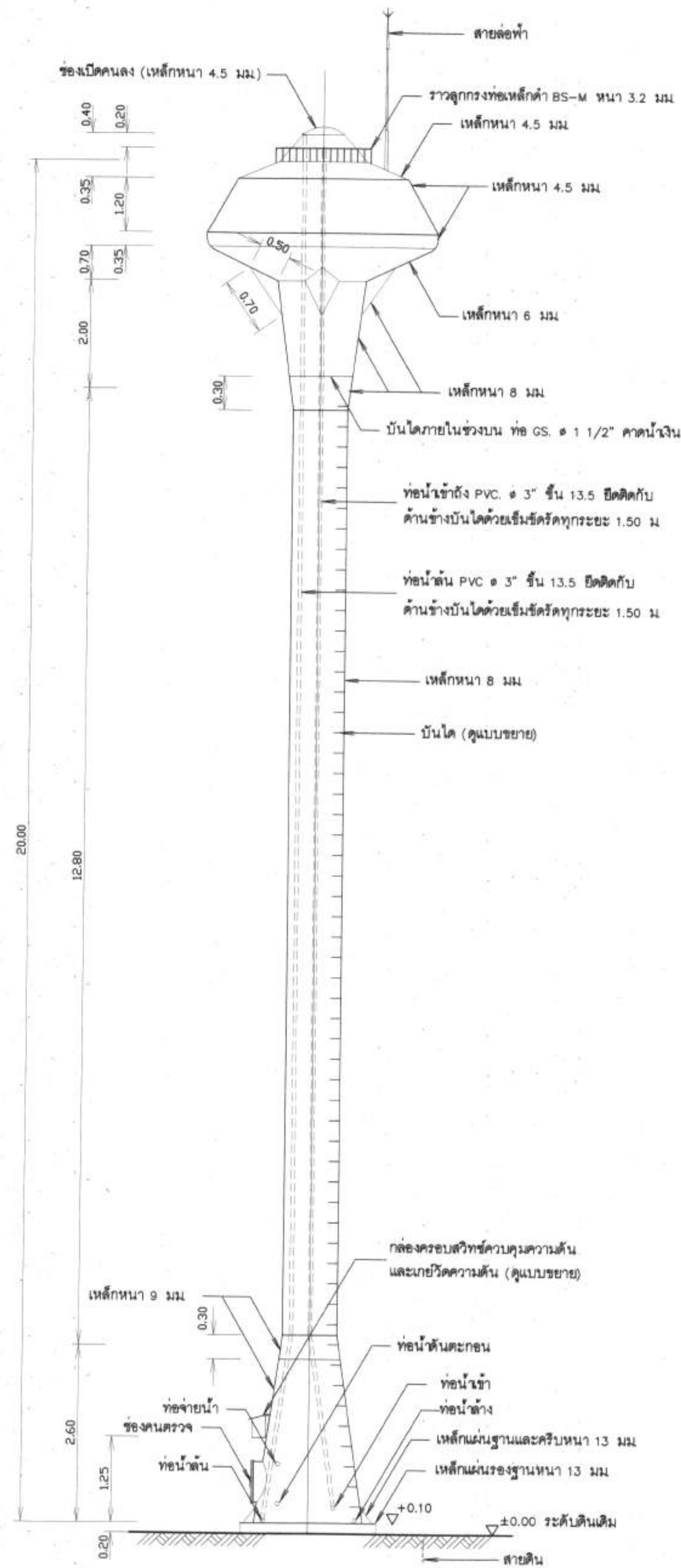
รูปด้านข้างหอดึงสูง แบบถังเหล็กทรงกลมแป้น
