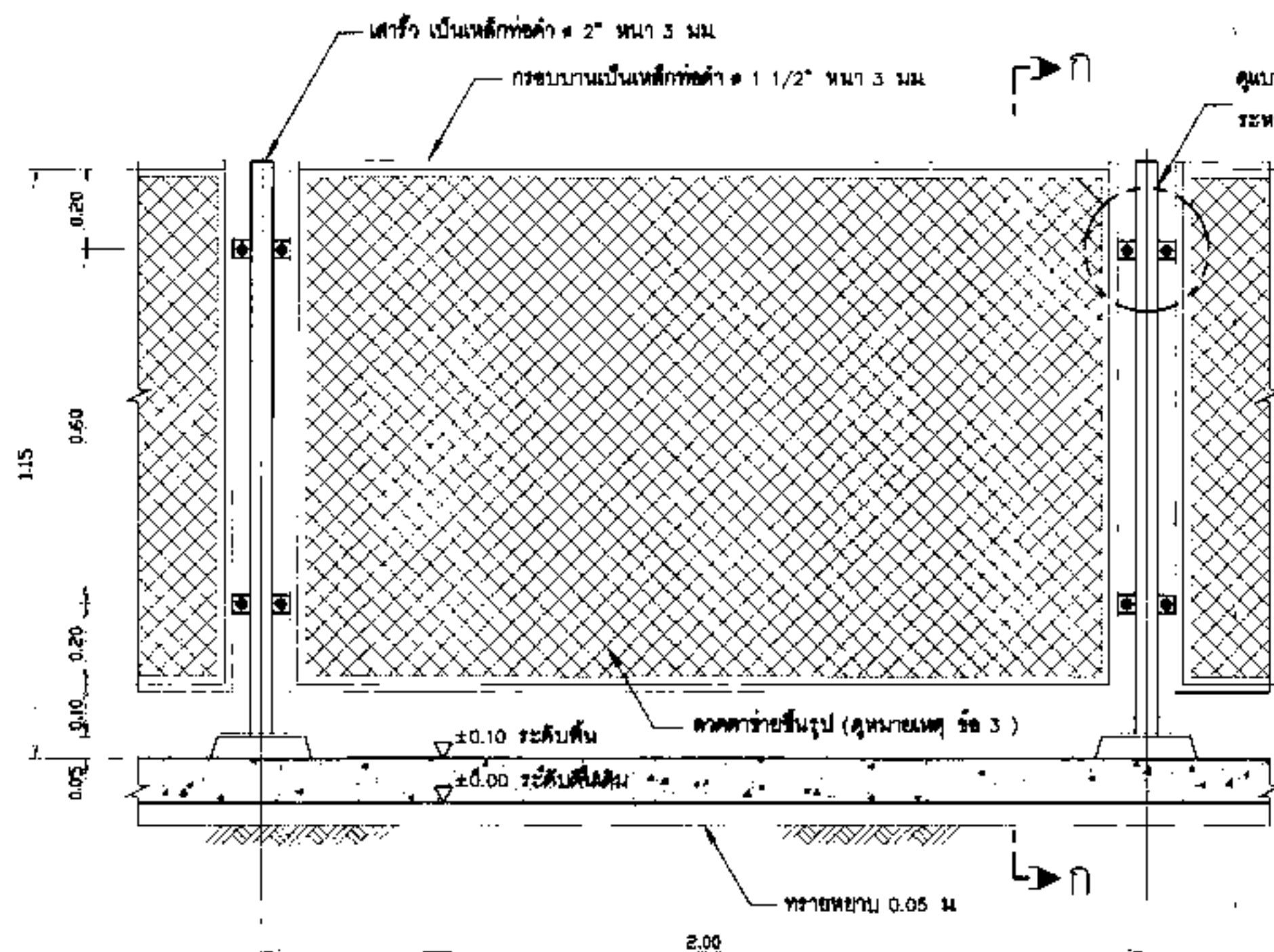
แบบขยายรื้อลดตายาย มาตราส่วน 1:10
