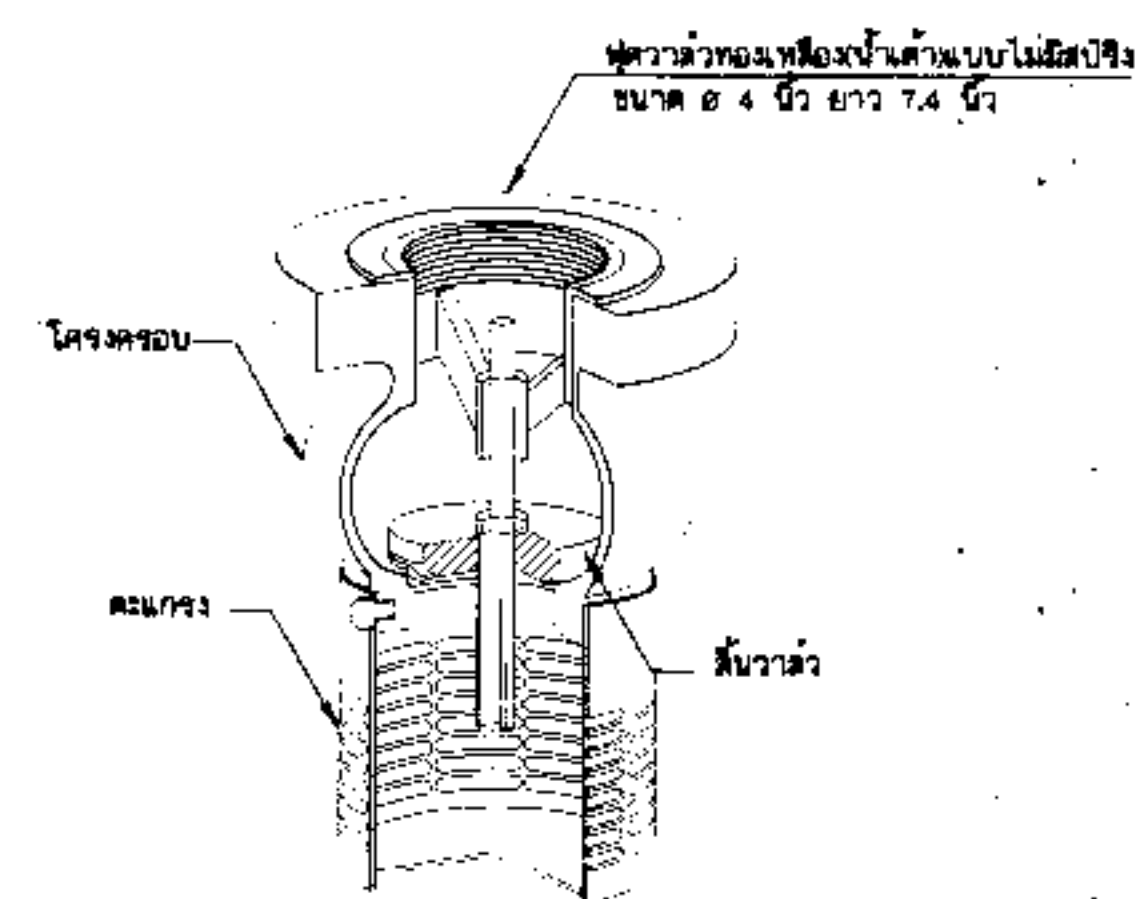
16. ชุดวาล์วของเครื่องปรับอากาศแบบไม่มีสปริง ไม่แสดงมาตราส่วน
