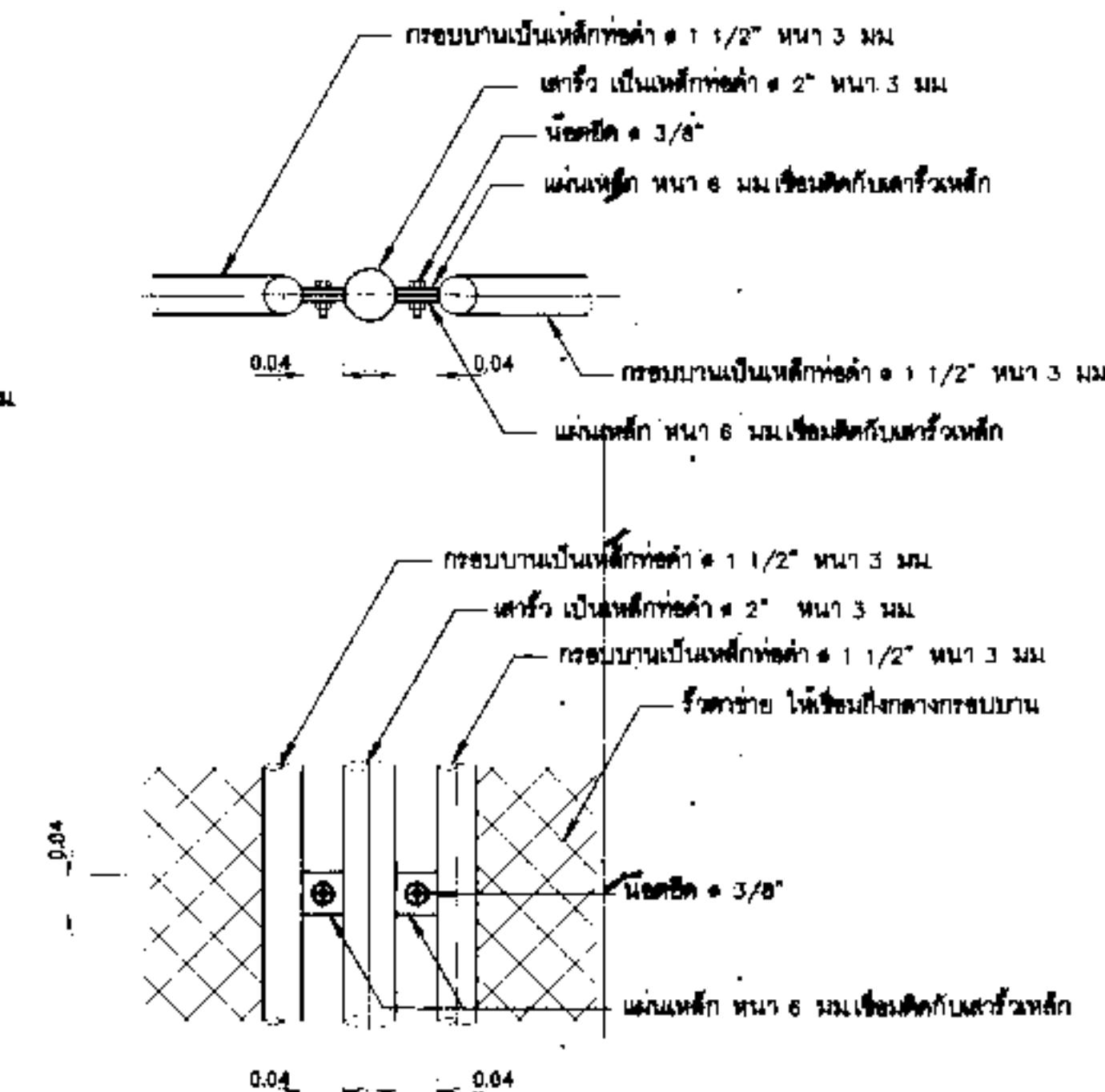
แบบขยายรายละเอียดแสดงการยึดระหว่างรื้อกับเสา มาตราส่วน 1:5
