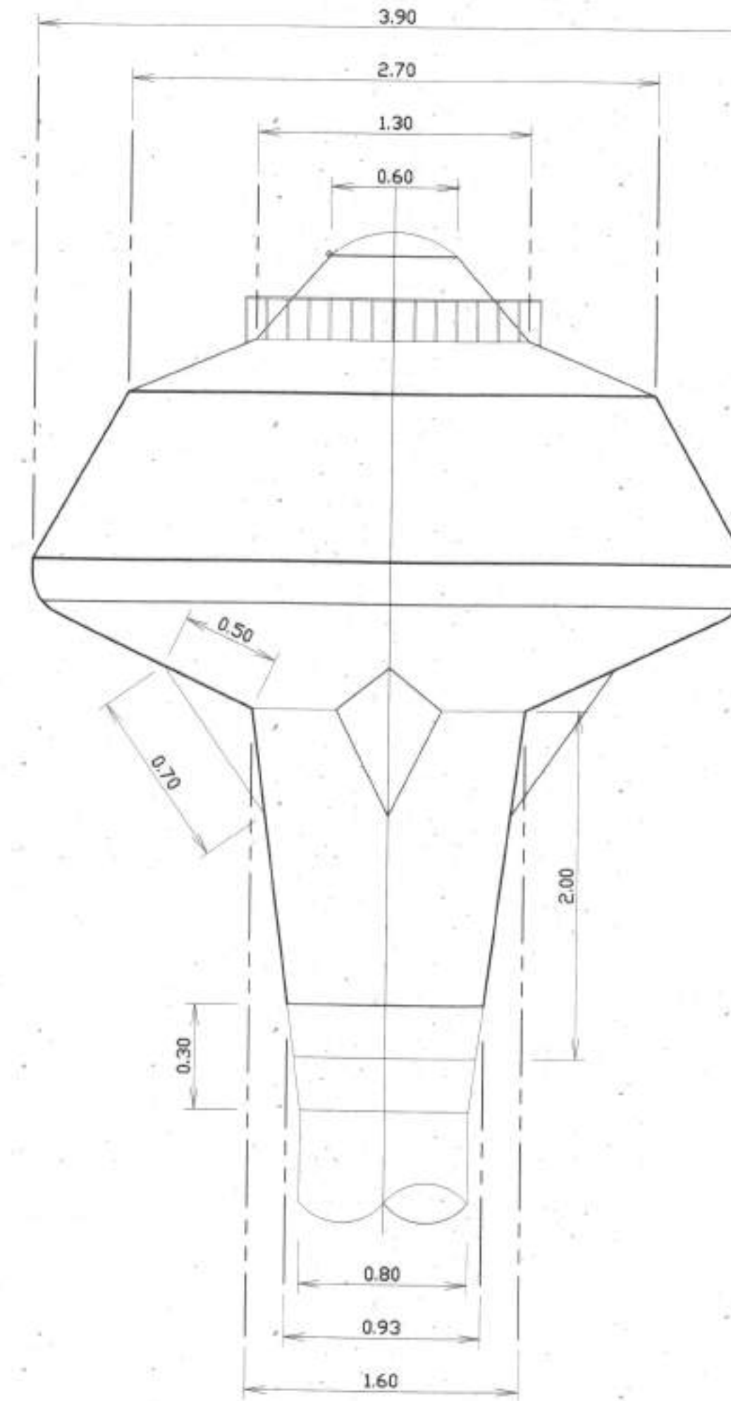
แบบขยายแมนโฮลบนหอดึงสูง
