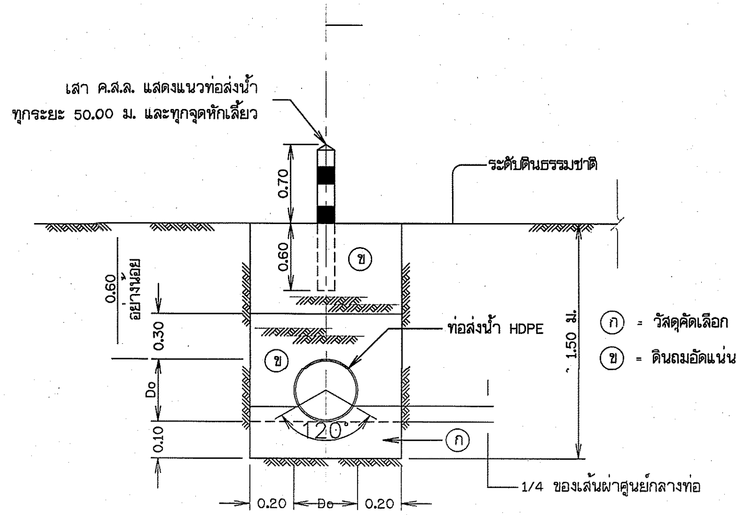
รูปตัดขวางการฝังท่อพีวี (ท่อHDPE)
