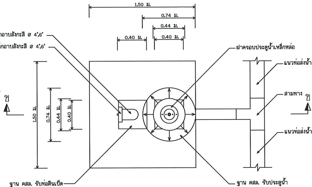
แปลนประติรูประบายตะกอน มาตราส่วน No Scale
