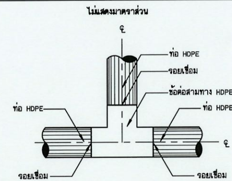
การบรรจุท่อสามทาง HDPE กับท่อ HDPE ไม่แสดงมาตรฐาน
