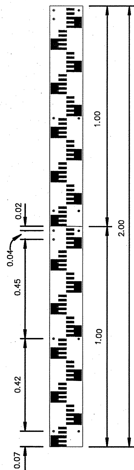
แผ่นเหล็กบอกระดับน้ำ
