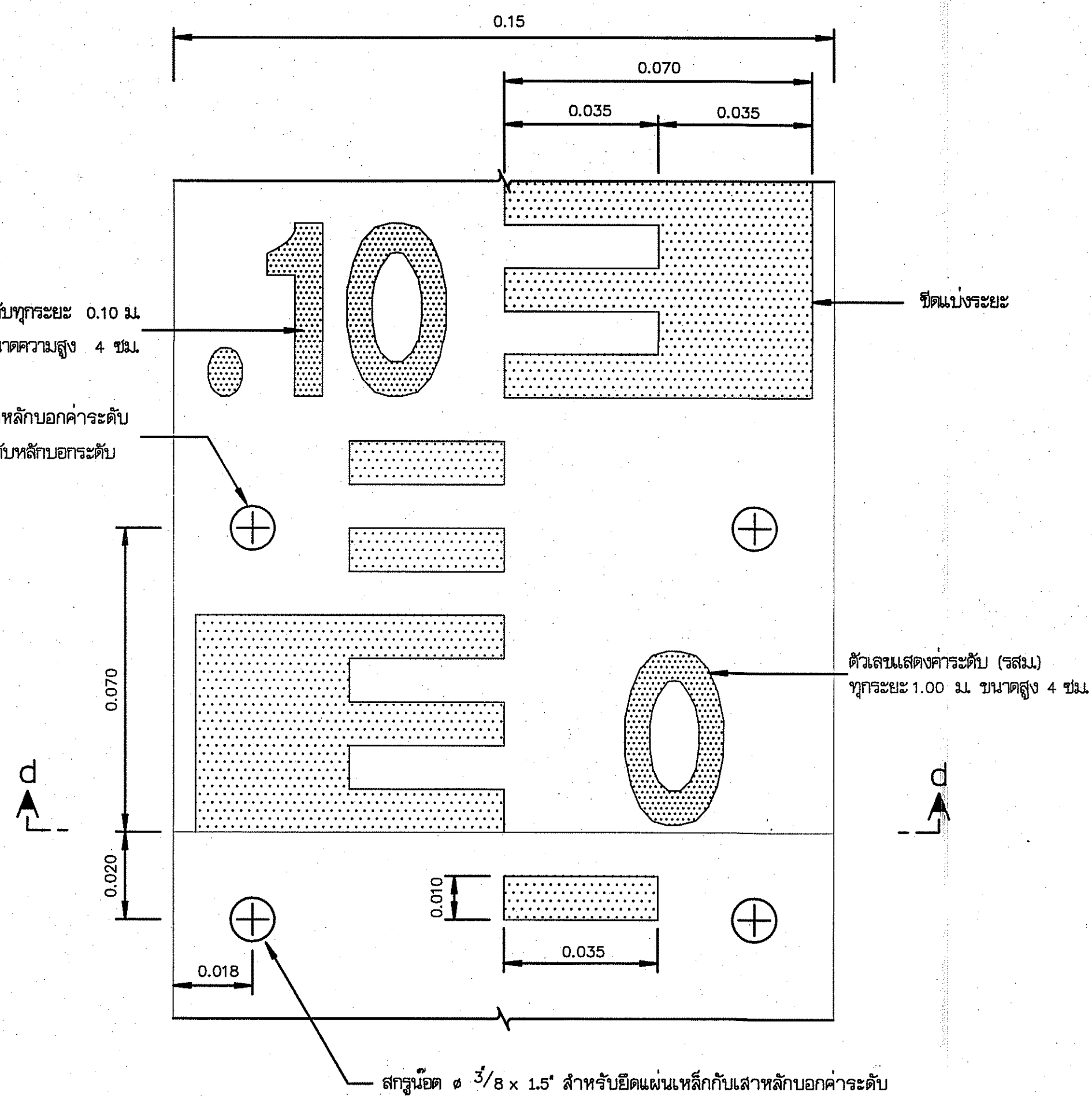
ขยายแผ่นเหล็กบอกระดับน้ำ
