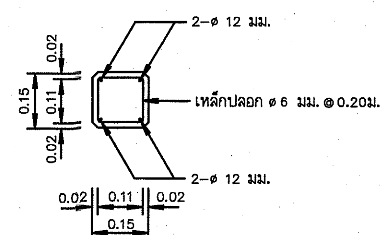
รูปตัด ข - ข มาตราส่วน 1:1
