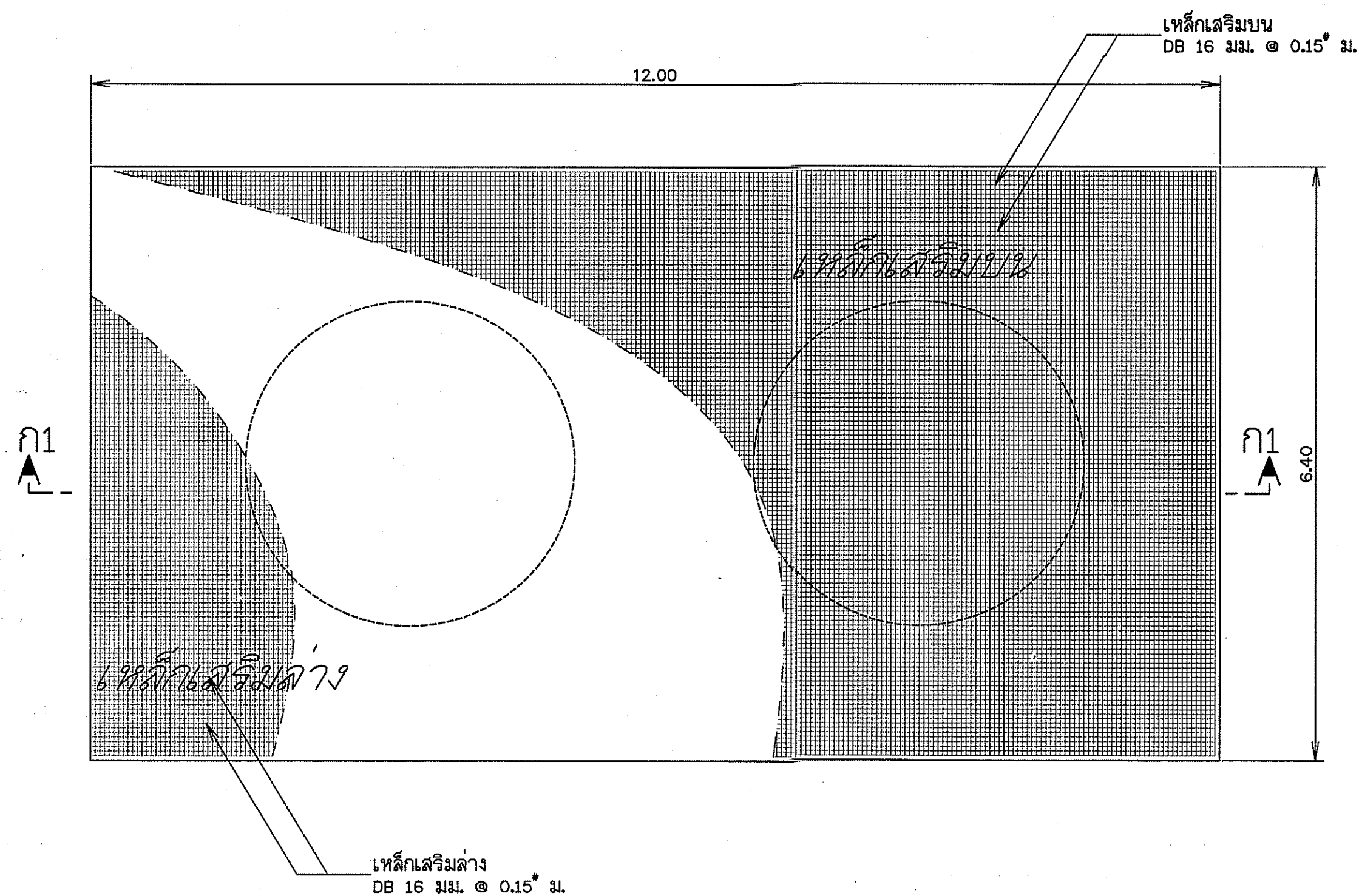
แปลนเสริมเหล็กพื้น
