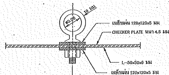
รูปขยายพ่วงยึดแผลสูบน้ำ
