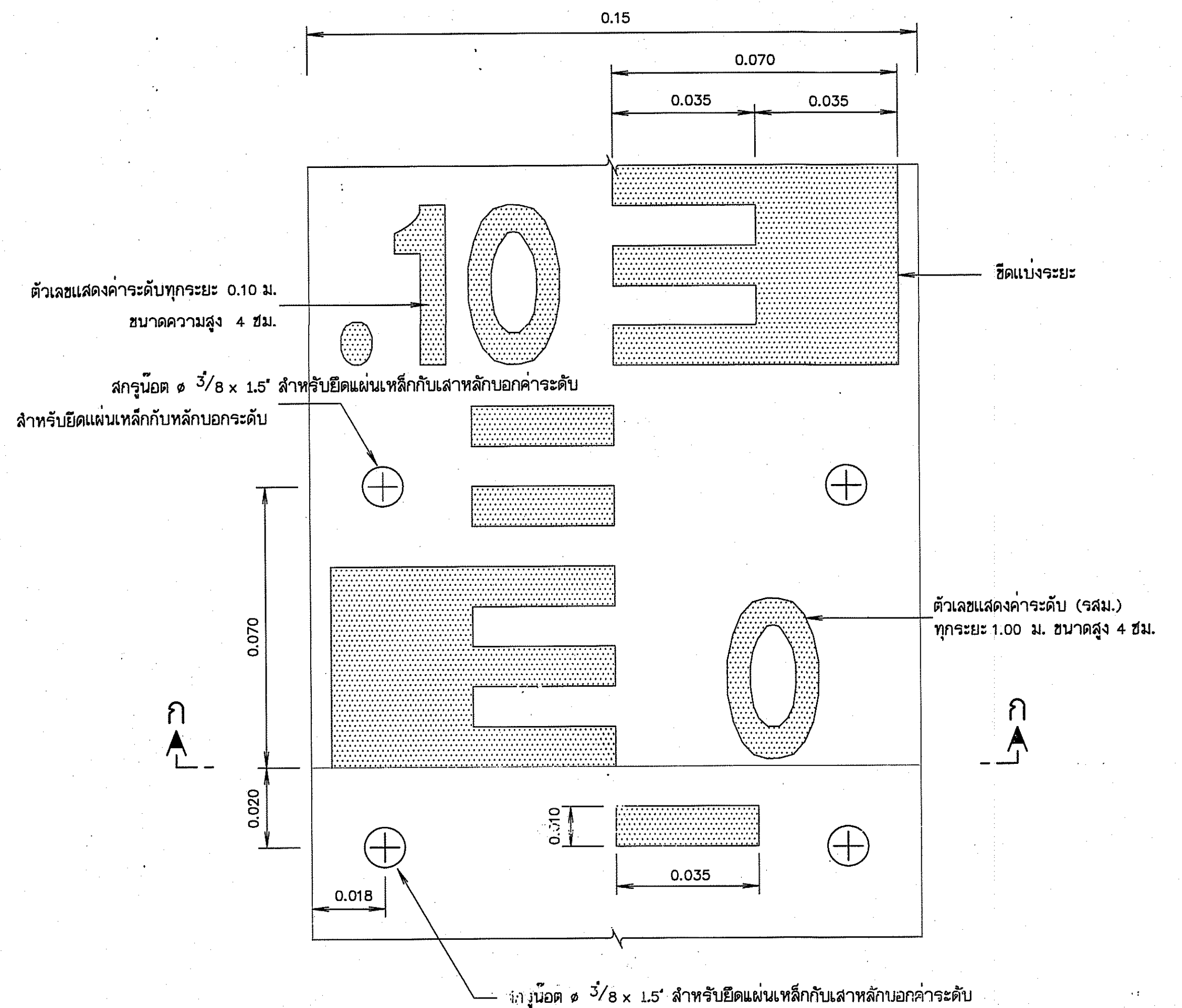
ขยายแผ่นเหล็กบอกระดับน้ำ
