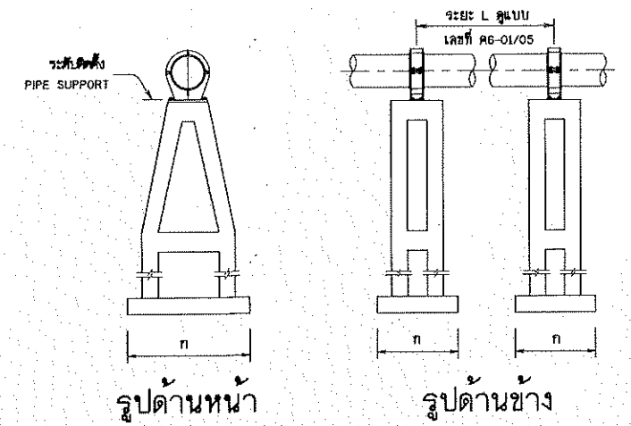
คอมมอรับทอแบบที่ 3,4
