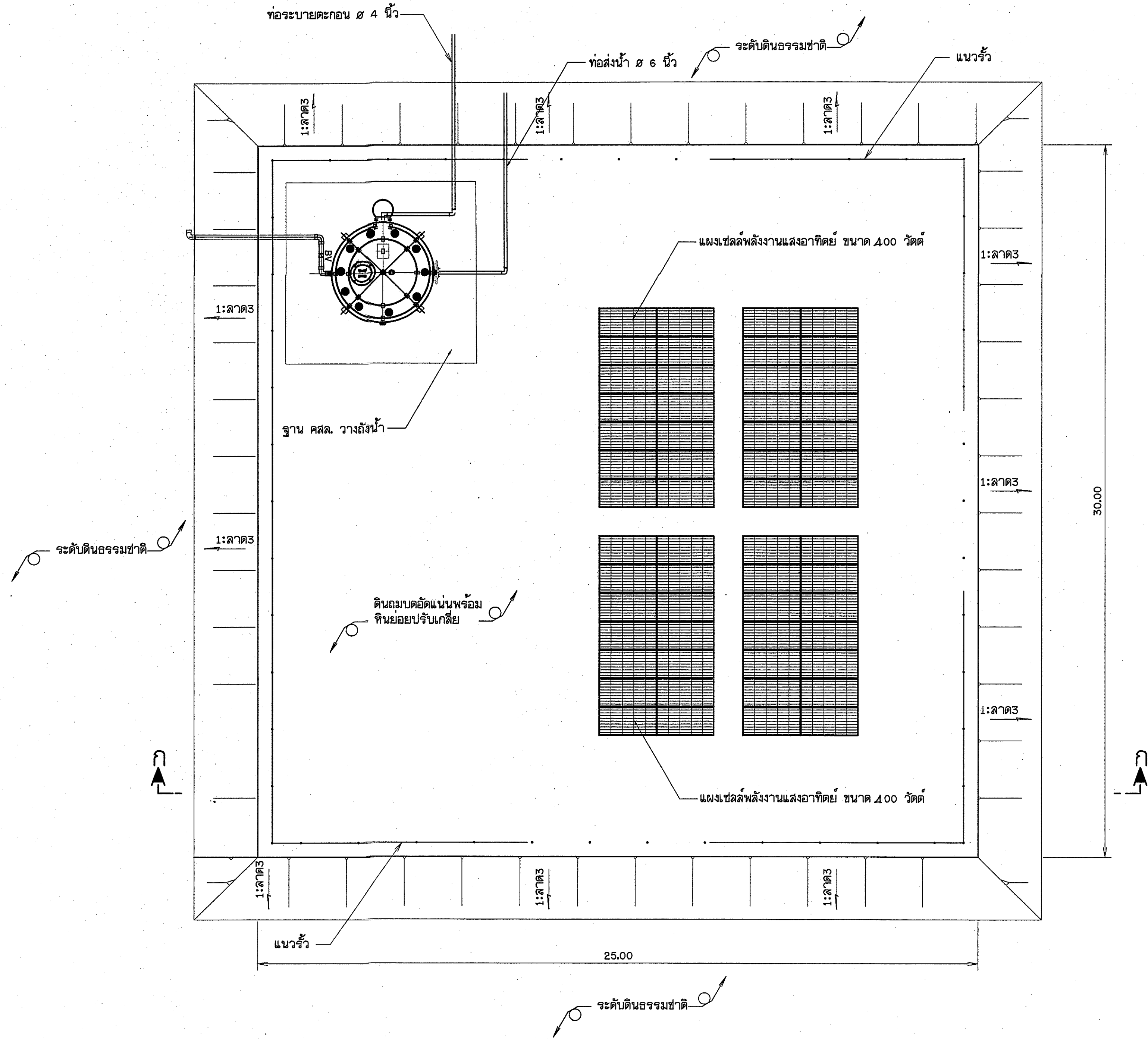
แปลนทั่วไป มาตราส่วน ไม่แสดงมาตราส่วน
