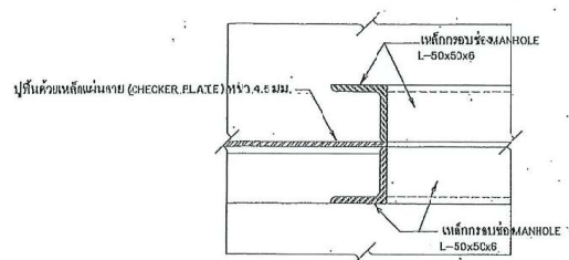
รูปขยาย 1
