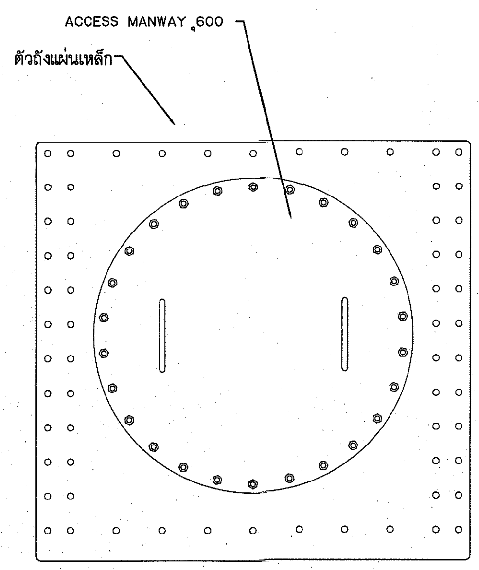
แบบขยาย 5รูปแบบประกอบหน้าแปลน Scale NTC.
