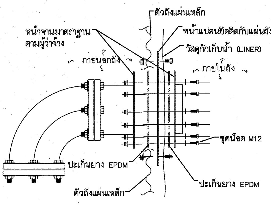
แบบขยาย 5รูปแบบประกอบหน้าแปลน Scale NTC.
