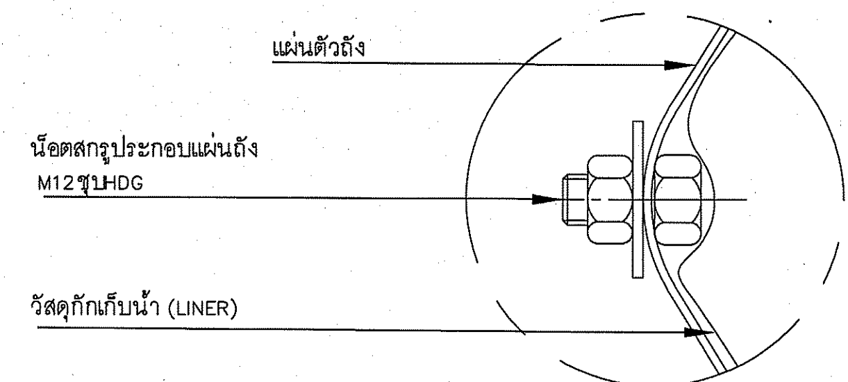
แบบขยาย 9-รูปแบบการประกอบแผ่นถัง Scale NTC.
