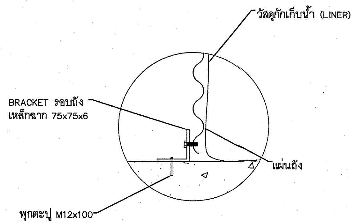
แบบขยาย 11-ติดตั้งผนังกับฐานราก Scale NTC.
