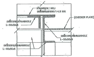
รูปขยาย 2
