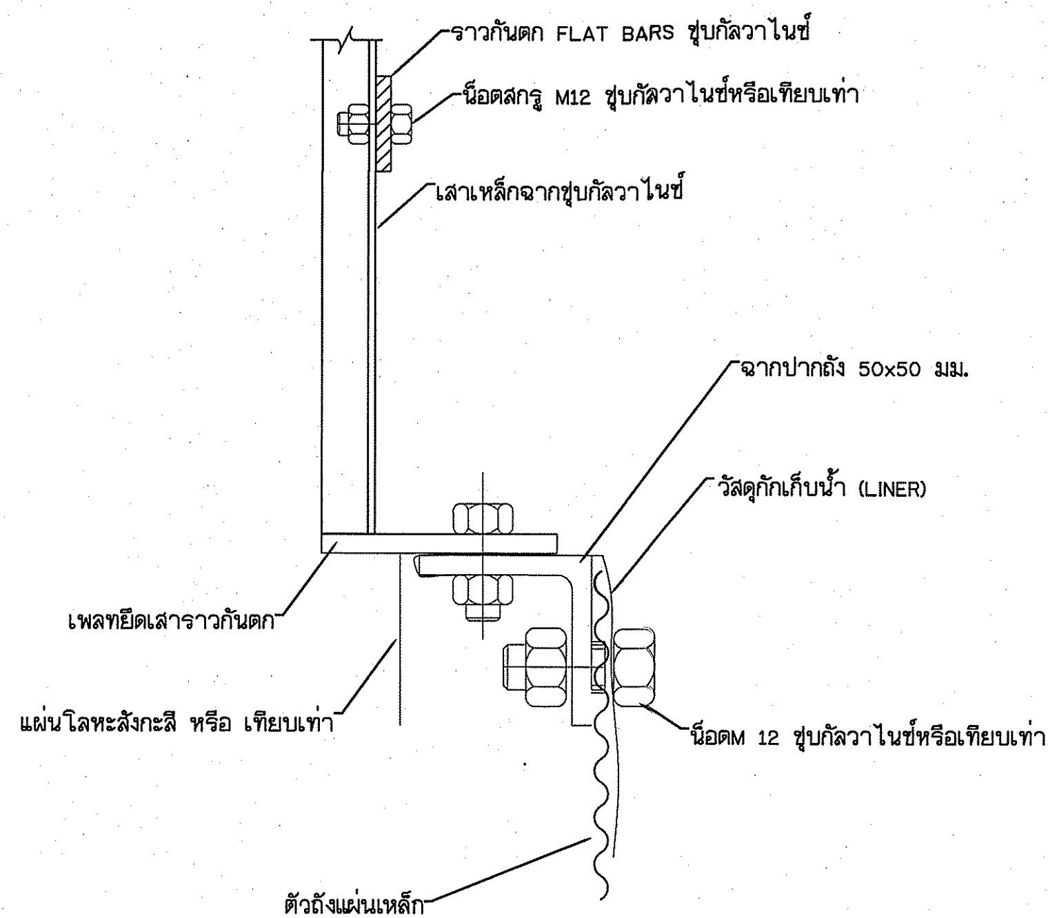
แบบขยาย 8 Scale NTC.
