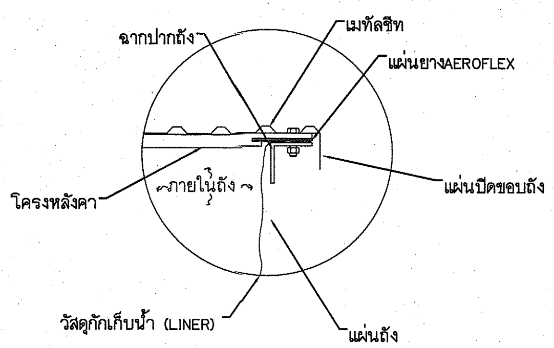
แบบขยาย 3จุดยึดหลังคาถังกับแผ่นถัง Scale NTC.
