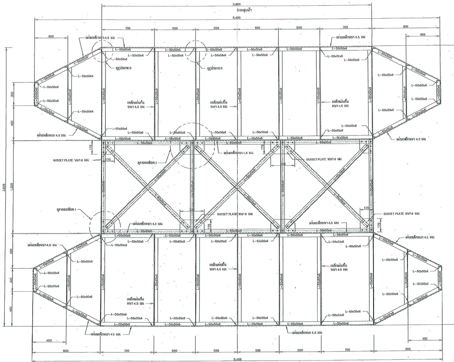
รูปตัด ก-ก ขนาดส่วน 1 : 10
