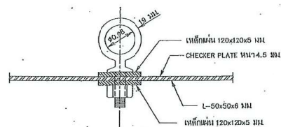
รูปขยายห้วงยึดแป้นสูบน้ำ
