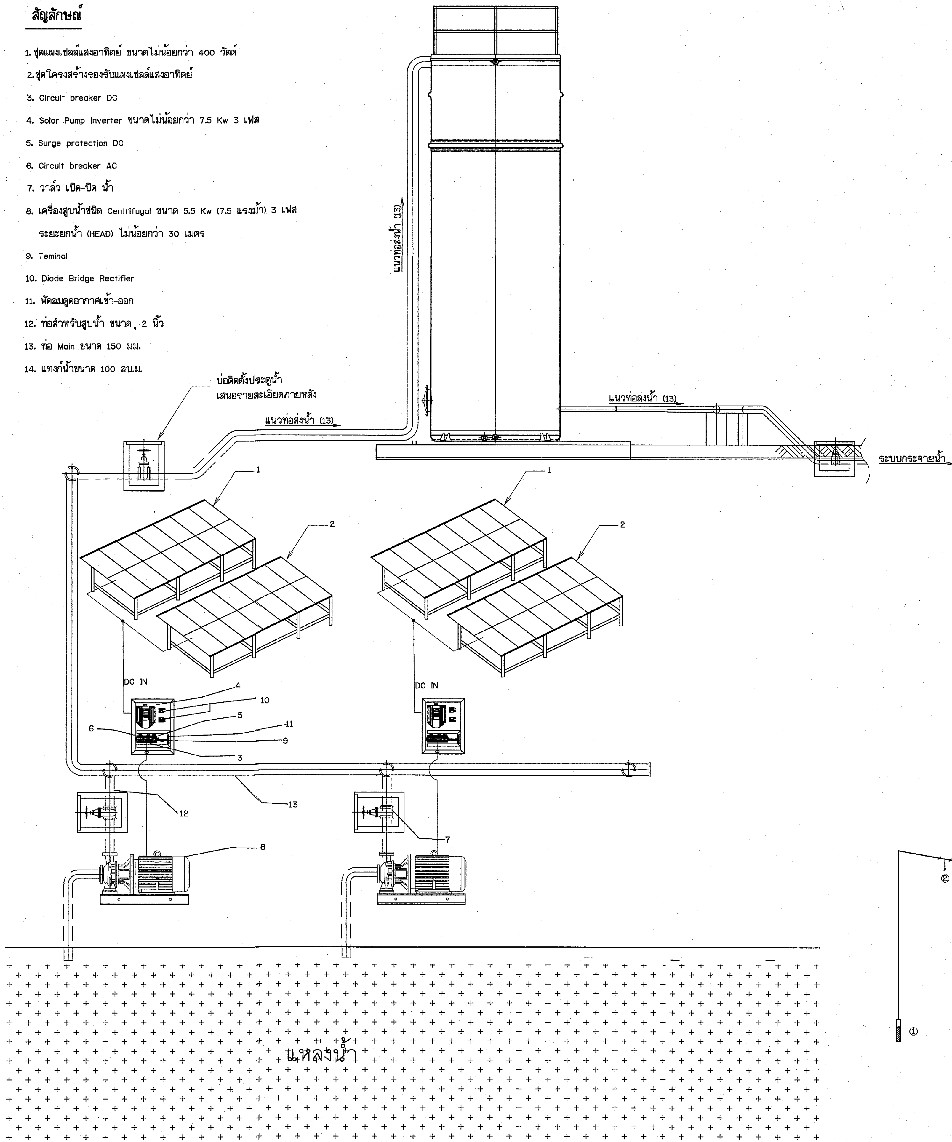
แบบระบบกระจายน้ำด้วยพลังงานแสงอาทิตย์ มาตราส่วน ไม่แสดงมาตราส่วน
