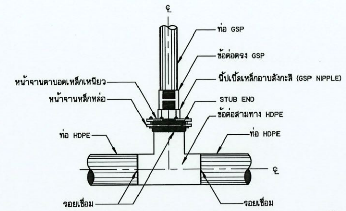
การบรรจุท่อสามทาง HDPE กับท่อ GSP แบบข้อต่อ (สำหรับอาคารจุดปล่อยน้ำ อาคารประจักษ์ประยาตตะกอน อาคารท่อระบายอากาศ กรณีที่ท่อส่งน้ำขนาดเส้นผ่านศูนย์กลางมากกว่า 315 มม.)
