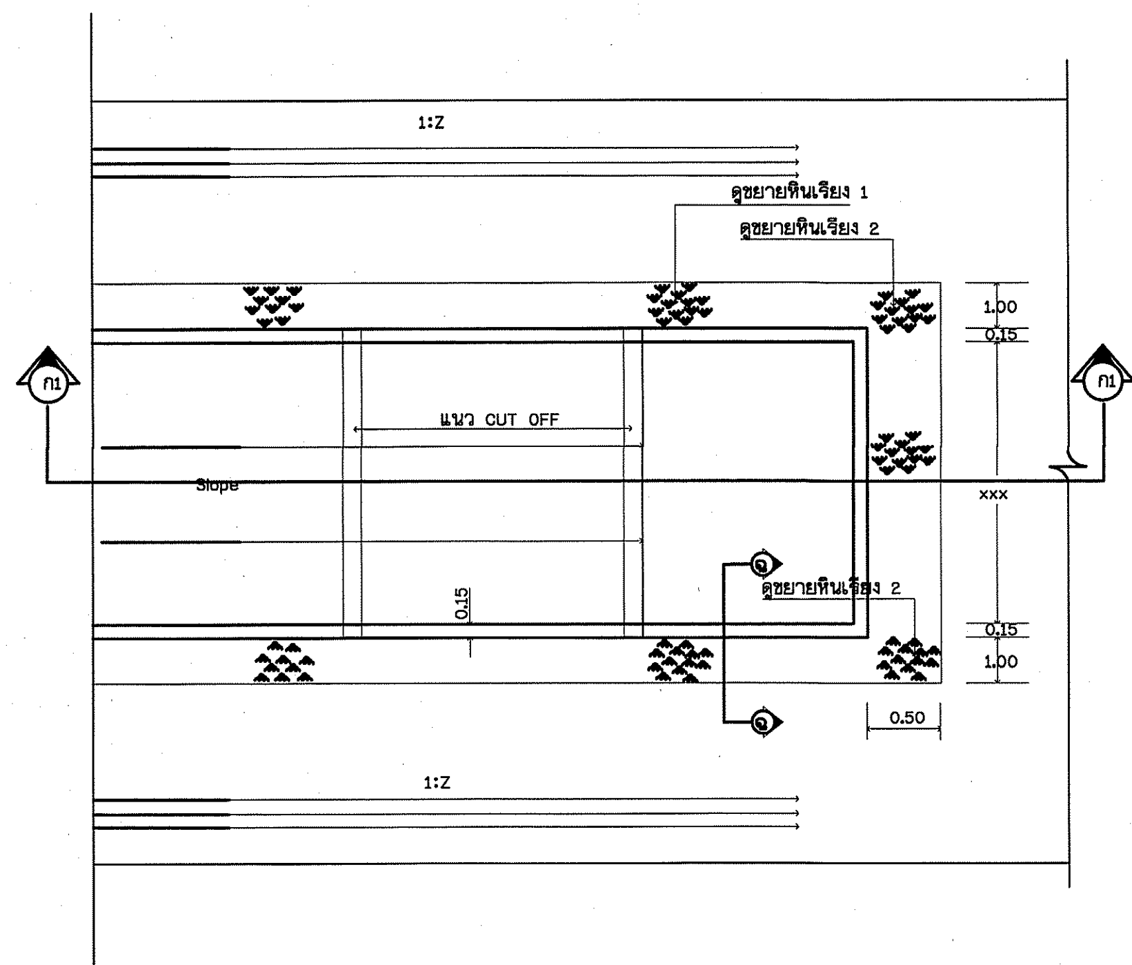
แปลนอาคารราง Chute (กรณีไม่มีชันพัก) ไม่แสดงมาตราส่วน
