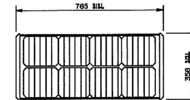
แผงเซลล์แสงอาทิตย์เสาไฟ
