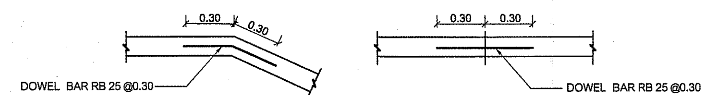
รายละเอียด 1 ไม่แสดงมาตราส่วน
