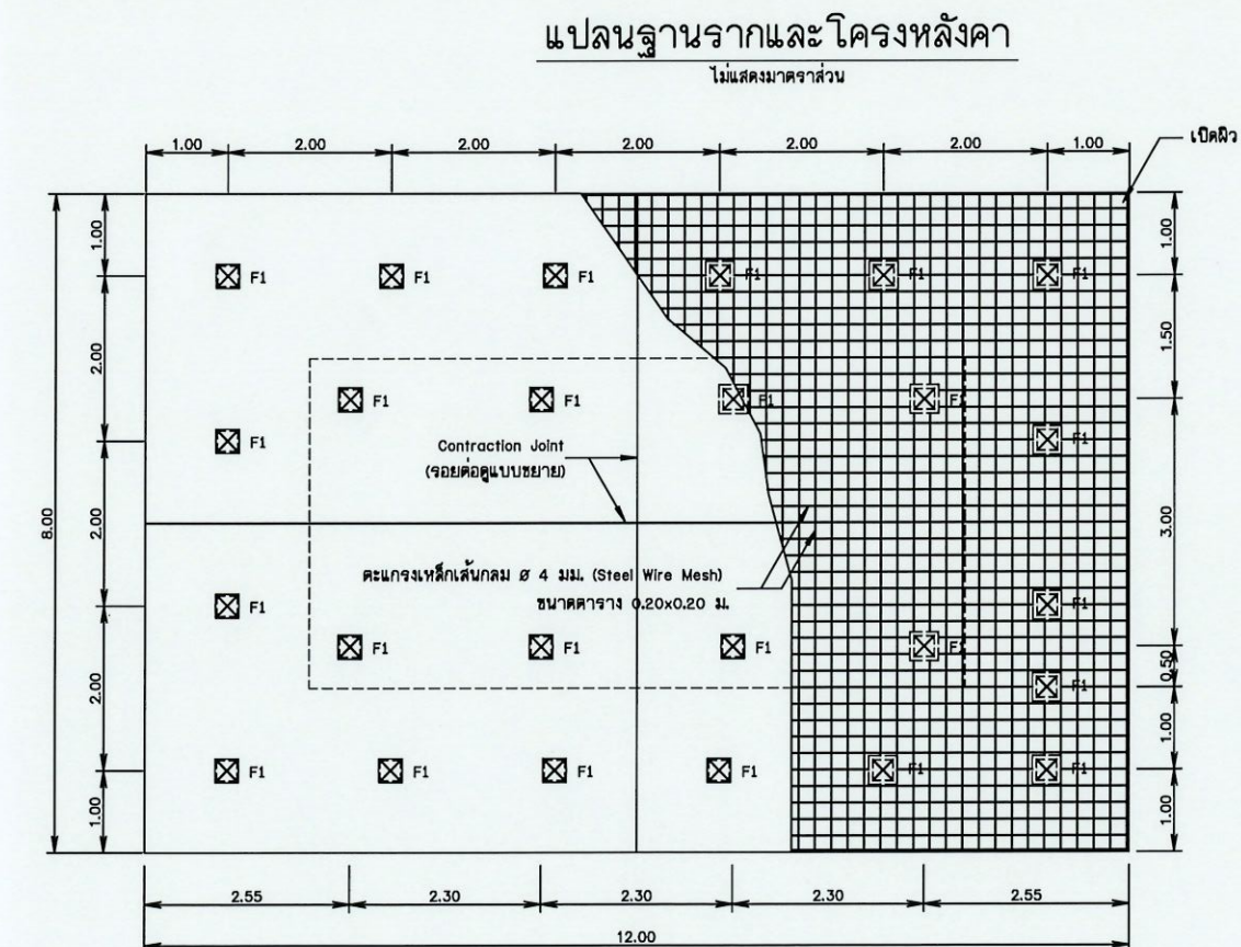
รูปขยายพื้นคอนกรีต ไม่แสดงมาตราส่วน
