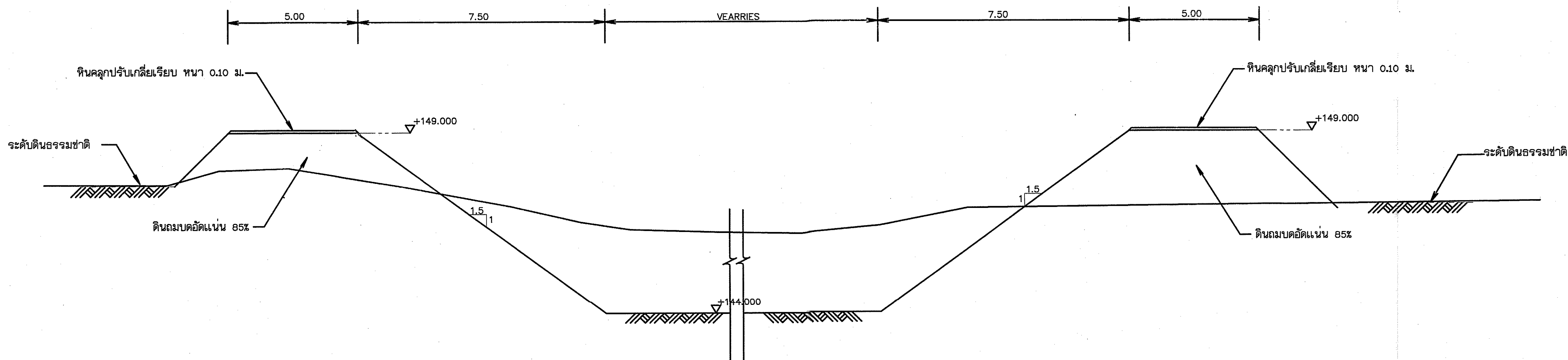
รูปตัดทั่วไป
