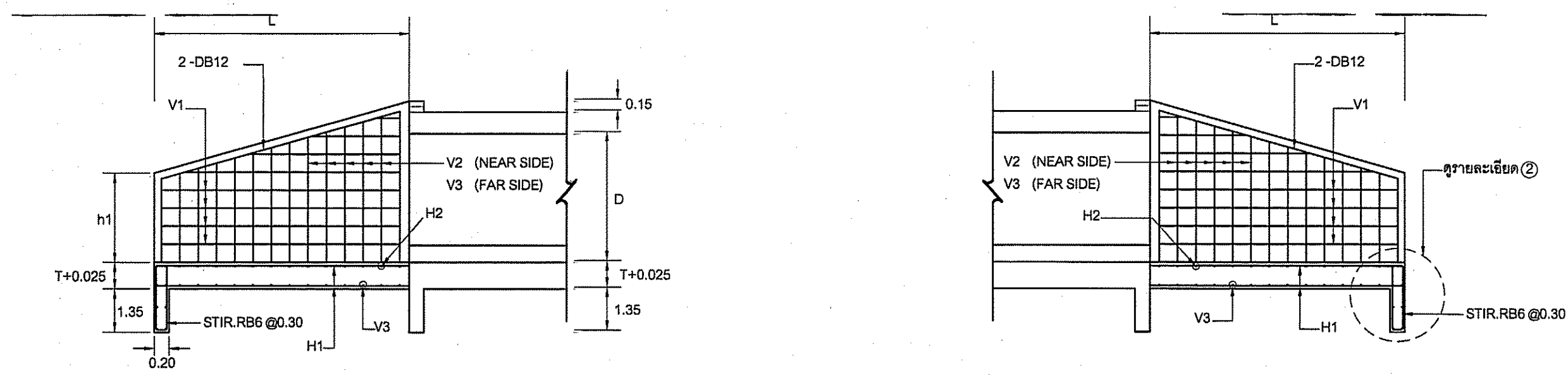
รูปตัด ① NOT TO SCALE
