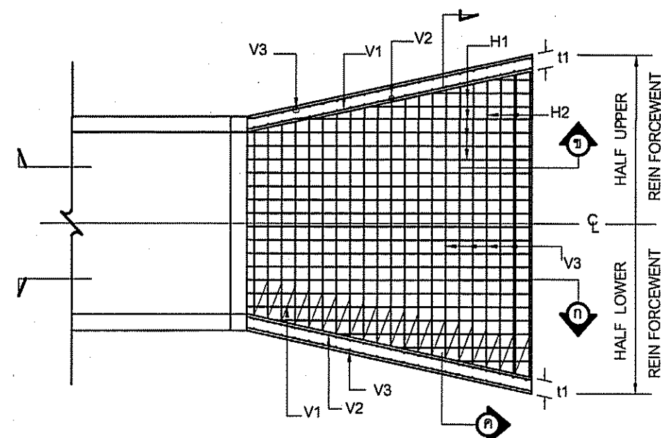
รูปตัด ② NOT TO SCALE
