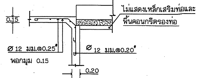
ขยาย (ง) ไม่แสดงมาตราส่วน
