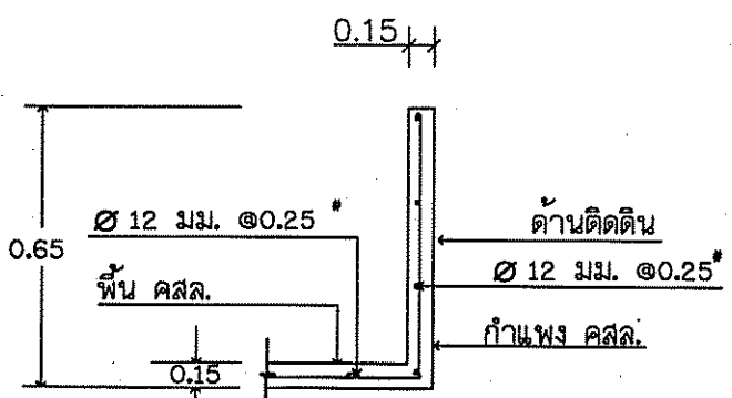
รูปตัด (ข) - (ข) (ความหนา 0.15 ม.) ไม่แสดงมาตราส่วน
