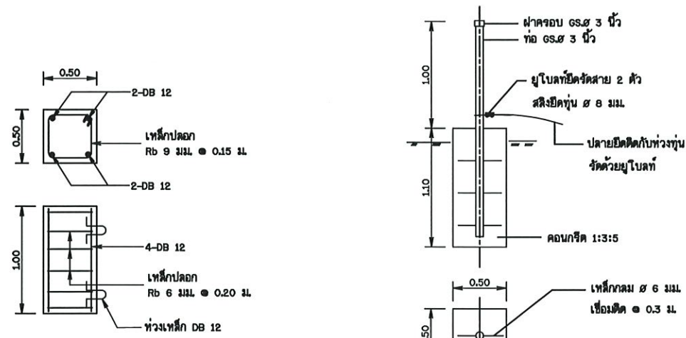
รูปขยายทึบ คสล. ยึดแพ มาตราส่วน 1:50
