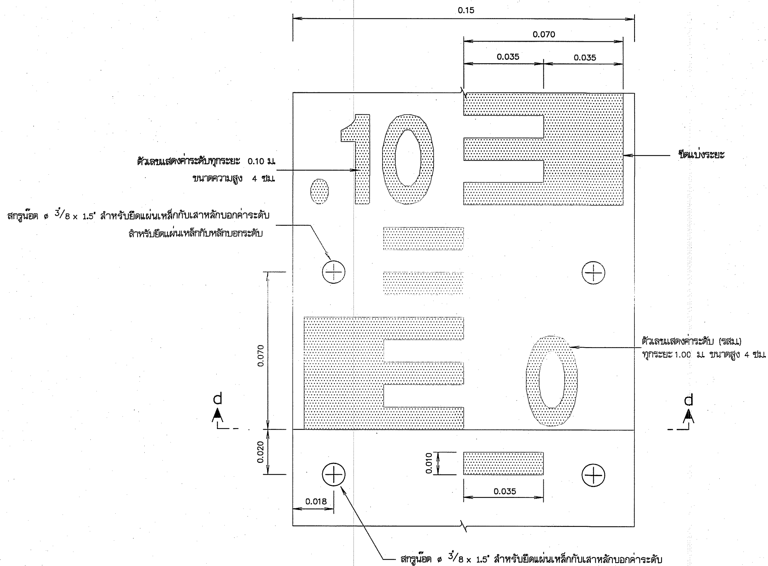
ขยายแผ่นหลักบอการค้าระดับน้ำ
