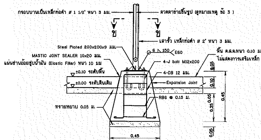
รูปขยายฐานจากโครงสร้างรับแผง F1 (คอมมู คสล. หล่อค้ำรูปหรือมอดิตัง) ไม่แสดงขนาดจั่ว
