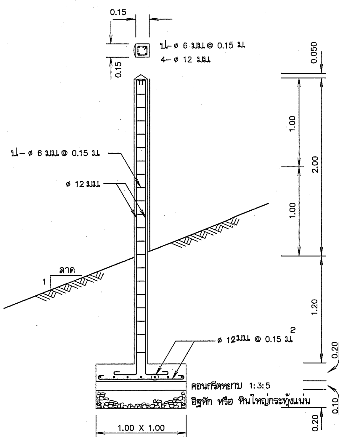
ขยายหลัก คสล.บอการค้าระดับน้ำ
