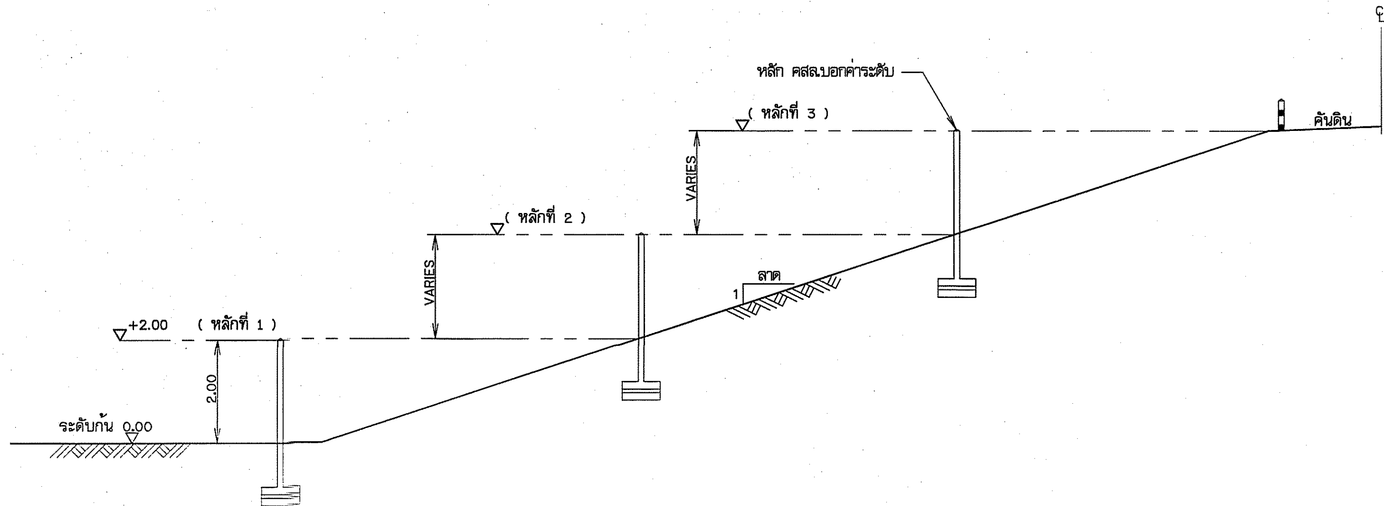
รูปตัดจั่ว ไปแสดงตำแหน่งหลักบอการค้าระดับน้ำ
