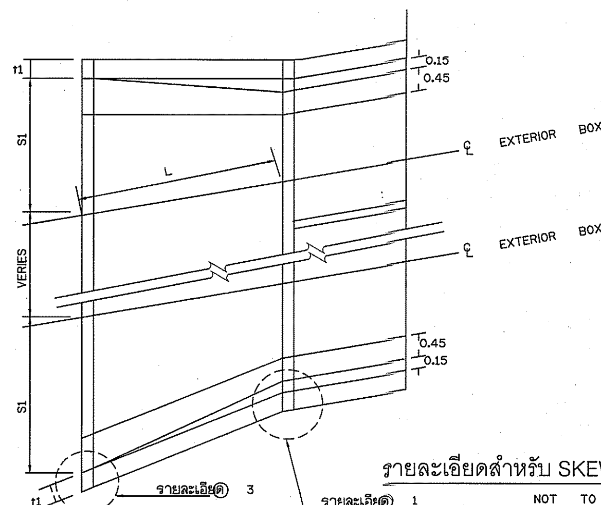
รายละเอียดสำหรับ SKEW SINGLE BOX
