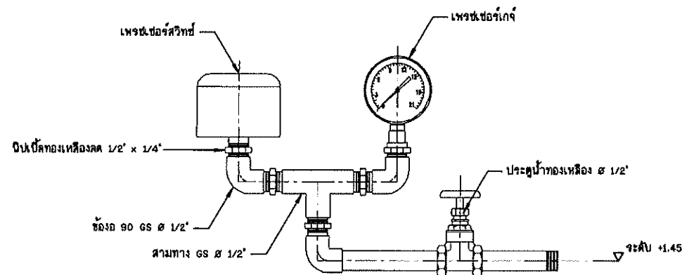
แบบขยายสวิตช์ควบคุมและเกจวัดความดัน ไม่แสดงขนาดจั่วส่วน
