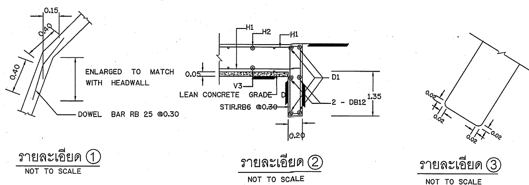
รายละเอียดหลักเส้น NOT TO SCALE
