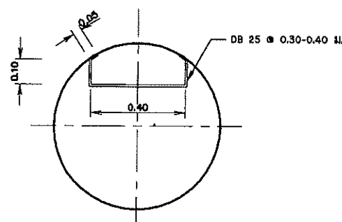
รูปขยายบันไดภายในส่วน column ไม่แสดงขนาดจั่วส่วน
