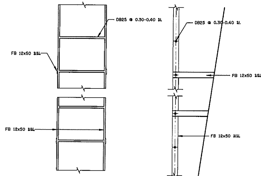
แบบขยายบันได ภายในท่อถึงสูง ไม่แสดงขนาดจั่วส่วน
