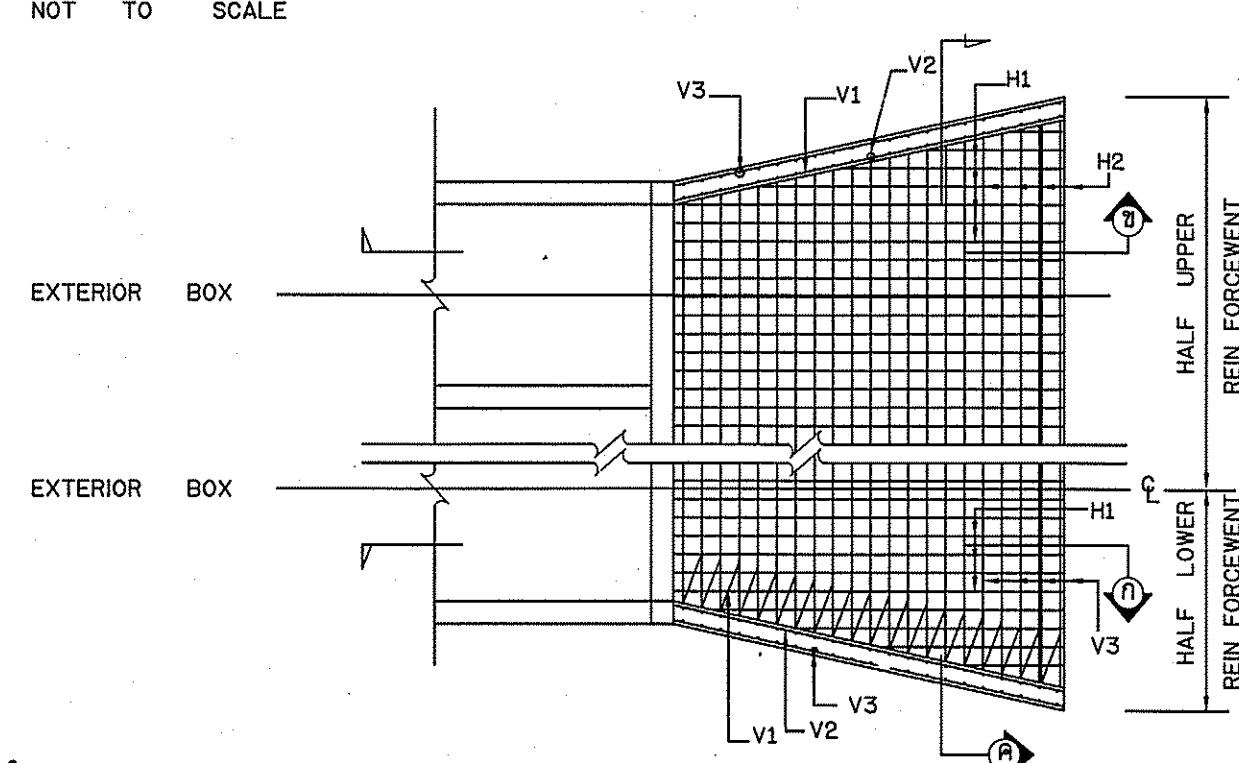
รายละเอียดสำหรับ MULTIPLE BOX NOT TO SCALE
