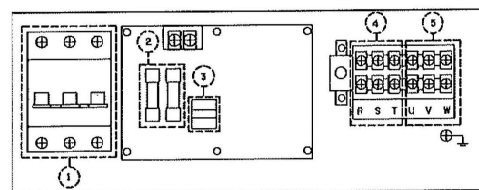
รายละเอียดตู้ควบคุมการปิด - เปิด
