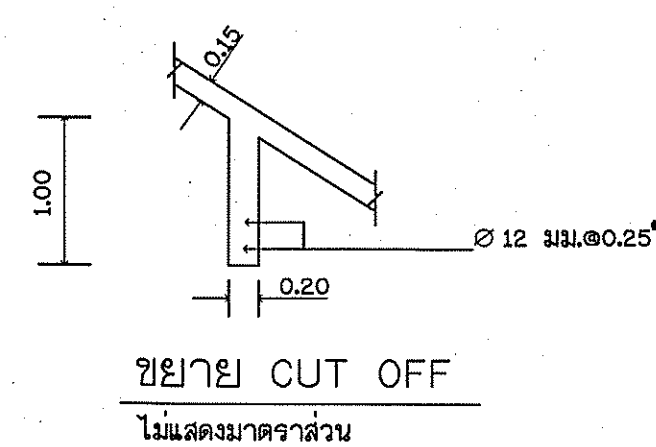
รูปตัด (ข) - (ข) (ความหนาพื้น 0.15 ม.) ไม่แสดงขนาดราส่วน
