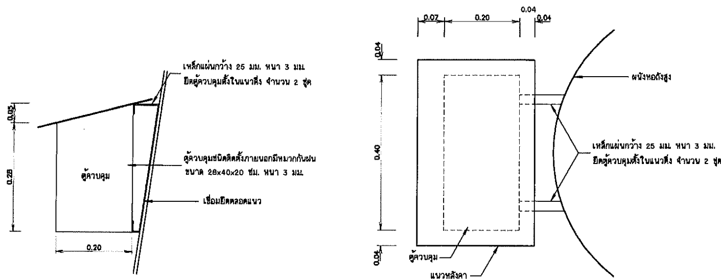
แบบขยายตัวควบคุม ไม่แสดงขนาดจั่วส่วน
