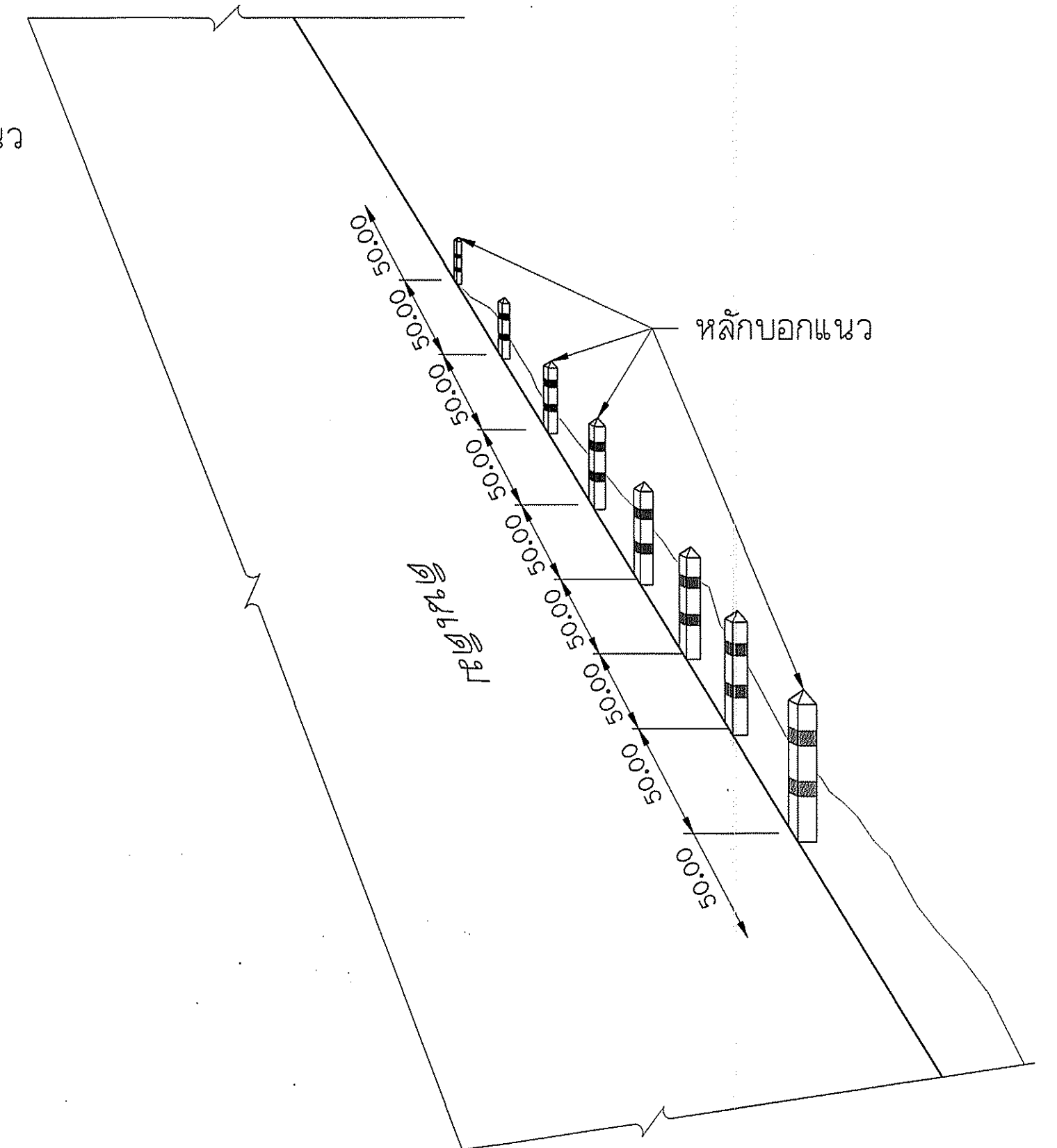
แสดงการติดตั้งหลักปักแนว NO SCALE
