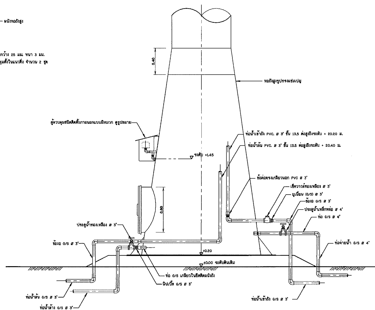
แบบแสดงการเดินท่อในท่อถึงสูง ไม่แสดงขนาดจั่วส่วน
