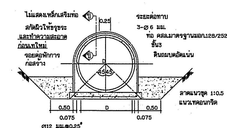
รูปตัดการวางท่อ คลส. ไม่แสดงมาตราส่วน
