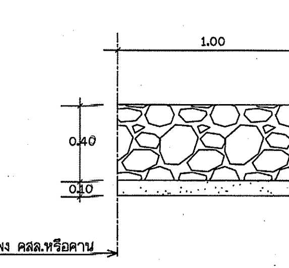
ขยายหินเรียง 2 ไม่แสดงขนาดราส่วน
