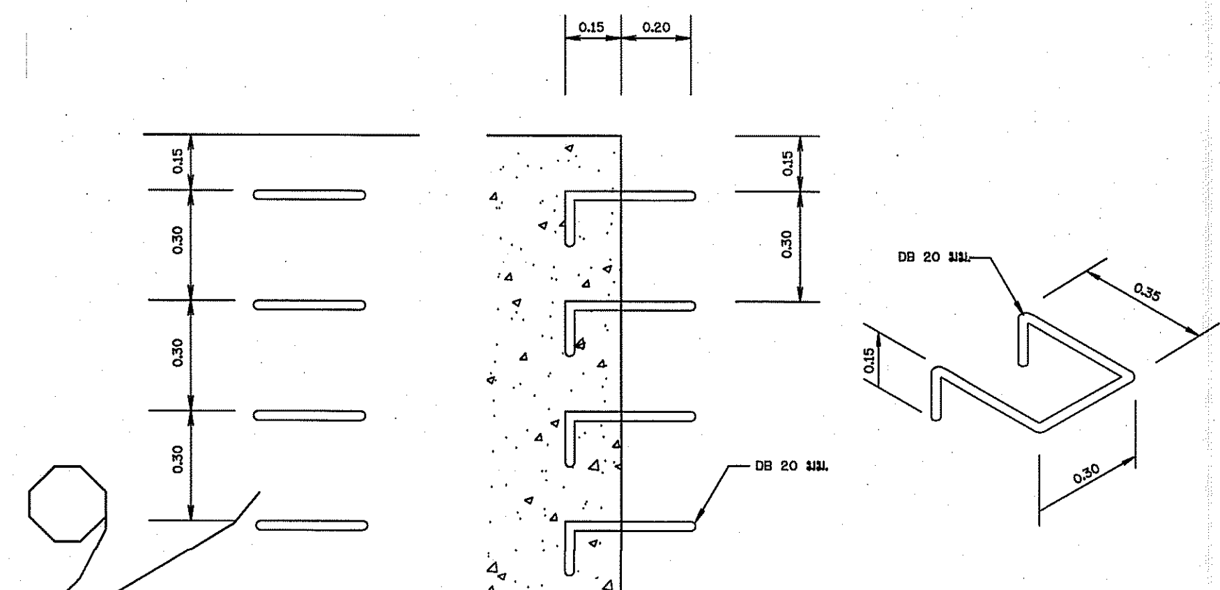
รูปขยายบันไดลิง มาตราส่วน 1:10
