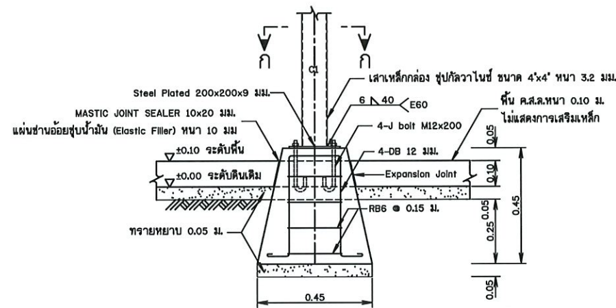
รูปขยายฐานรากโครงสร้างรับแผง F1 (ต่อม่อ ค.ส.ท. หล่อสำเร็จรูปพร้อมติดตั้ง) ไม่แสดงมาตราส่วน
