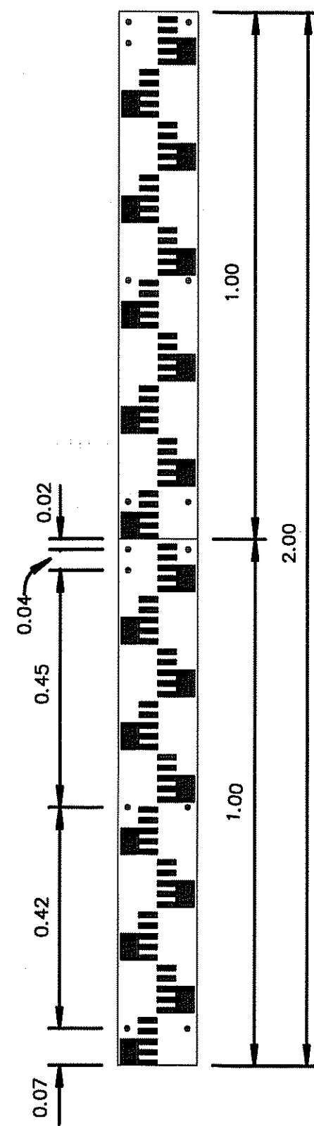
แผ่นหลักบอกค่าระดับ มาตราส่วน 1:10
