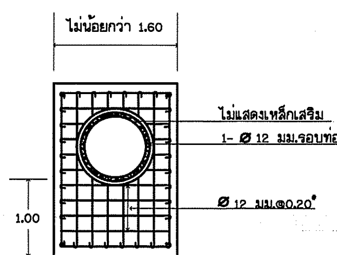
ขยายการเสริมเหล็กกำแพงปากท่อและท้ายท่อ ไม่แสดงมาตราส่วน
