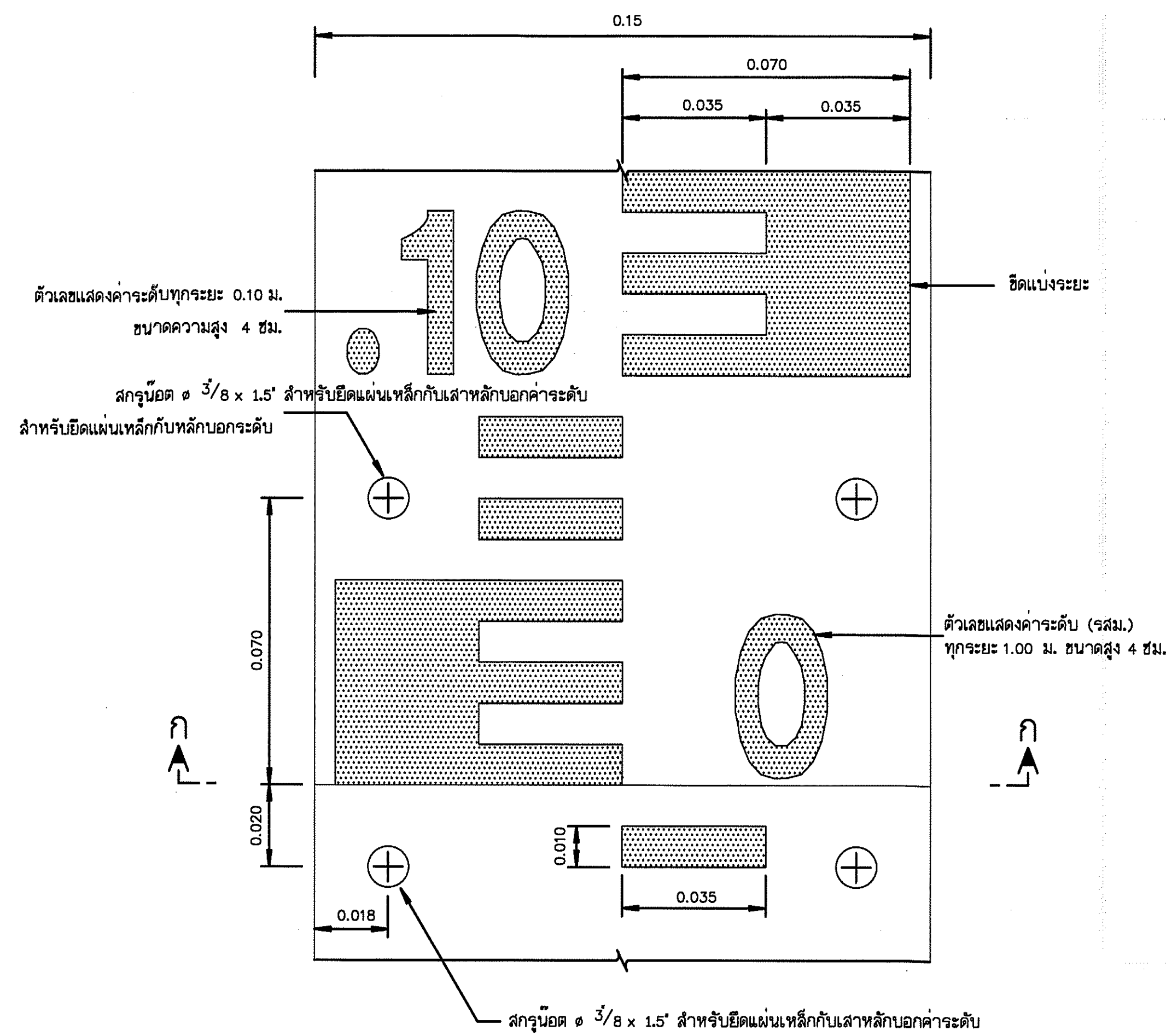
ขยายแผ่นหลักบอกค่าระดับ มาตราส่วน 1:1
