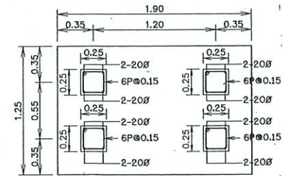
รูปตัด ๖-๖
