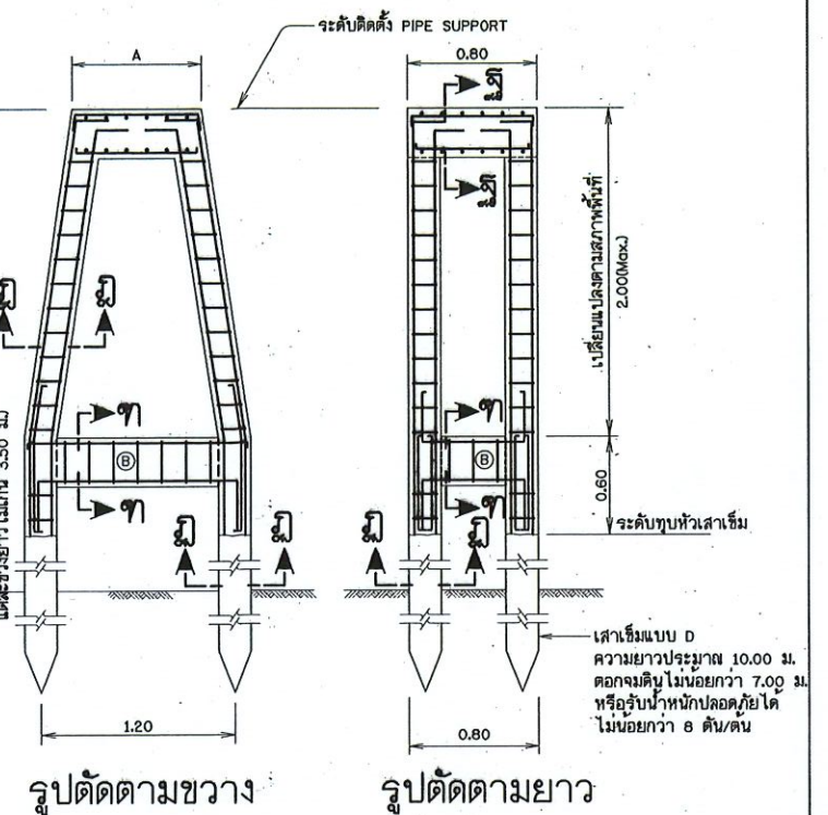
การเสริมเหล็ก คอม่อแบบที่ 4
