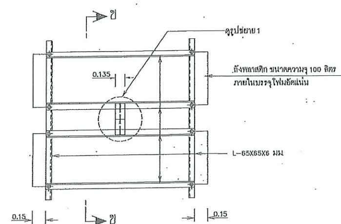
แปลน รายละเอียดท่อน้ำวางท่อข้างคาน
