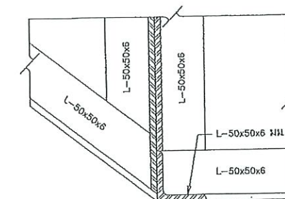
รูปตัด ข-ข มาตราส่วน 1 : 2.5
