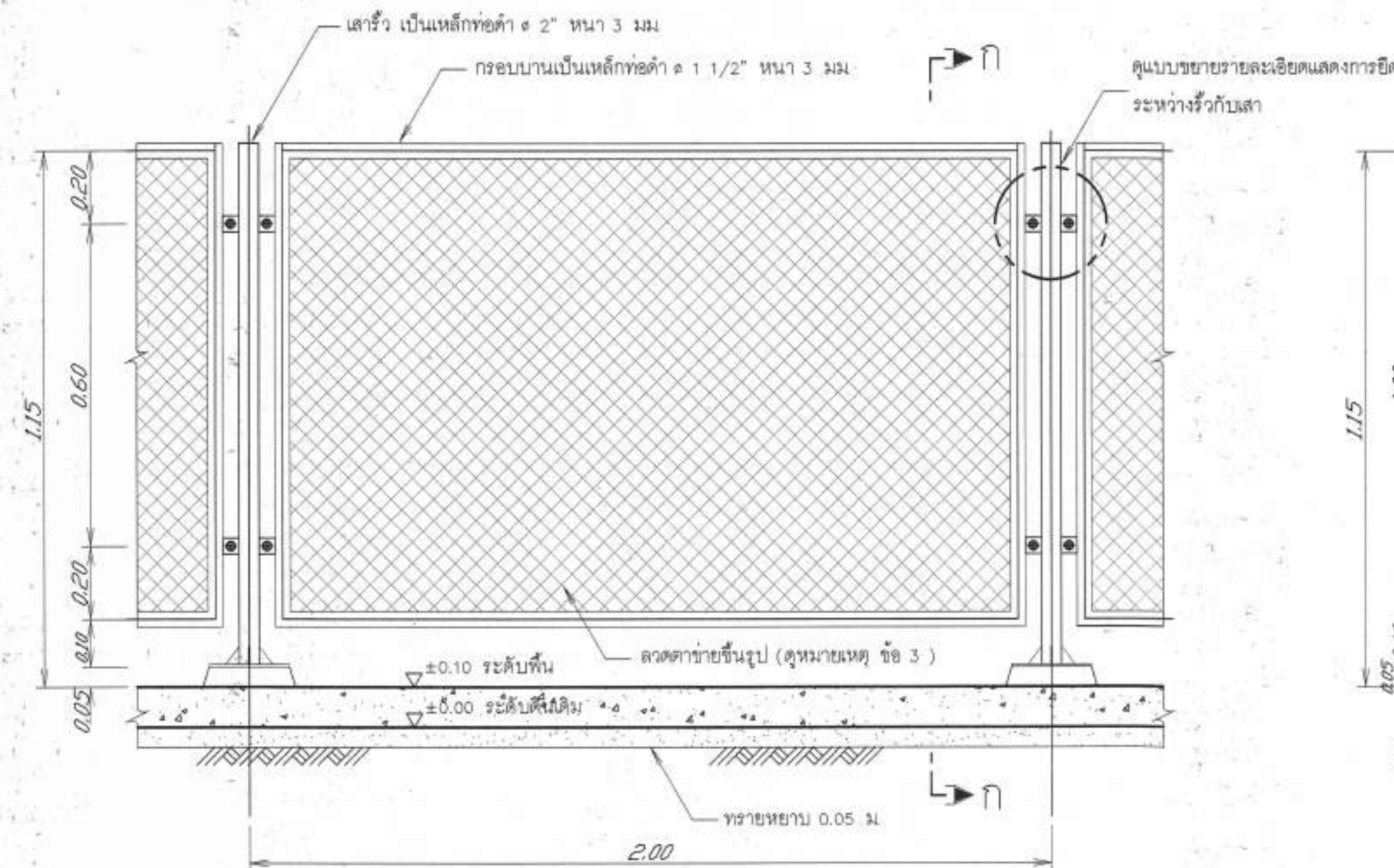
แบบขยายรูลวดตาข่าย
