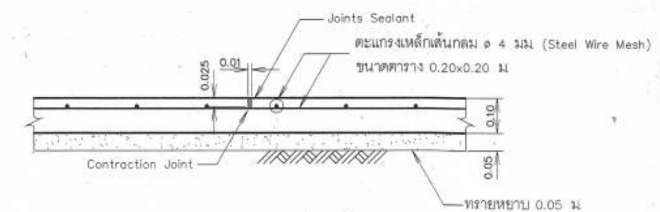
แบบขยายรอยต่อพื้น (Contraction Joint) ไว้แสดงมาตราส่วน
