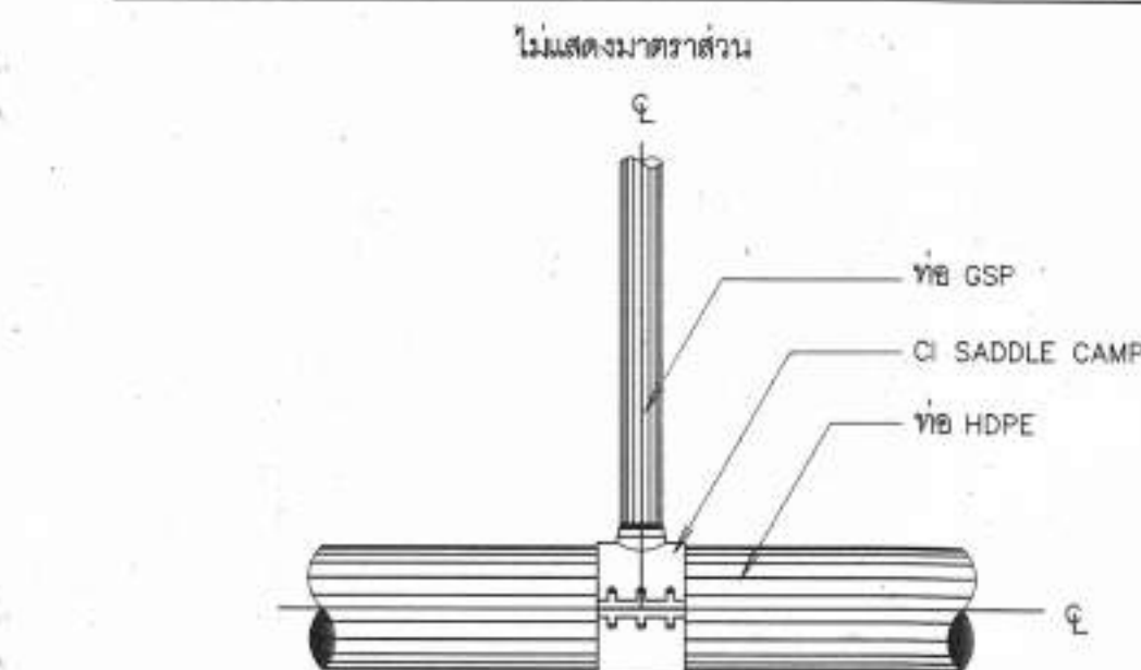
การบรรจุบ่อสามทาง HDPE กับท่อ GSP
