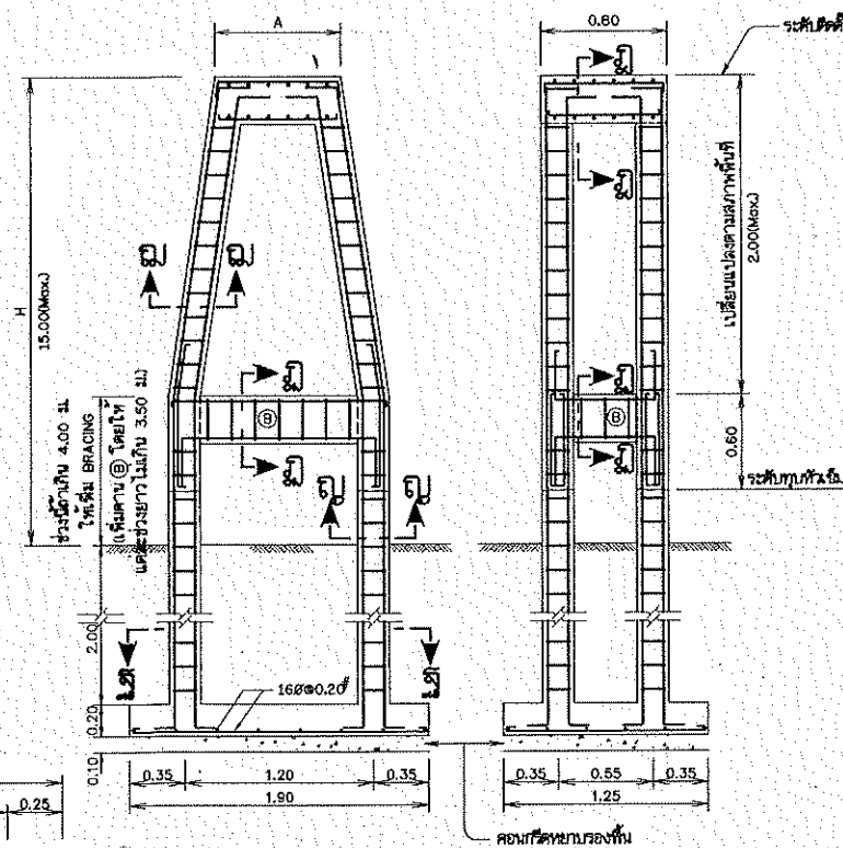
รูปตัดตามขวาง
