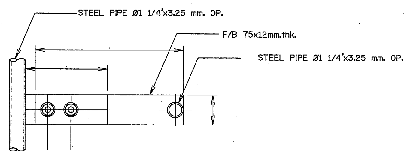
รูปตัด ง - ง มาตราส่วน 1:5
