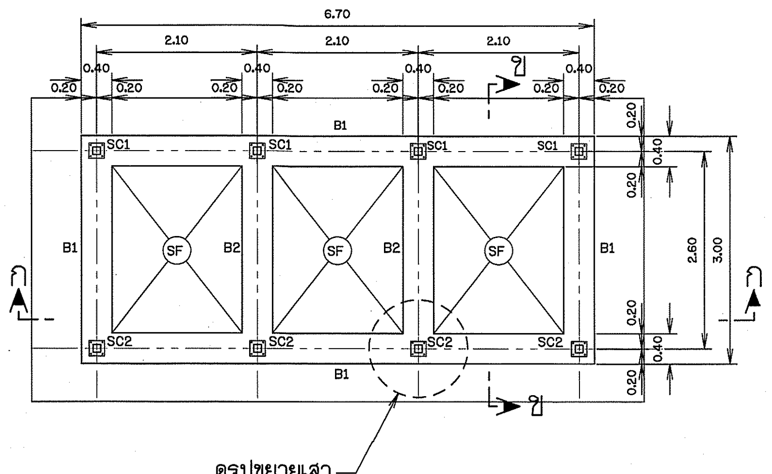
แปลนคานคอดิน มาตราส่วน 1:50
