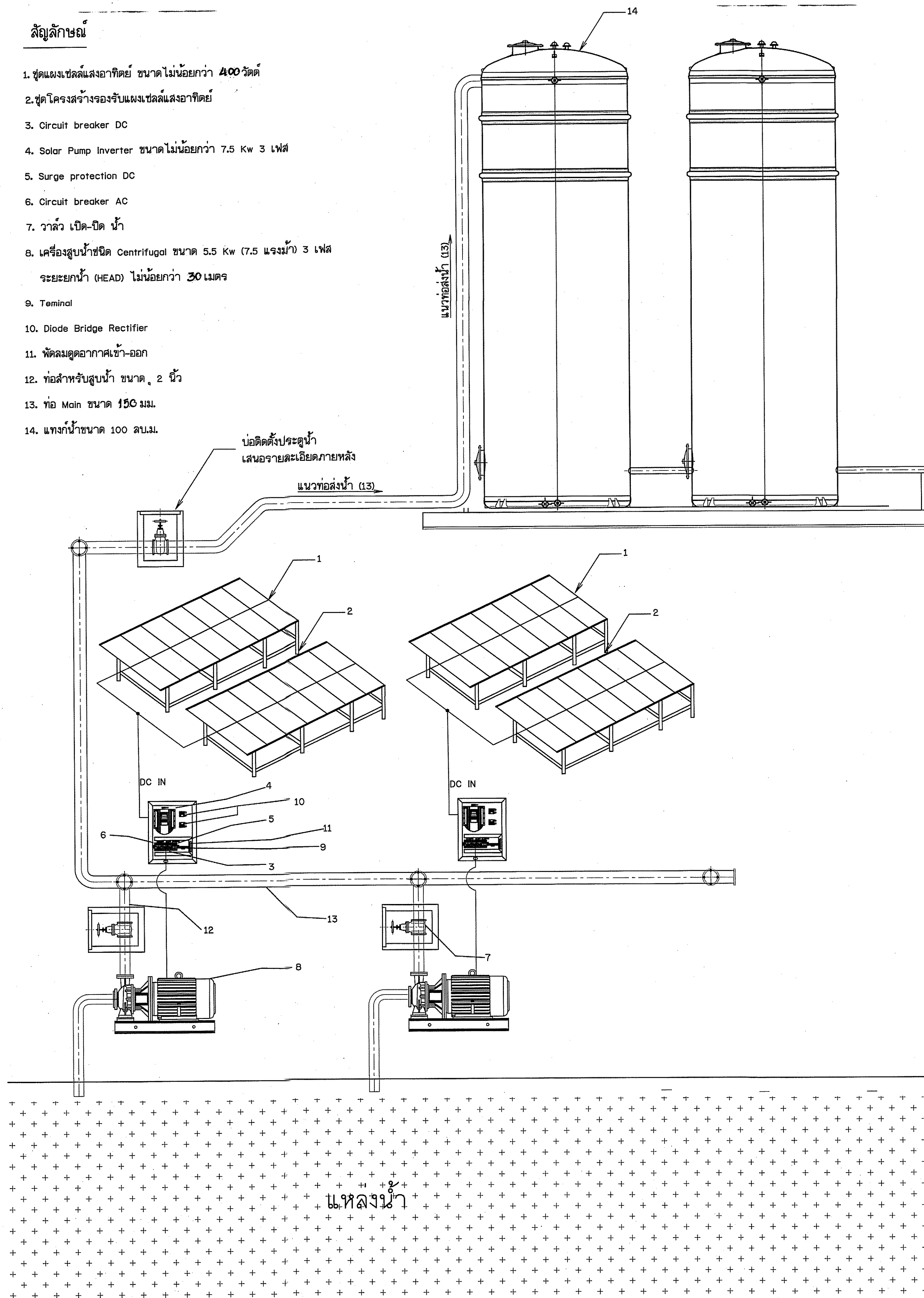
แบบระบบกระจายน้ำด้วยพลังงานแสงอาทิตย์ มาตรฐาน ไม่แสดงมาตรฐาน
