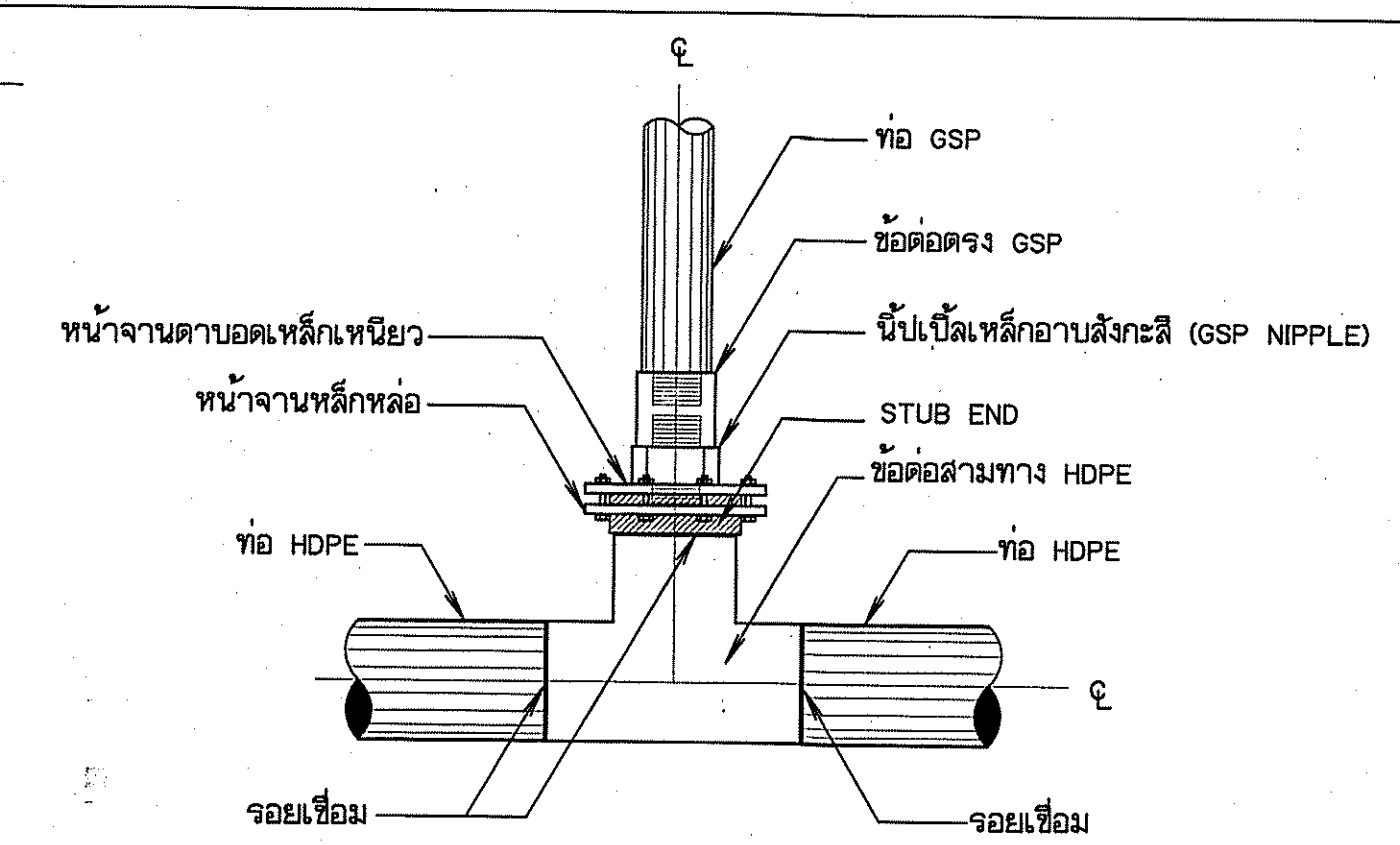
การบรรจุท่อสามทาง HDPE กับท่อ GSP แบบข้อต่อ (สำหรับอาคารจุดปล่อยน้ำ อาคารประตูประบายตะกอน อาคารท่อระบายอากาศ กรณีท่อส่งน้ำขนาดเส้นผ่าศูนย์กลางมากกว่า 315 มม.)
