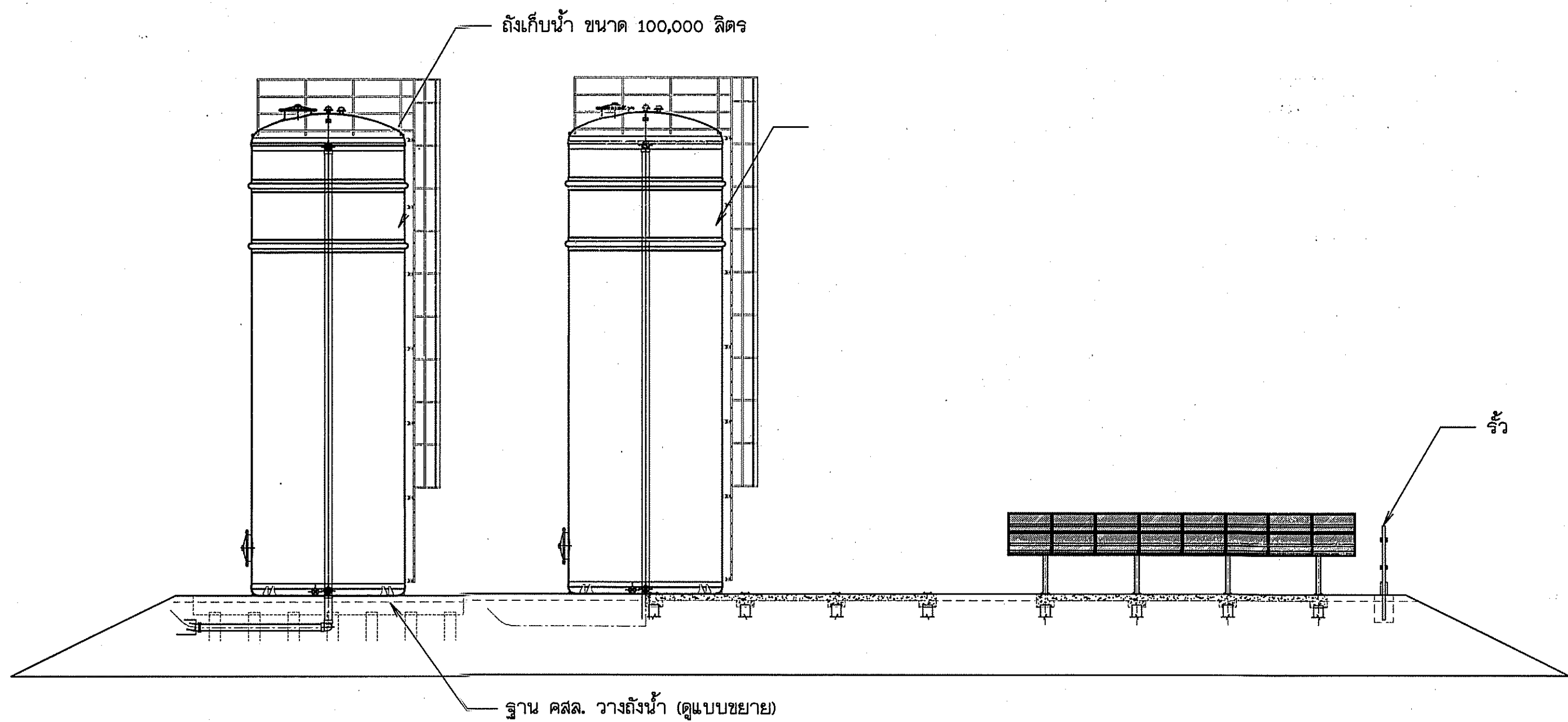
แปลนทั่วไป มาตราส่วน 1:100
