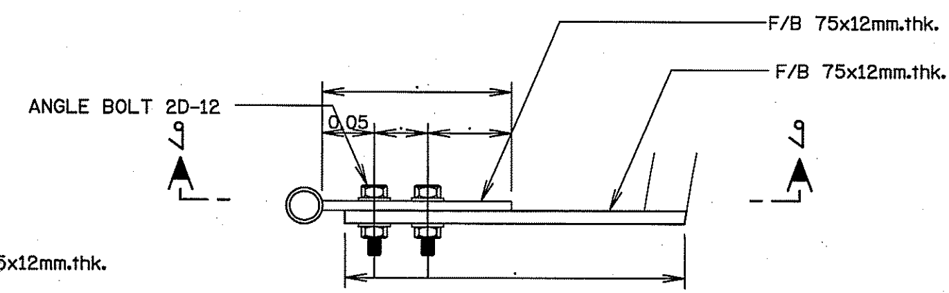
รูปตัด ก - ก มาตราส่วน 1:5
