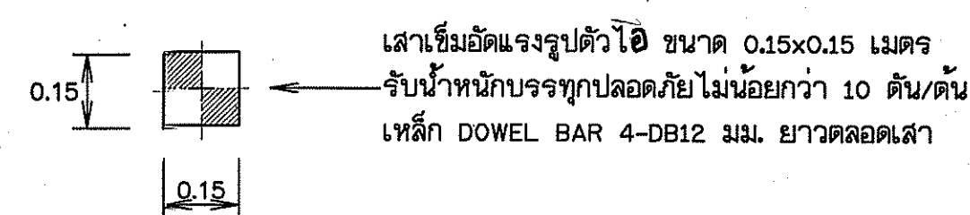
แบบขยายเสาเข็ม
