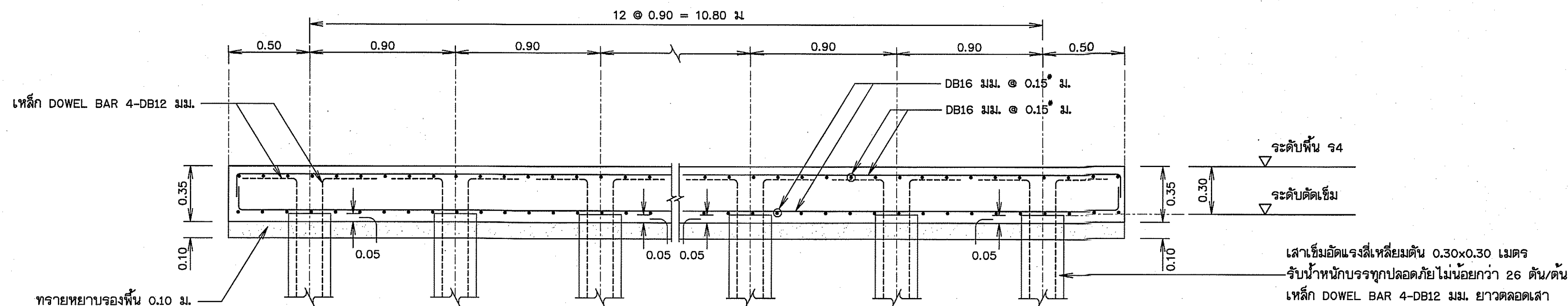
รูปตัด ก1 - ก1 มาตราส่วน 1:10
