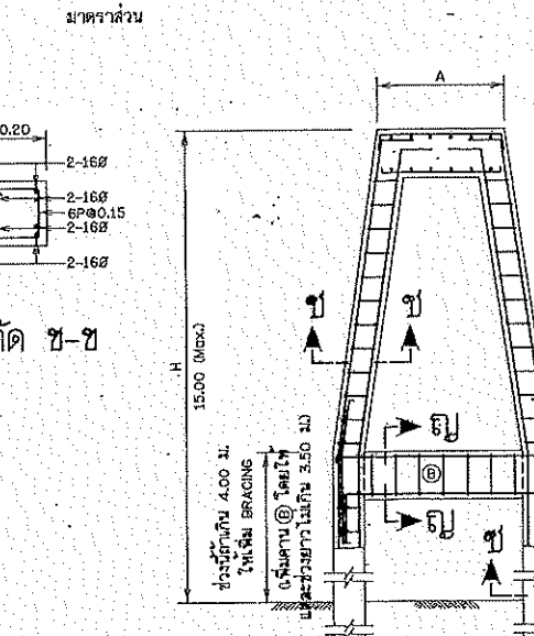
การเสริมเหล็ก คอมม่อแบบที่ 3
