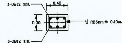
แบบขยายคาน B1 มาตราส่วน 1:40
