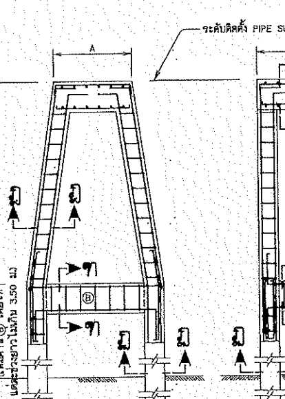
การเสริมเหล็ก คอมม่อแบบที่ 4
