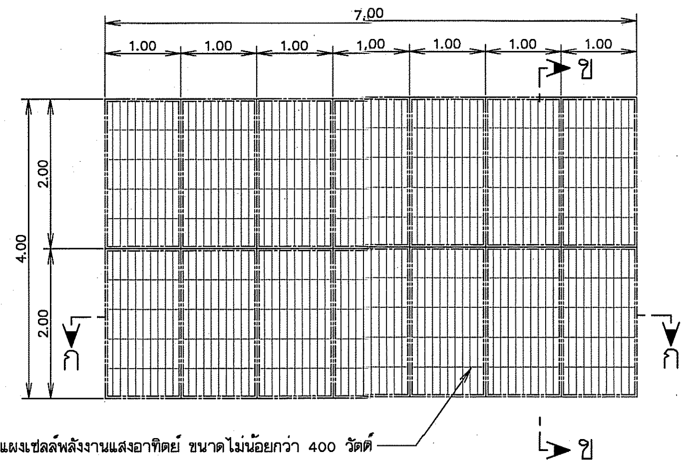
แปลนแผงเซลล์พลังงานแสงอาทิตย์ขนาดไม่น้อยกว่า 400 วัตต์ มาตราส่วน 1:50
