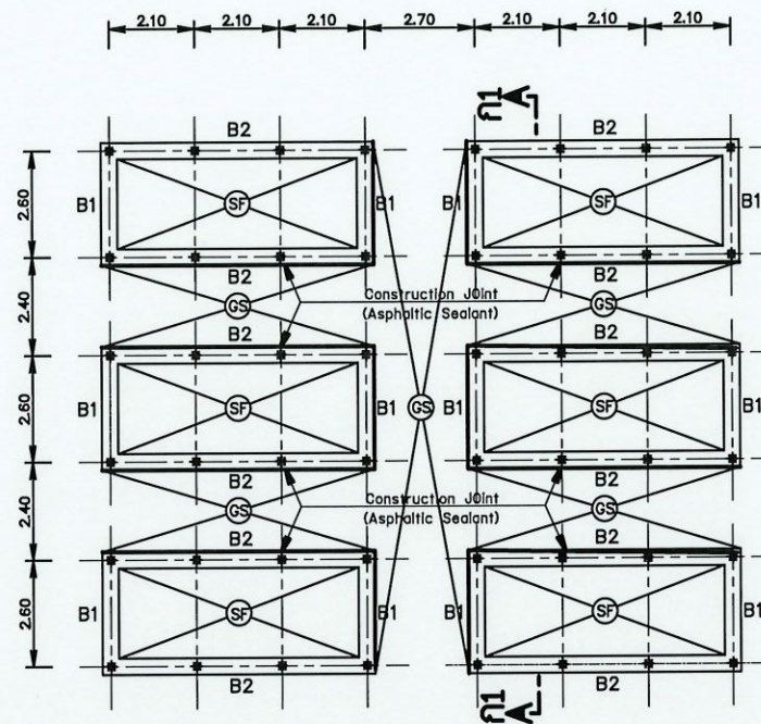
แปลนคานคอดินแผงเซลล์พลังงานแสงอาทิตย์ มาตราส่วน 1:20
