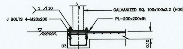
รูปตัด ก1 - ก1 มาตราส่วน 1:25
