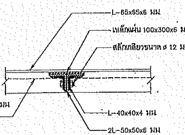
รูปตัด ค-ค
