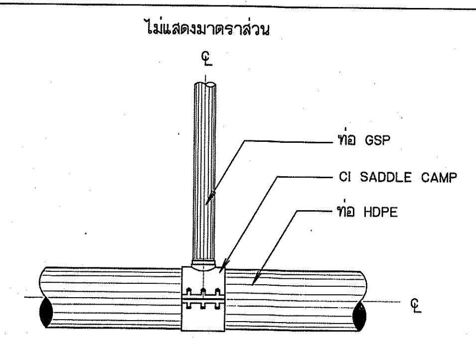
การบรรจุท่อสามทาง HDPE กับท่อ GSP แบบ CI SADDLE CLAMP (สำหรับอาคารจุดปล่อยน้ำ อาคารประตูประบายตะกอน อาคารท่อระบายอากาศ กรณีท่อส่งน้ำขนาดเส้นผ่าศูนย์กลางน้อยกว่าหรือเท่ากับ 315 มม.)
