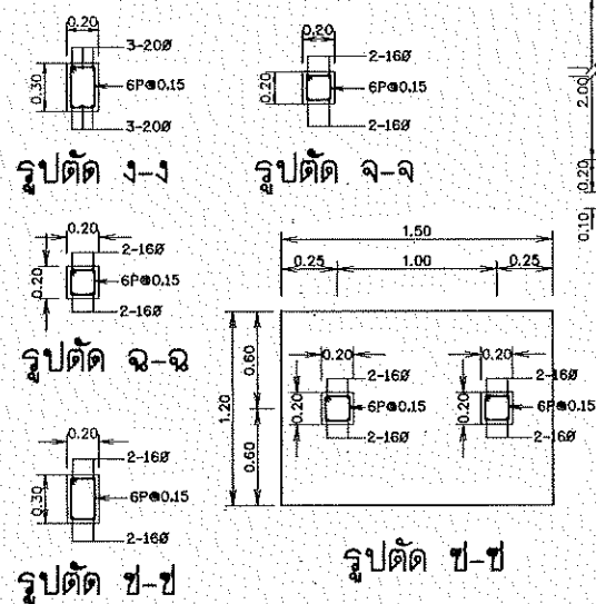
รูปตัดตามขวาง
