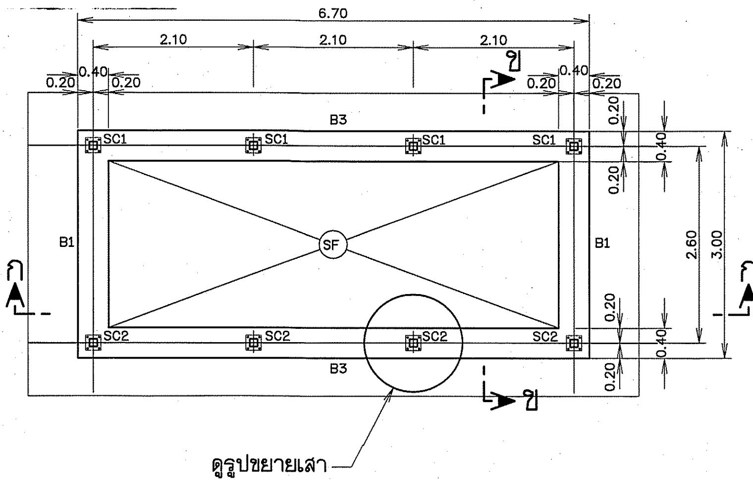
แปลนคานาคอนกรีต
