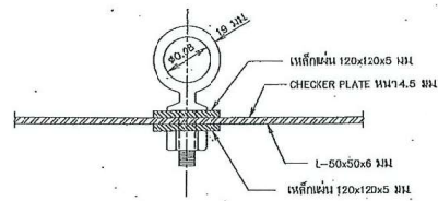
รูปขยายห้วงยึดแป้นน้ำ
