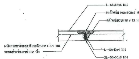
รูปตัด ค-ค
