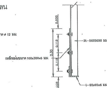
รูปตัด ข-ข
