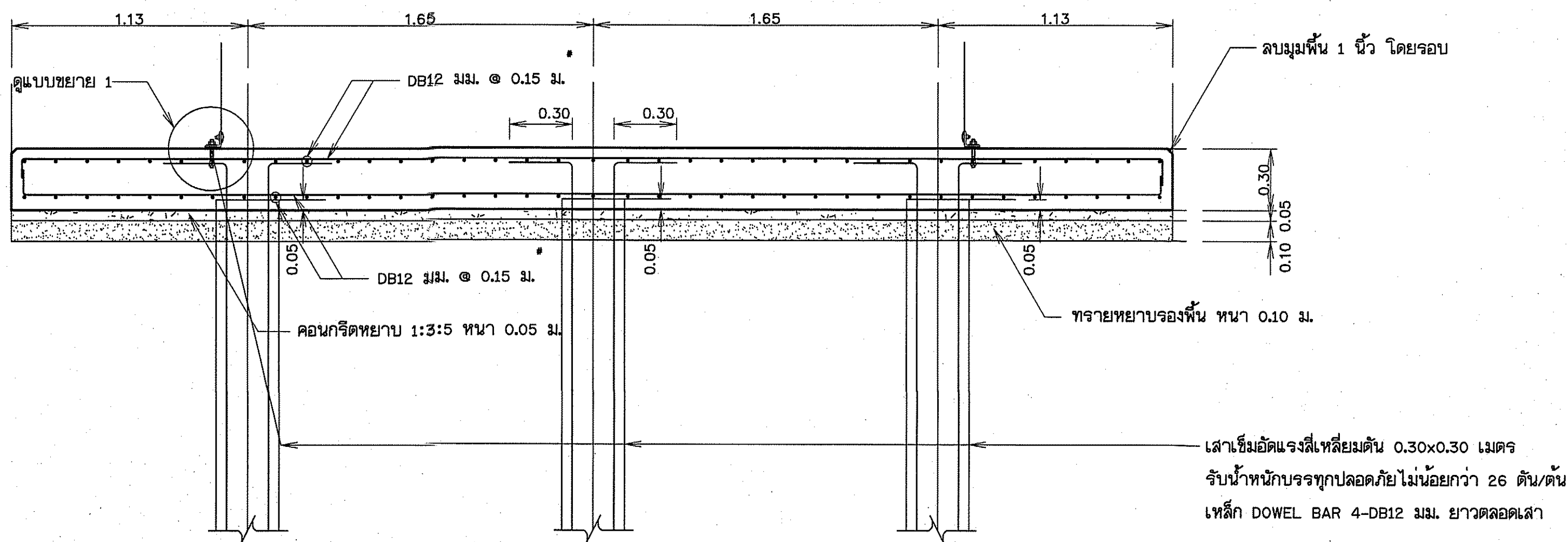
รูปตัด ก - ก
