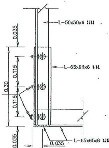
รูปตัด ก-ก
