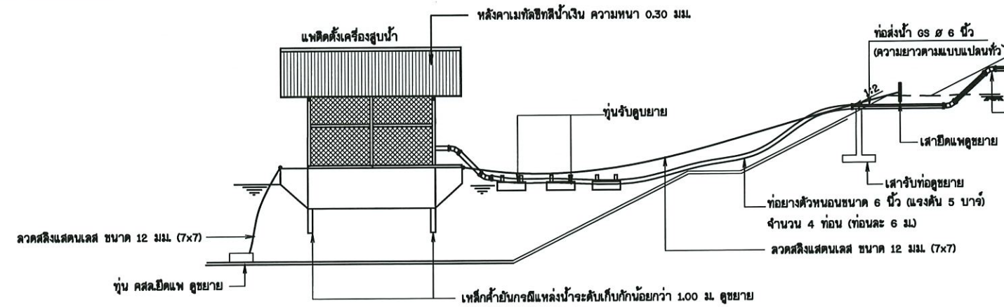
ขยายเหล็กค้ำยันแพลอยน้ำ
