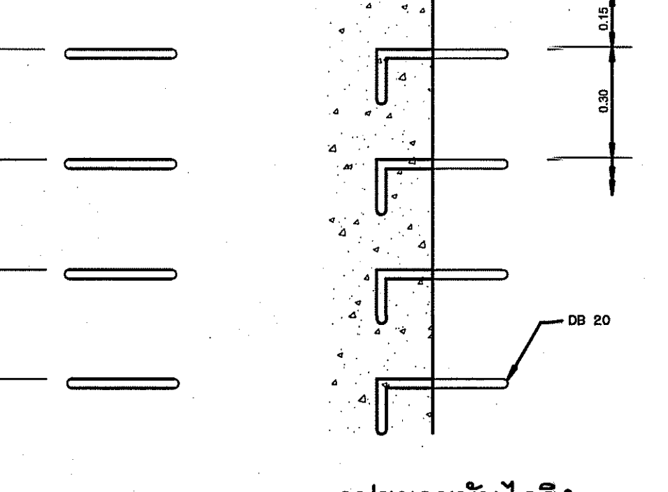
รูปขยายบันไดลิง ไม่แสดงขนาดราส่วน
