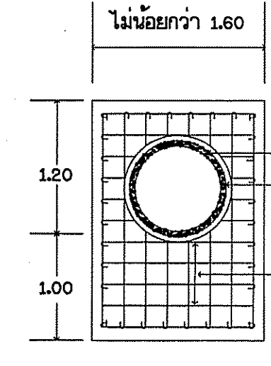
ขยายการเสริมเหล็กกำแพงปากท่อและท้ายท่อ (HEAD WALLS) ไม่แสดงขนาดราส่วน
