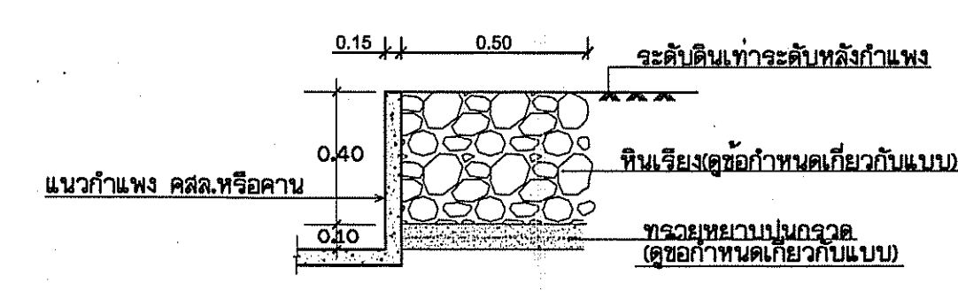
ขยายหินเรียง 1 ไม่แสดงขนาดราส่วน
