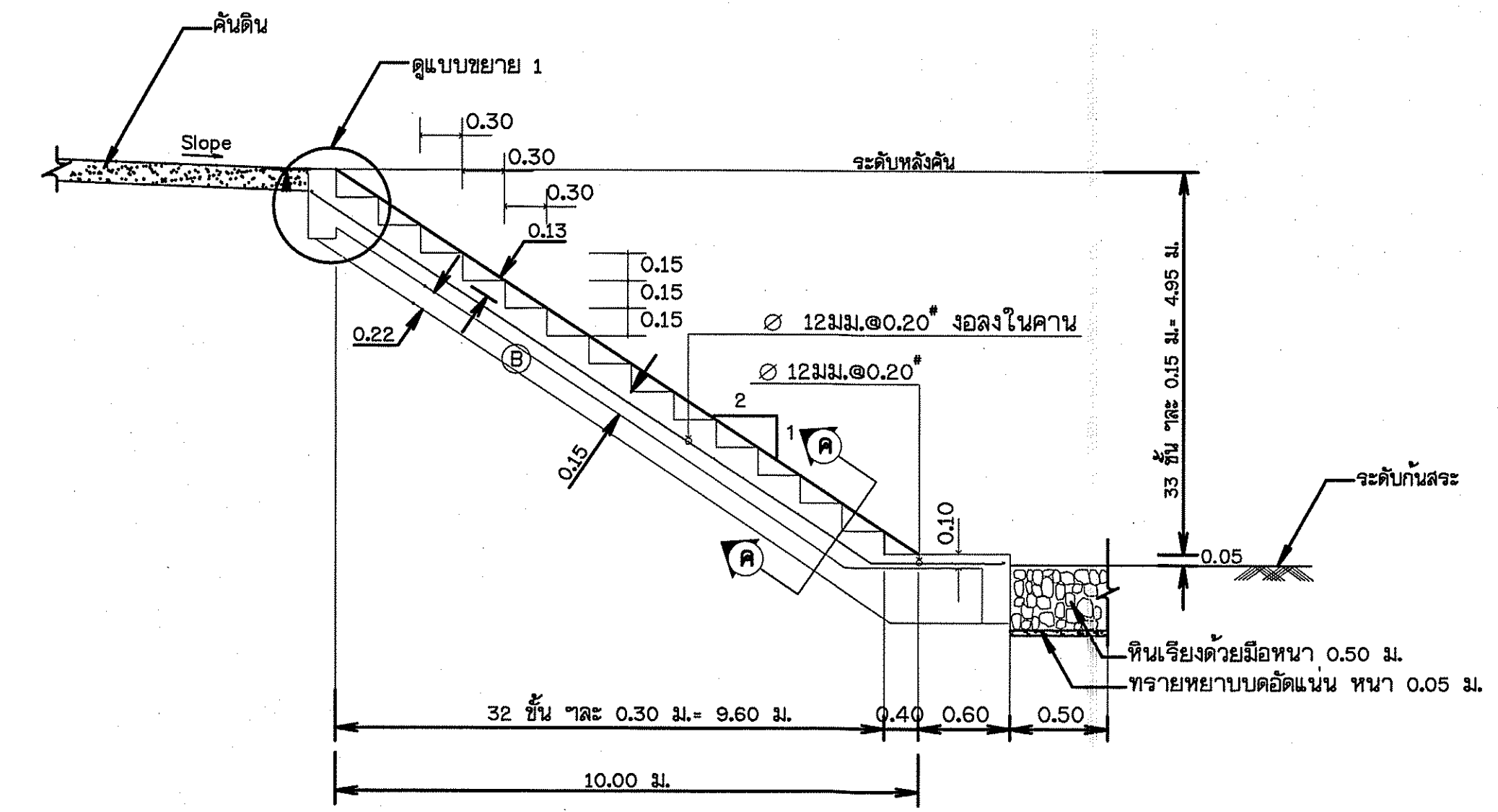
รูปตัด ข - ข ไม่แสดงขนาดราส่วน
