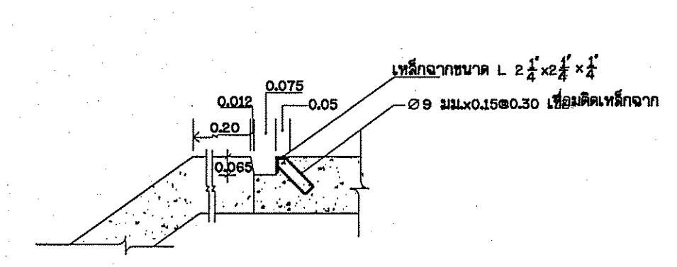
ขยายร่องไสบานประตูไม้ ไม่แสดงขนาดราส่วน
