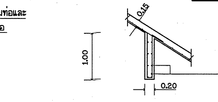
ขยาย CUT OFF ไม่แสดงขนาดราส่วน
