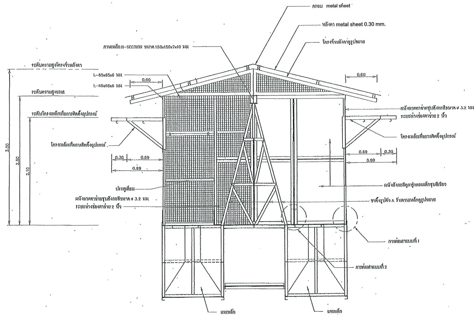
รูปตัด ก - ก (ใช้แสดงฐานรองรับเครื่องสูบน้ำ) มาตราส่วน 1 : 20
