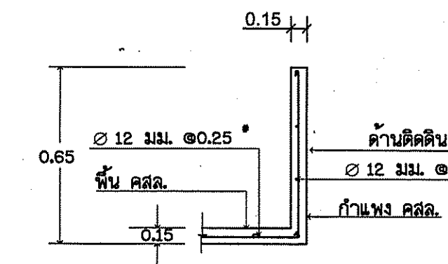
รูปตัด ๑-๑ (ความหนาพื้น ๐.๑๕ มม) ไม่แสดงขนาดราส่วน
