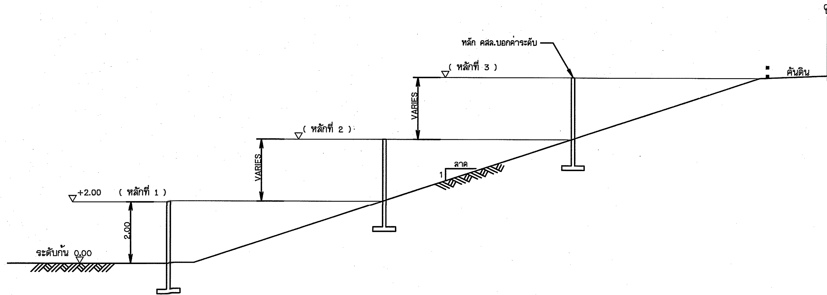
รูปตัดทัว ไปแสดงตำแหน่งหลักบอกระดับน้ำ
