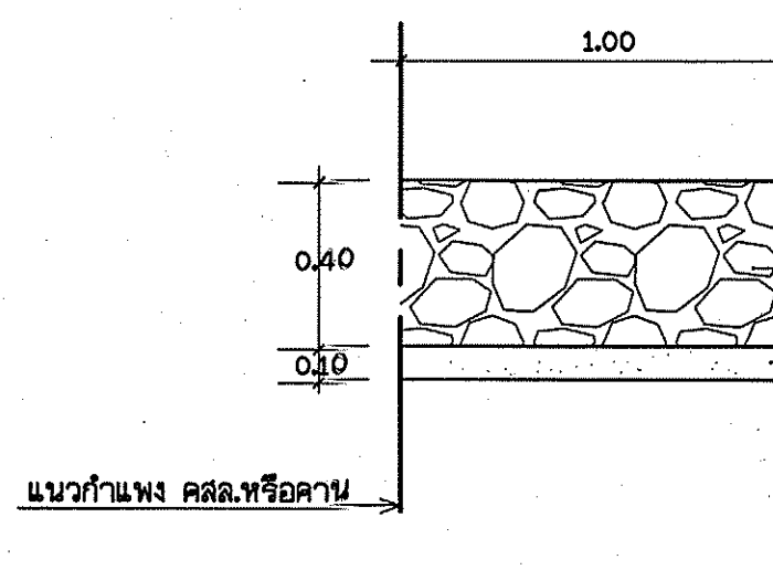
ขยายหินเรียง 2 ไม่แสดงขนาดราส่วน
