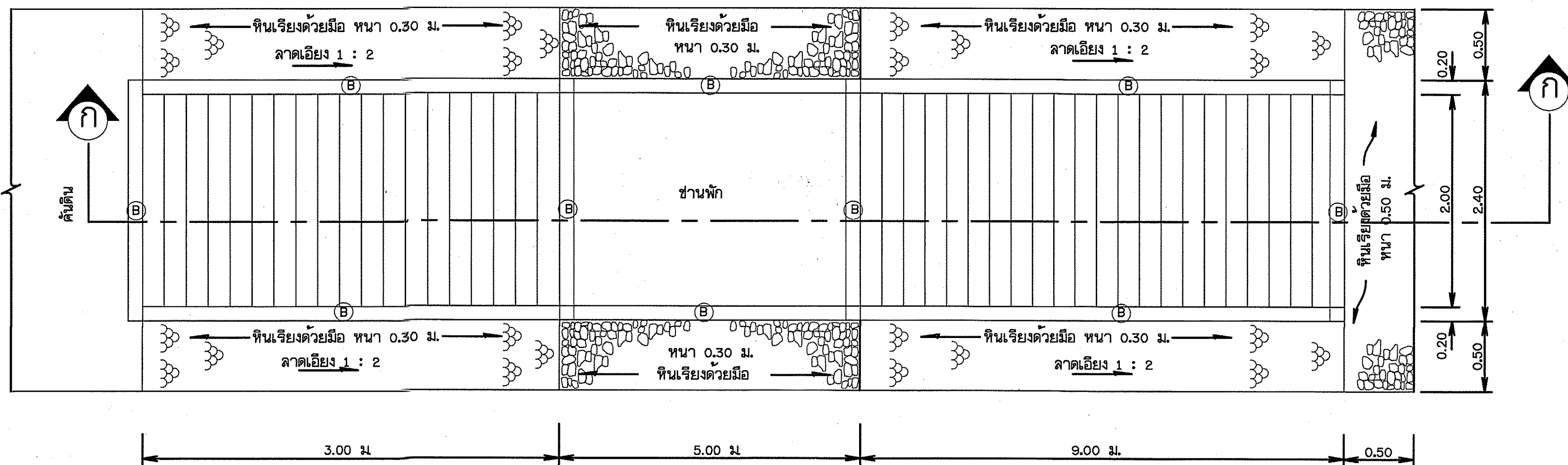
แปลนบันได คสล. แบบมีชานพัก ไม่แสดงขนาดราส่วน
