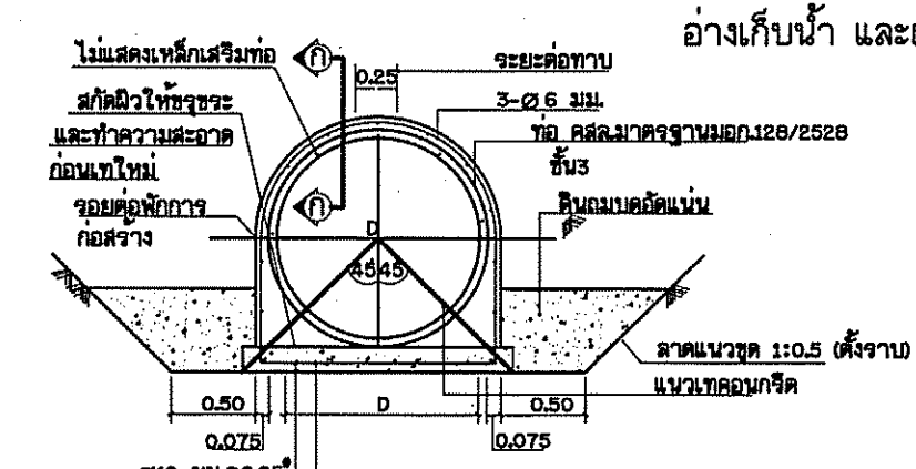
รูปตัดการวางท่อ คสล. ไม่แสดงขนาดราส่วน
