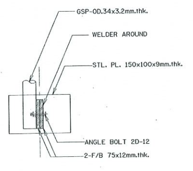
รูปตัด ค - ค มาตราส่วน 1:5
