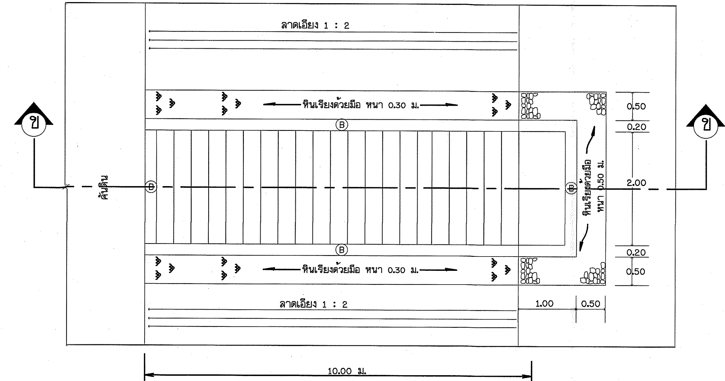
แปลนบันได คสล. แบบไม่มีชานพัก ไม่แสดงขนาดราส่วน
