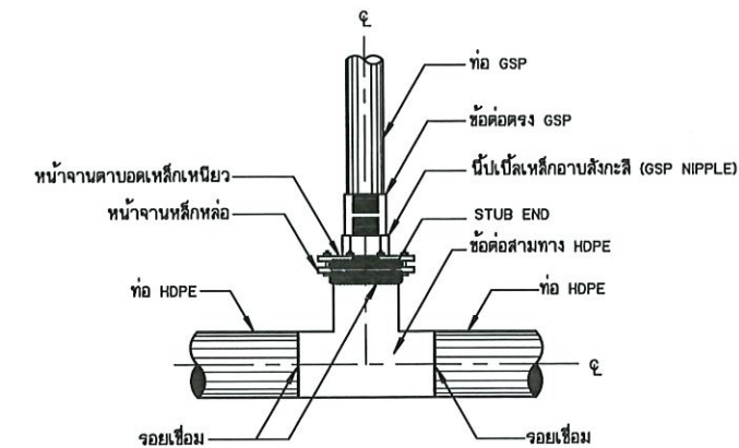
การบรรจุท่อสามทาง HDPE กับท่อ GSP แบบข้อต่อ (สำหรับอาคารจุดปล่อยน้ำ อาคารประจําขยะบดก่อน อาคารท่อระบายอากาศ กรณีท่อส่งน้ำขนาดเส้นผ่าศูนย์กลางมากกว่า 315 มม.)
