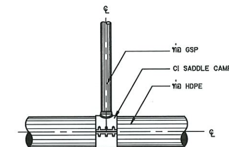
การบรรจุท่อสามทาง HDPE กับท่อ GSP แบบ CI SADDLE CLAMP (สำหรับอาคารจุดปล่อยน้ำ อาคารประจําขยะบดก่อน อาคารท่อระบายอากาศ กรณีท่อส่งน้ำขนาดเส้นผ่าศูนย์กลางน้อยกว่าหรือเท่ากับ 315 มม.)
