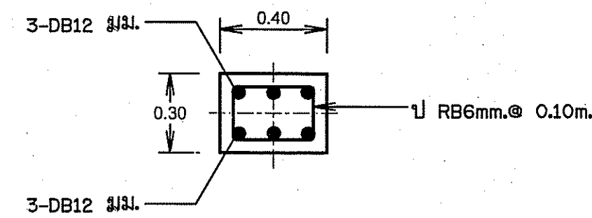
แบบขยายคาน B1
