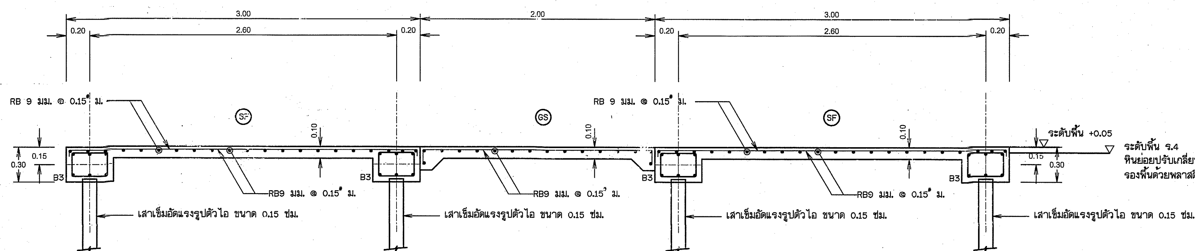
รูปตัด ก1 - ก1
