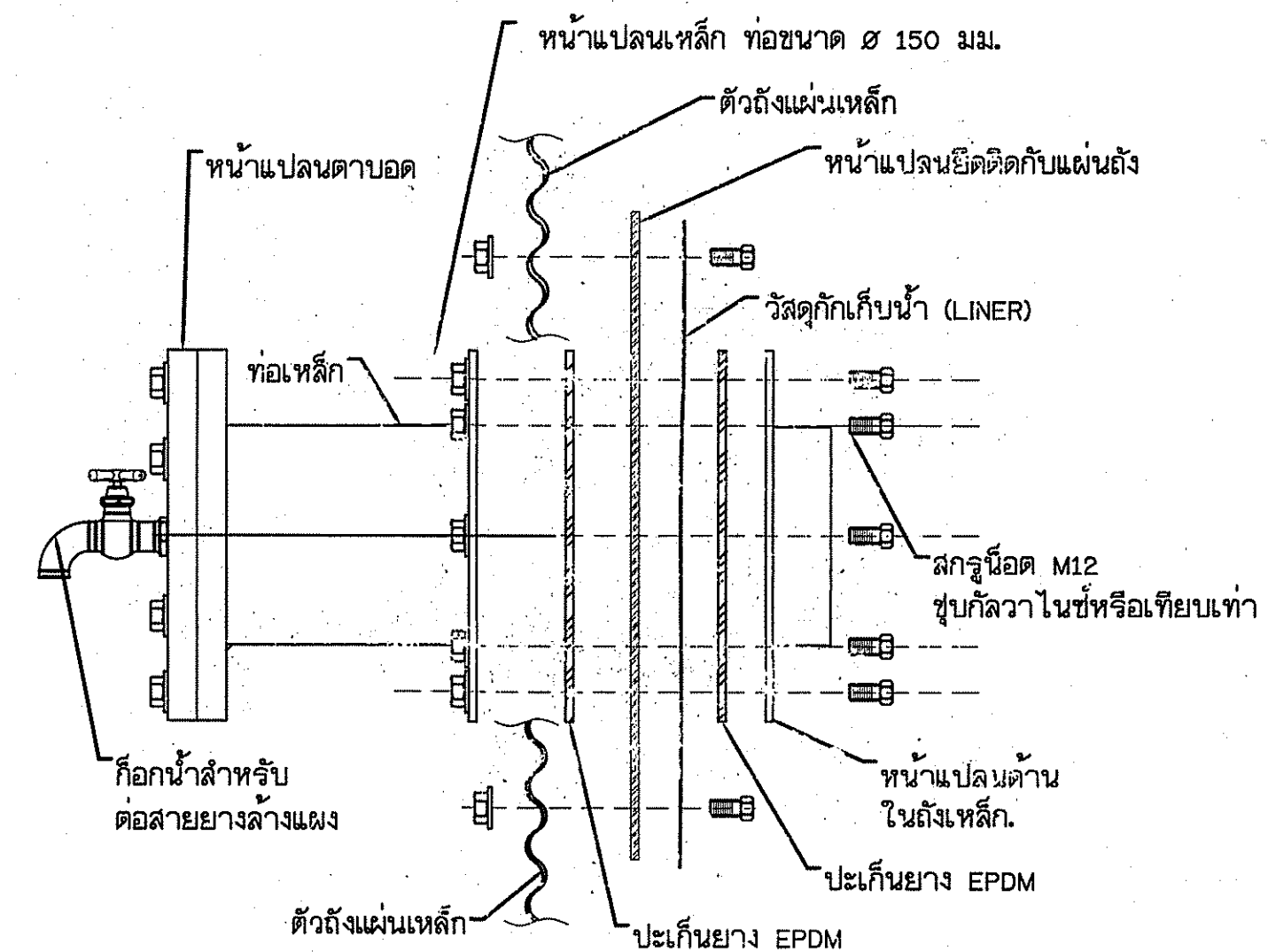
แบบขยายหน้าแปลนดาดบอด Scale NTC.
