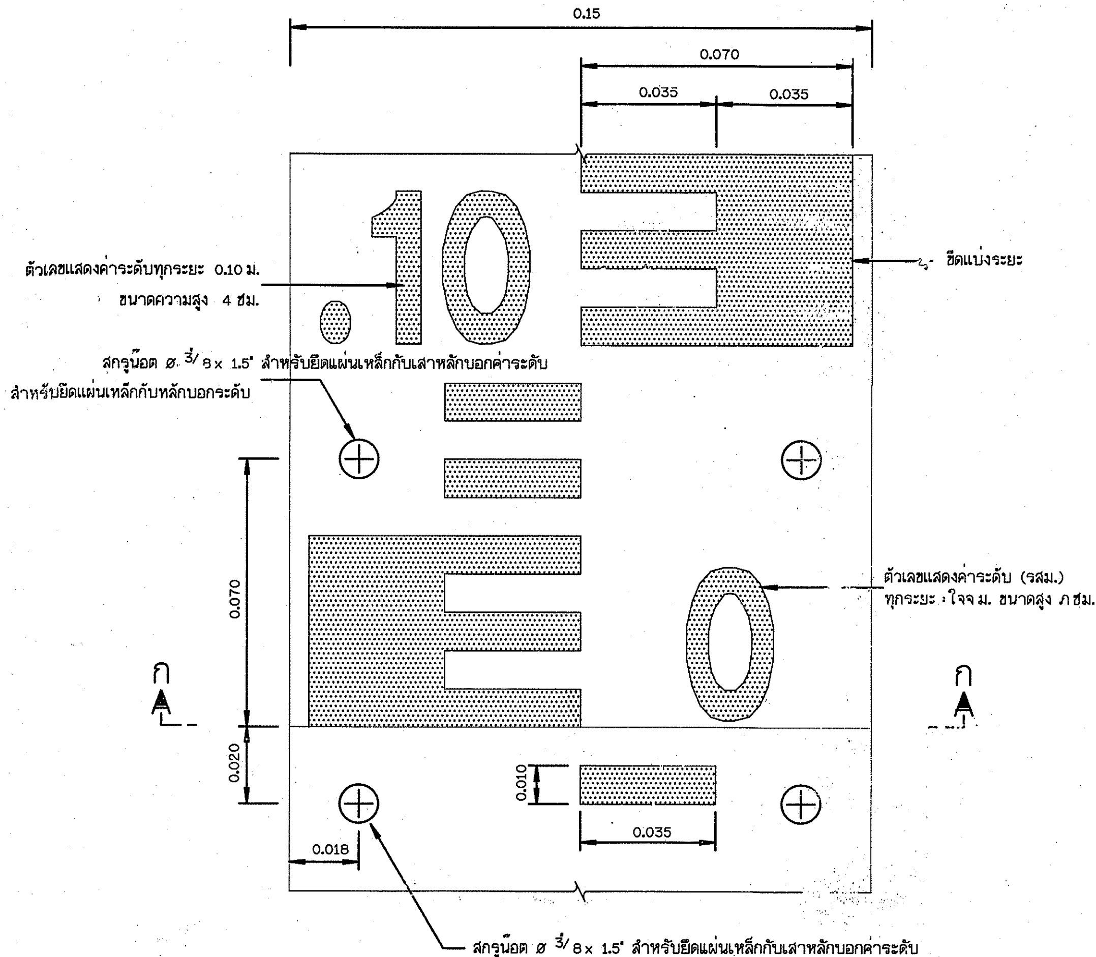
ขยายแผ่นเหล็กบอการค้าระดับ
