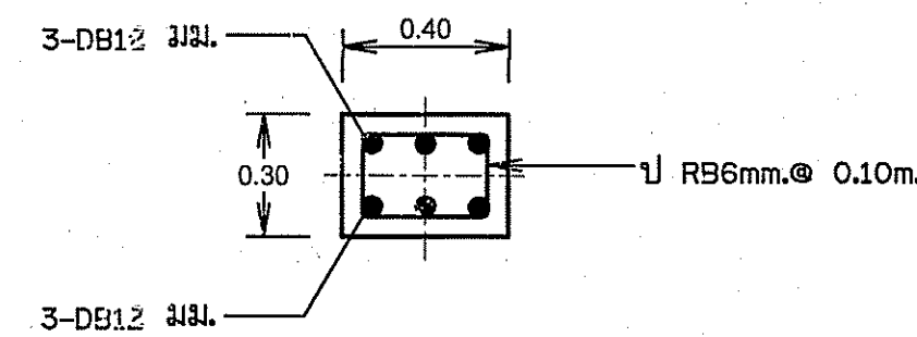
แบบขยายคาน B2
