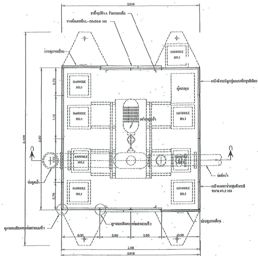
แปลนพื้น มาตราส่วน 1 : 20
