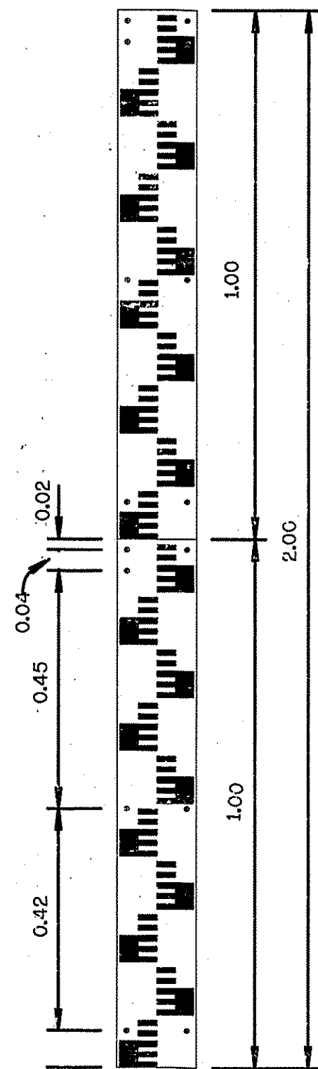
แผ่นเหล็กบอการค้าระดับ
