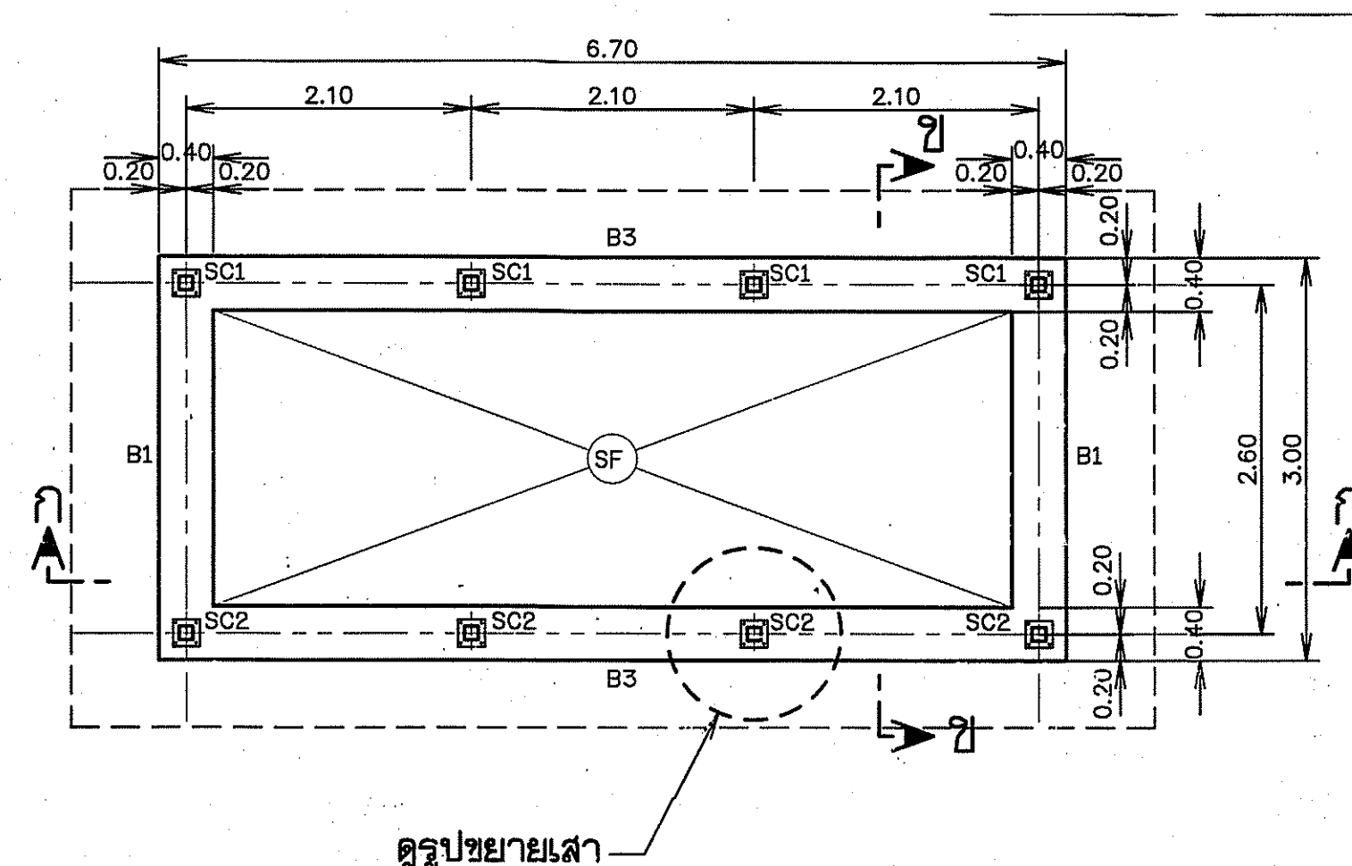
แปลนคานาคอนดิน มาตราส่วน ไม่แสดงมาตราส่วน
